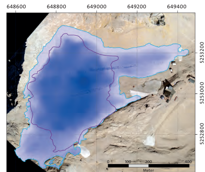
Eisdicken 2009 in m Das Maximum der Eisdicke lag 2009 noch bei etwa 50 m. Die blaue Linie zeigt die Umrisslinie des Gletschers im Jahr 2009, die violette im Jahr 2018.
