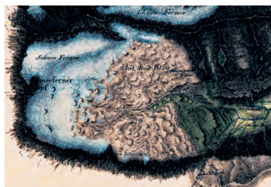
Nicht maßstabsgetreue Darstellung (1826) der ersten Vermessung des Zugspitzplatts von 1820 bis 1825.
