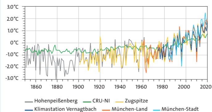
Änderung der Jahresmitteltemperatur relativ zum Mittelwert 1981–2010
