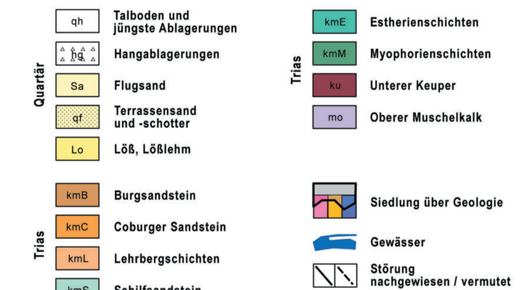
Geologische Karte der Umgebung von Ziegelanger
