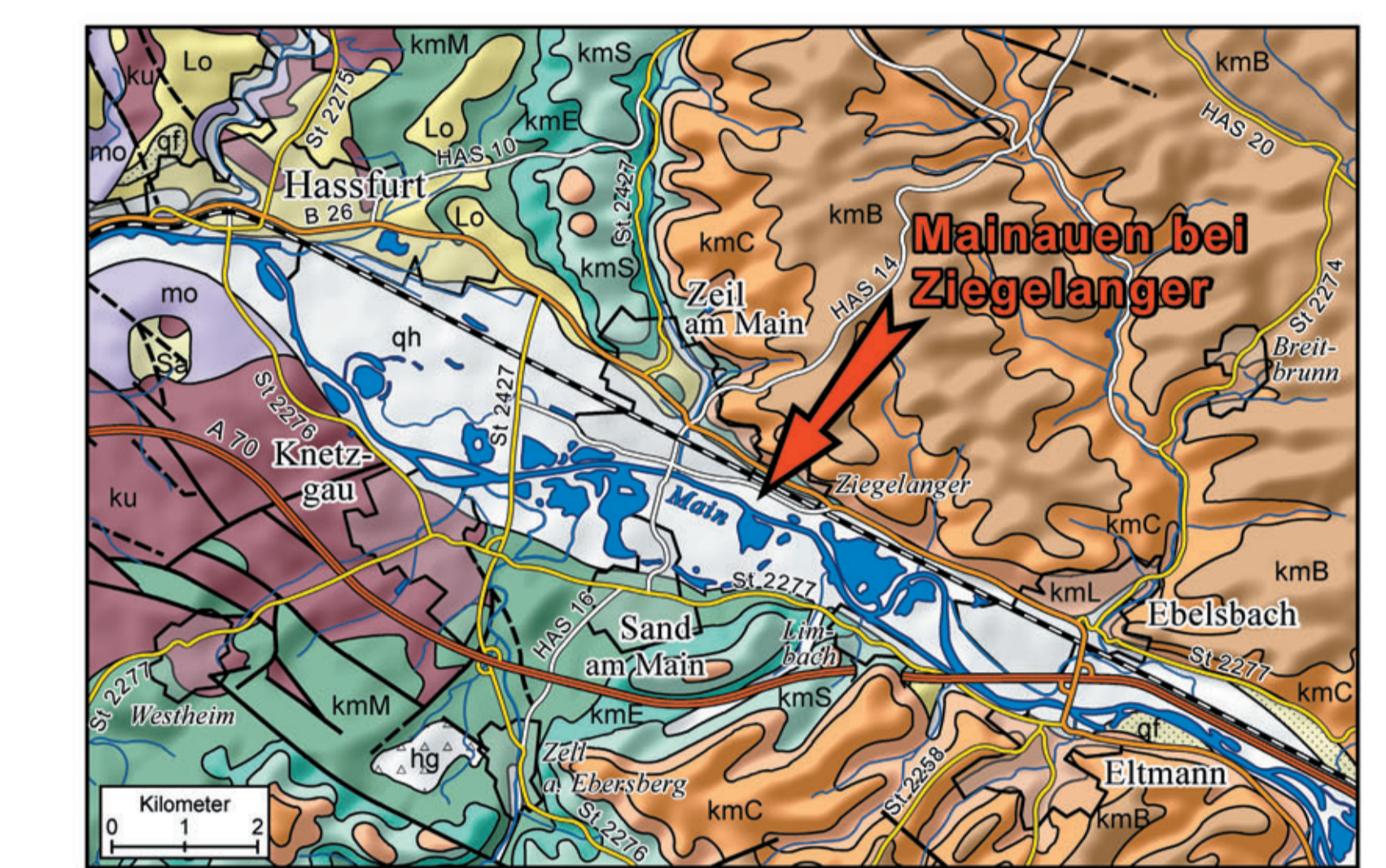
Geologische Karte der Umgebung von Ziegelanger
