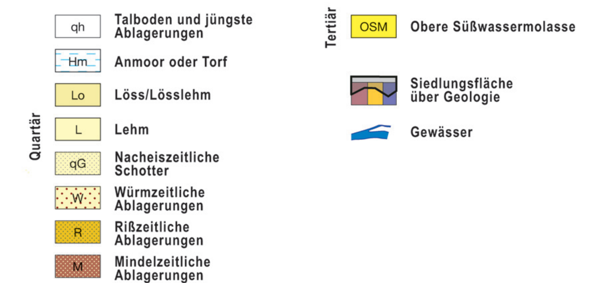
Geologische Karte der Umgebung von Aubenham
