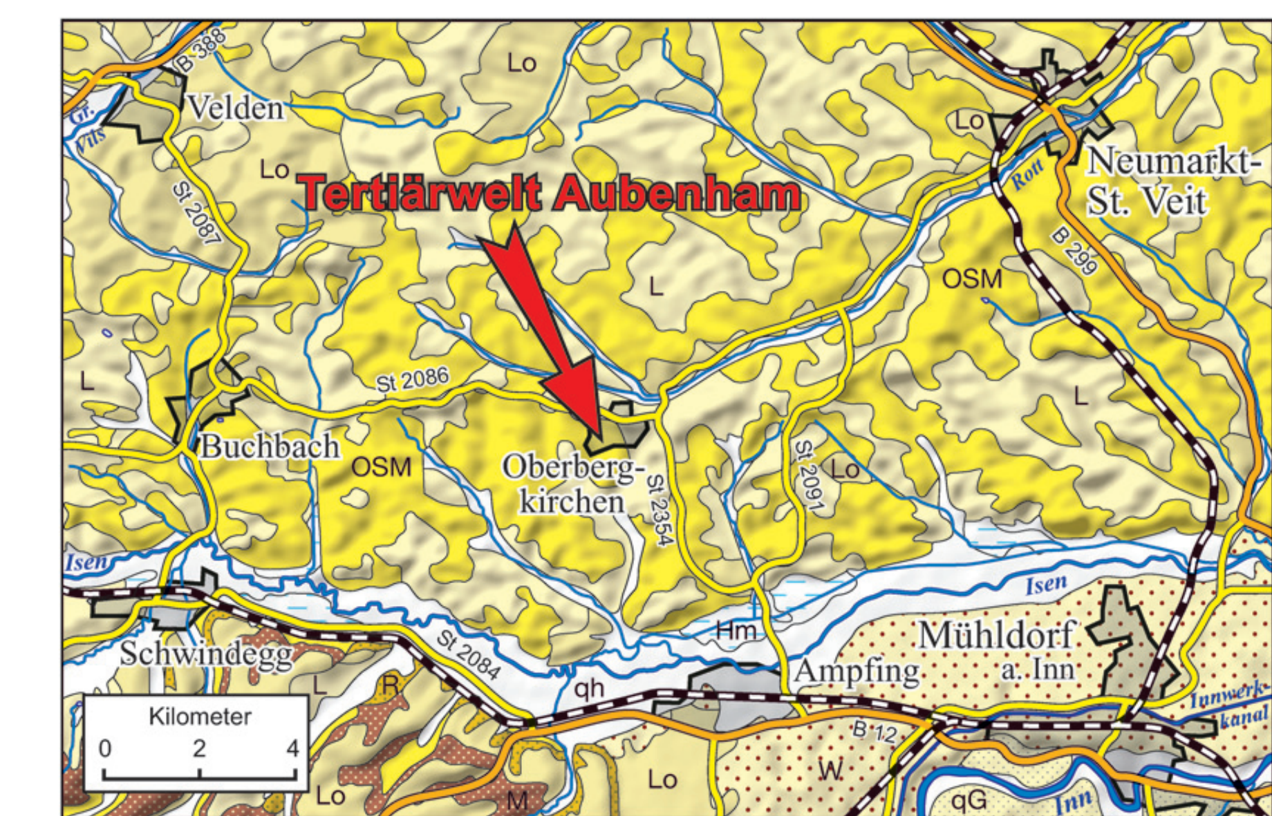
Geologische Karte der Umgebung von Aubenham
