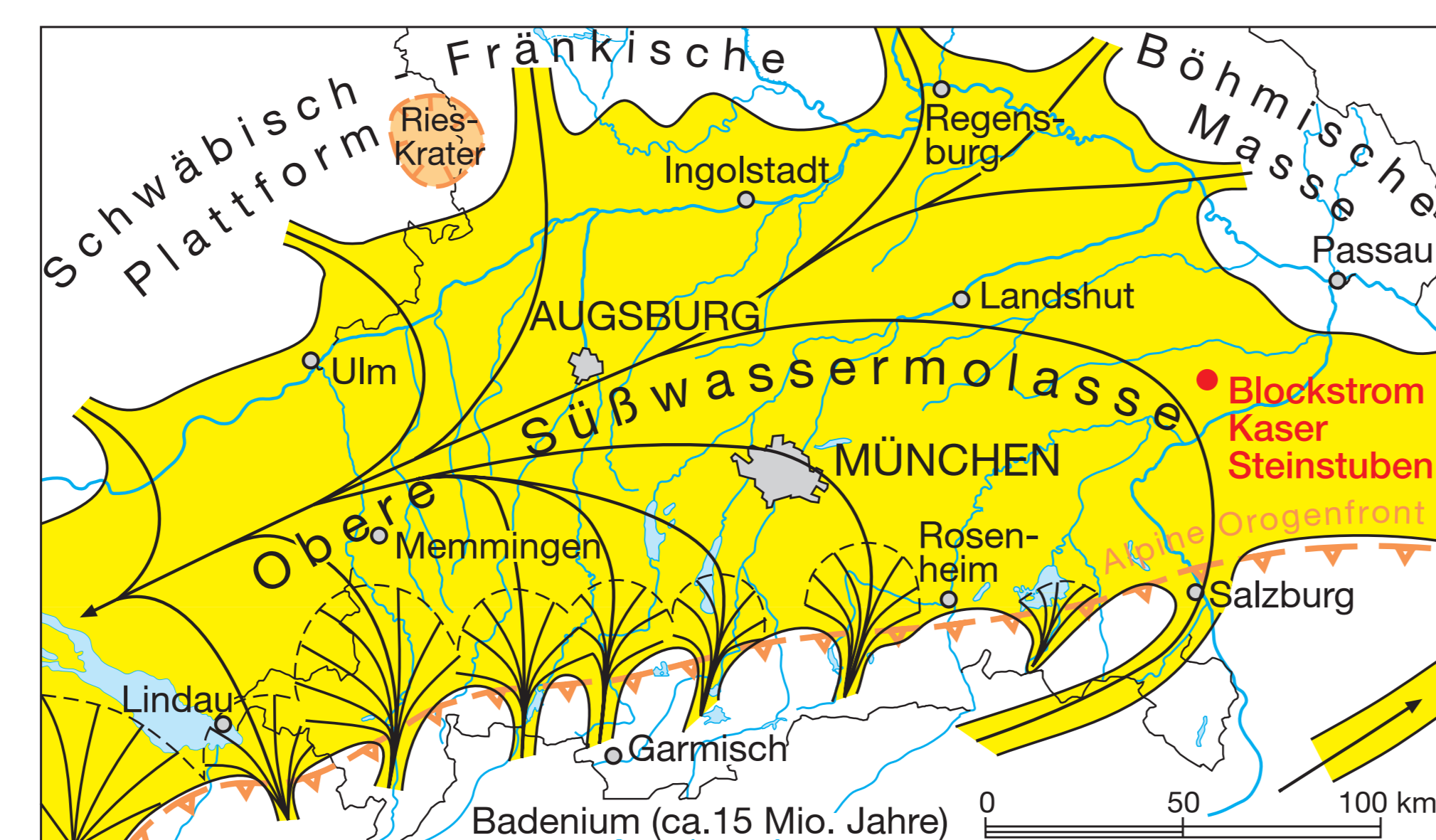
Das Molassebecken während des mittleren Miozäns bei Bildung der Oberen Süßwassermolasse
