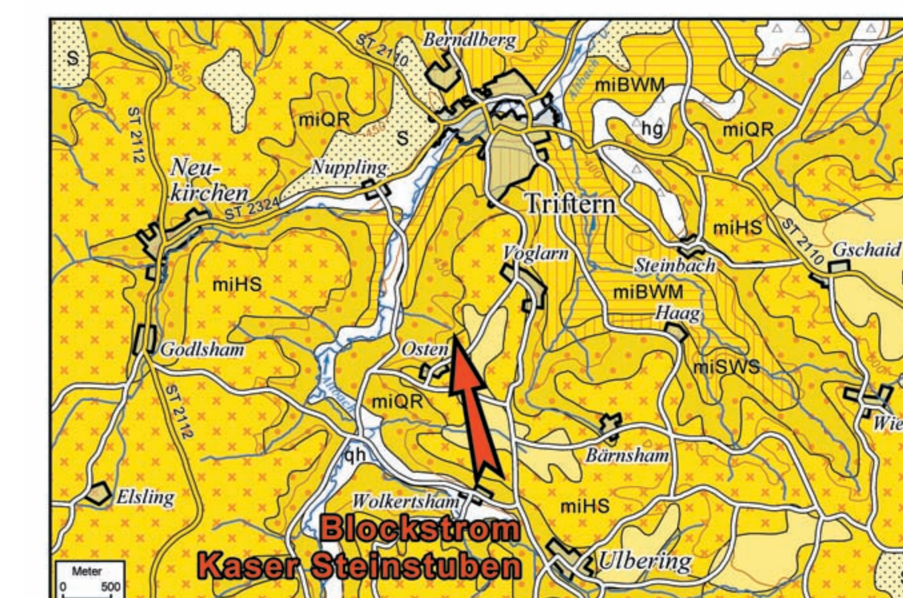
Geologische Karte der Umgebung des Blockstroms Kaser Steinstuben
