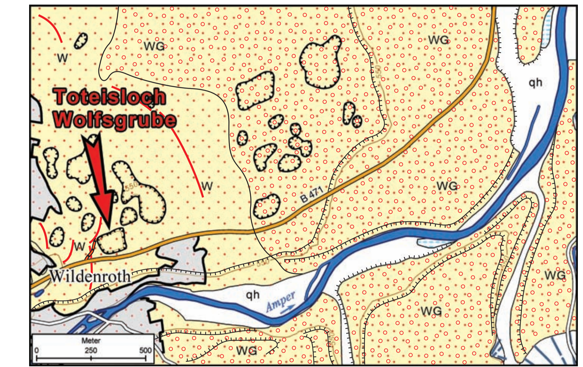
Geologische Karte der Umgebung von Wildenroth
