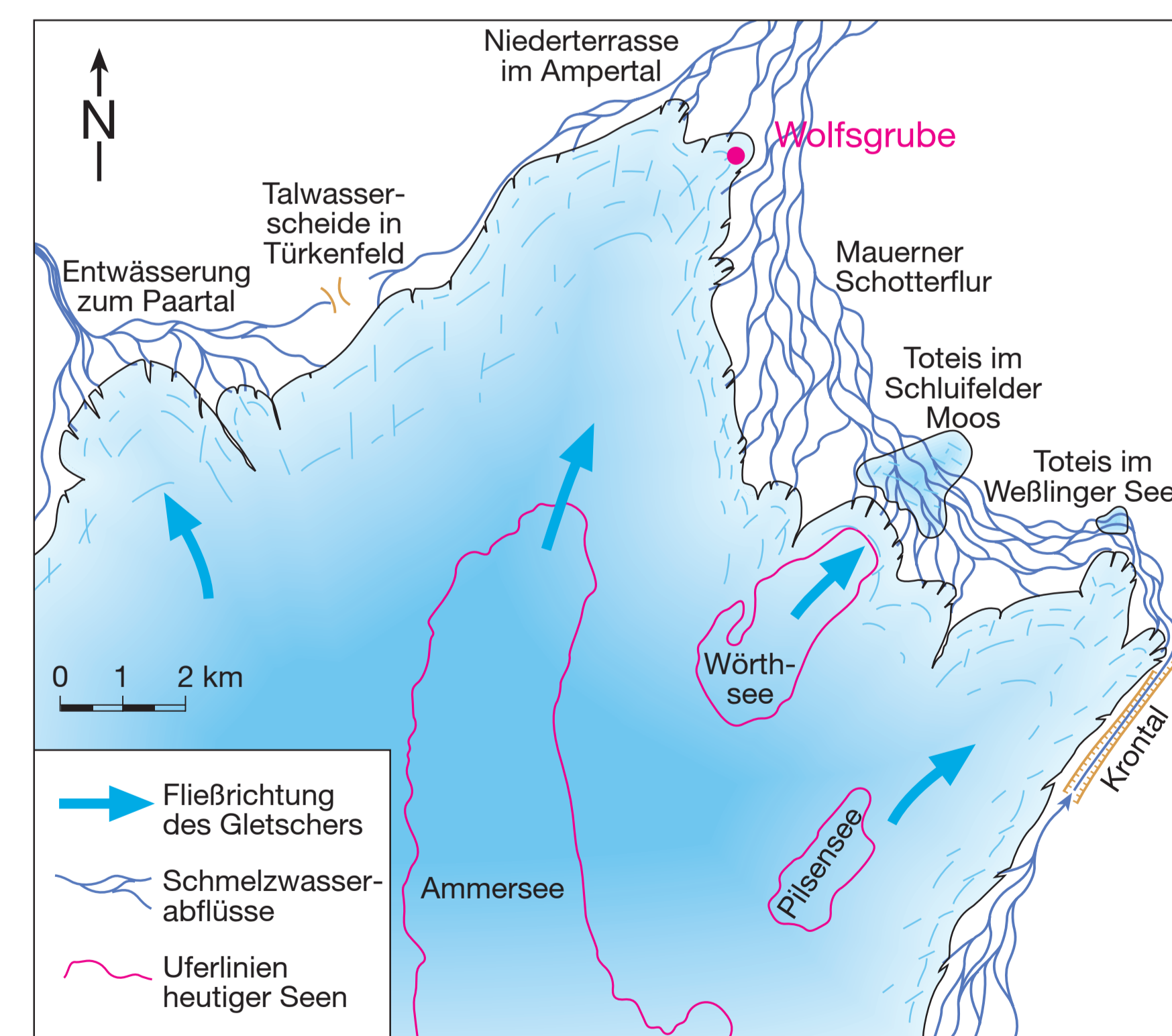
Eisstände des Ammerseegletschers zur Zeit der Rückzugsphase von St. Ottilien-Wildenroth
