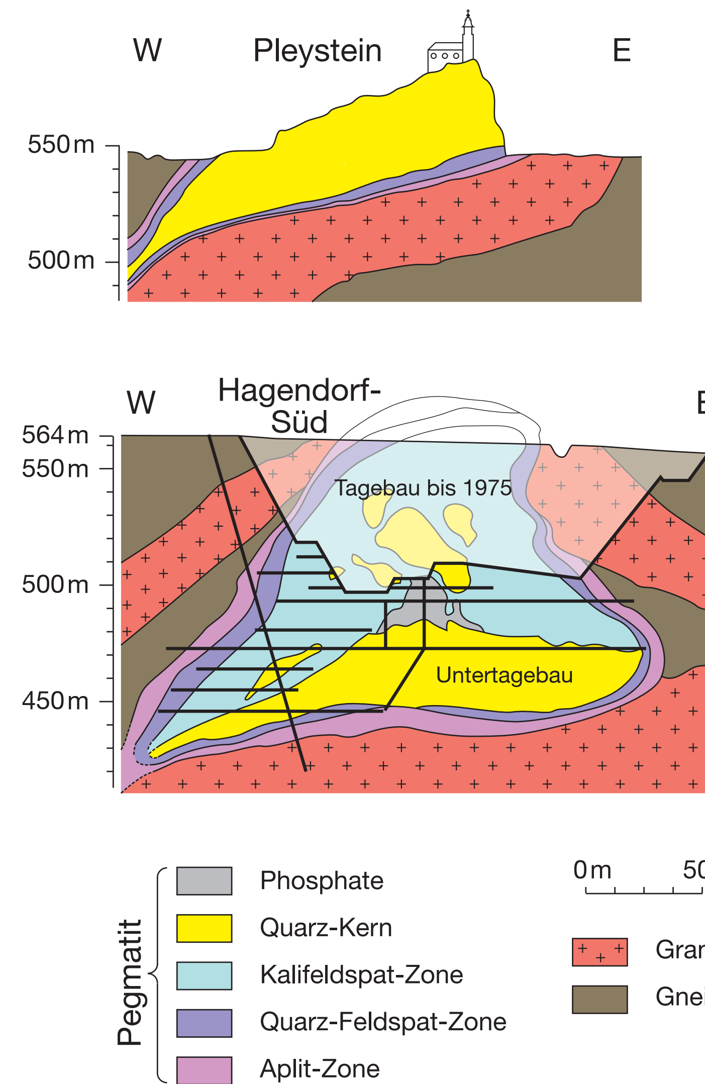
Profile durch die Pegmatite von Pleystein und Hagendorf-Süd
