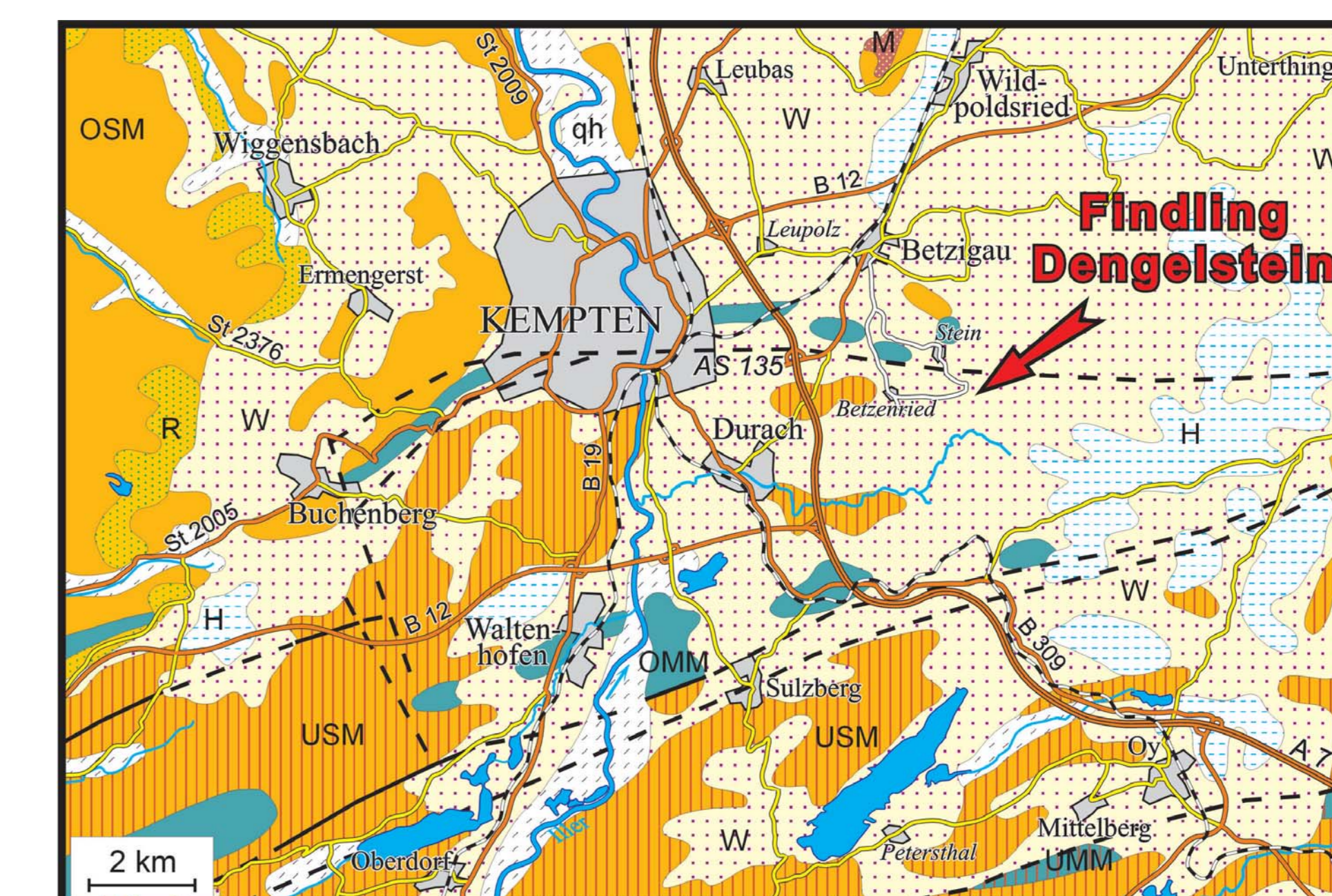
Geologische Karte der Umgebung von Kempten
