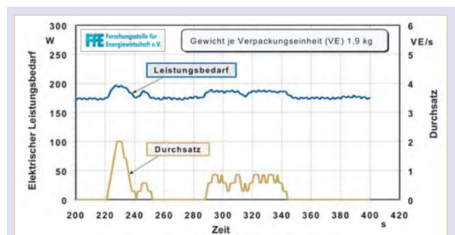
Abbildung 4-8: Durchsatz und Leistungsbedarf eines Bandförderers
