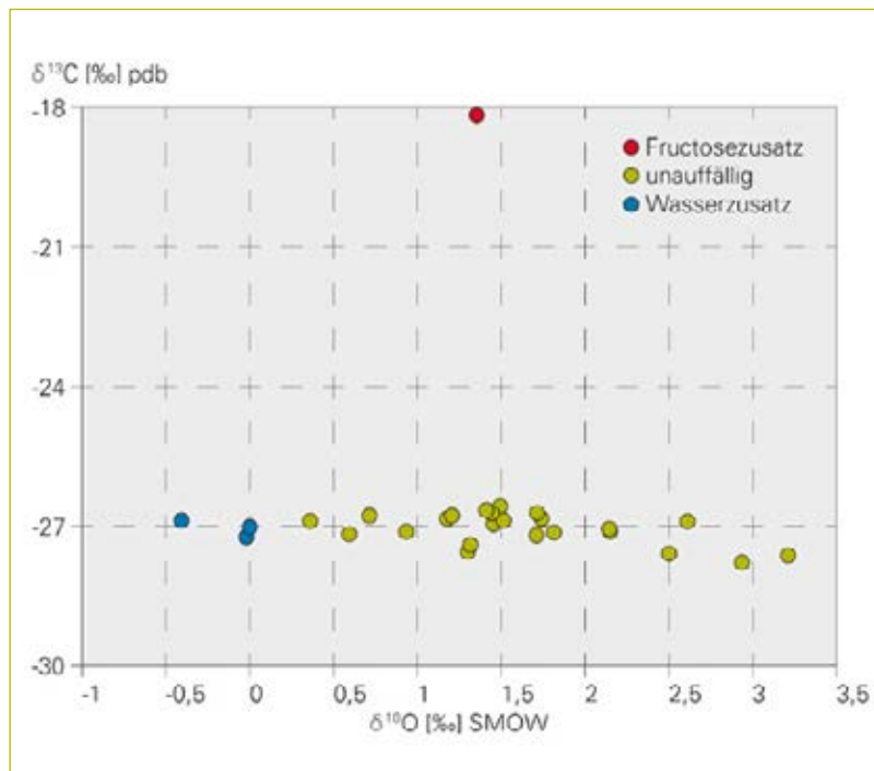
Abbildung 45: Authentizitätsprüfung von Weinen der Lese 2012 aus den Abruzzen anhand der Stabilisotopenverhältnisse des Sauerstoffs ( \delta^{18}\text{O} ) und des Kohlenstoffs ( \delta^{13}\text{C} )
