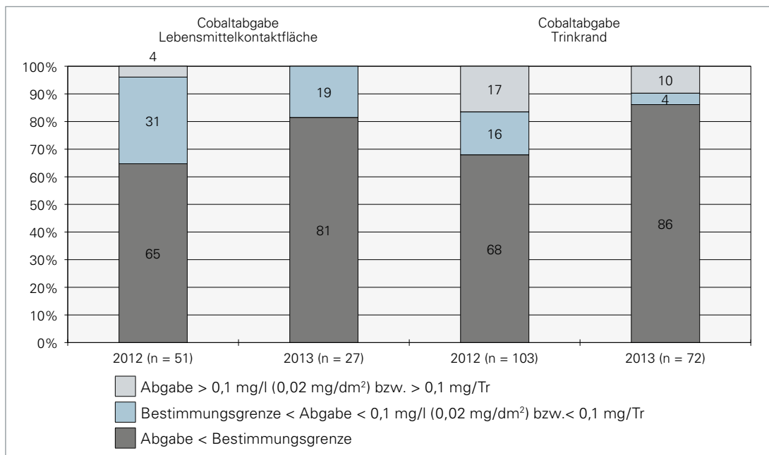
Abbildung 7: Cobaltabgabe aus der Lebensmittelkontaktfläche und aus dem Trinkrand keramischer Lebensmittelbedarfsgegenstände
