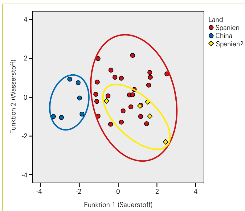
Abbildung 29: Herkunftsbestimmung von Knoblauch verschiedener Herkunftsländer durch Diskriminanzanalyse
