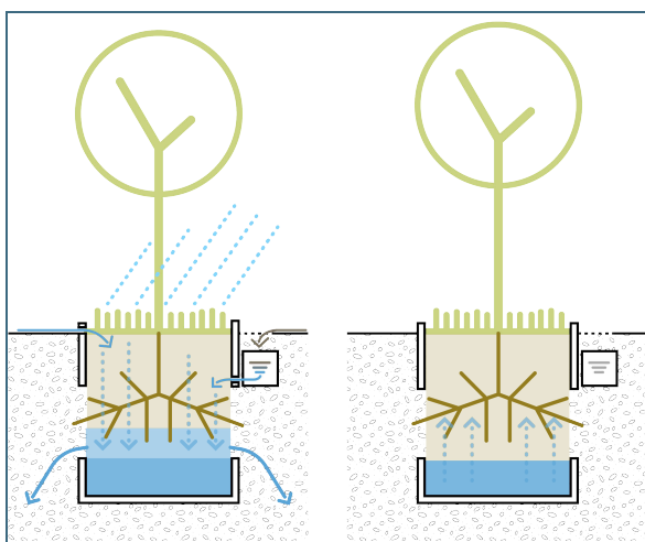
Abb. 19: Beispiel für die Gestaltung bei Baumstandorten im Siedlungsbereich zur multifunktionalen Nutzung; schematische Darstellung des Funktionsprinzips:
