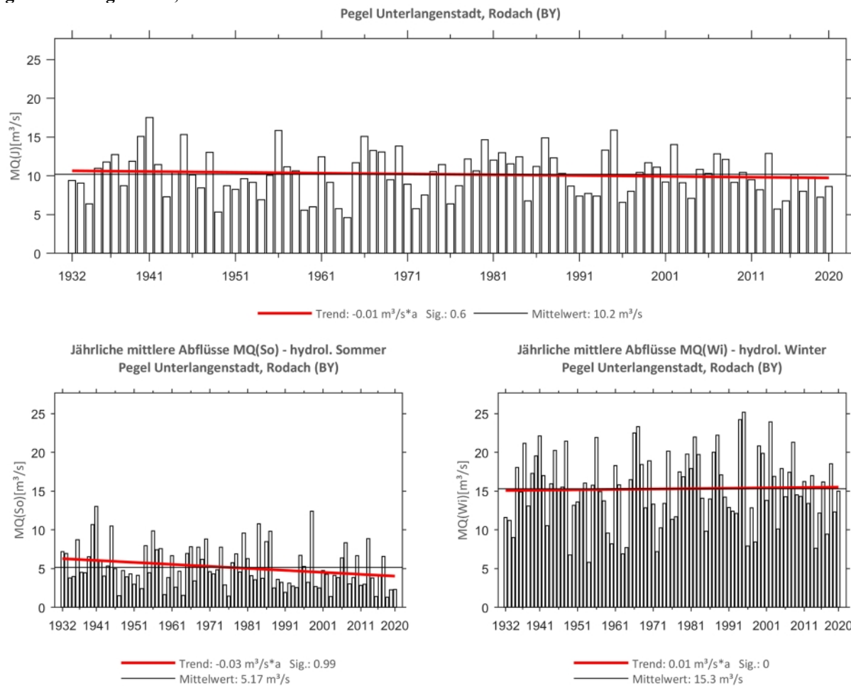
Abb. 174: Trenduntersuchungen von jährlichen mittleren Abflüssen für den Zeitraum 1932 bis 2020.
