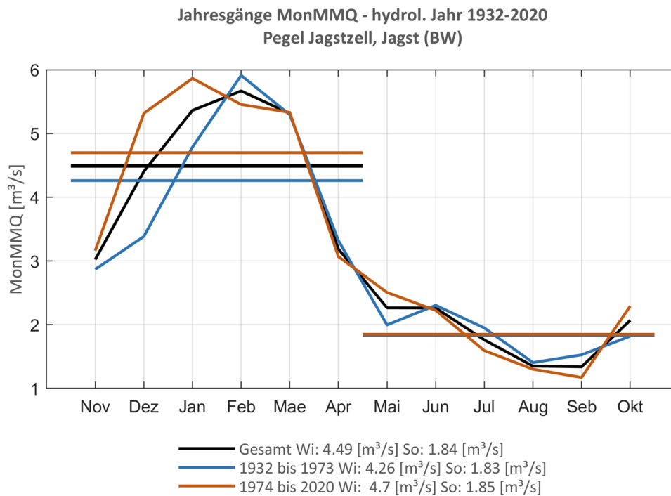
Abb. 29: Jahresgang des MonMMQ und Halbjahresmittel für 1932-2020 sowie 1932-1973 und 1974-2020.
