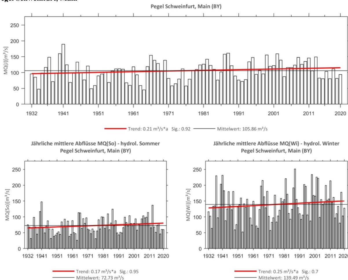
Abb. 178: Trenduntersuchungen von jährlichen mittleren Abflüssen für den Zeitraum 1932 bis 2020.
