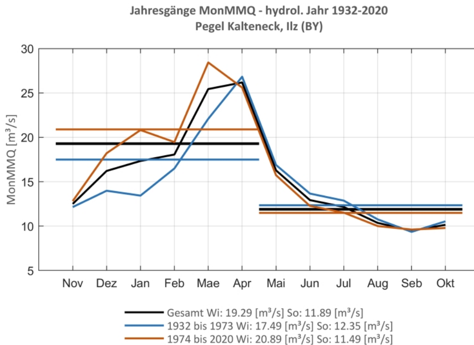
Abb. 73: Jahresgang des MonMMQ und Halbjahresmittel für 1932-2020 sowie 1932-1973 und 1974-2020
