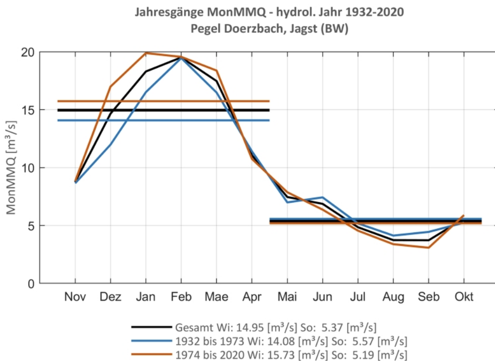
Abb. 23: Jahresgang des MonMMQ und Halbjahresmittel für 1932-2020 sowie 1932-1973 und 1974-2020.
