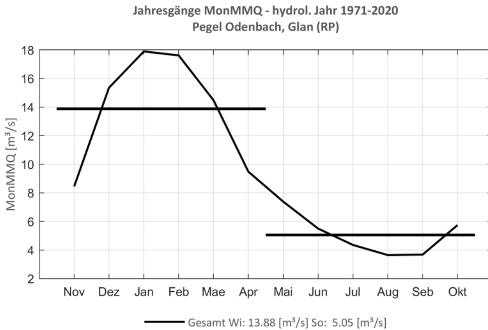
Abb. 266: Jahresgang des MonMMQ und Halbjahresmittel für 1971-2020.
