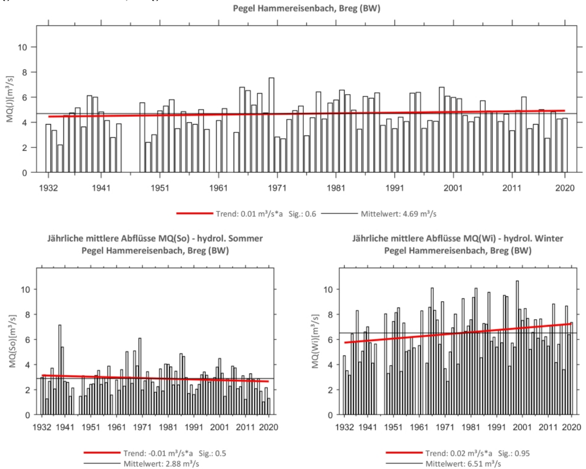
Abb. 52: Trenduntersuchungen von jährlichen mittleren Abflüssen für den Zeitraum 1932 bis 2020.
