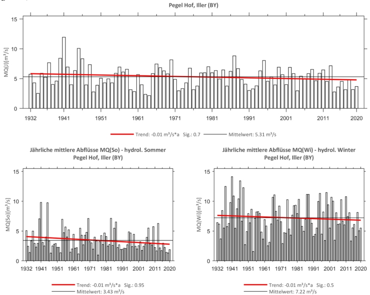
Abb. 68: Trenduntersuchungen von jährlichen mittleren Abflüssen für den Zeitraum 1932 bis 2020.
