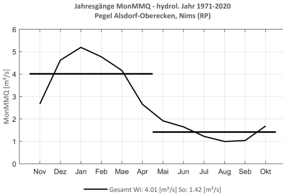
Abb. 190: Jahresgang des MonMMQ und Halbjahresmittel für 1971-2020.
