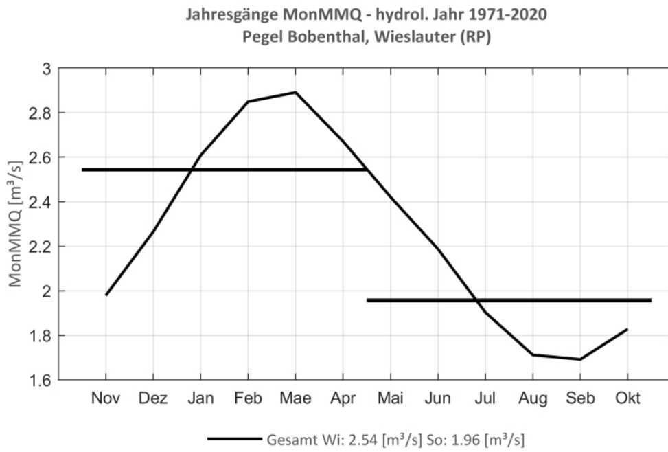
Abb. 234: Jahresgang des MonMMQ und Halbjahresmittel für 1971-2020.
