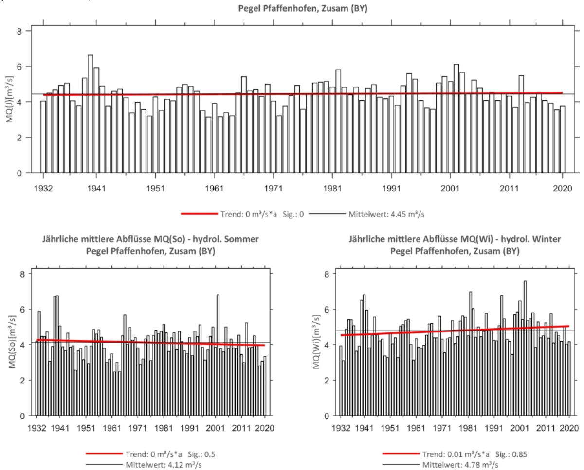
Abb. 88: Trenduntersuchungen von jährlichen mittleren Abflüssen für den Zeitraum 1932 bis 2020.
