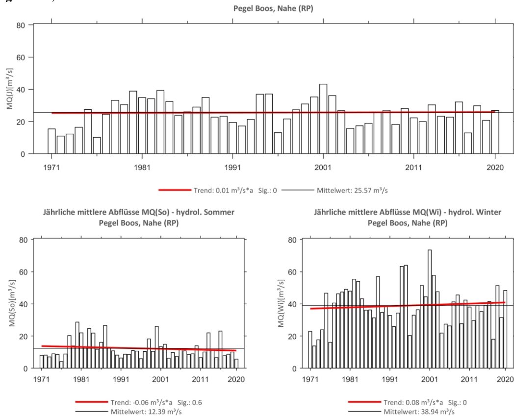
Abb. 236: Trenduntersuchungen von jährlichen mittleren Abflüssen für den Zeitraum 1971 bis 2020.
