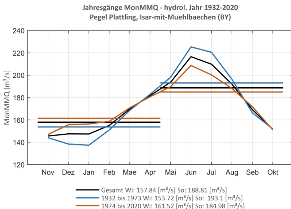
Abb. 127: Jahresgang des MonMMQ und Halbjahresmittel für 1932-2020 sowie 1932-1973 und 1974-2020
