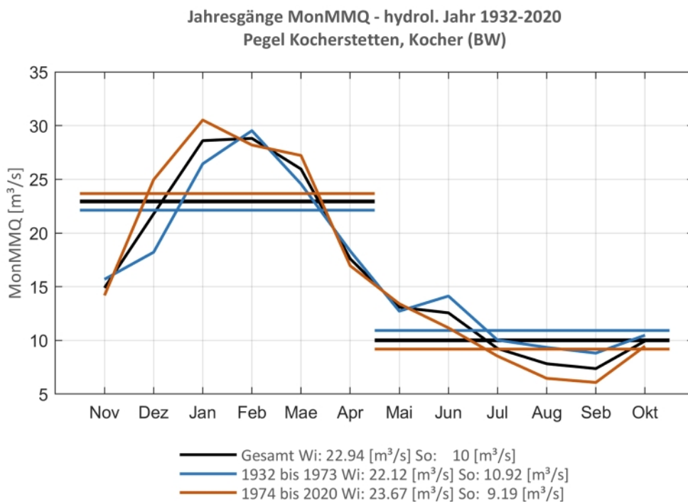
Abb. 31: Jahresgang des MonMMQ und Halbjahresmittel für 1932-2020 sowie 1932-1973 und 1974-2020.
