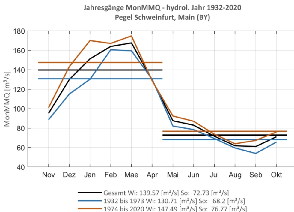
Abb. 179: Jahresgang des MonMMQ und Halbjahresmittel für 1932-2020 sowie 1932-1973 und 1974-2020
