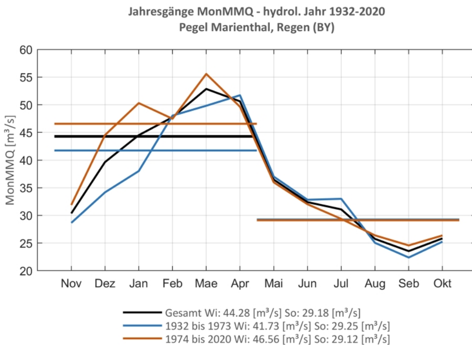
Abb. 75: Jahresgang des MonMMQ und Halbjahresmittel für 1932-2020 sowie 1932-1973 und 1974-2020
