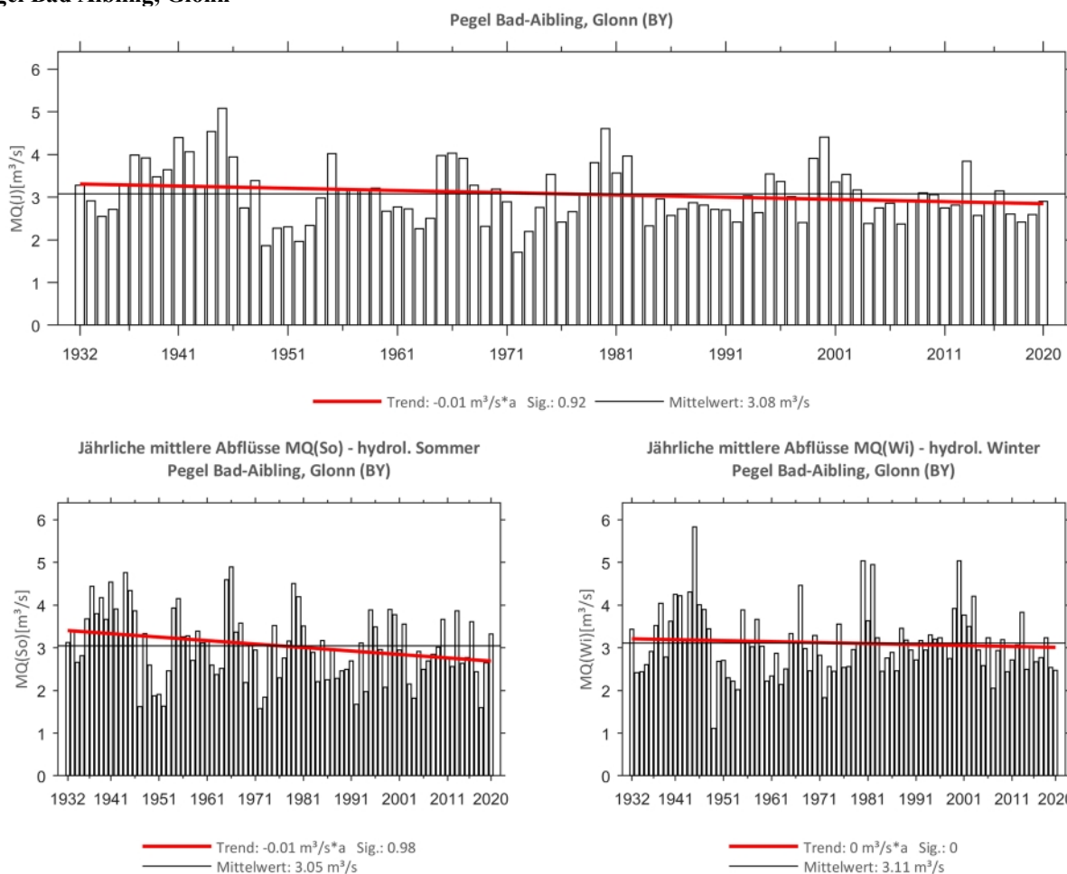
Abb. 98: Trenduntersuchungen von jährlichen mittleren Abflüssen für den Zeitraum 1932 bis 2020.
