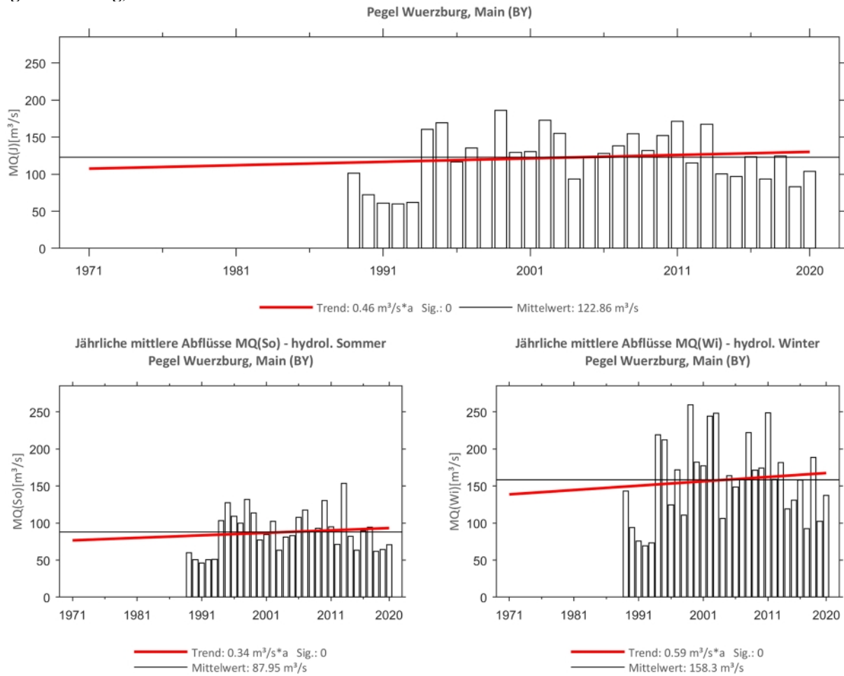
Abb. 182: Trenduntersuchungen von jährlichen mittleren Abflüssen für den Zeitraum 1989 bis 2020.
