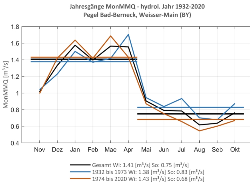
Abb. 155: Jahresgang des MonMMQ und Halbjahresmittel für 1932-2020 sowie 1932-1973 und 1974-2020
