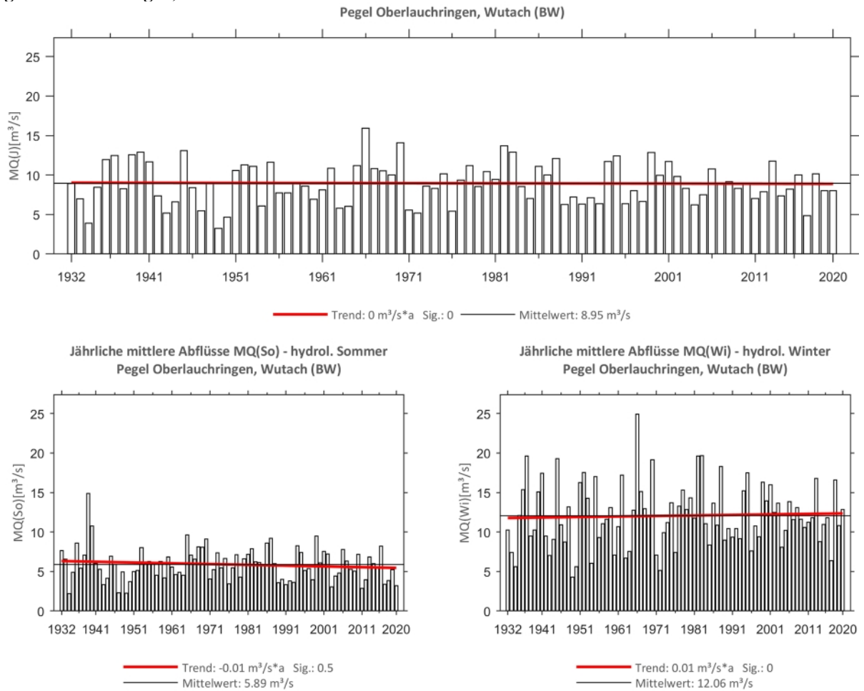
Abb. 12: Trenduntersuchungen von jährlichen mittleren Abflüssen für den Zeitraum 1932 bis 2020.
