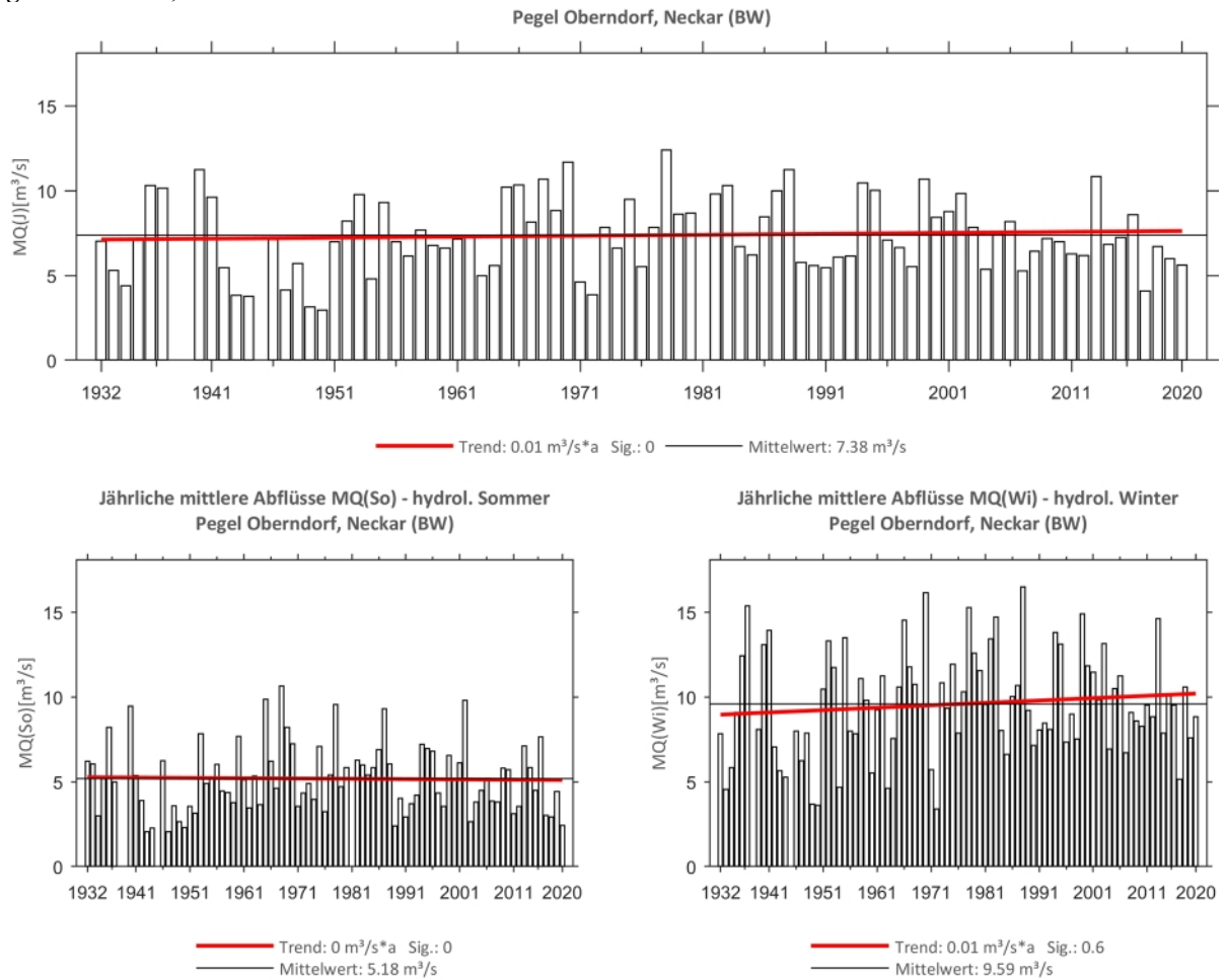
Abb. 36: Trenduntersuchungen von jährlichen mittleren Abflüssen für den Zeitraum 1932 bis 2020.
