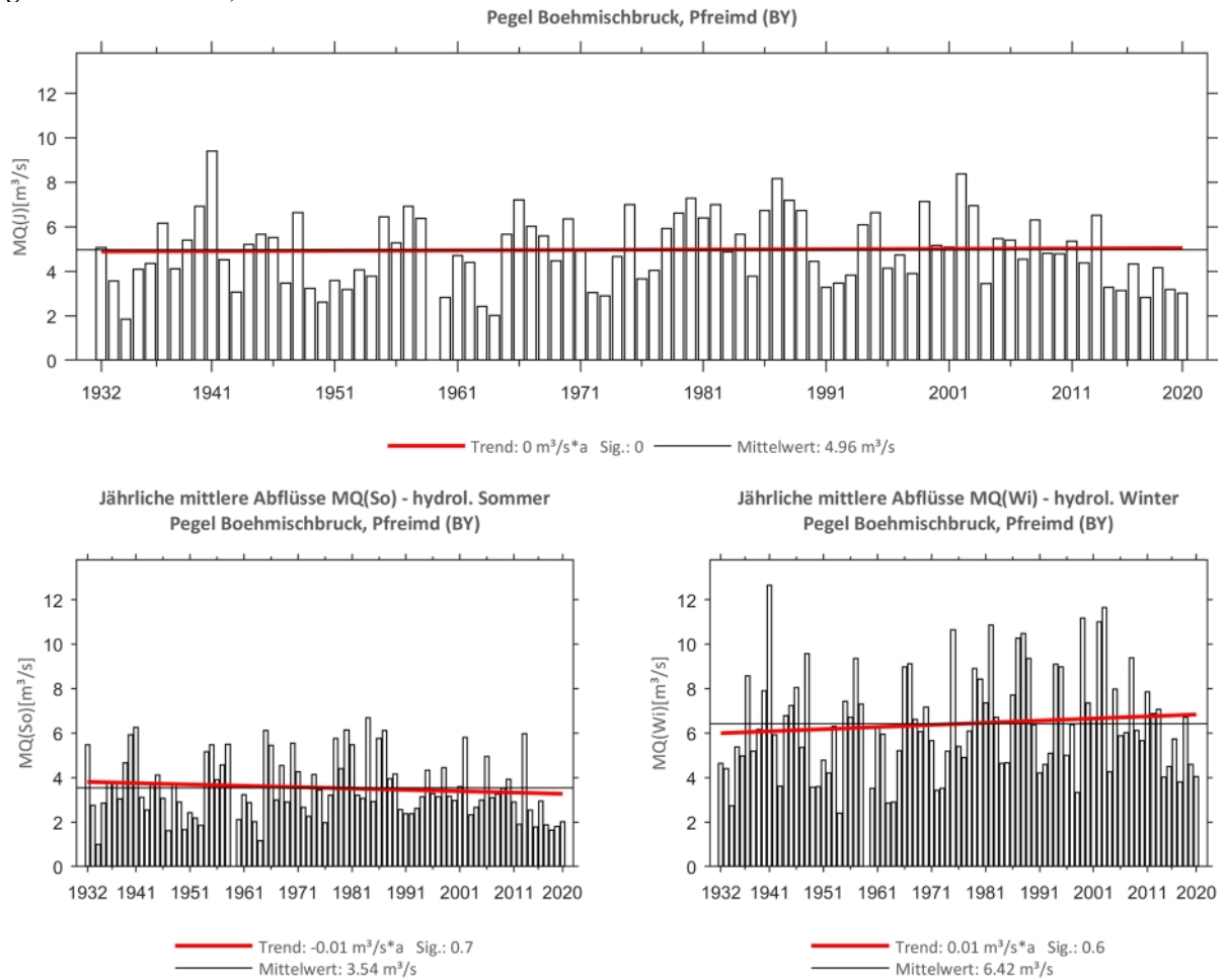
Abb. 64: Trenduntersuchungen von jährlichen mittleren Abflüssen für den Zeitraum 1932 bis 2020.
