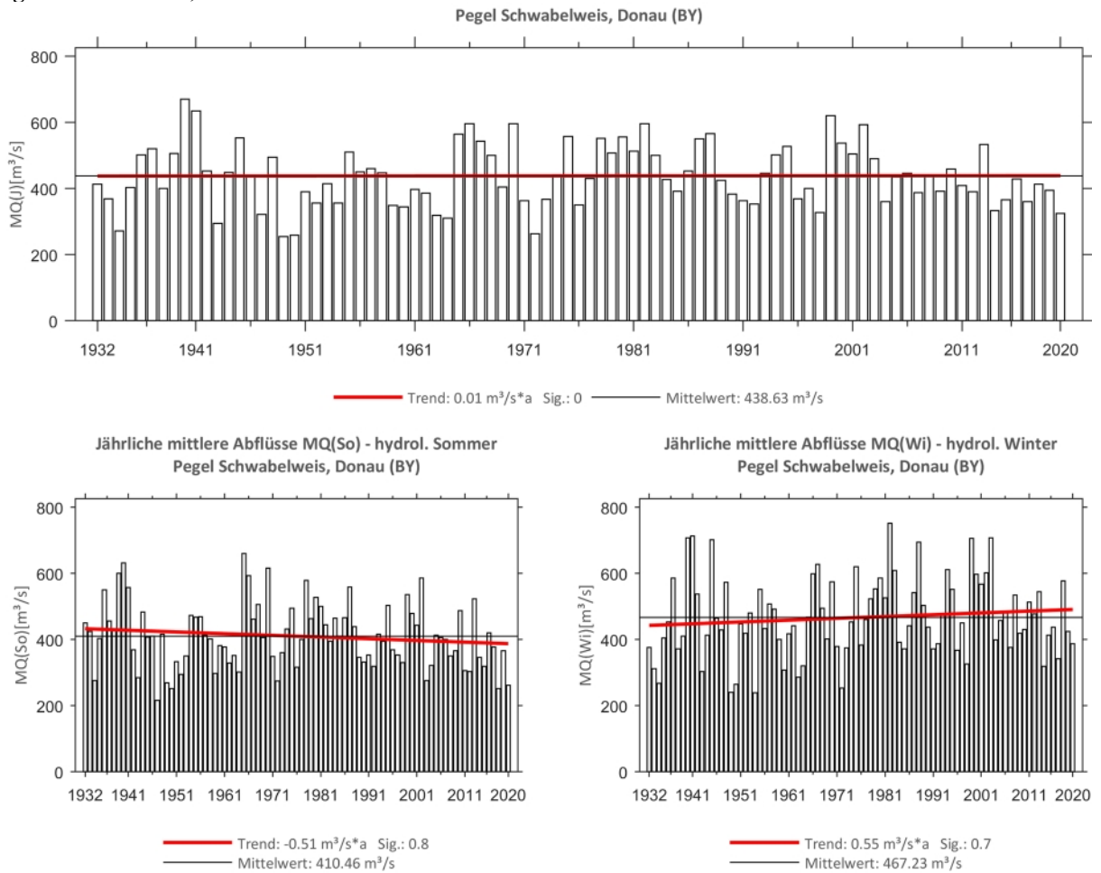
Abb. 152: Trenduntersuchungen von jährlichen mittleren Abflüssen für den Zeitraum 1932 bis 2020.
