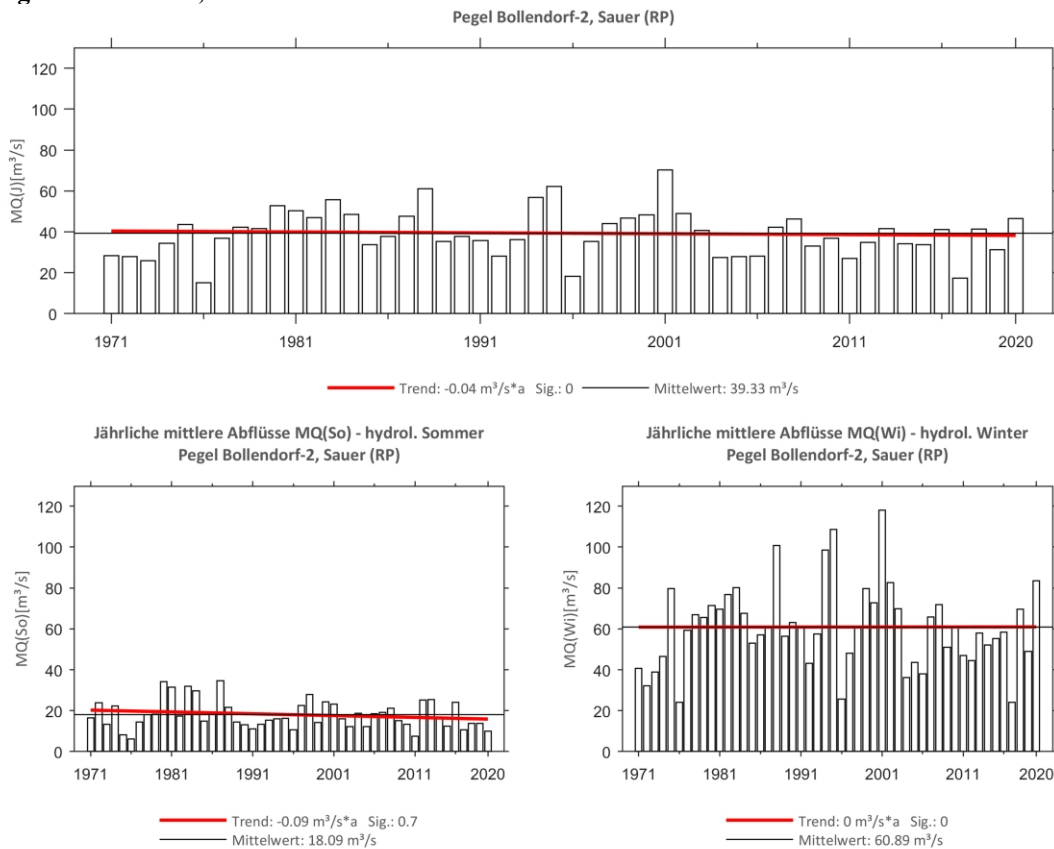
Abb. 200: Trenduntersuchungen von jährlichen mittleren Abflüssen für den Zeitraum 1971 bis 2020.
