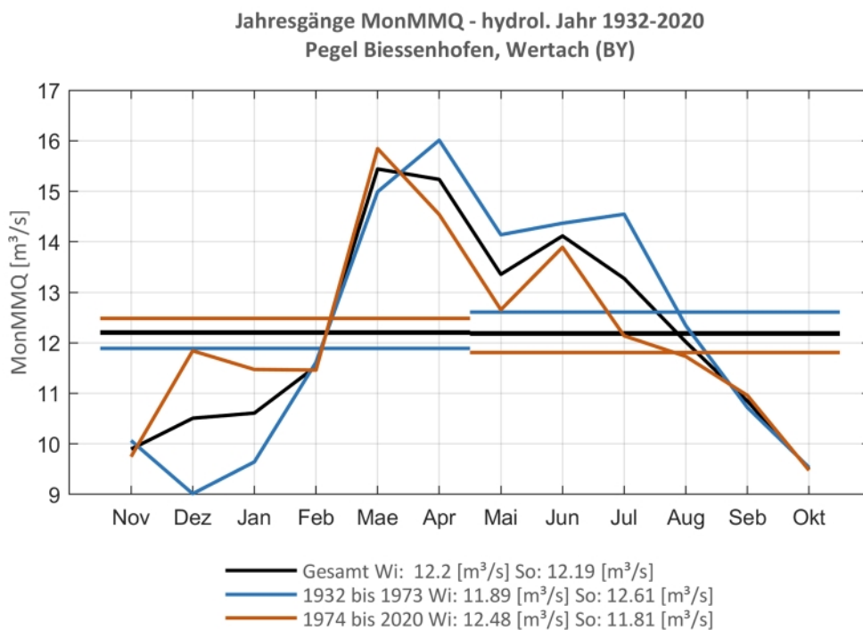
Abb. 79: Jahresgang des MonMMQ und Halbjahresmittel für 1932-2020 sowie 1932-1973 und 1974-2020
