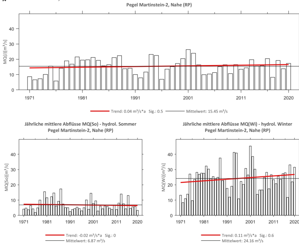
Abb. 254: Trenduntersuchungen von jährlichen mittleren Abflüssen für den Zeitraum 1971 bis 2020. Pegel Martinstein-2, Nahe (RP)
