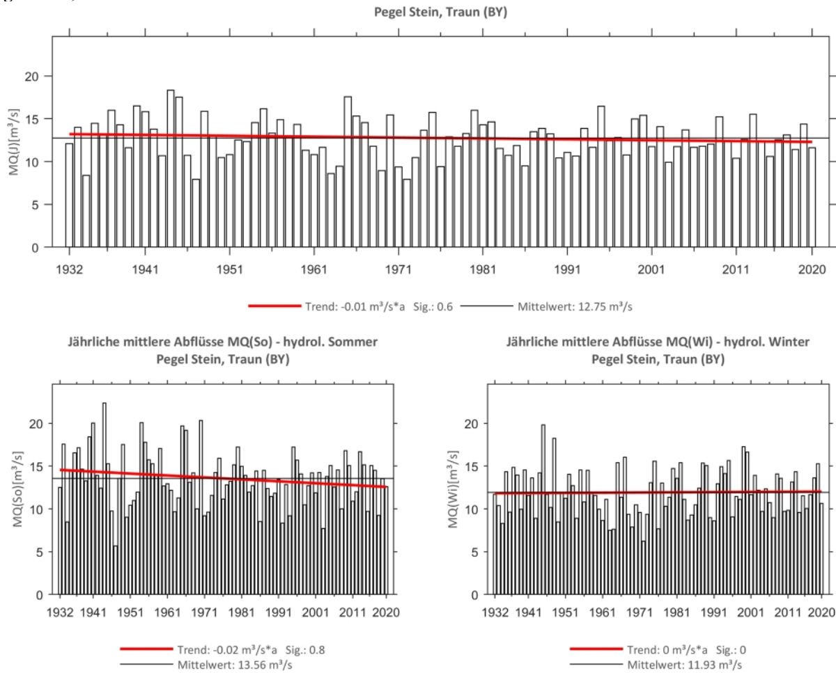
Abb. 134: Trenduntersuchungen von jährlichen mittleren Abflüssen für den Zeitraum 1932 bis 2020.
