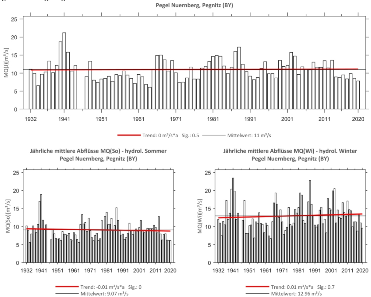
Abb. 168: Trenduntersuchungen von jährlichen mittleren Abflüssen für den Zeitraum 1932 bis 2020.
