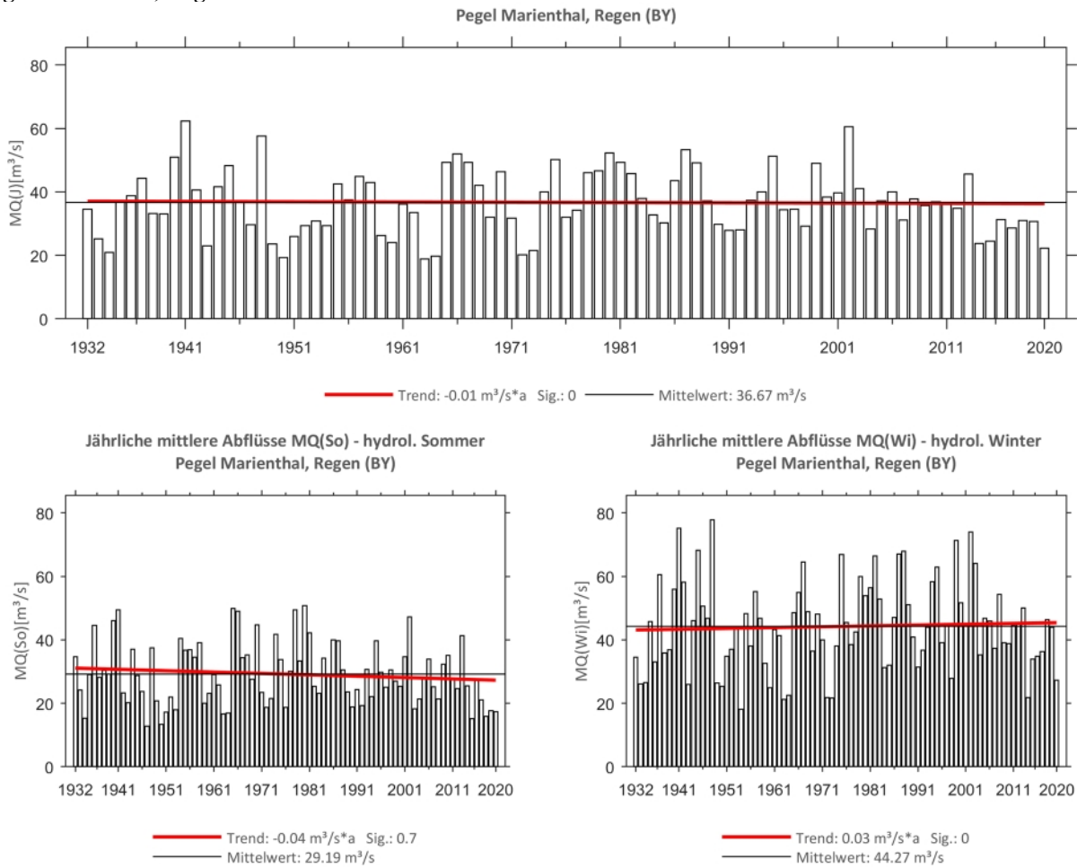
Abb. 74: Trenduntersuchungen von jährlichen mittleren Abflüssen für den Zeitraum 1932 bis 2020.
