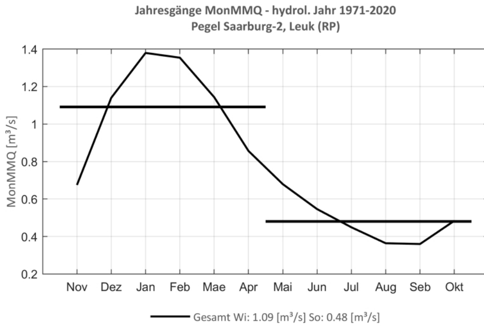
Abb. 226: Jahresgang des MonMMQ und Halbjahresmittel für 1971-2020.
