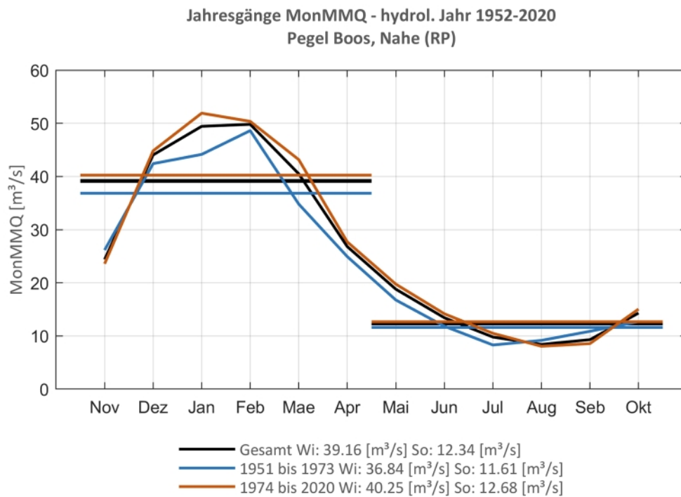
Abb. 239: Jahresgang des MonMMQ und Halbjahresmittel für 1952-2020 sowie 1952-1973 und 1974-2020.
