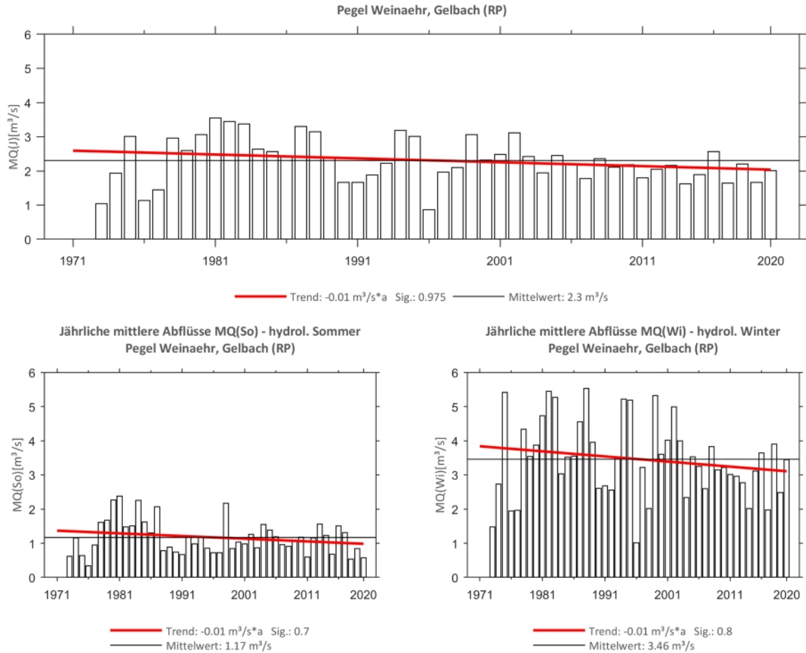
Abb. 184: Trenduntersuchungen von jährlichen mittleren Abflüssen für den Zeitraum 1973 bis 2020.
