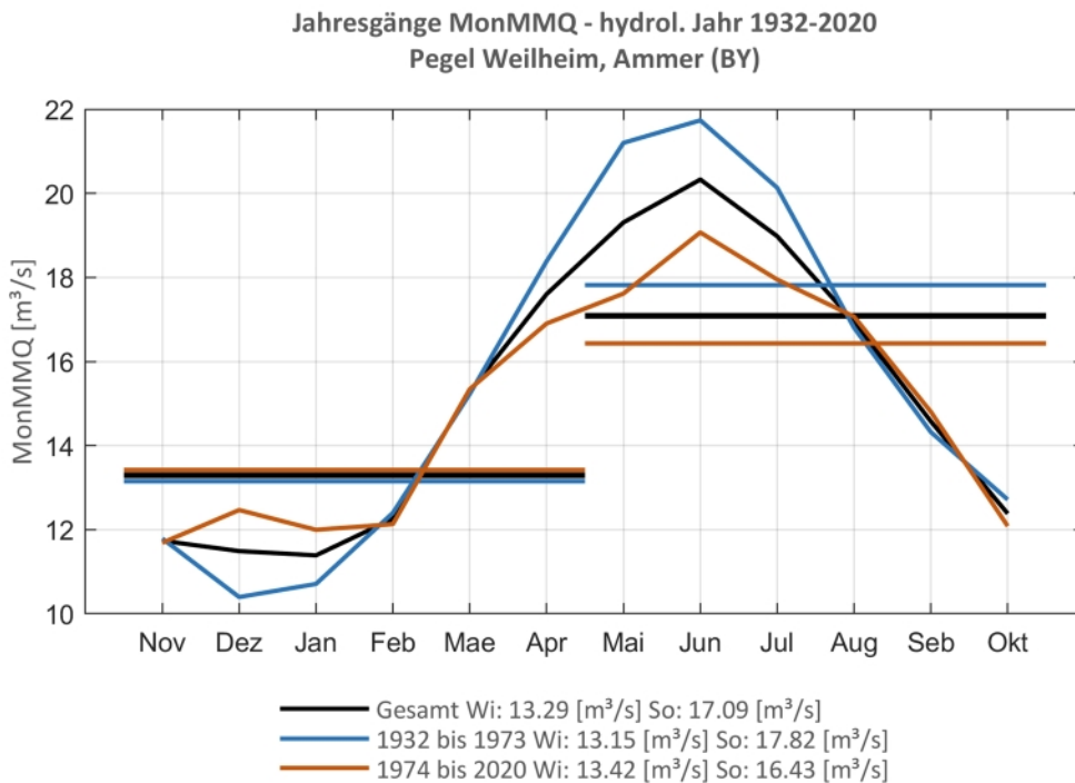
Abb. 139: Jahresgang des MonMMQ und Halbjahresmittel für 1932-2020 sowie 1932-1973 und 1974-2020
