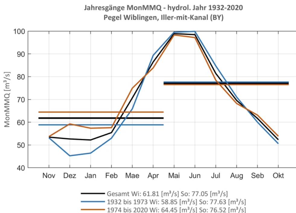
Abb. 95: Jahresgang des MonMMQ und Halbjahresmittel für 1932-2020 sowie 1932-1973 und 1974-2020
