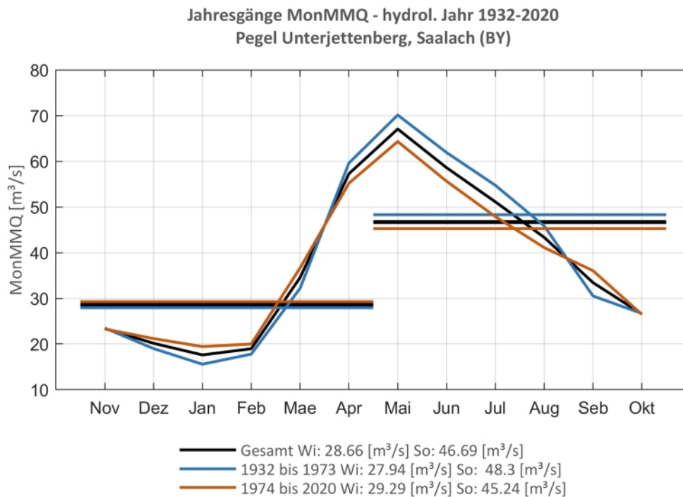
Abb. 137: Jahresgang des MonMMQ und Halbjahresmittel für 1932-2020 sowie 1932-1973 und 1974-2020
