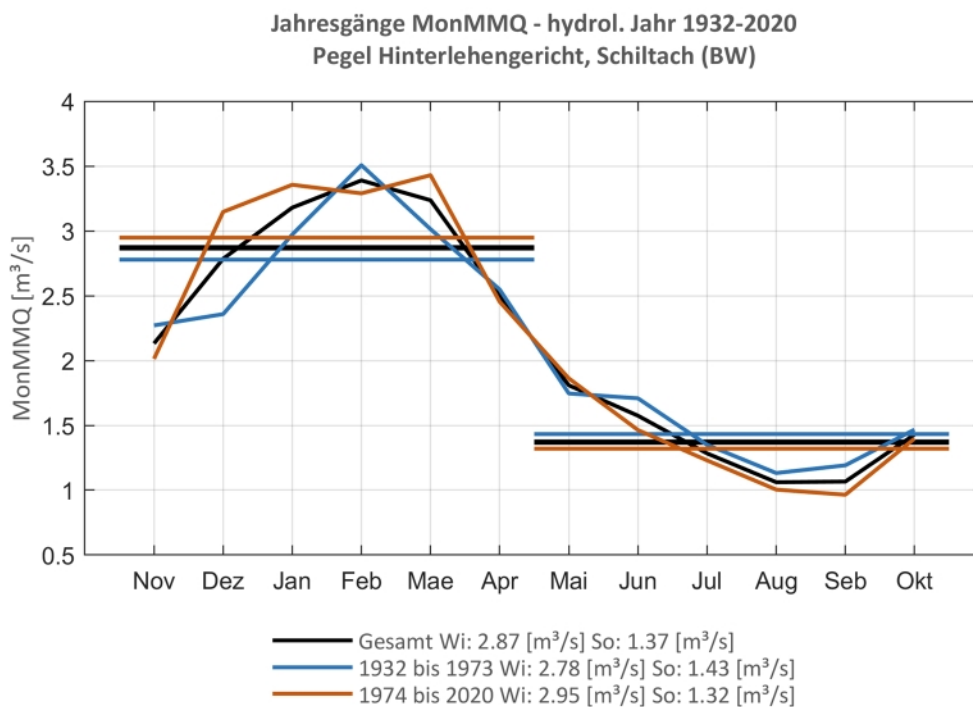
Abb. 11: Jahresgang des MonMMQ und Halbjahresmittel für 1932-2020 sowie 1932-1973 und 1974-2020.
