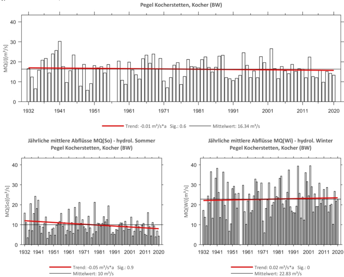
Abb. 30: Trenduntersuchungen von jährlichen mittleren Abflüssen für den Zeitraum 1932 bis 2020.
