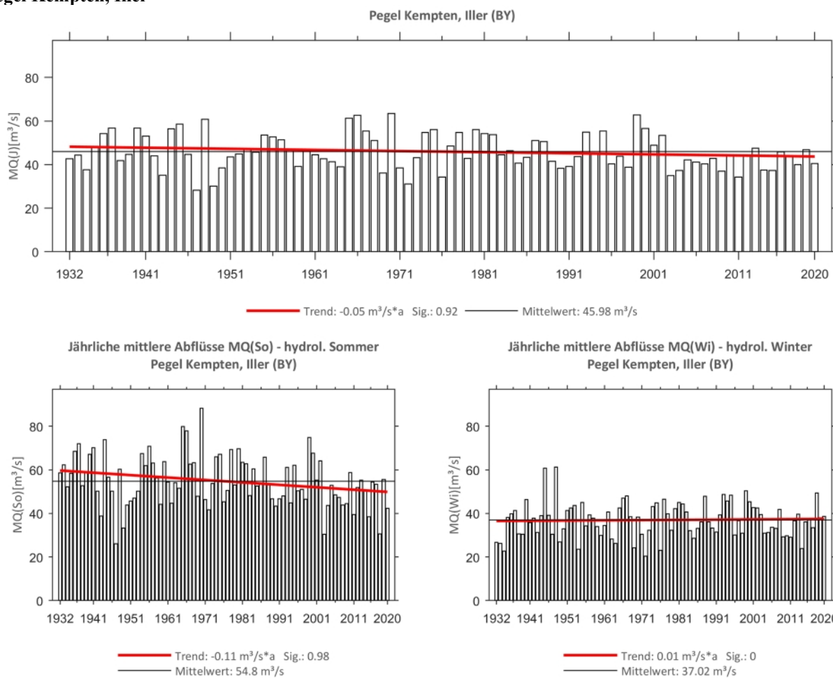
Abb. 82: Trenduntersuchungen von jährlichen mittleren Abflüssen für den Zeitraum 1932 bis 2020.
