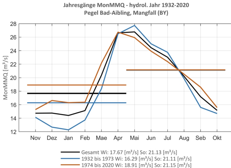
Abb. 101: Jahresgang des MonMMQ und Halbjahresmittel für 1932-2020 sowie 1932-1973 und 1974-2020
