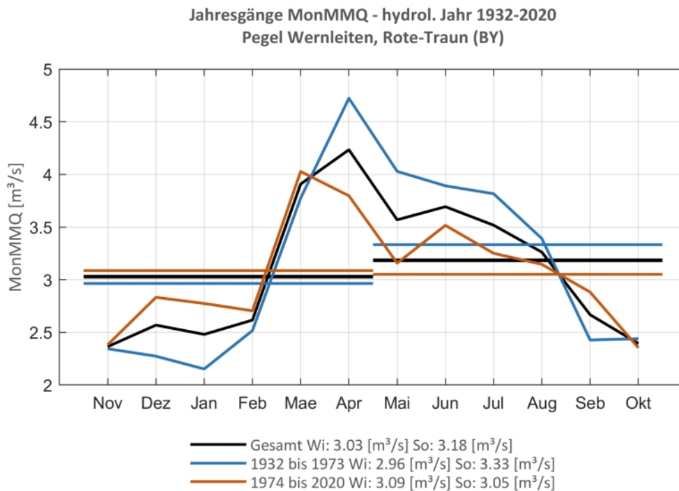
Abb. 141: Jahresgang des MonMMQ und Halbjahresmittel für 1932-2020 sowie 1932-1973 und 1974-2020
