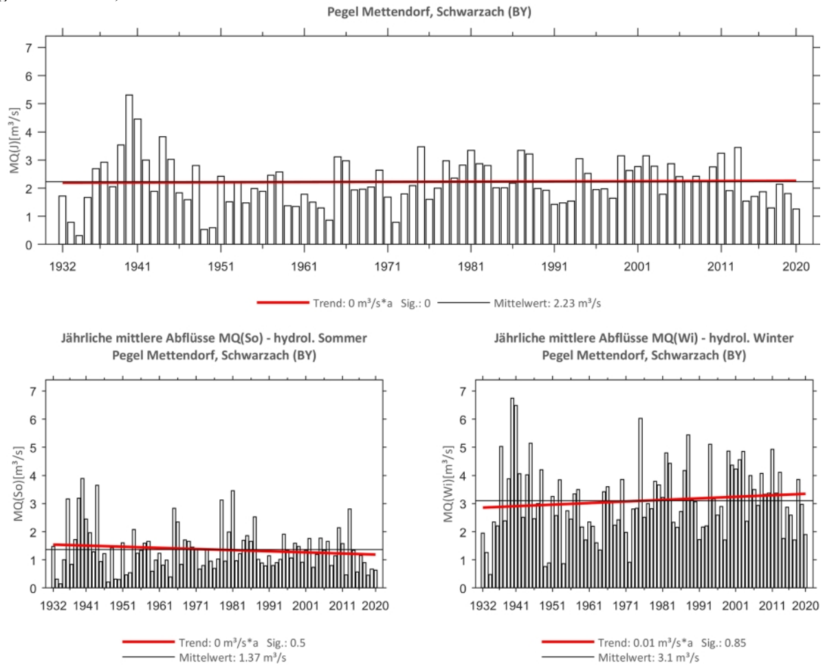
Abb. 148: Trenduntersuchungen von jährlichen mittleren Abflüssen für den Zeitraum 1932 bis 2020.
