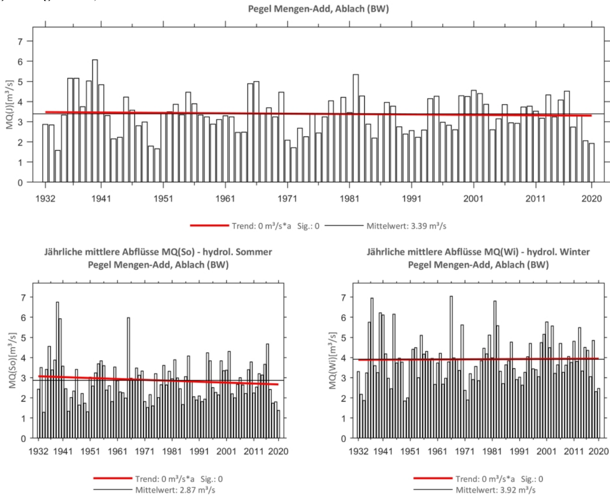
Abb. 58: Trenduntersuchungen von jährlichen mittleren Abflüssen für den Zeitraum 1932 bis 2020.
