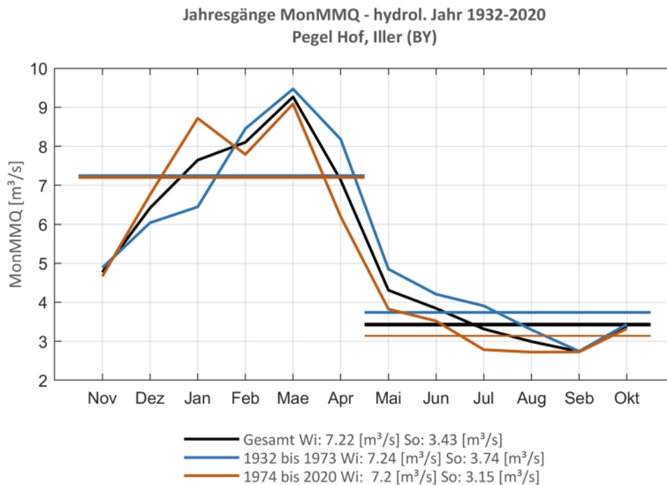
Abb. 69: Jahresgang des MonMMQ und Halbjahresmittel für 1932-2020 sowie 1932-1973 und 1974-2020
