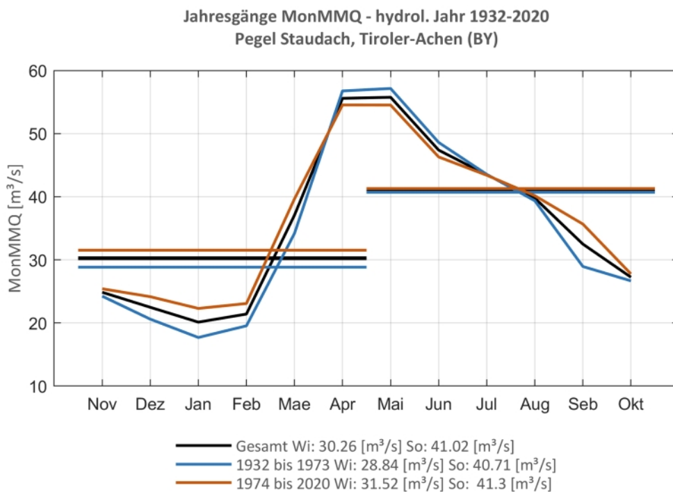
Abb. 135: Jahresgang des MonMMQ und Halbjahresmittel für 1932-2020 sowie 1932-1973 und 1974-2020
