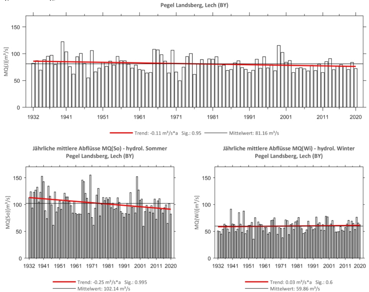
Abb. 84: Trenduntersuchungen von jährlichen mittleren Abflüssen für den Zeitraum 1932 bis 2020.
