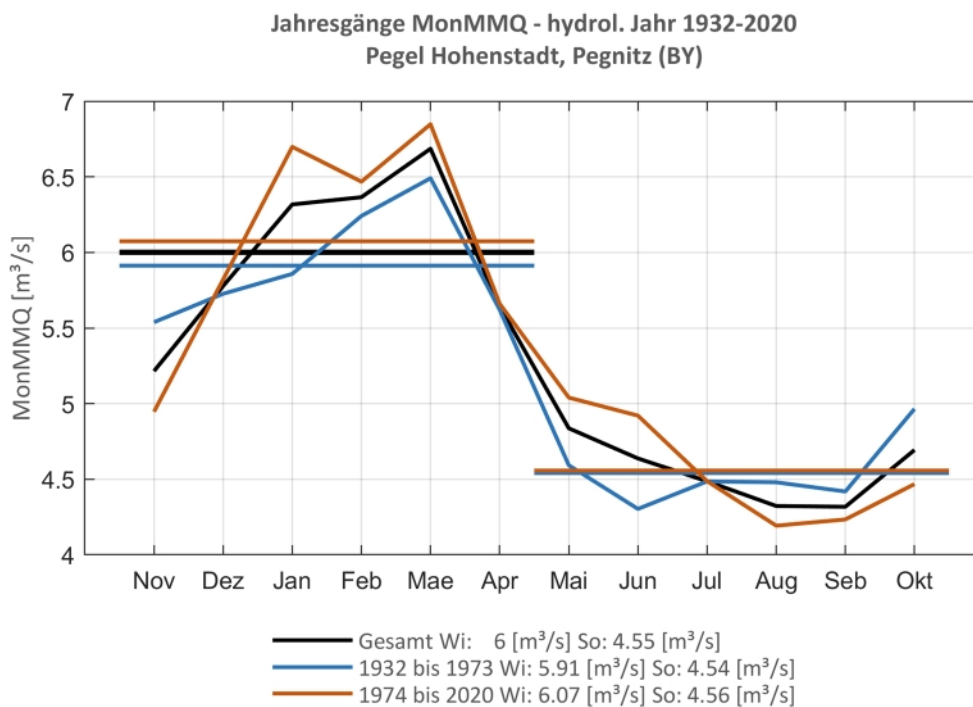
Abb. 159: Jahresgang des MonMMQ und Halbjahresmittel für 1932-2020 sowie 1932-1973 und 1974-2020
