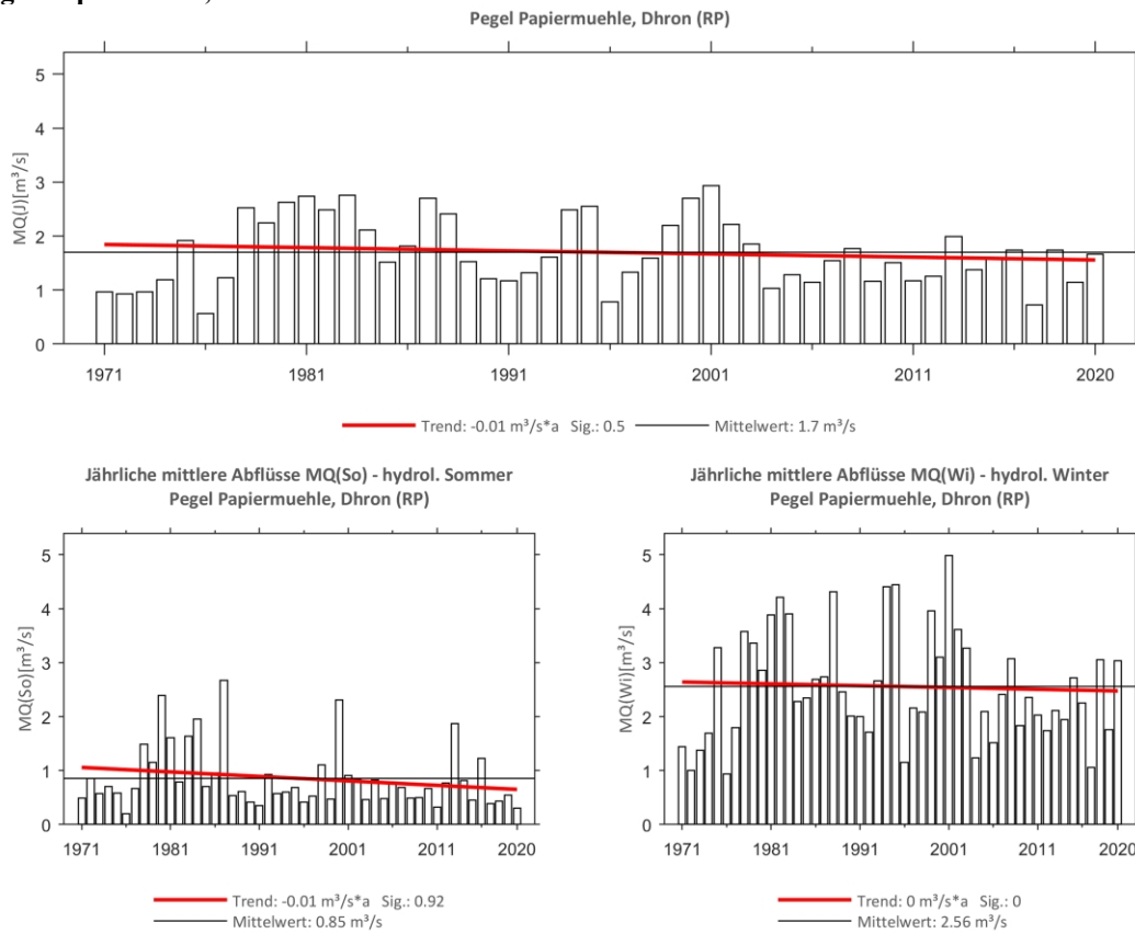
Abb. 218: Trenduntersuchungen von jährlichen mittleren Abflüssen für den Zeitraum 1971 bis 2020.
