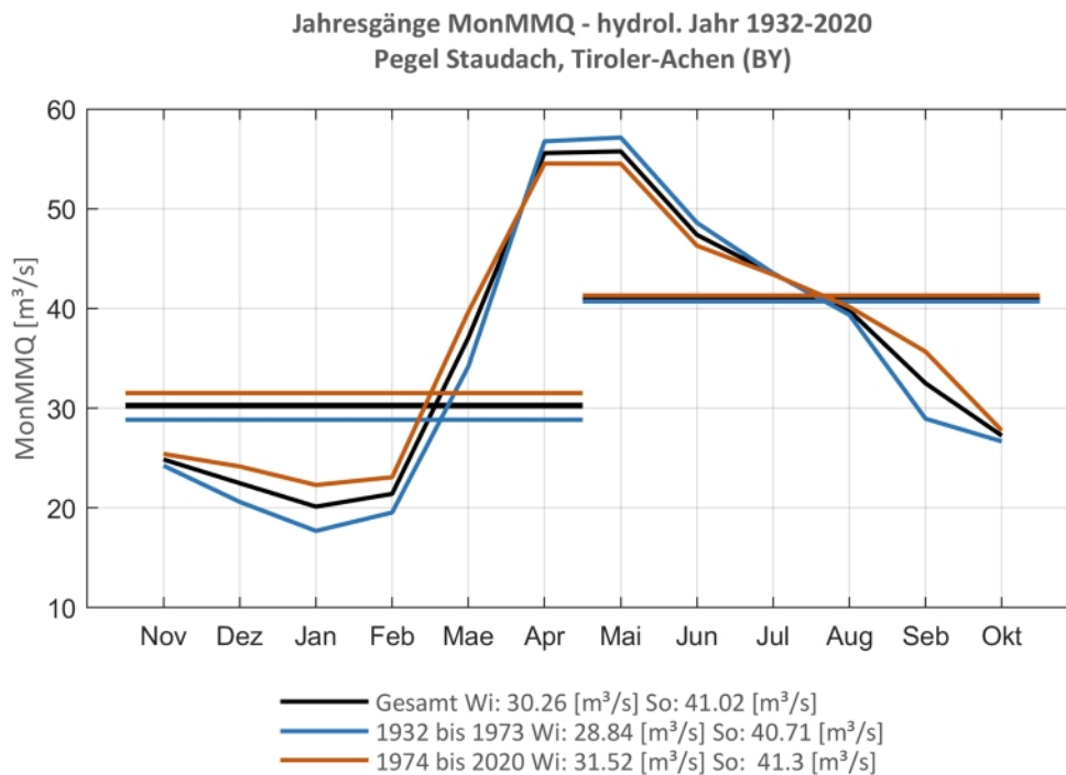
Abb. 133: Jahresgang des MonMMQ und Halbjahresmittel für 1932-2020 sowie 1932-1973 und 1974-2020
