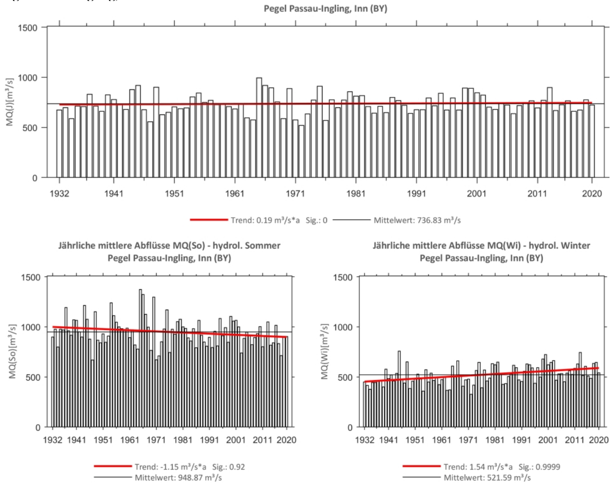
Abb. 124: Trenduntersuchungen von jährlichen mittleren Abflüssen für den Zeitraum 1932 bis 2020.
