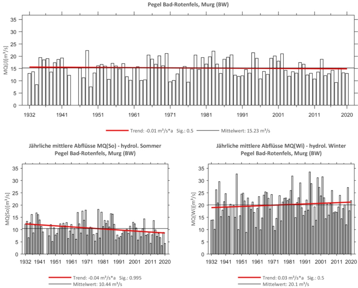
Abb. 2: Trenduntersuchungen von jährlichen mittleren Abflüssen für den Zeitraum 1932 bis 2020.
