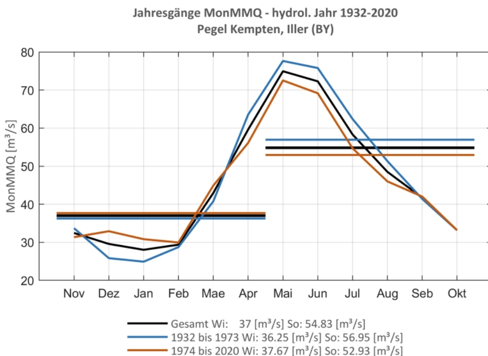
Abb. 83: Jahresgang des MonMMQ und Halbjahresmittel für 1932-2020 sowie 1932-1973 und 1974-2020
