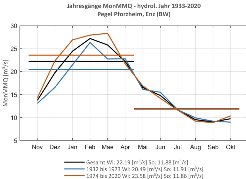
Abb. 39: Jahresgang des MonMMQ und Halbjahresmittel für 1933-2020 sowie 1933-1973 und 1974-2020.
