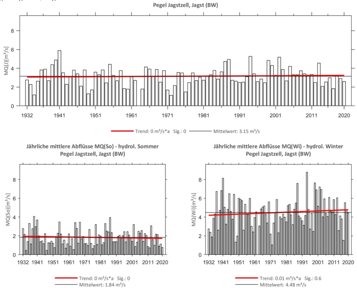
Abb. 28: Trenduntersuchungen von jährlichen mittleren Abflüssen für den Zeitraum 1932 bis 2020.
