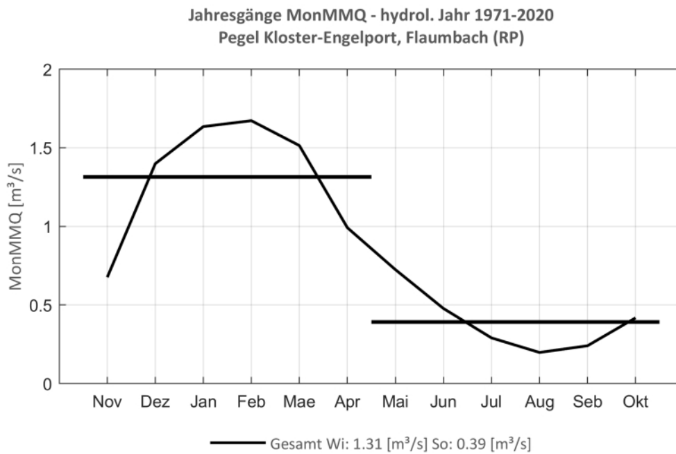
Abb. 212: Jahresgang des MonMMQ und Halbjahresmittel für 1971-2020.
