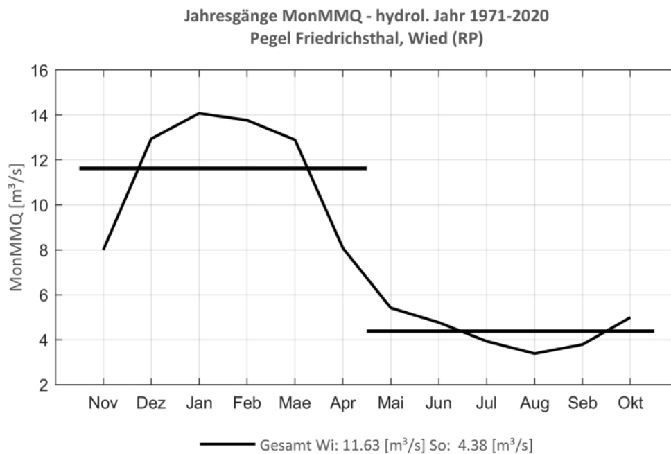
Abb. 206: Jahresgang des MonMMQ und Halbjahresmittel für 1971-2020.
