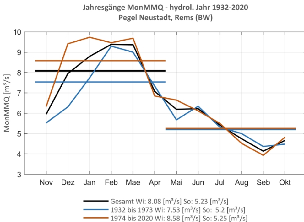
Abb. 35: Jahresgang des MonMMQ und Halbjahresmittel für 1932-2020 sowie 1932-1973 und 1974-2020.
