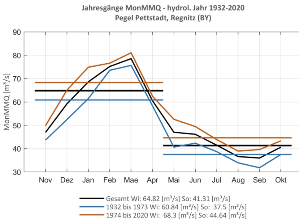
Abb. 171: Jahresgang des MonMMQ und Halbjahresmittel für 1932-2020 sowie 1932-1973 und 1974-2020
