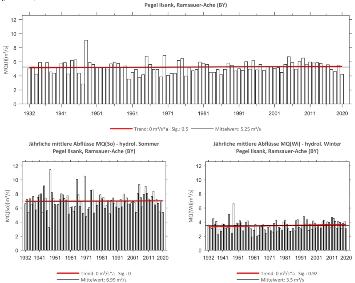
Abb. 112: Trenduntersuchungen von jährlichen mittleren Abflüssen für den Zeitraum 1932 bis 2020.
