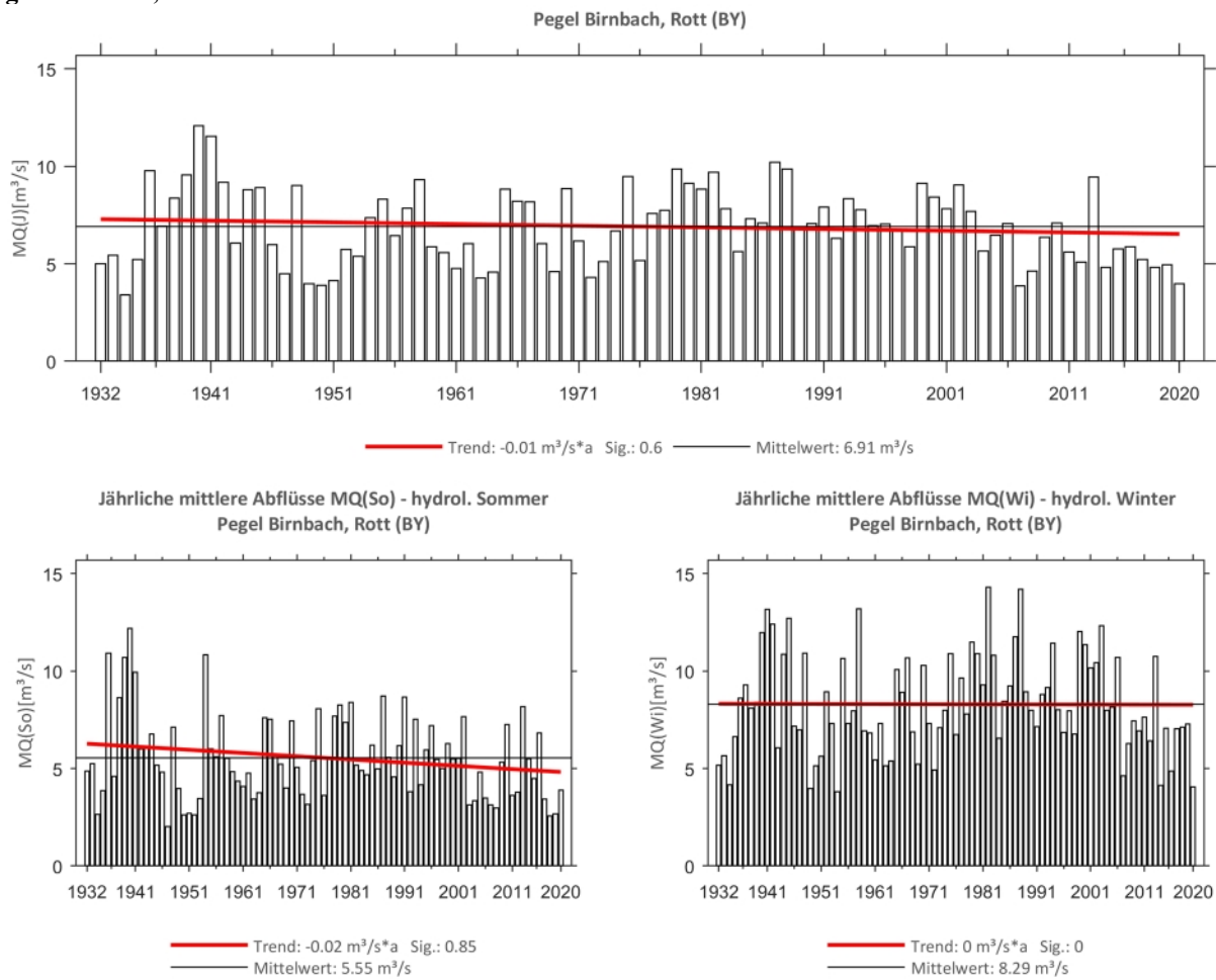
Abb. 102: Trenduntersuchungen von jährlichen mittleren Abflüssen für den Zeitraum 1932 bis 2020.
