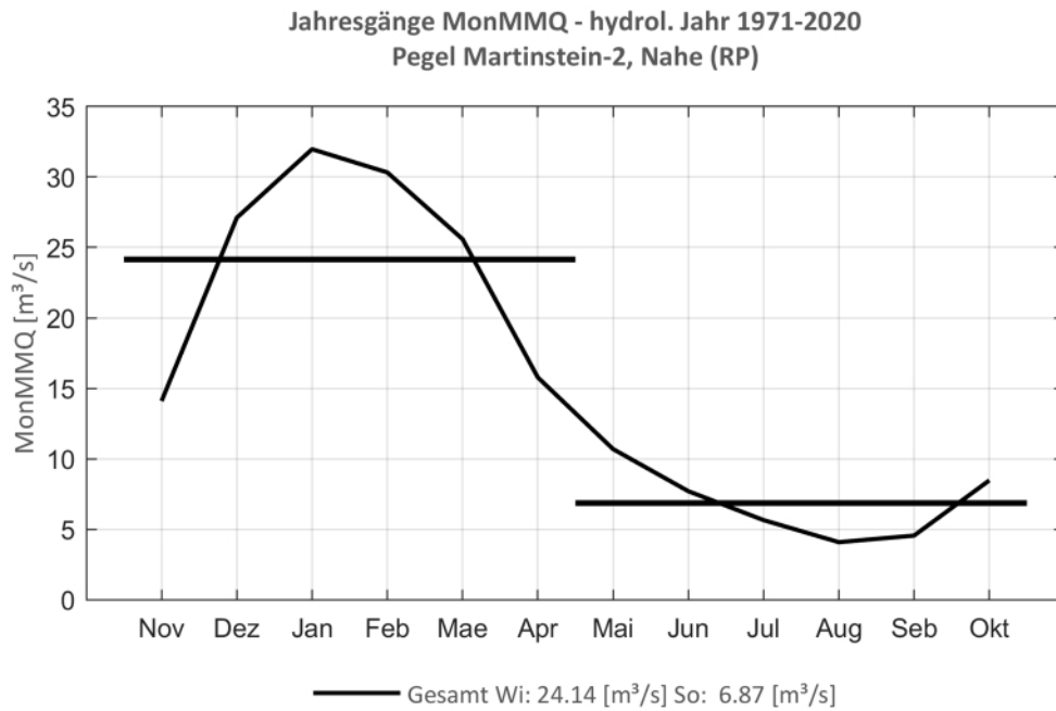
Abb. 256: Jahresgang des MonMMQ und Halbjahresmittel für 1971-2020.
