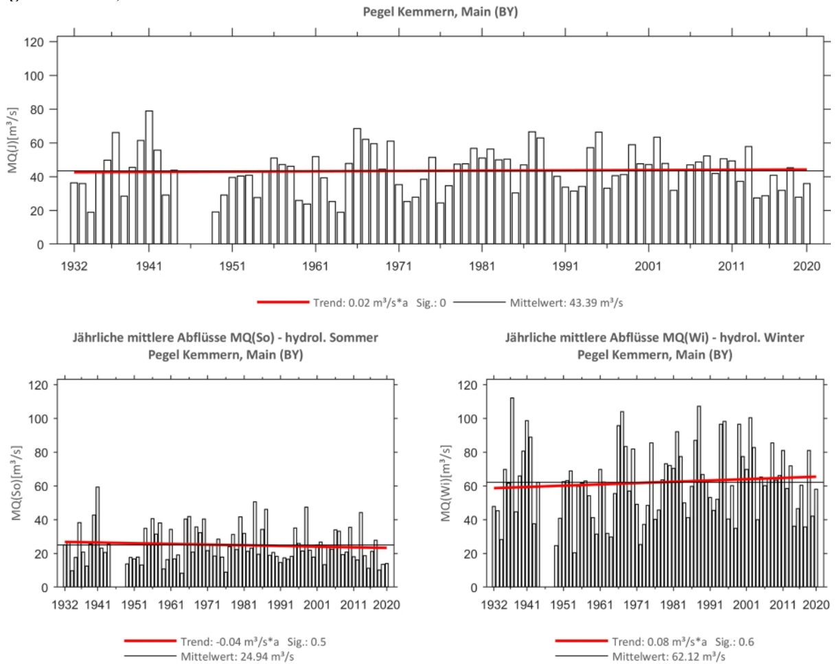
Abb. 160: Trenduntersuchungen von jährlichen mittleren Abflüssen für den Zeitraum 1932 bis 2020.
