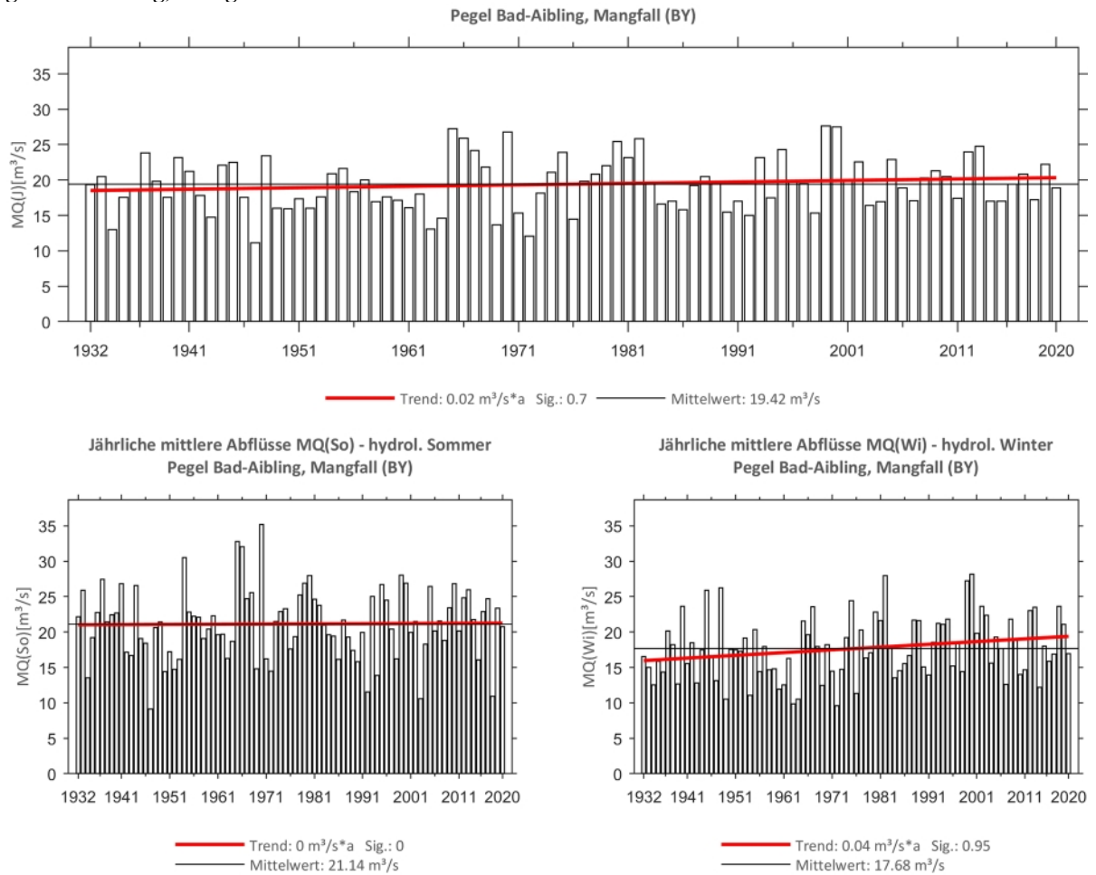
Abb. 100: Trenduntersuchungen von jährlichen mittleren Abflüssen für den Zeitraum 1932 bis 2020.
