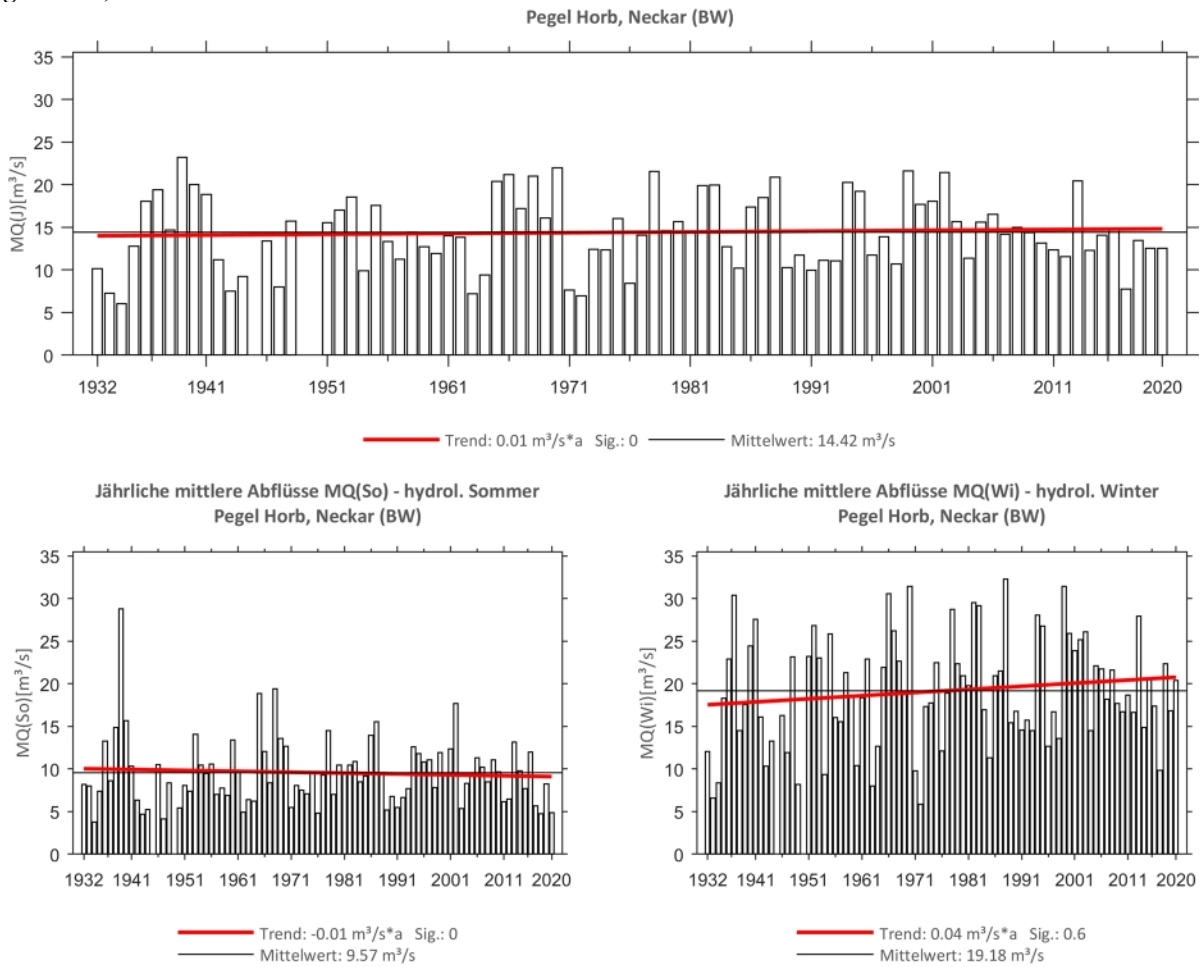
Abb. 26: Trenduntersuchungen von jährlichen mittleren Abflüssen für den Zeitraum 1932 bis 2020.
