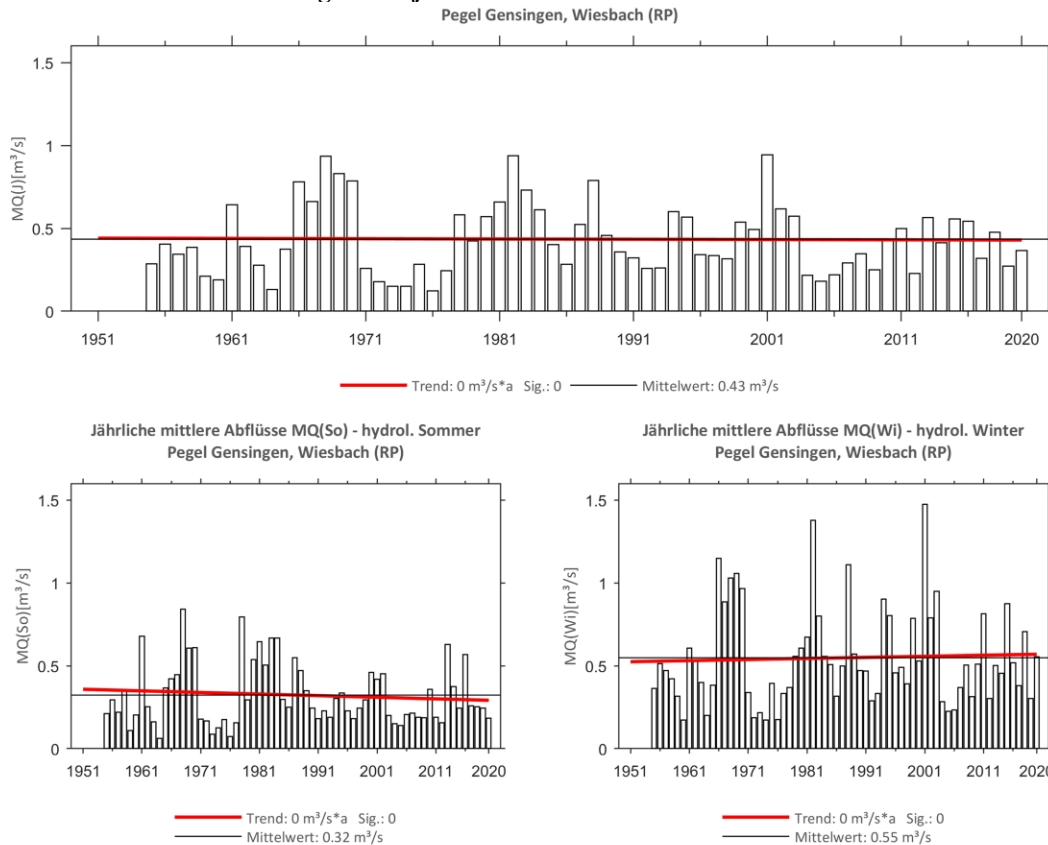
Abb. 247: Trenduntersuchungen von jährlichen mittleren Abflüssen für den Zeitraum 1955 bis 2020.
