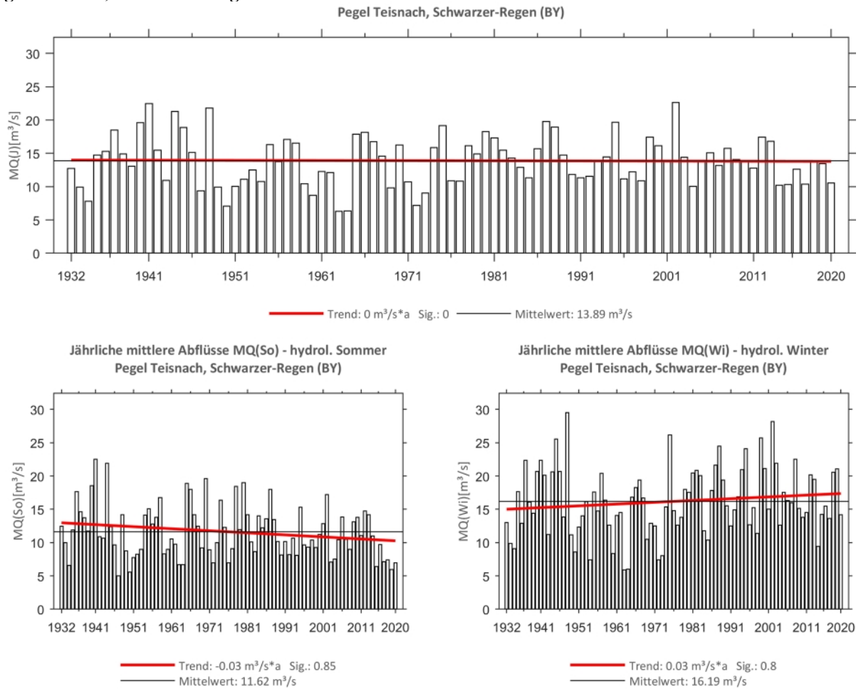
Abb. 76: Trenduntersuchungen von jährlichen mittleren Abflüssen für den Zeitraum 1932 bis 2020.
