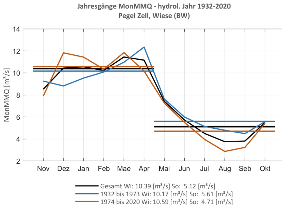
Abb. 21: Jahresgang des MonMMQ und Halbjahresmittel für 1932-2020 sowie 1932-1973 und 1974-2020.
