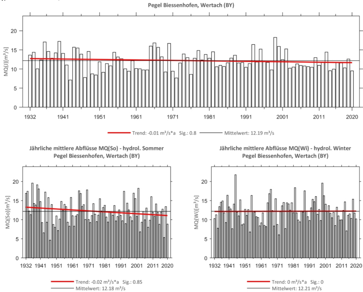
Abb. 78: Trenduntersuchungen von jährlichen mittleren Abflüssen für den Zeitraum 1932 bis 2020.
