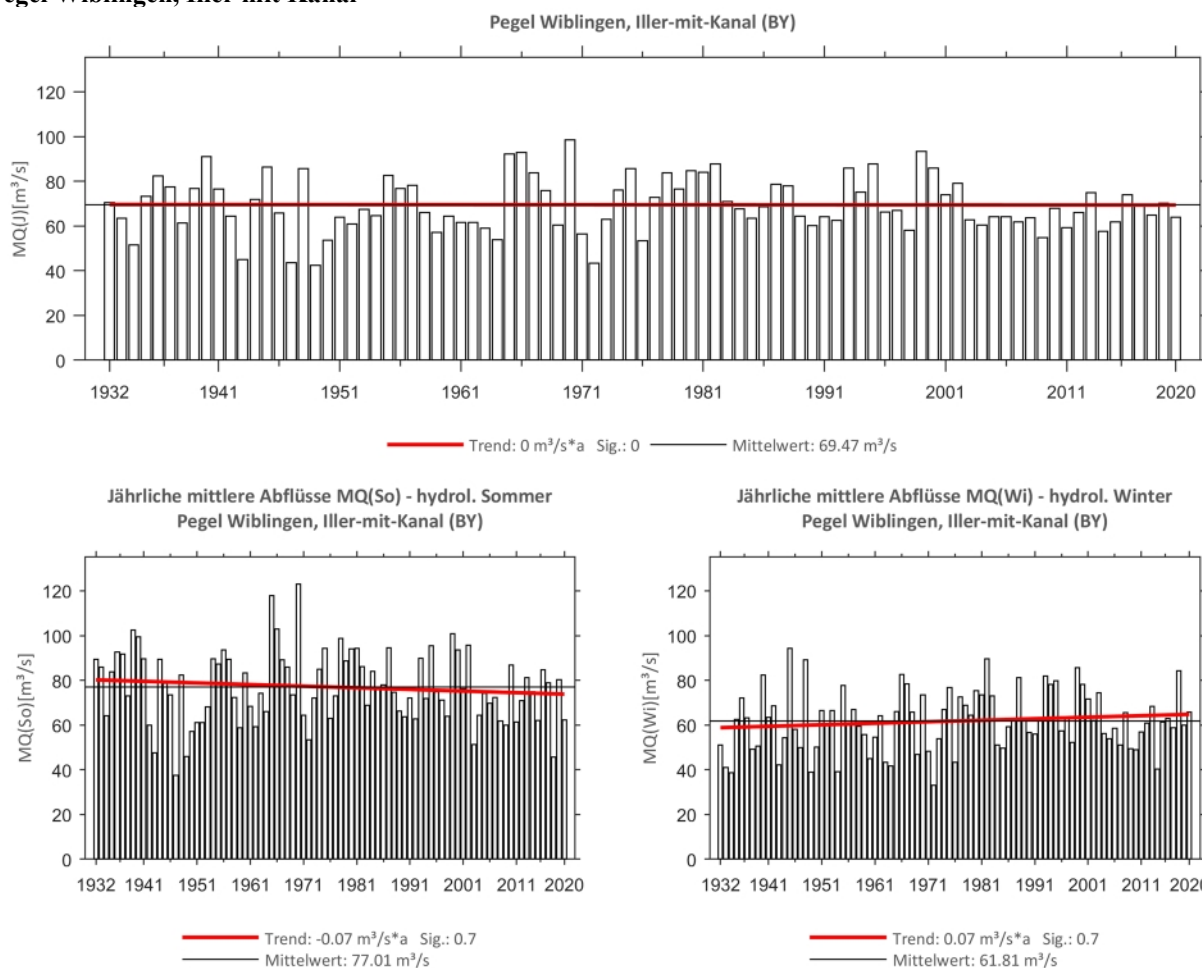
Abb. 94: Trenduntersuchungen von jährlichen mittleren Abflüssen für den Zeitraum 1932 bis 2020.
