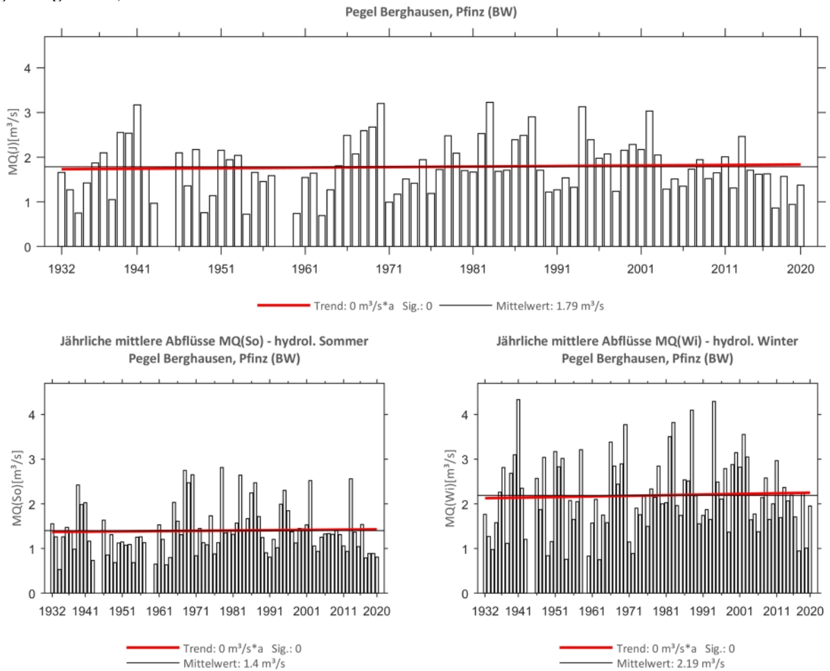
Abb. 4: Trenduntersuchungen von jährlichen mittleren Abflüssen für den Zeitraum 1932 bis 2020.
