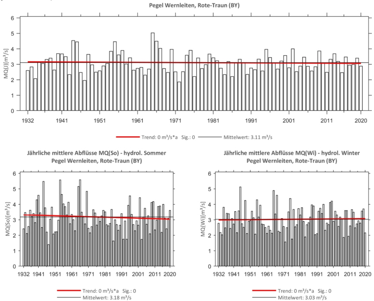
Abb. 140: Trenduntersuchungen von jährlichen mittleren Abflüssen für den Zeitraum 1932 bis 2020.
