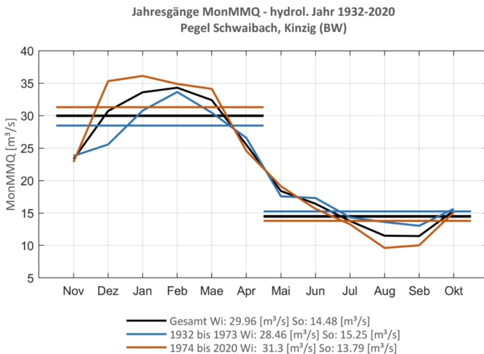
Abb. 19: Jahresgang des MonMMQ und Halbjahresmittel für 1932-2020 sowie 1932-1973 und 1974-2020.
