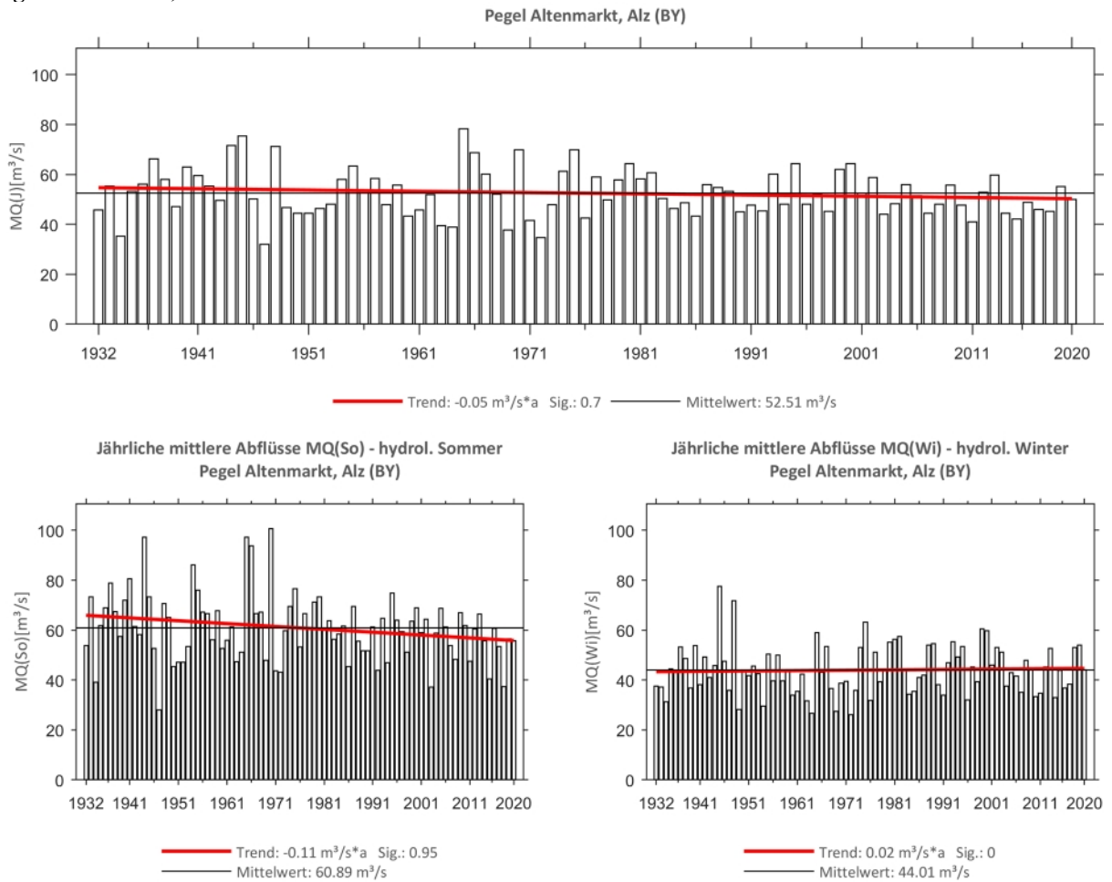
Abb. 96: Trenduntersuchungen von jährlichen mittleren Abflüssen für den Zeitraum 1932 bis 2020.
