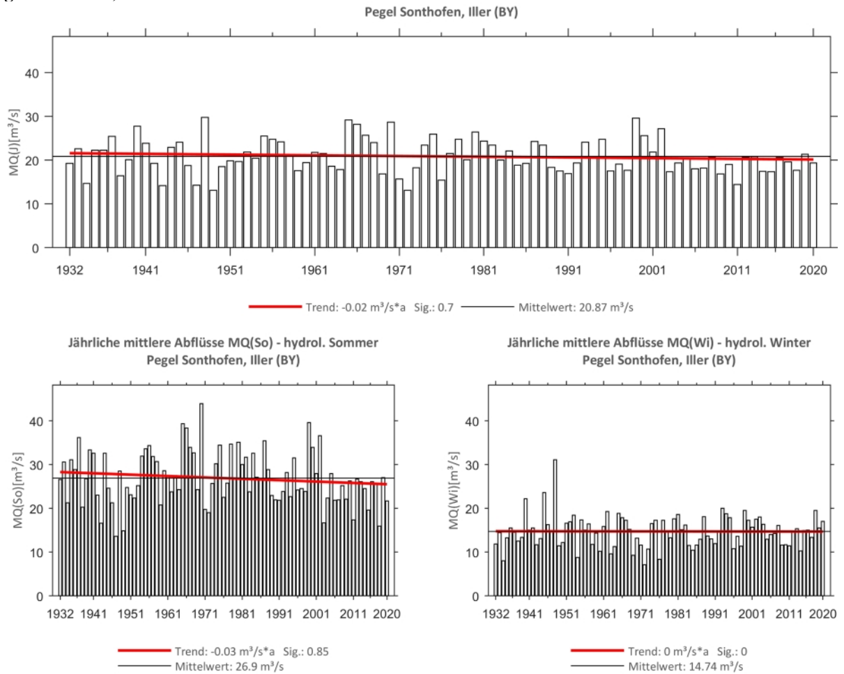
Abb. 92: Trenduntersuchungen von jährlichen mittleren Abflüssen für den Zeitraum 1932 bis 2020.
