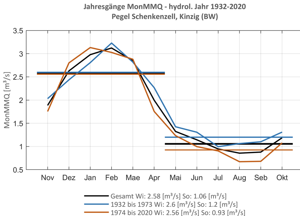
Abb. 17: Jahresgang des MonMMQ und Halbjahresmittel für 1932-2020 sowie 1932-1973 und 1974-2020.
