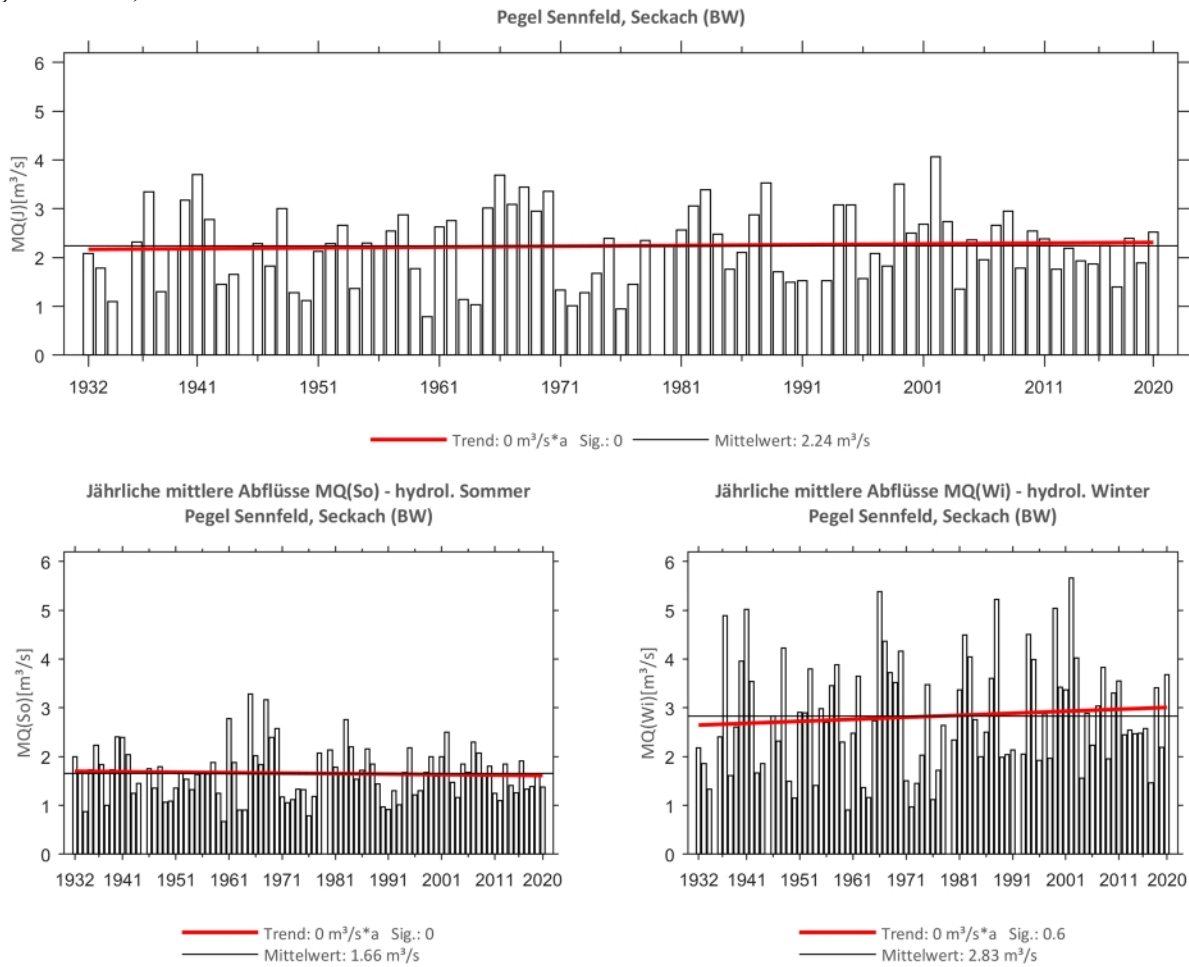
Abb. 42: Trenduntersuchungen von jährlichen mittleren Abflüssen für den Zeitraum 1932 bis 2020.
