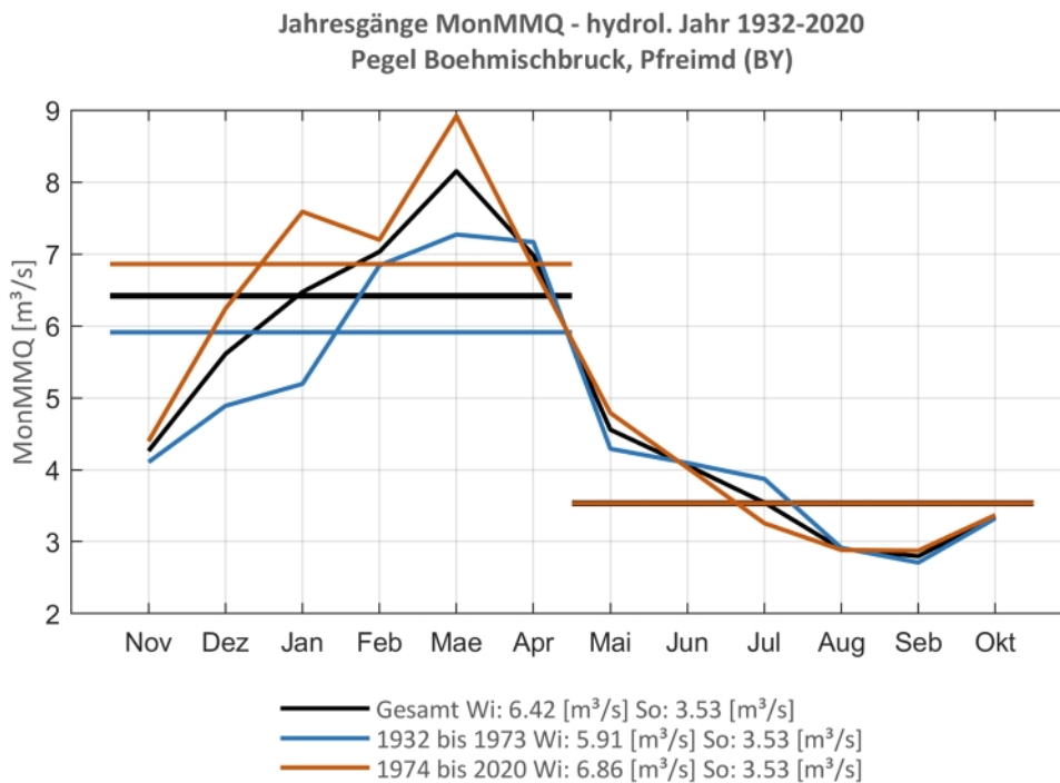
Abb. 65: Jahresgang des MonMMQ und Halbjahresmittel für 1932-2020 sowie 1932-1973 und 1974-2020
