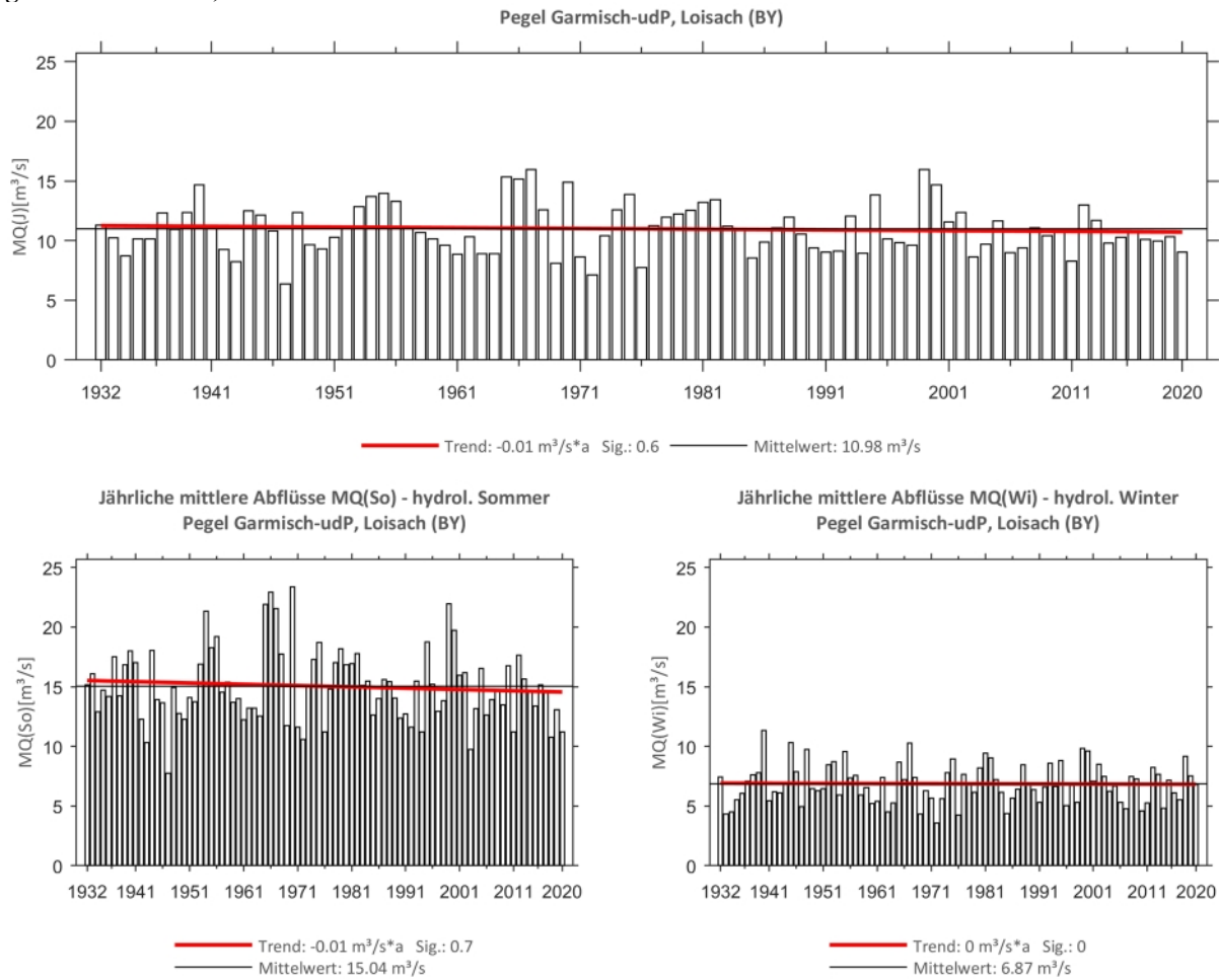
Abb. 110: Trenduntersuchungen von jährlichen mittleren Abflüssen für den Zeitraum 1932 bis 2020.
