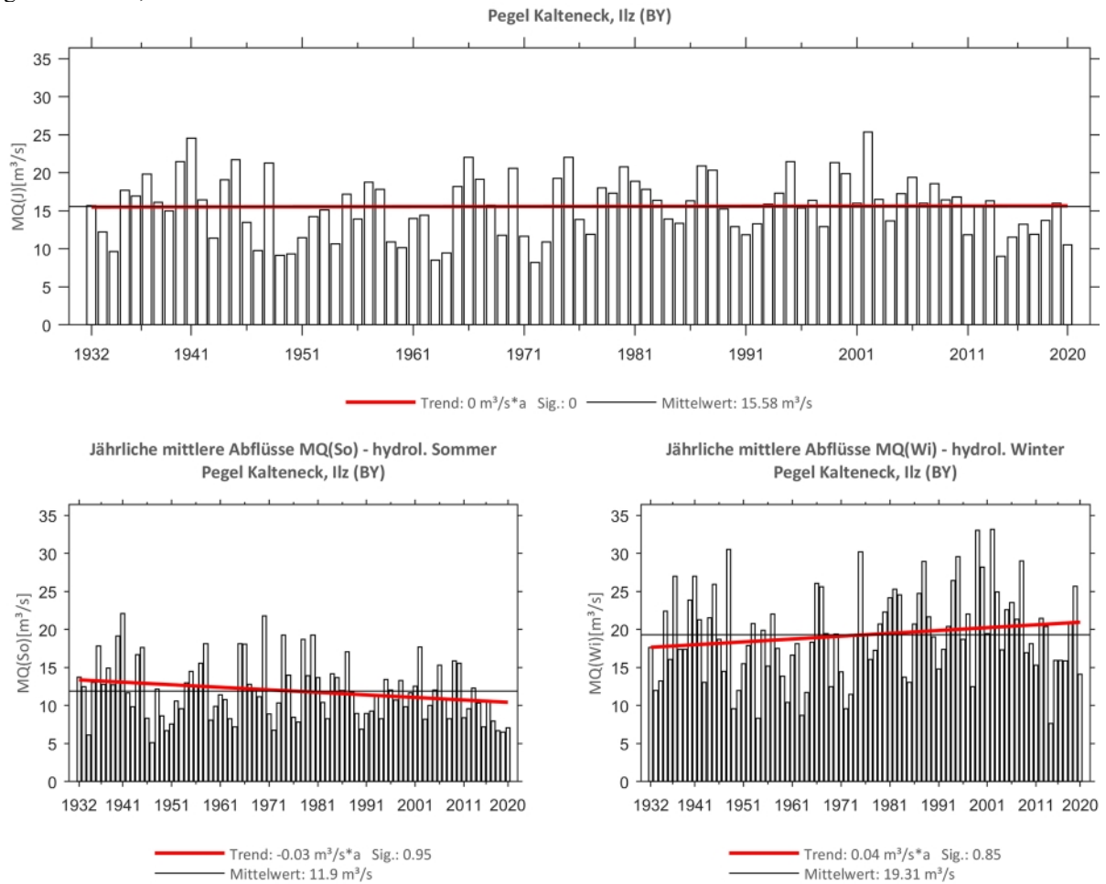
Abb. 72: Trenduntersuchungen von jährlichen mittleren Abflüssen für den Zeitraum 1932 bis 2020.
