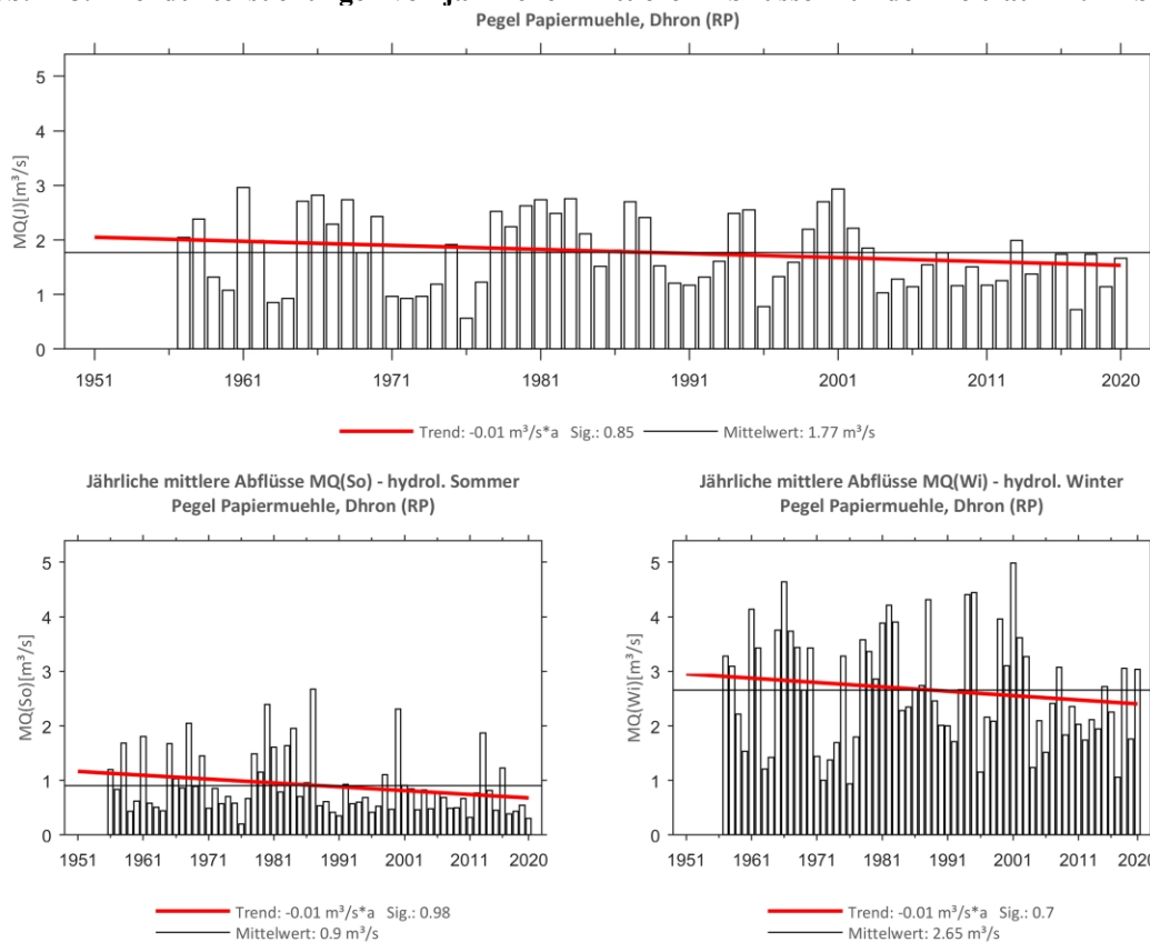
Abb. 219: Trenduntersuchungen von jährlichen mittleren Abflüssen für den Zeitraum 1957 bis 2020.
