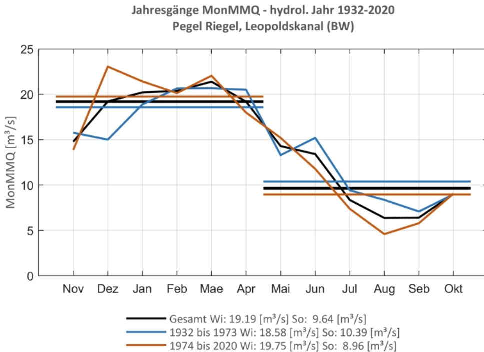
Abb. 15: Jahresgang des MonMMQ und Halbjahresmittel für 1932-2020 sowie 1932-1973 und 1974-2020.
