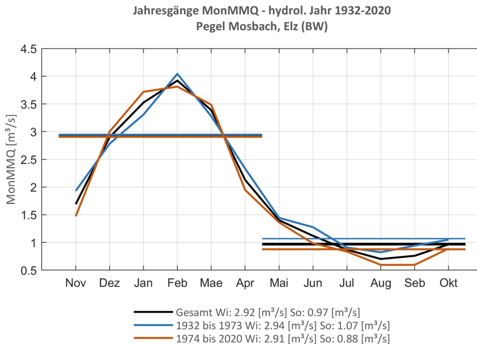
Abb. 33: Jahresgang des MonMMQ und Halbjahresmittel für 1932-2020 sowie 1932-1973 und 1974-2020.
