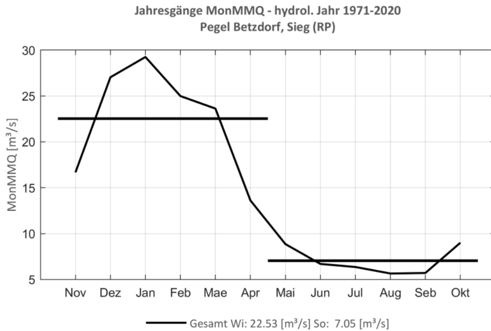
Abb. 198: Jahresgang des MonMMQ und Halbjahresmittel für 1971-2020.
