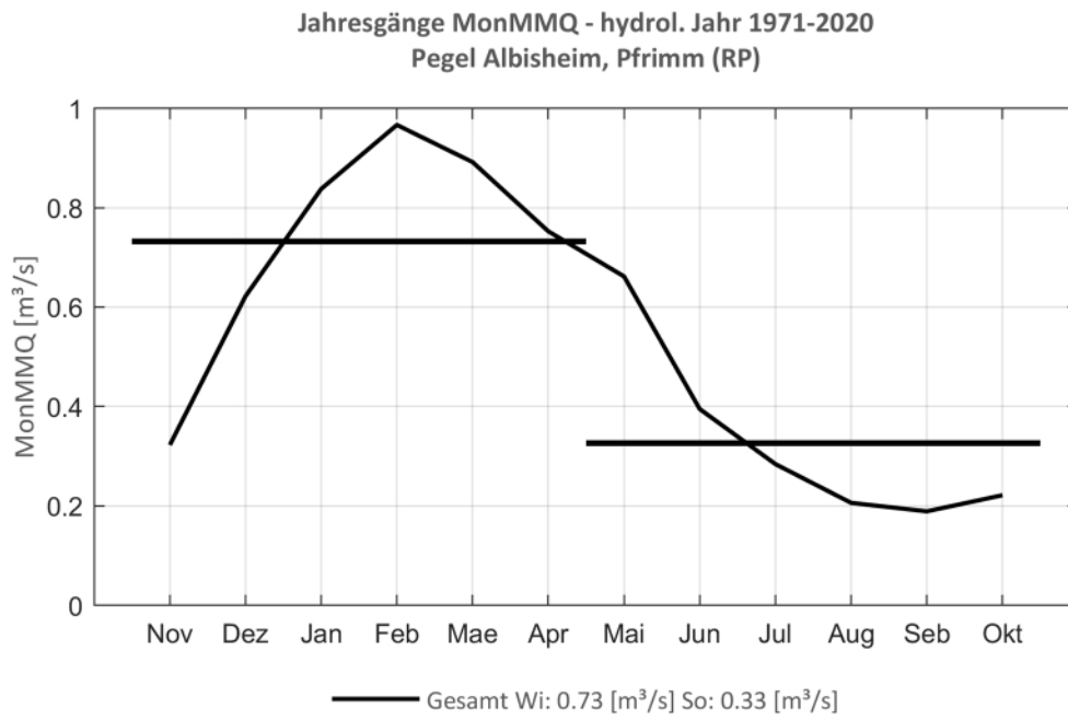
Abb. 230: Jahresgang des MonMMQ und Halbjahresmittel für 1971-2020.
