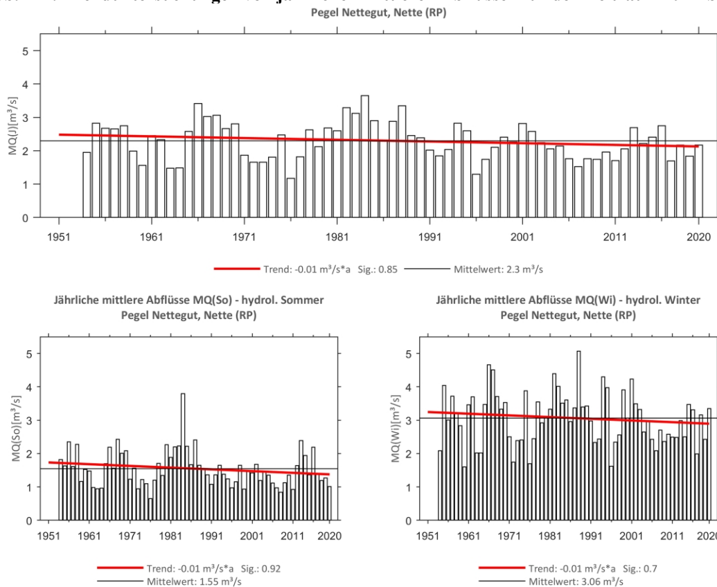
Abb. 215: Trenduntersuchungen von jährlichen mittleren Abflüssen für den Zeitraum 1954 bis 2020.
