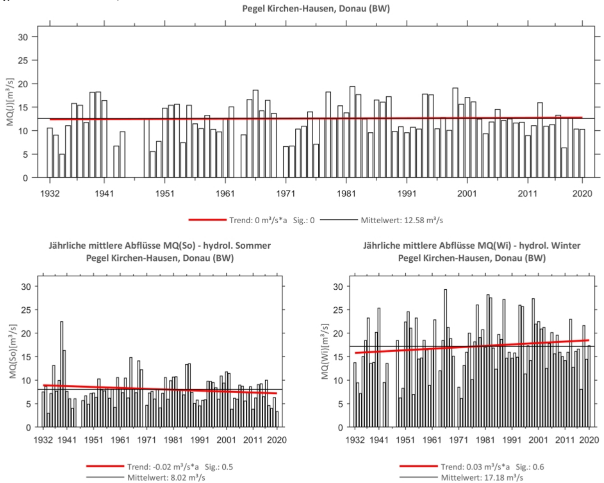
Abb. 56: Trenduntersuchungen von jährlichen mittleren Abflüssen für den Zeitraum 1932 bis 2020.
