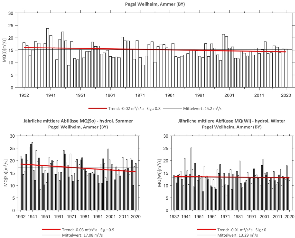
Abb. 138: Trenduntersuchungen von jährlichen mittleren Abflüssen für den Zeitraum 1932 bis 2020.
