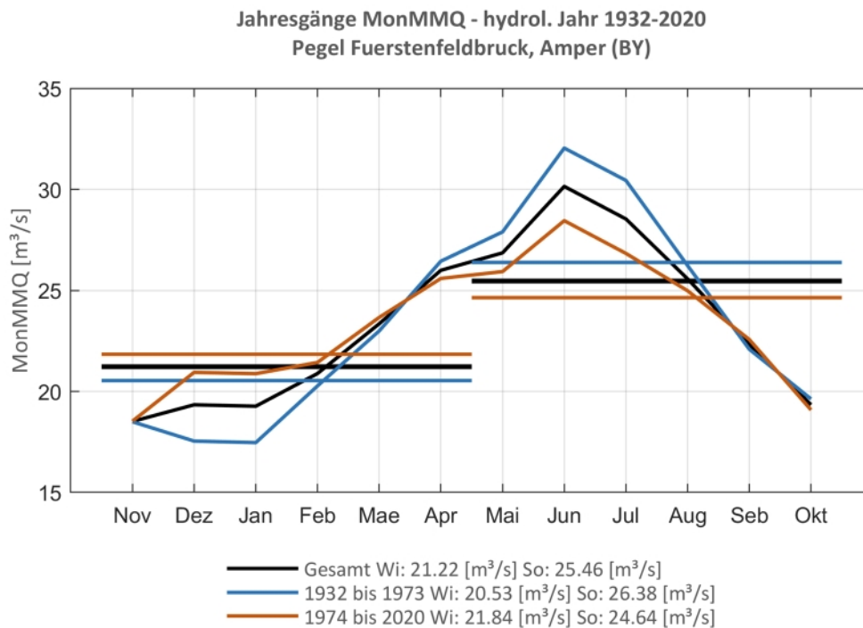
Abb. 109: Jahresgang des MonMMQ und Halbjahresmittel für 1932-2020 sowie 1932-1973 und 1974-2020
