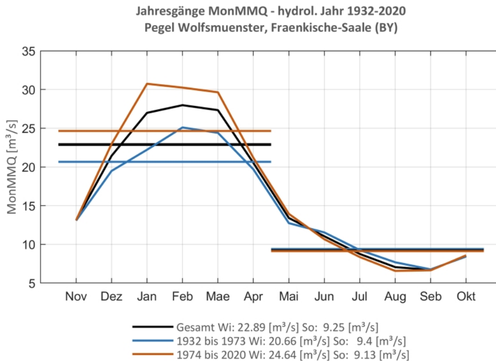
Abb. 181: Jahresgang des MonMMQ und Halbjahresmittel für 1932-2020 sowie 1932-1973 und 1974-2020
