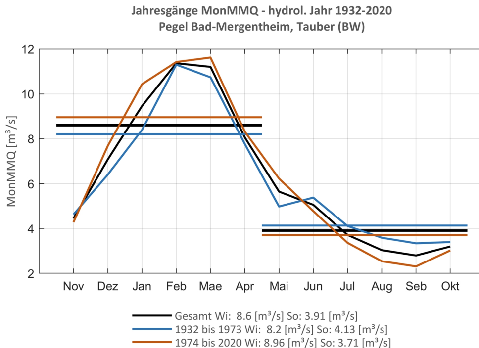
Abb. 61: Jahresgang des MonMMQ und Halbjahresmittel für 1932-2020 sowie 1932-1973 und 1974-2020.
