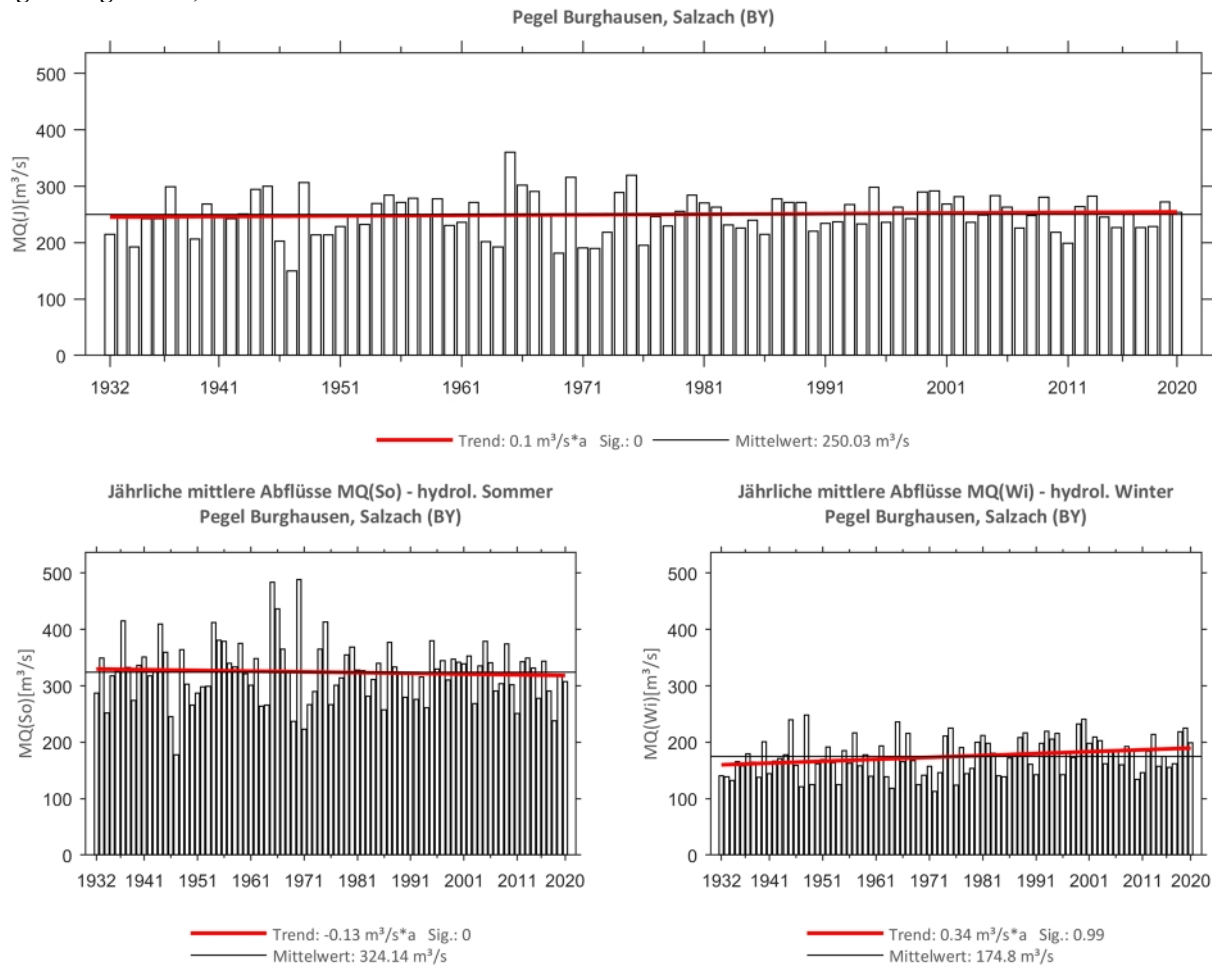
Abb. 104: Trenduntersuchungen von jährlichen mittleren Abflüssen für den Zeitraum 1932 bis 2020.
