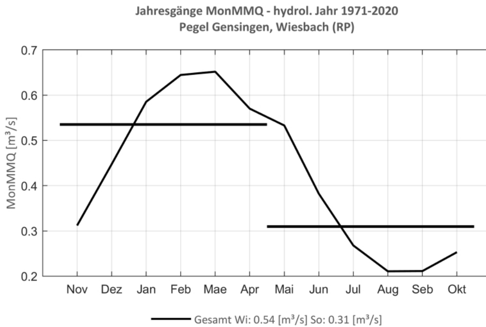
Abb. 248: Jahresgang des MonMMQ und Halbjahresmittel für 1971-2020.
