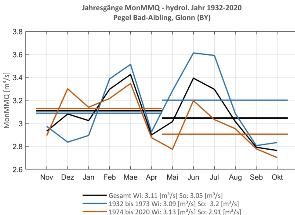
Abb. 99: Jahresgang des MonMMQ und Halbjahresmittel für 1932-2020 sowie 1932-1973 und 1974-2020
