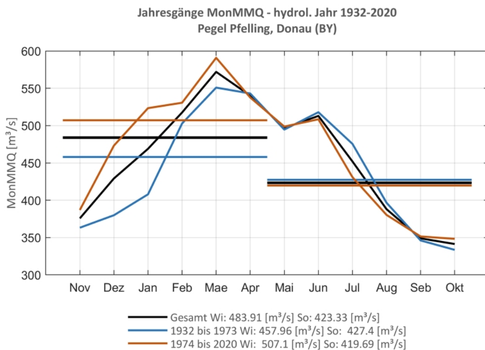
Abb. 151: Jahresgang des MonMMQ und Halbjahresmittel für 1932-2020 sowie 1932-1973 und 1974-2020
