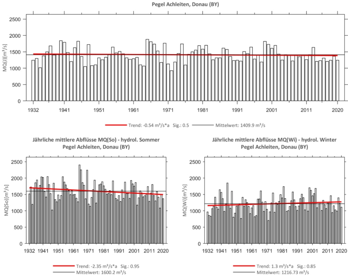
Abb. 62: Trenduntersuchungen von jährlichen mittleren Abflüssen für den Zeitraum 1932 bis 2020.
