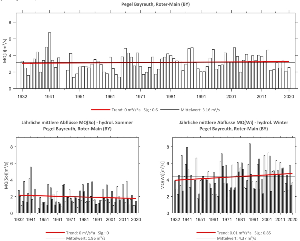
Abb. 156: Trenduntersuchungen von jährlichen mittleren Abflüssen für den Zeitraum 1932 bis 2020.
