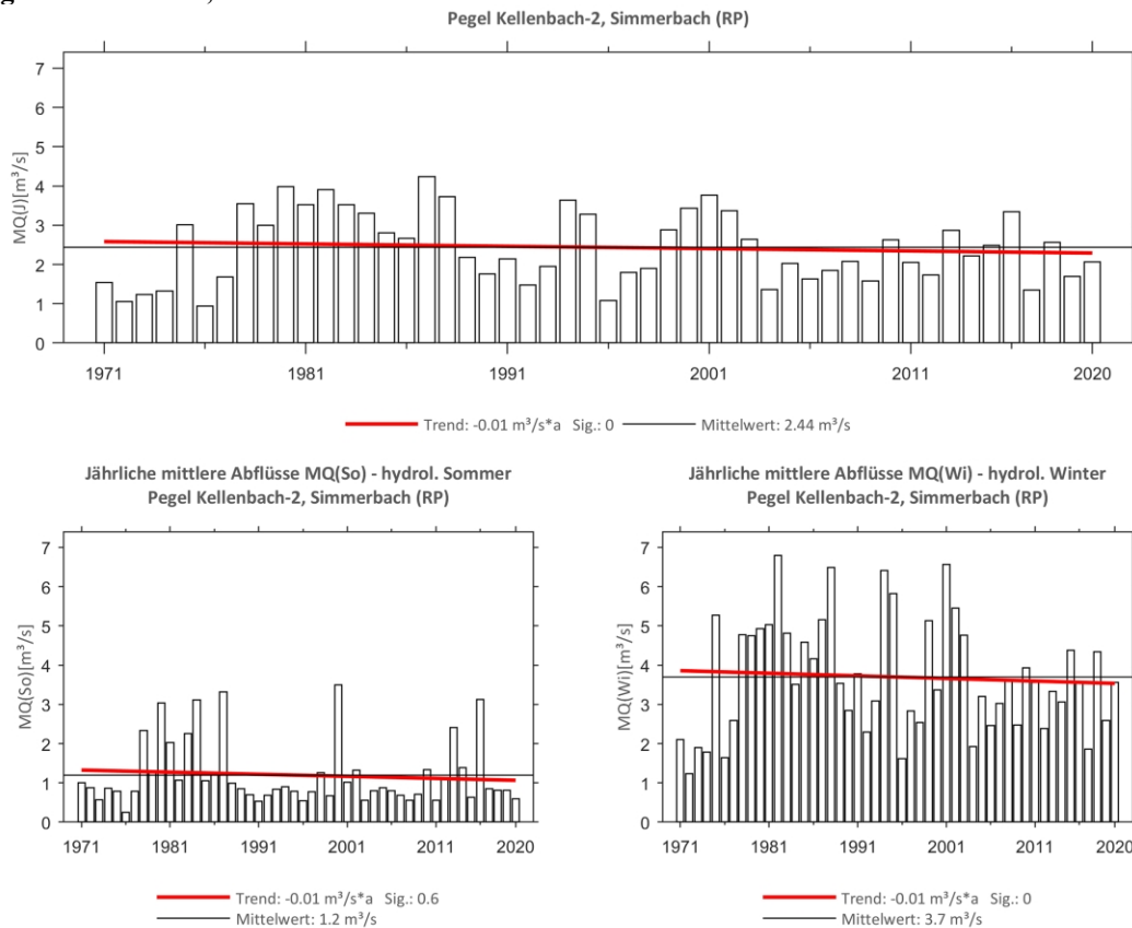
Abb. 250: Trenduntersuchungen von jährlichen mittleren Abflüssen für den Zeitraum 1971 bis 2020. Pegel Kellenbach-2, Simmerbach (RP)
