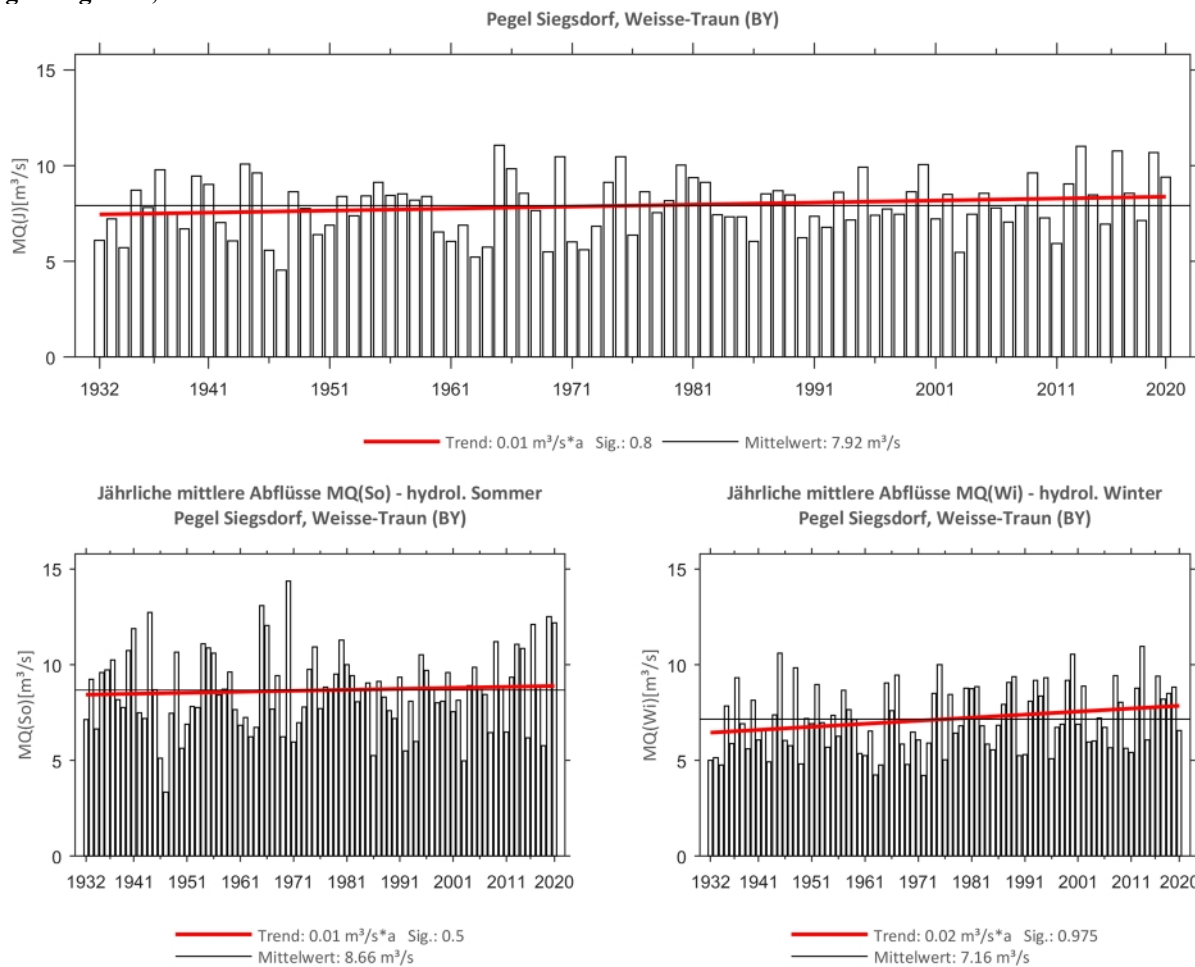
Abb. 130: Trenduntersuchungen von jährlichen mittleren Abflüssen für den Zeitraum 1932 bis 2020.
