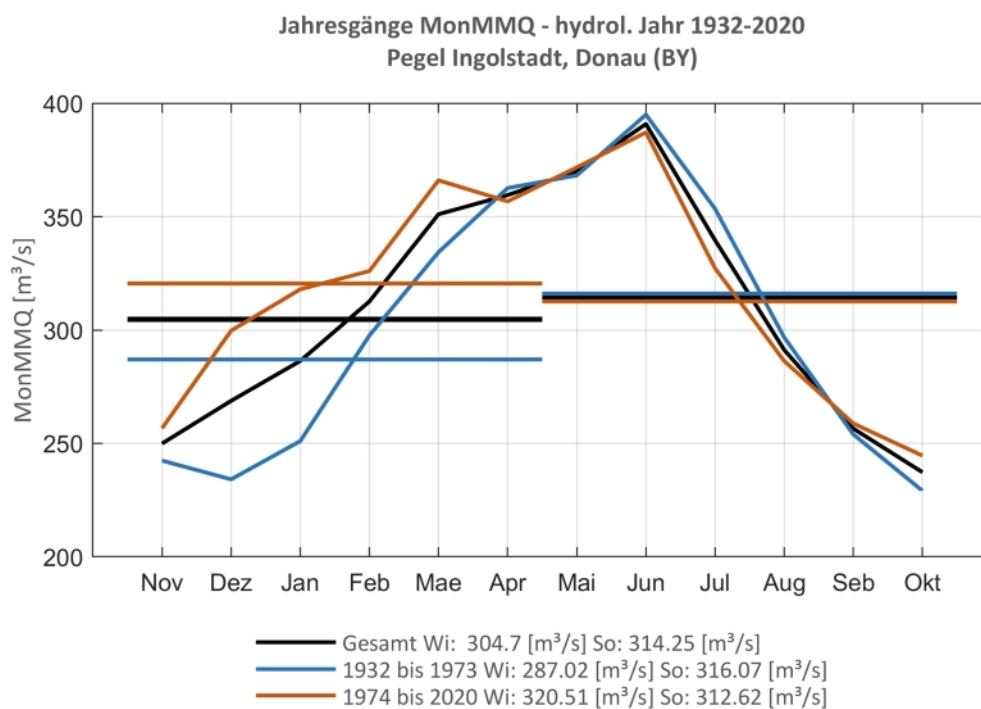
Abb. 143: Jahresgang des MonMMQ und Halbjahresmittel für 1932-2020 sowie 1932-1973 und 1974-2020
