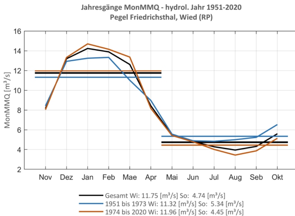
Abb. 207: Jahresgang des MonMMQ und Halbjahresmittel für 1951-2020 sowie 1951-1973 und 1974-2020.
