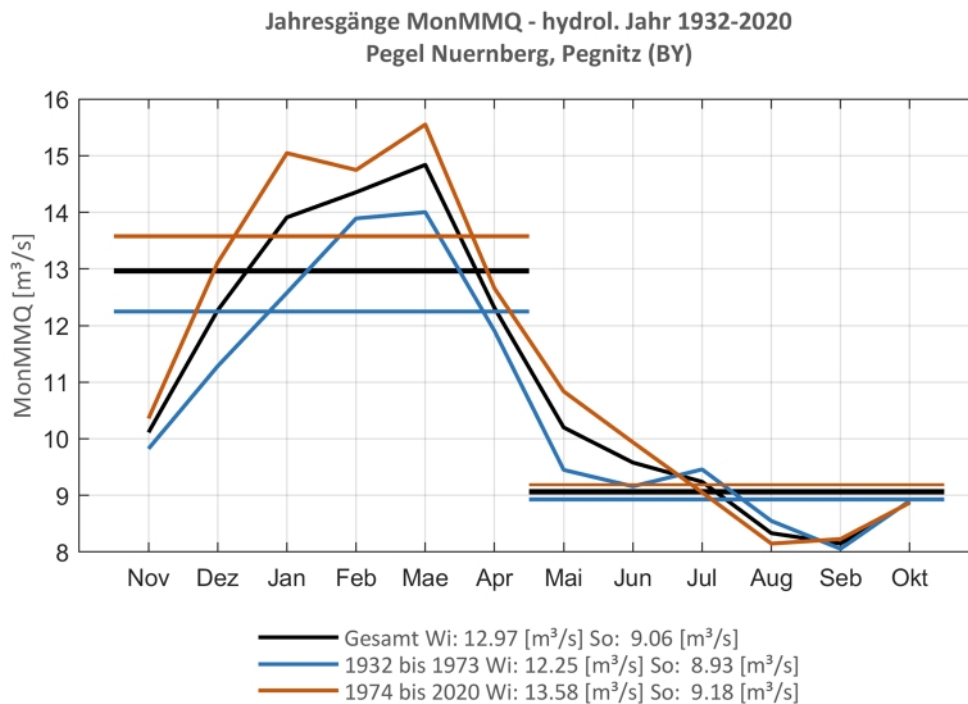
Abb. 169: Jahresgang des MonMMQ und Halbjahresmittel für 1932-2020 sowie 1932-1973 und 1974-2020
