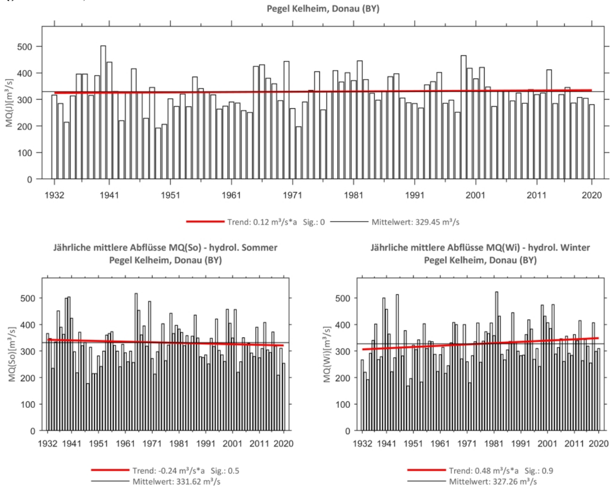
Abb. 144: Trenduntersuchungen von jährlichen mittleren Abflüssen für den Zeitraum 1932 bis 2020.
