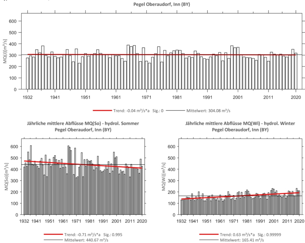
Abb. 122: Trenduntersuchungen von jährlichen mittleren Abflüssen für den Zeitraum 1932 bis 2020.
