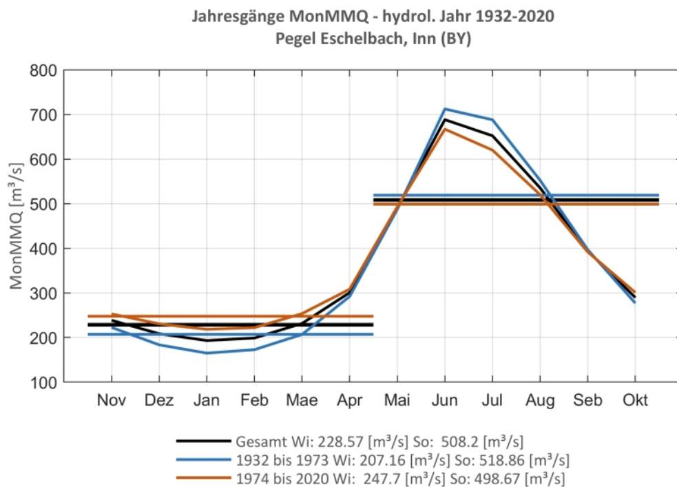
Abb. 107: Jahresgang des MonMMQ und Halbjahresmittel für 1932-2020 sowie 1932-1973 und 1974-2020
