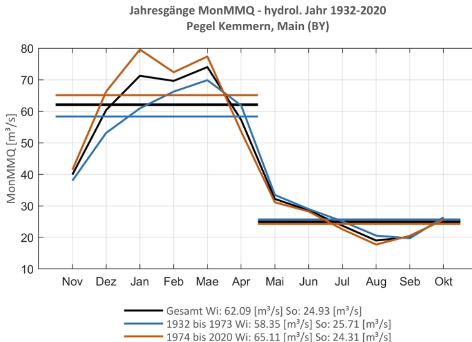
Abb. 161: Jahresgang des MonMMQ und Halbjahresmittel für 1932-2020 sowie 1932-1973 und 1974-2020
