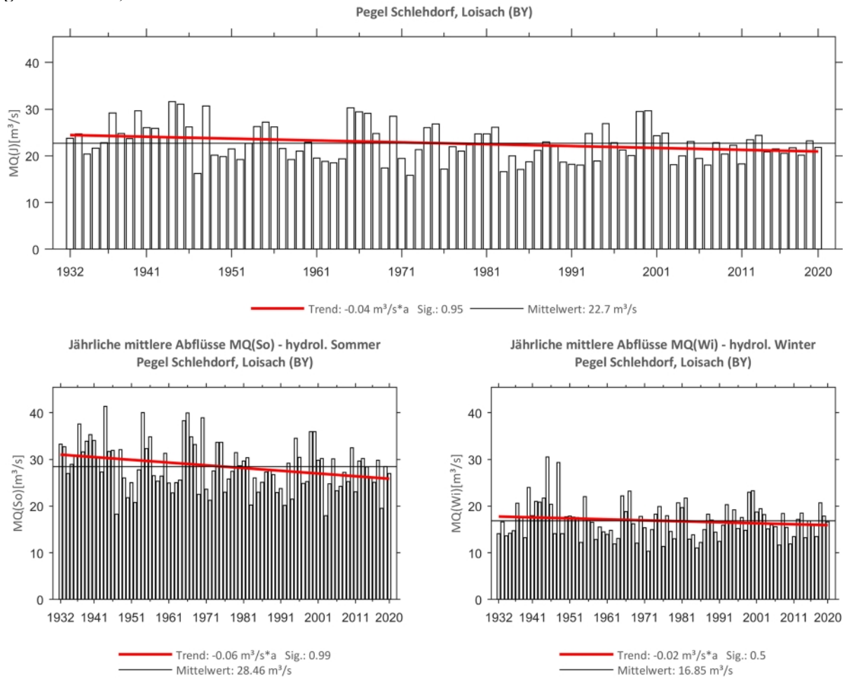
Abb. 128: Trenduntersuchungen von jährlichen mittleren Abflüssen für den Zeitraum 1932 bis 2020.
