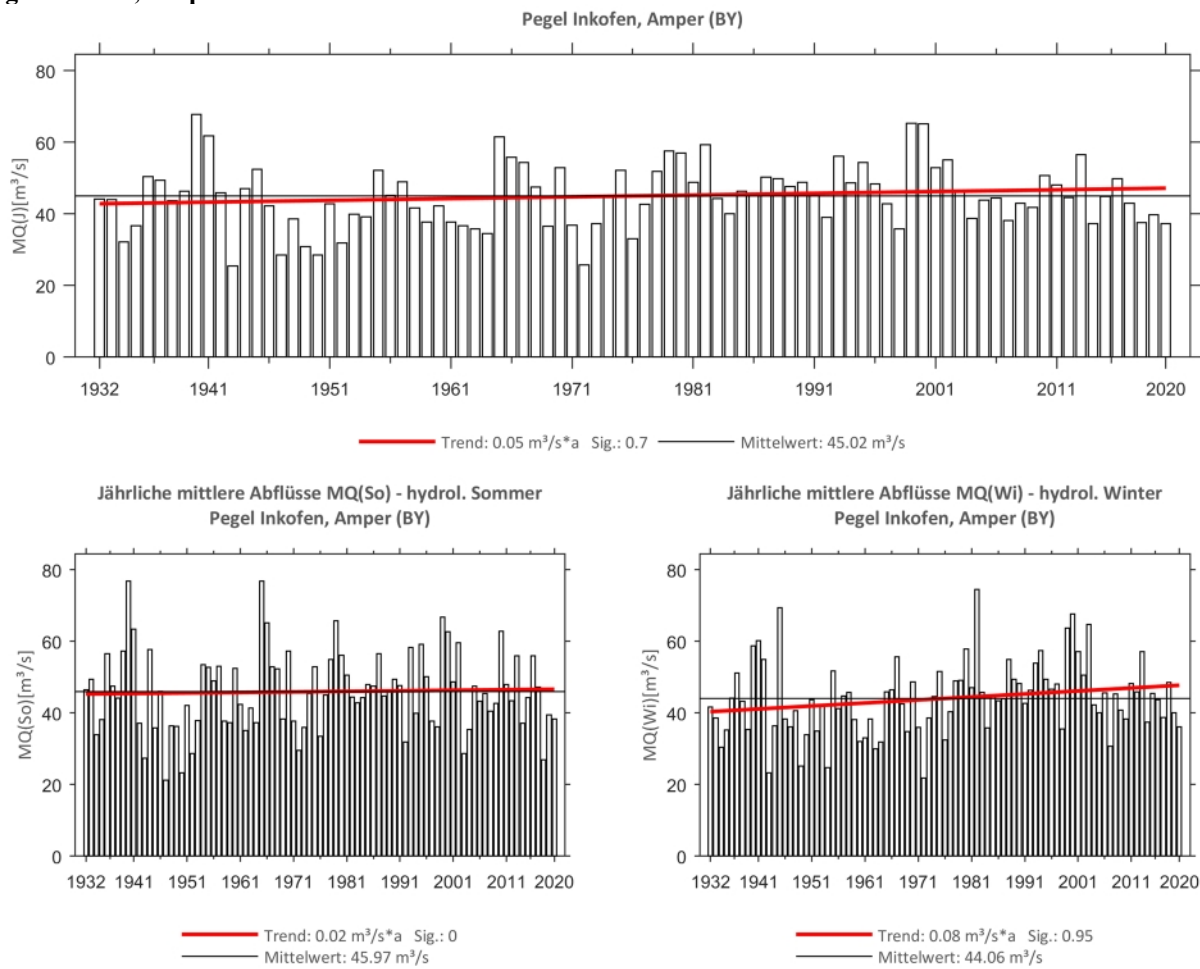
Abb. 114: Trenduntersuchungen von jährlichen mittleren Abflüssen für den Zeitraum 1932 bis 2020.
