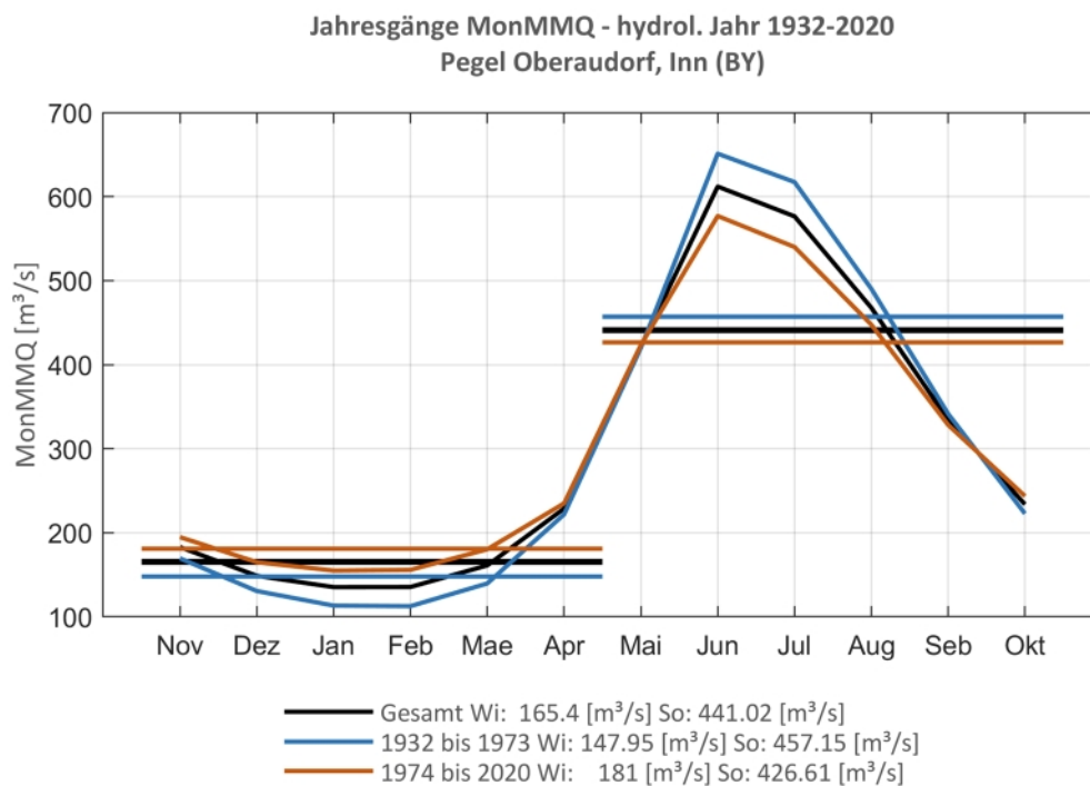
Abb. 123: Jahresgang des MonMMQ und Halbjahresmittel für 1932-2020 sowie 1932-1973 und 1974-2020
