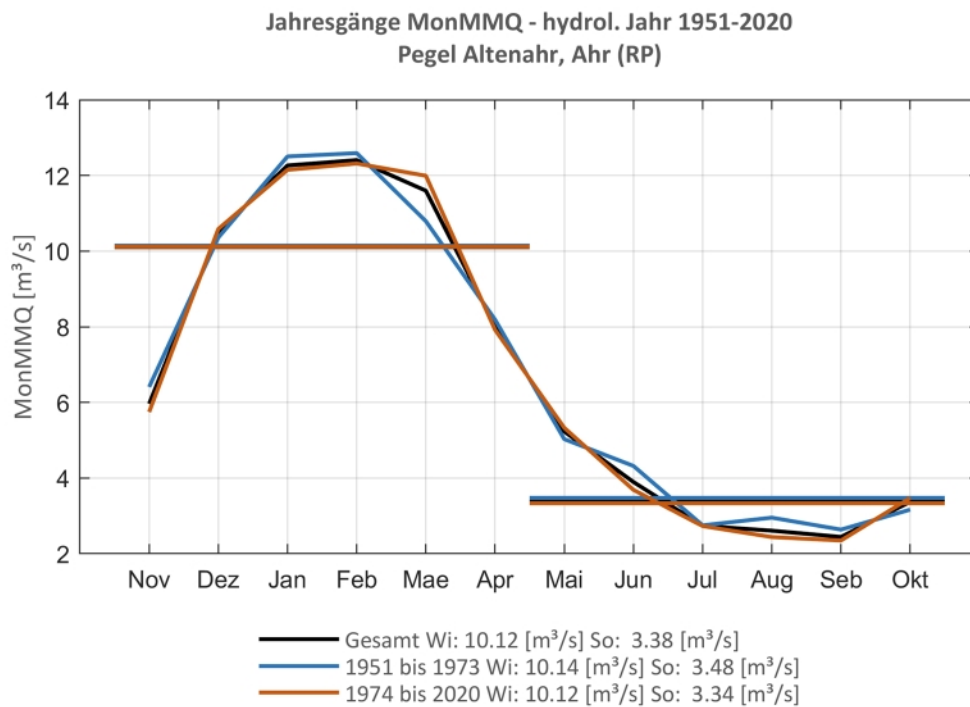
Abb. 195: Jahresgang des MonMMQ und Halbjahresmittel für 1951-2020 sowie 1951-1973 und 1974-2020.
