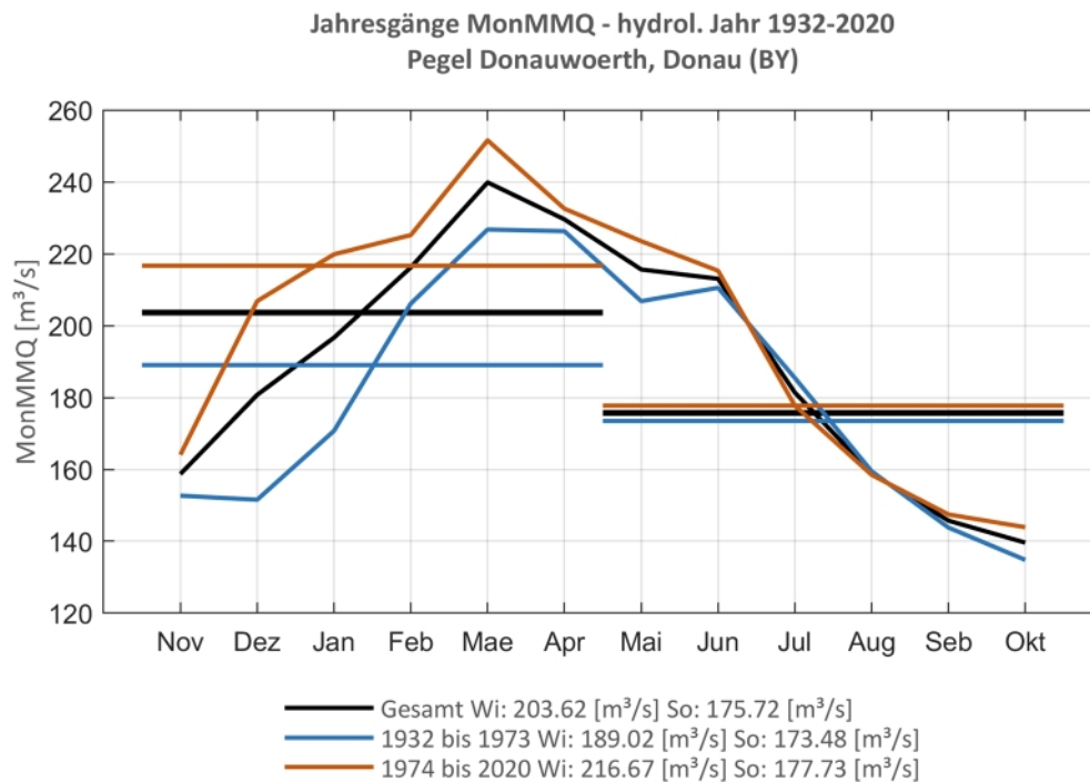
Abb. 81: Jahresgang des MonMMQ und Halbjahresmittel für 1932-2020 sowie 1932-1973 und 1974-2020
