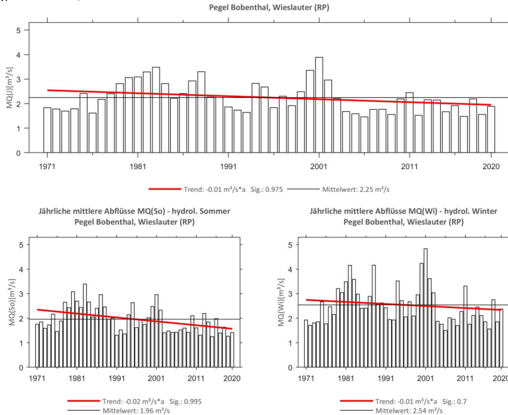
Abb. 232: Trenduntersuchungen von jährlichen mittleren Abflüssen für den Zeitraum 1971 bis 2020.
