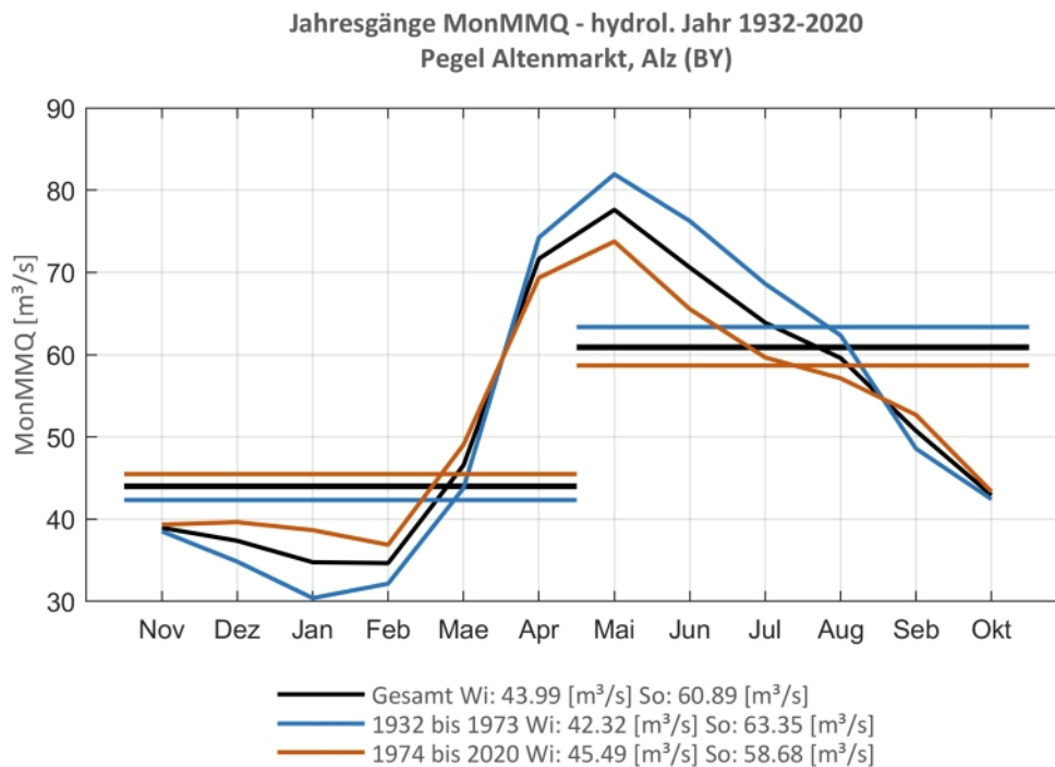
Abb. 97: Jahresgang des MonMMQ und Halbjahresmittel für 1932-2020 sowie 1932-1973 und 1974-2020
