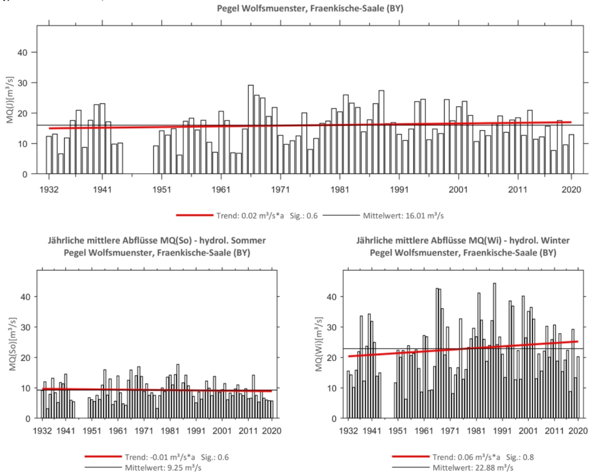
Abb. 180: Trenduntersuchungen von jährlichen mittleren Abflüssen für den Zeitraum 1932 bis 2020.
