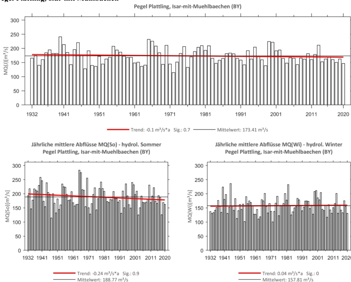
Abb. 126: Trenduntersuchungen von jährlichen mittleren Abflüssen für den Zeitraum 1932 bis 2020.
