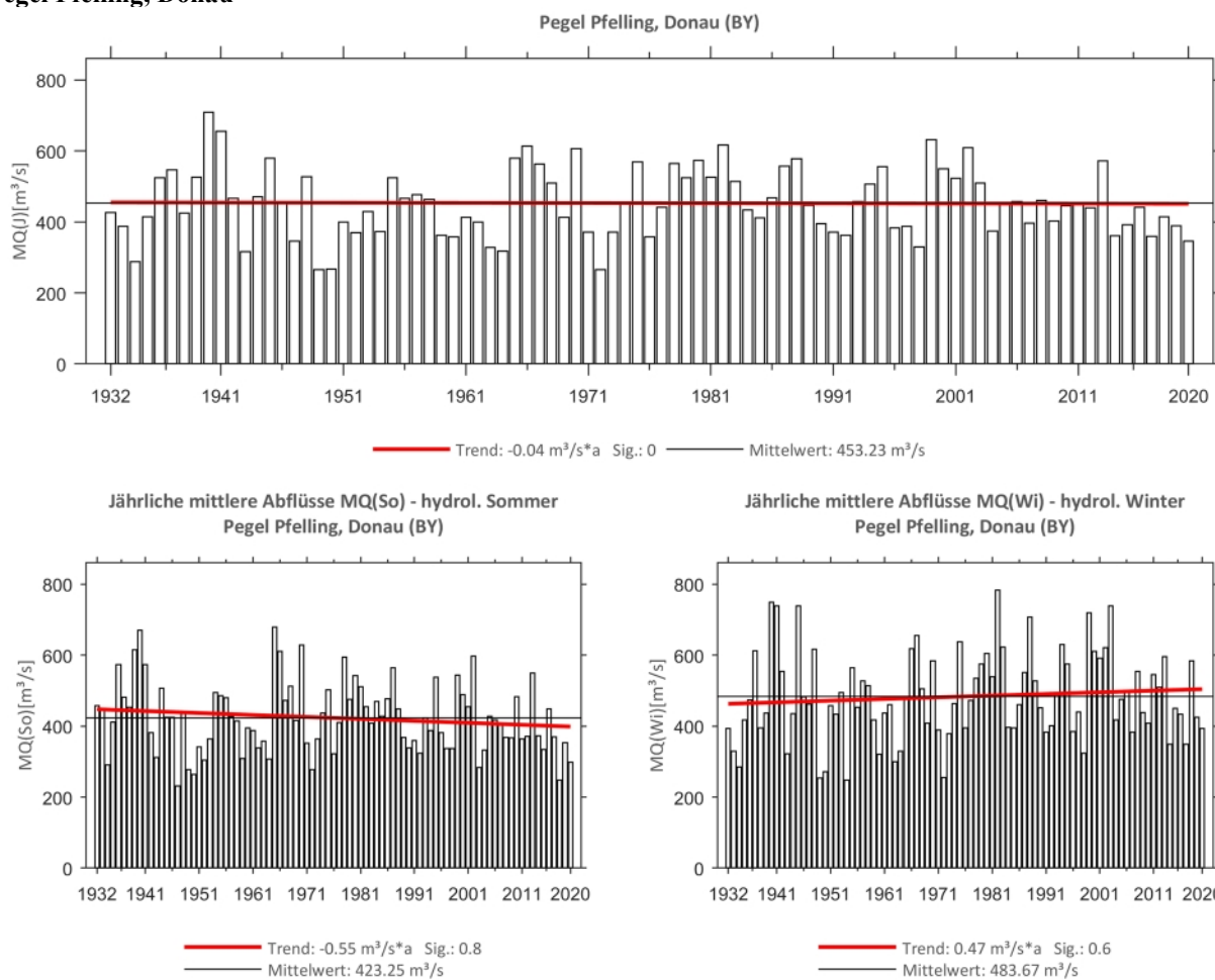
Abb. 150: Trenduntersuchungen von jährlichen mittleren Abflüssen für den Zeitraum 1932 bis 2020.
