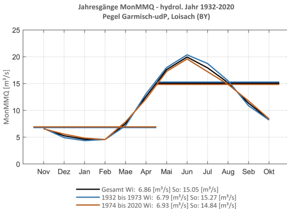
Abb. 111: Jahresgang des MonMMQ und Halbjahresmittel für 1932-2020 sowie 1932-1973 und 1974-2020
