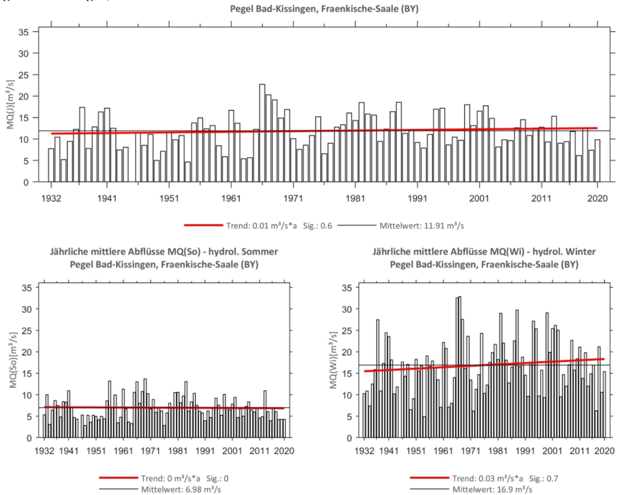
Abb. 176: Trenduntersuchungen von jährlichen mittleren Abflüssen für den Zeitraum 1932 bis 2020.
