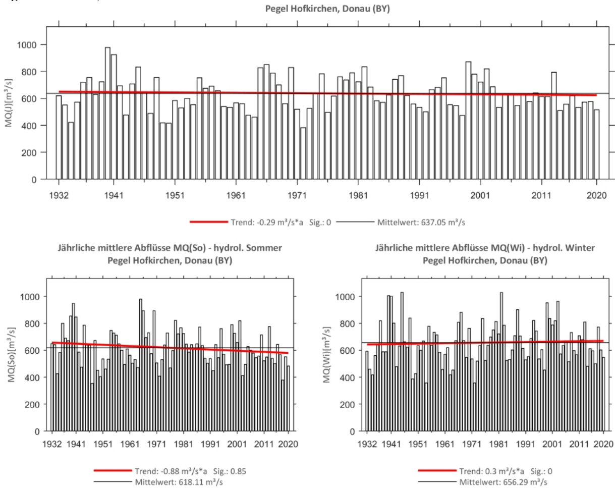
Abb. 70: Trenduntersuchungen von jährlichen mittleren Abflüssen für den Zeitraum 1932 bis 2020.
