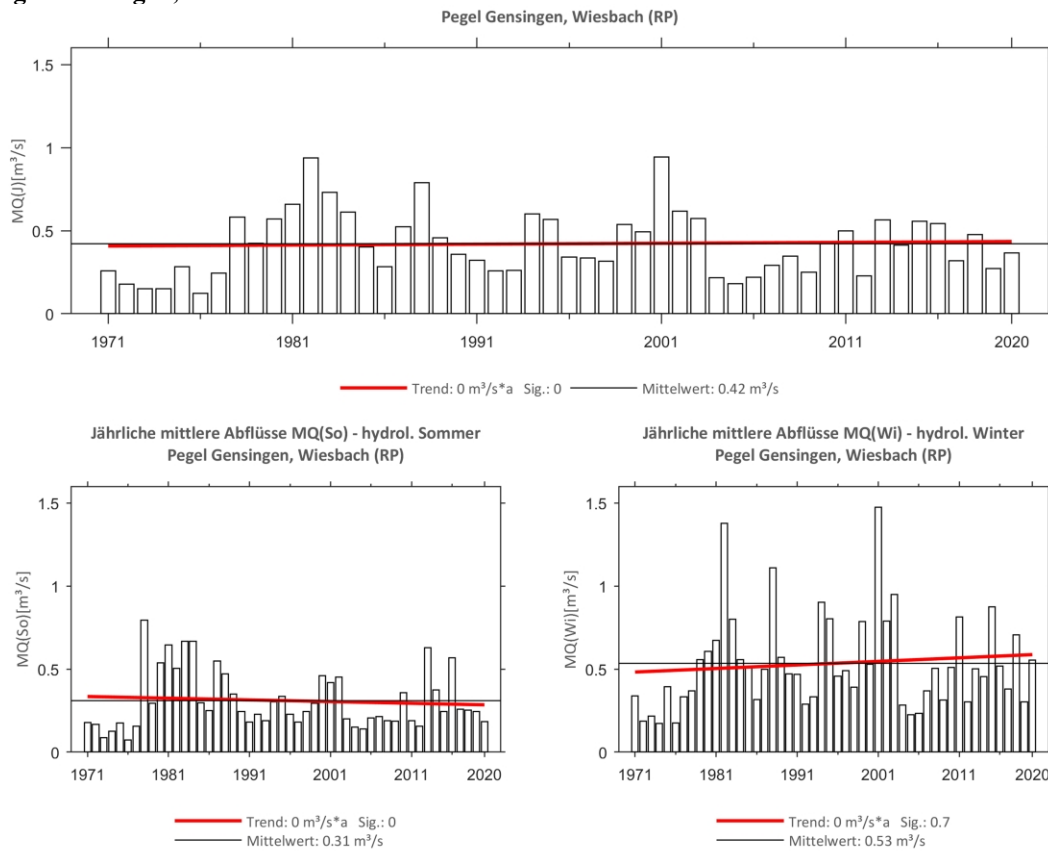
Abb. 246: Trenduntersuchungen von jährlichen mittleren Abflüssen für den Zeitraum 1971 bis 2020.
