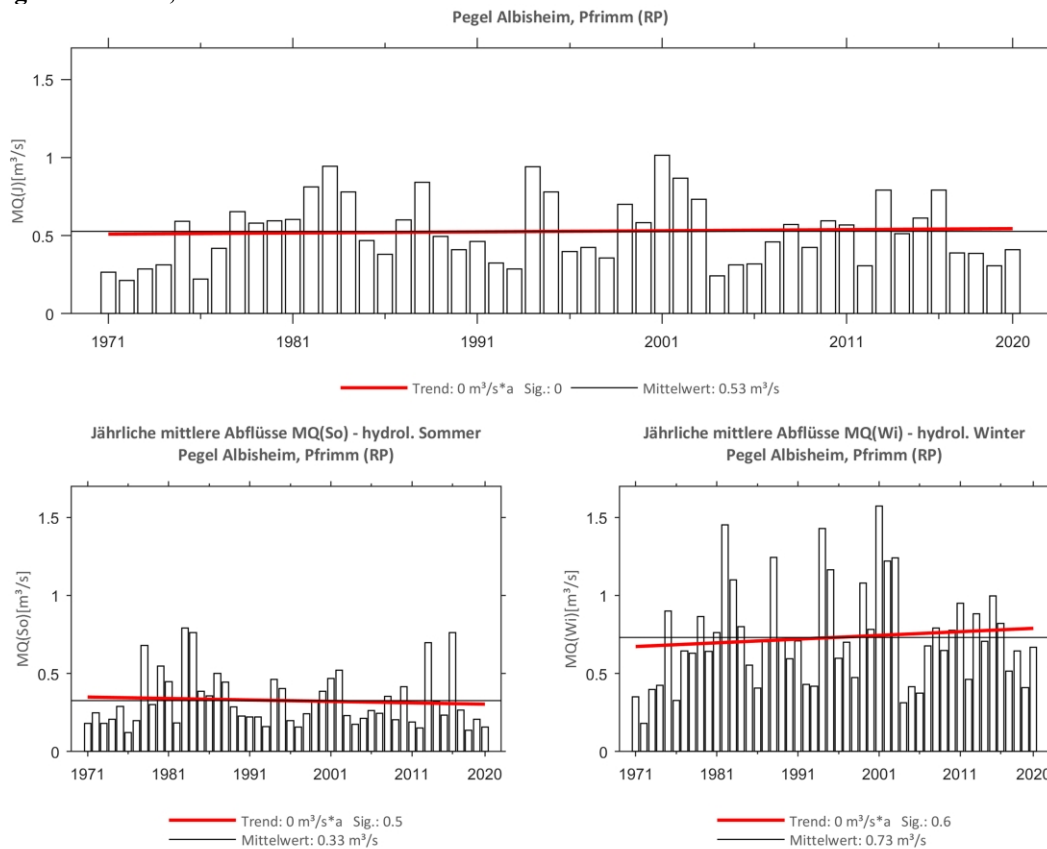
Abb. 228: Trenduntersuchungen von jährlichen mittleren Abflüssen für den Zeitraum 1971 bis 2020.
