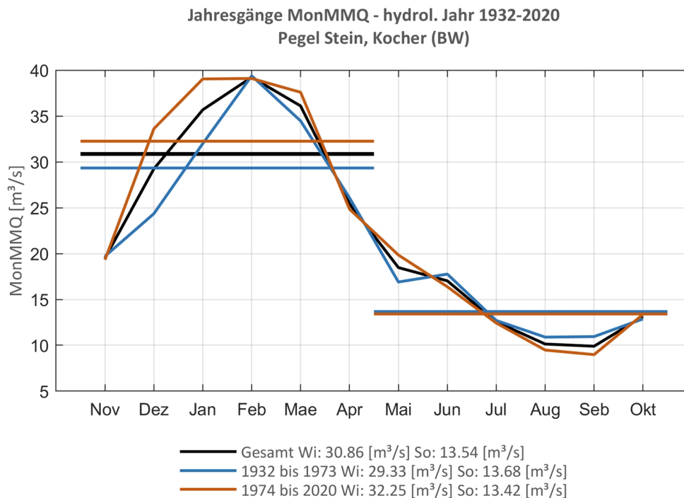
Abb. 45: Jahresgang des MonMMQ und Halbjahresmittel für 1932-2020 sowie 1932-1973 und 1974-2020.
