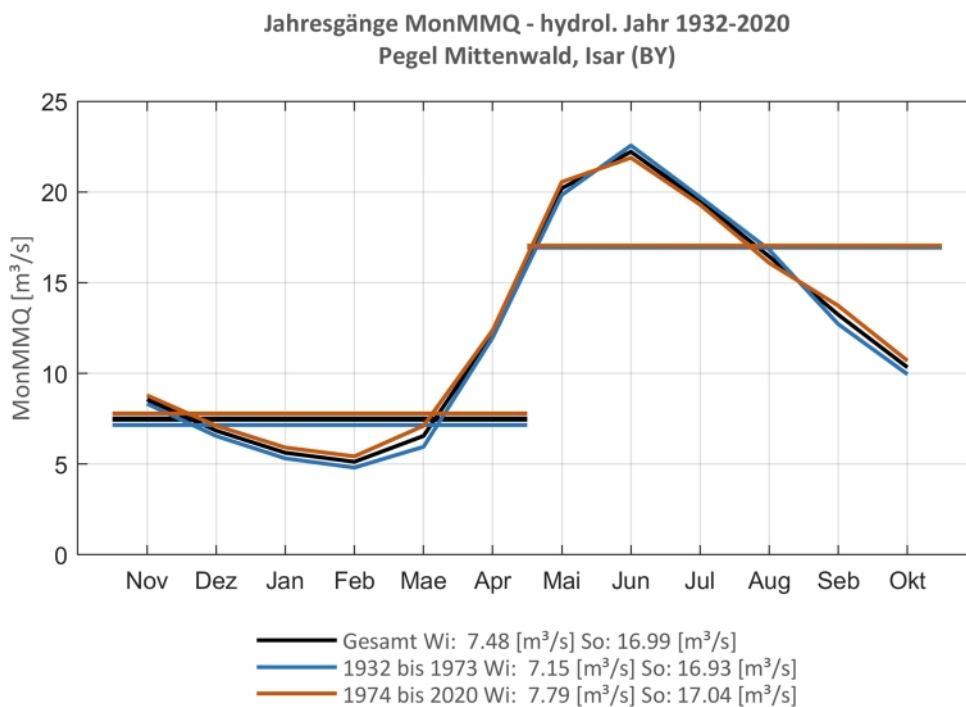
Abb. 119: Jahresgang des MonMMQ und Halbjahresmittel für 1932-2020 sowie 1932-1973 und 1974-2020
