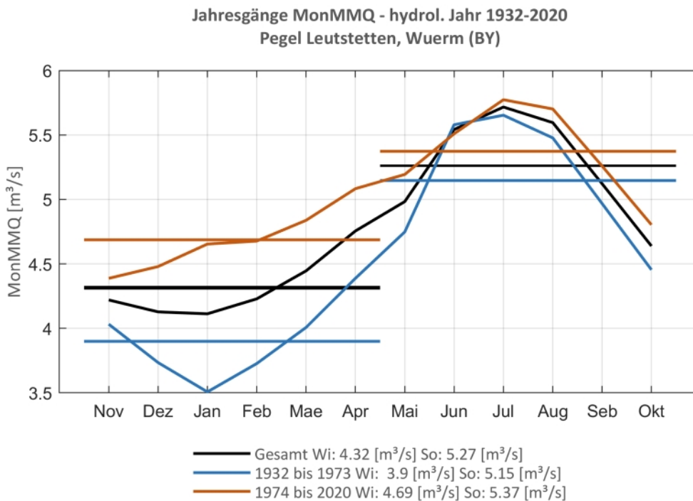
Abb. 117: Jahresgang des MonMMQ und Halbjahresmittel für 1932-2020 sowie 1932-1973 und 1974-2020
