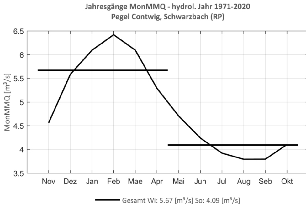
Abb. 242: Jahresgang des MonMMQ und Halbjahresmittel für 1971-2020.
