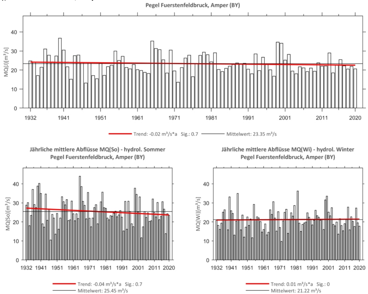
Abb. 108: Trenduntersuchungen von jährlichen mittleren Abflüssen für den Zeitraum 1932 bis 2020.
