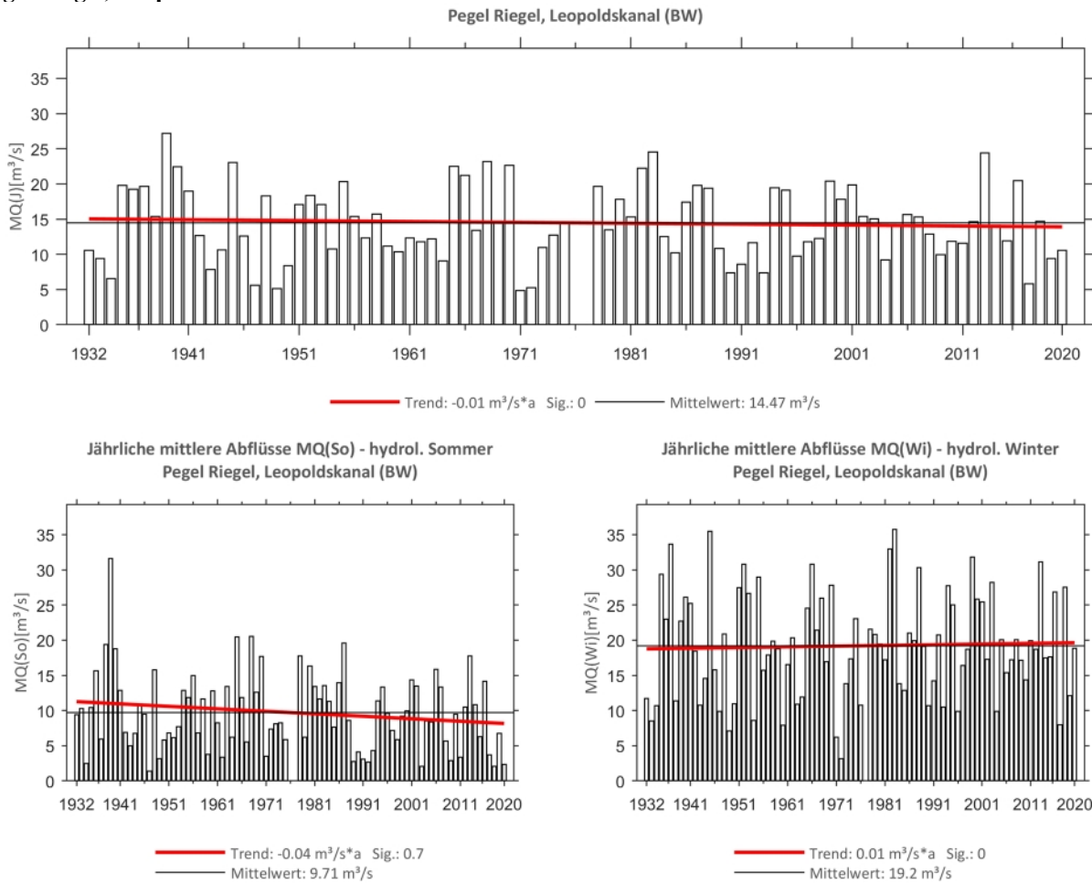
Abb. 14: Trenduntersuchungen von jährlichen mittleren Abflüssen für den Zeitraum 1932 bis 2020.
