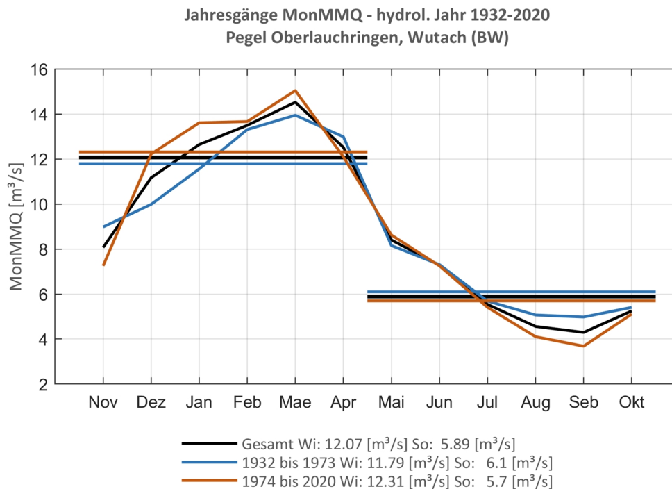
Abb. 13: Jahresgang des MonMMQ und Halbjahresmittel für 1932-2020 sowie 1932-1973 und 1974-2020.
