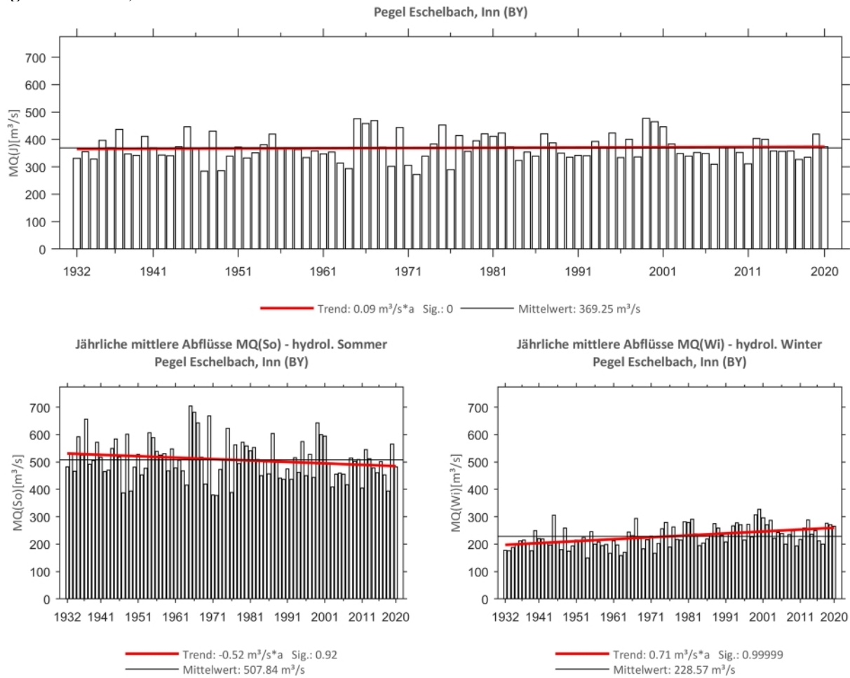
Abb. 106: Trenduntersuchungen von jährlichen mittleren Abflüssen für den Zeitraum 1932 bis 2020.
