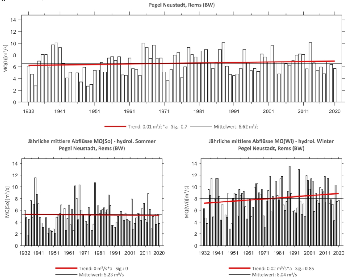
Abb. 34: Trenduntersuchungen von jährlichen mittleren Abflüssen für den Zeitraum 1932 bis 2020.
