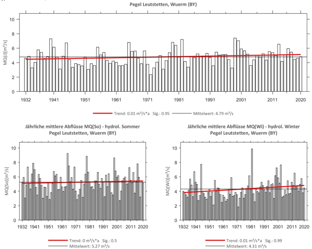
Abb. 116: Trenduntersuchungen von jährlichen mittleren Abflüssen für den Zeitraum 1932 bis 2020.
