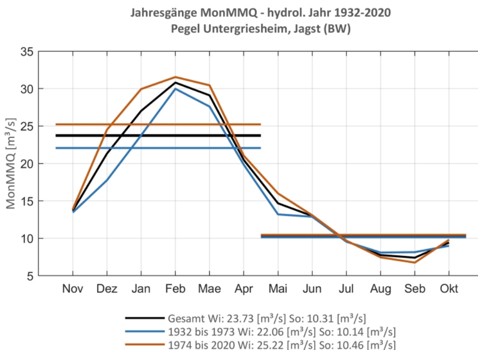
Abb. 47: Jahresgang des MonMMQ und Halbjahresmittel für 1932-2020 sowie 1932-1973 und 1974-2020.
