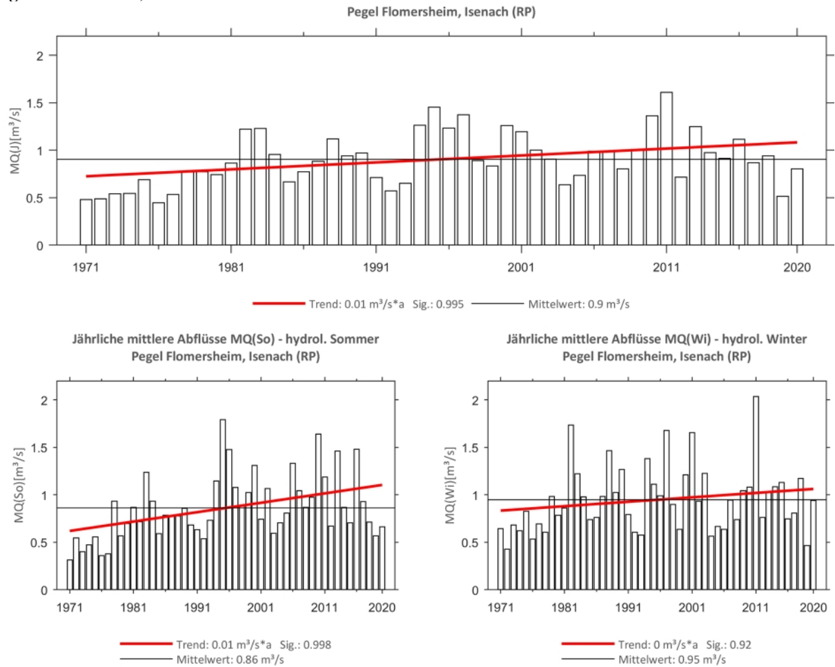
Abb. 244: Trenduntersuchungen von jährlichen mittleren Abflüssen für den Zeitraum 1971 bis 2020.
