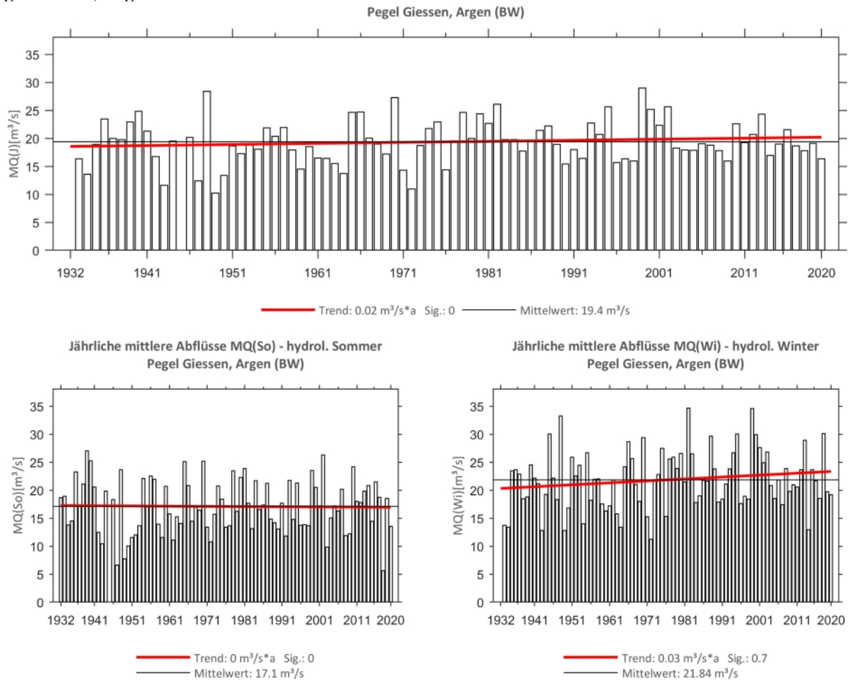
Abb. 8: Trenduntersuchungen von jährlichen mittleren Abflüssen für den Zeitraum 1933 bis 2020.
