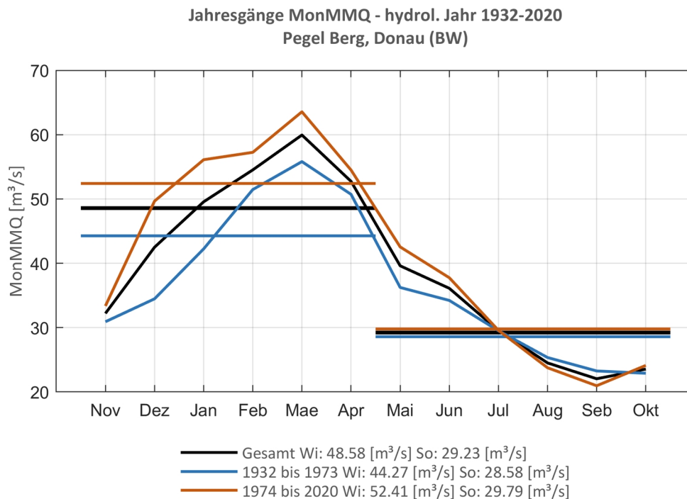
Abb. 49: Jahresgang des MonMMQ und Halbjahresmittel für 1932-2020 sowie 1932-1973 und 1974-2020.
