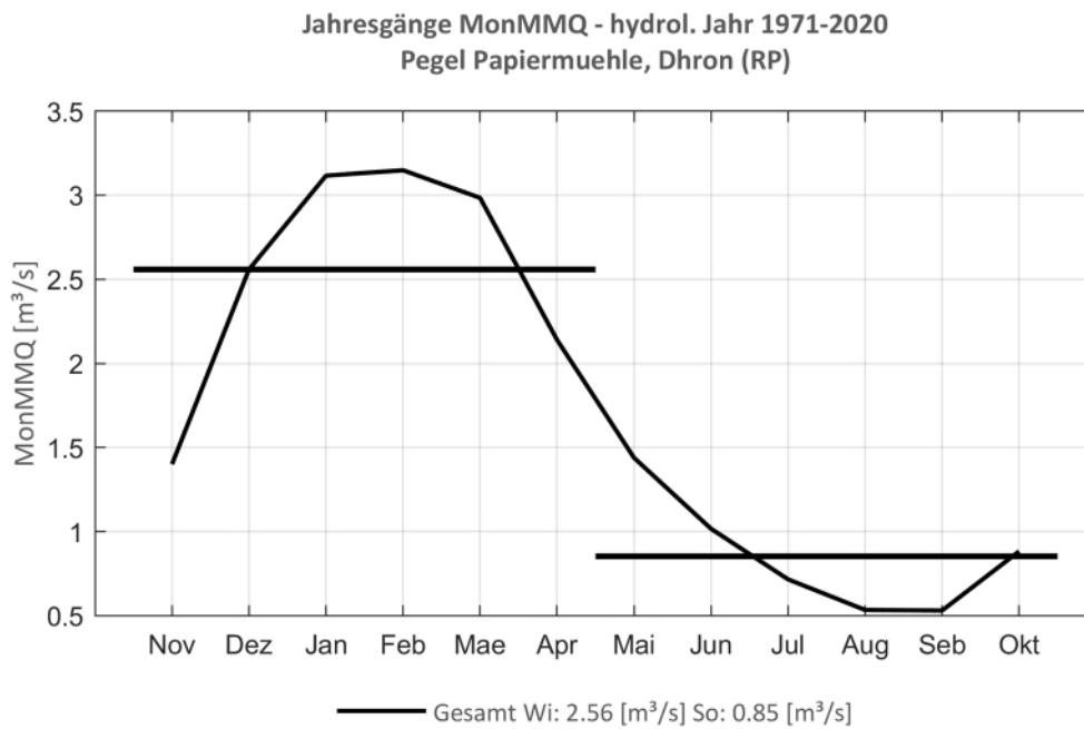
Abb. 220: Jahresgang des MonMMQ und Halbjahresmittel für 1971-2020.
