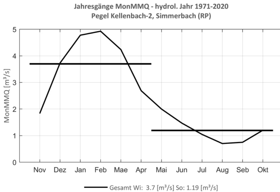
Abb. 252: Jahresgang des MonMMQ und Halbjahresmittel für 1971-2020.
