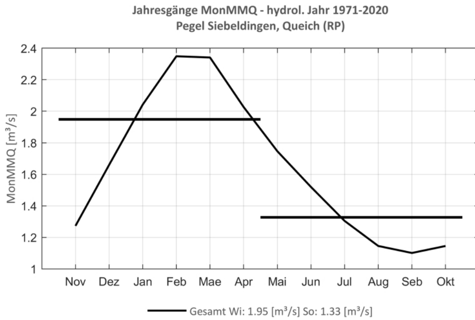
Abb. 270: Jahresgang des MonMMQ und Halbjahresmittel für 1971-2020.
