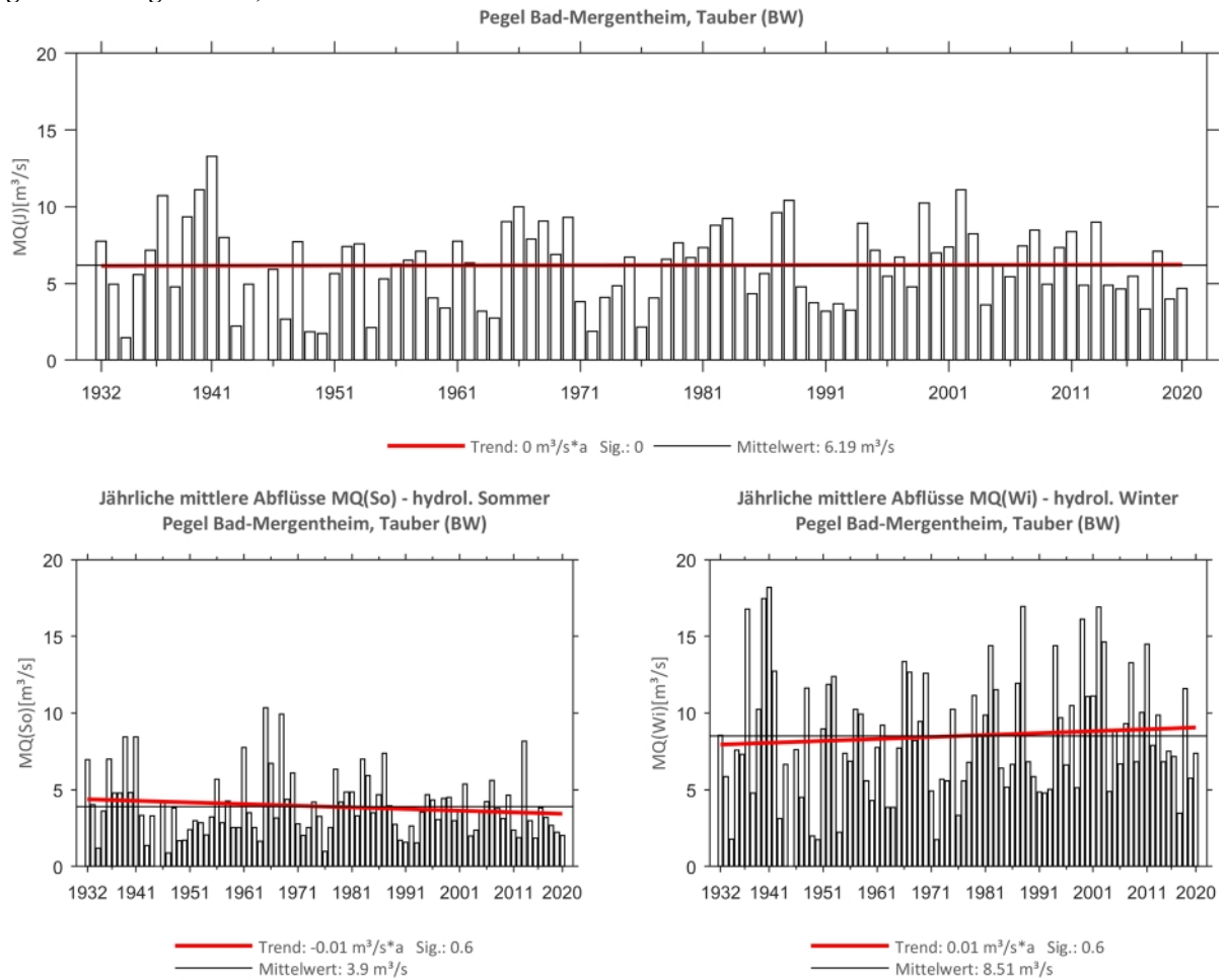
Abb. 60: Trenduntersuchungen von jährlichen mittleren Abflüssen für den Zeitraum 1932 bis 2020.
