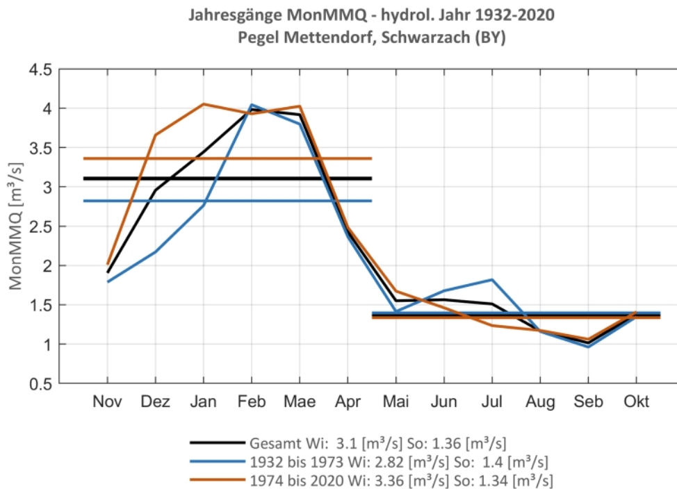
Abb. 149: Jahresgang des MonMMQ und Halbjahresmittel für 1932-2020 sowie 1932-1973 und 1974-2020
