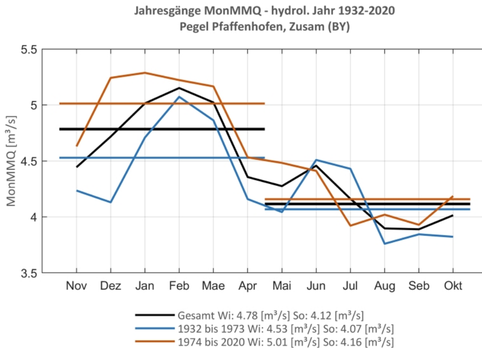
Abb. 89: Jahresgang des MonMMQ und Halbjahresmittel für 1932-2020 sowie 1932-1973 und 1974-2020
