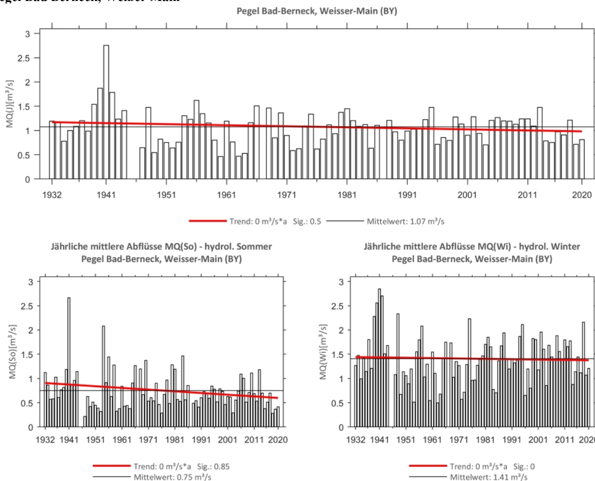
Abb. 154: Trenduntersuchungen von jährlichen mittleren Abflüssen für den Zeitraum 1932 bis 2020.
