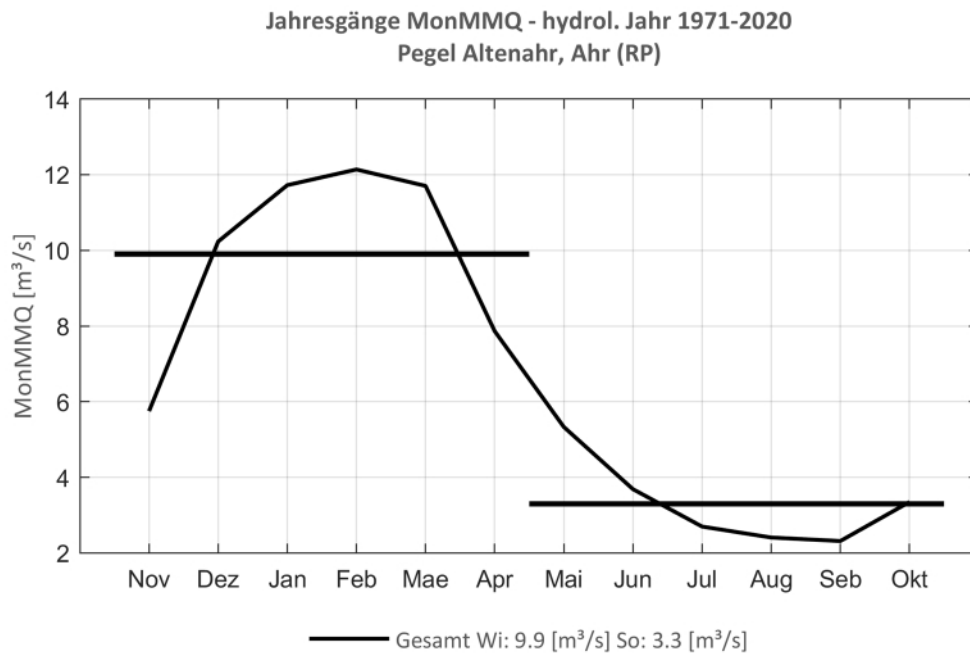
Abb. 194: Jahresgang des MonMMQ und Halbjahresmittel für 1971-2020.
