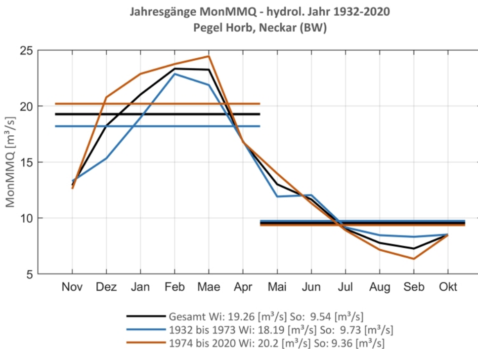
Abb. 27: Jahresgang des MonMMQ und Halbjahresmittel für 1932-2020 sowie 1932-1973 und 1974-2020.
