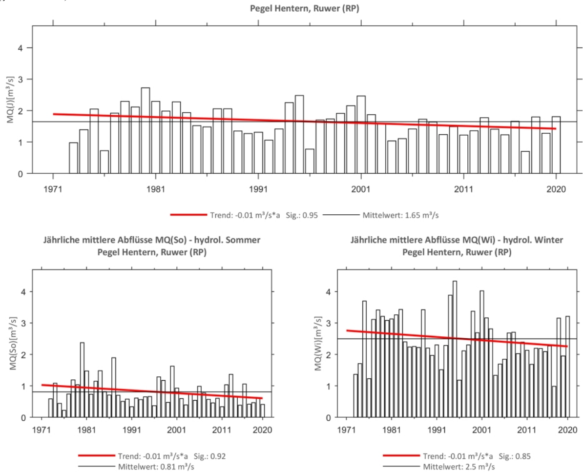
Abb. 208: Trenduntersuchungen von jährlichen mittleren Abflüssen für den Zeitraum 1973 bis 2020.
