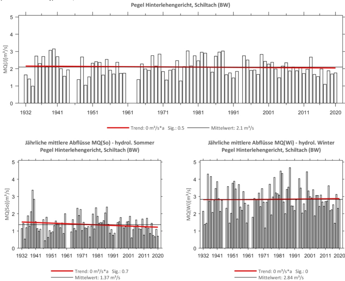
Abb. 10: Trenduntersuchungen von jährlichen mittleren Abflüssen für den Zeitraum 1932 bis 2020.
