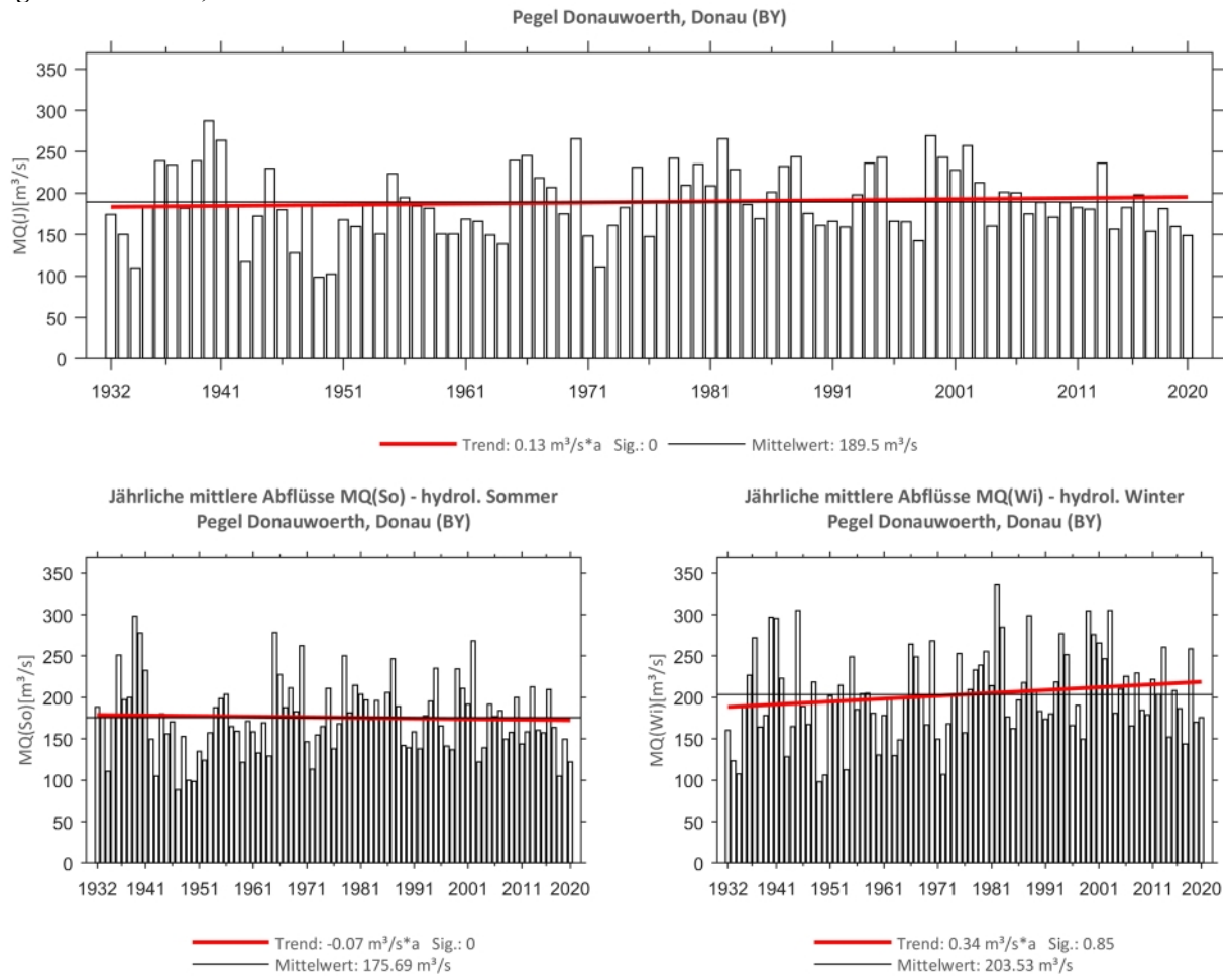
Abb. 80: Trenduntersuchungen von jährlichen mittleren Abflüssen für den Zeitraum 1932 bis 2020.
