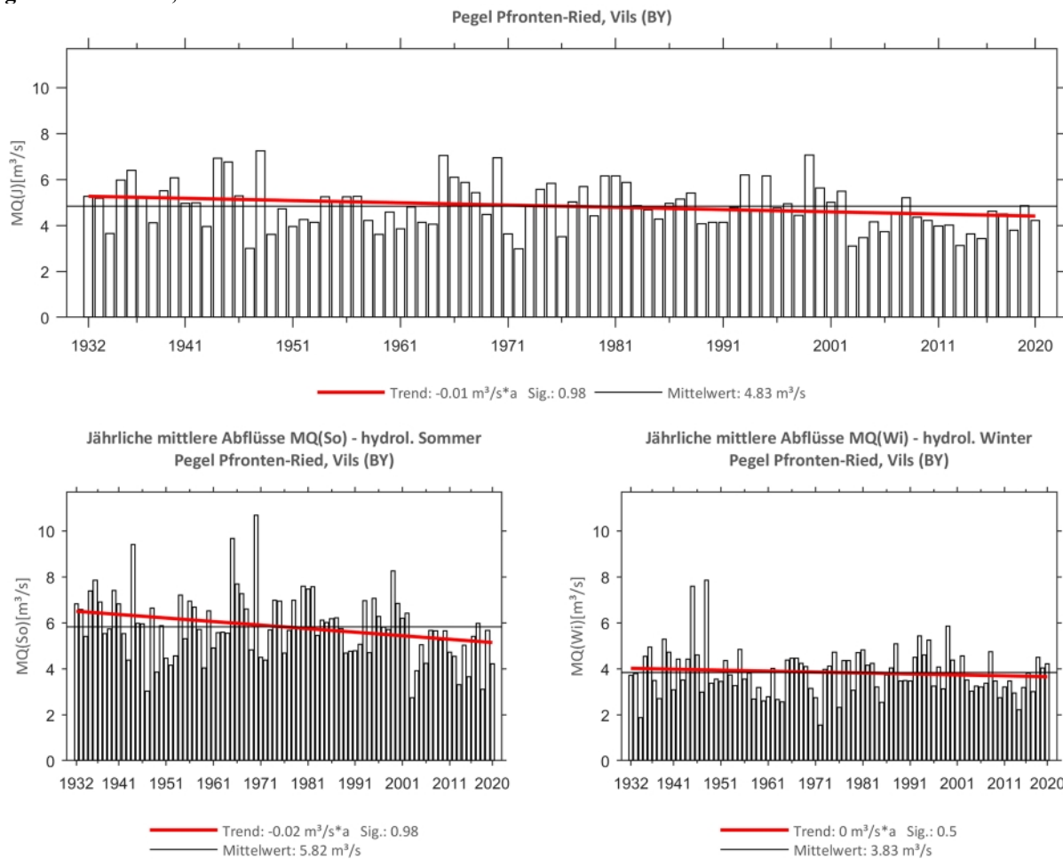
Abb. 90: Trenduntersuchungen von jährlichen mittleren Abflüssen für den Zeitraum 1932 bis 2020.
