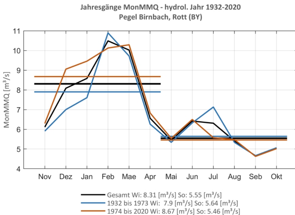
Abb. 103: Jahresgang des MonMMQ und Halbjahresmittel für 1932-2020 sowie 1932-1973 und 1974-2020
