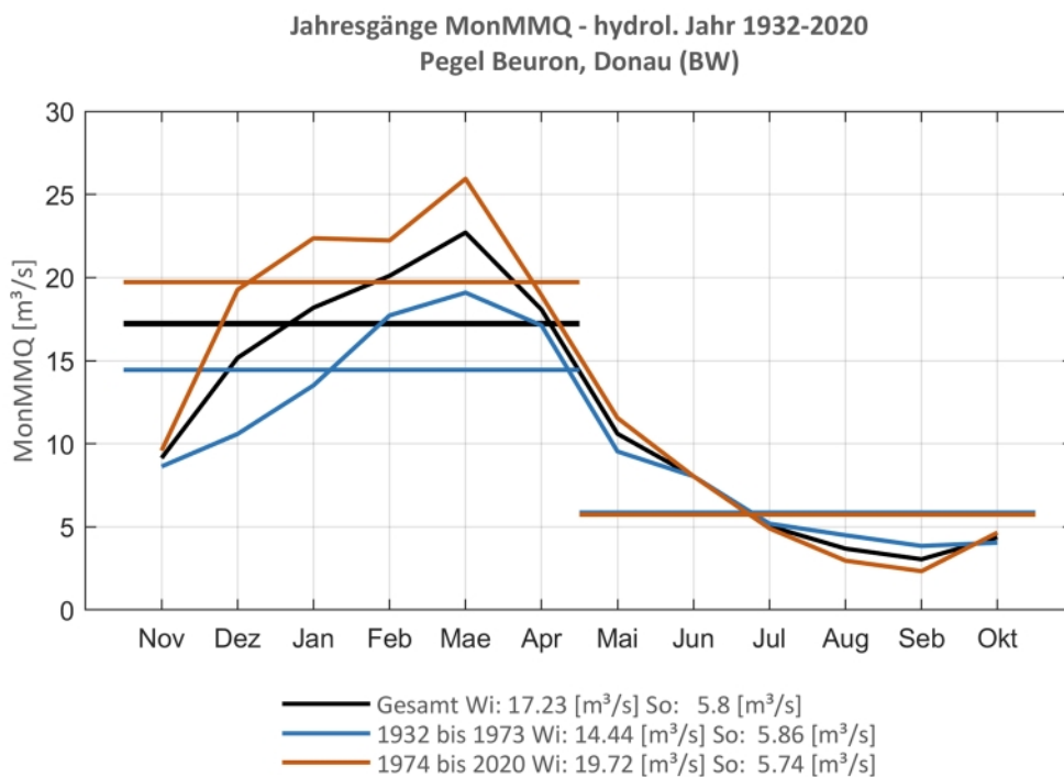
Abb. 51: Jahresgang des MonMMQ und Halbjahresmittel für 1932-2020 sowie 1932-1973 und 1974-2020.
