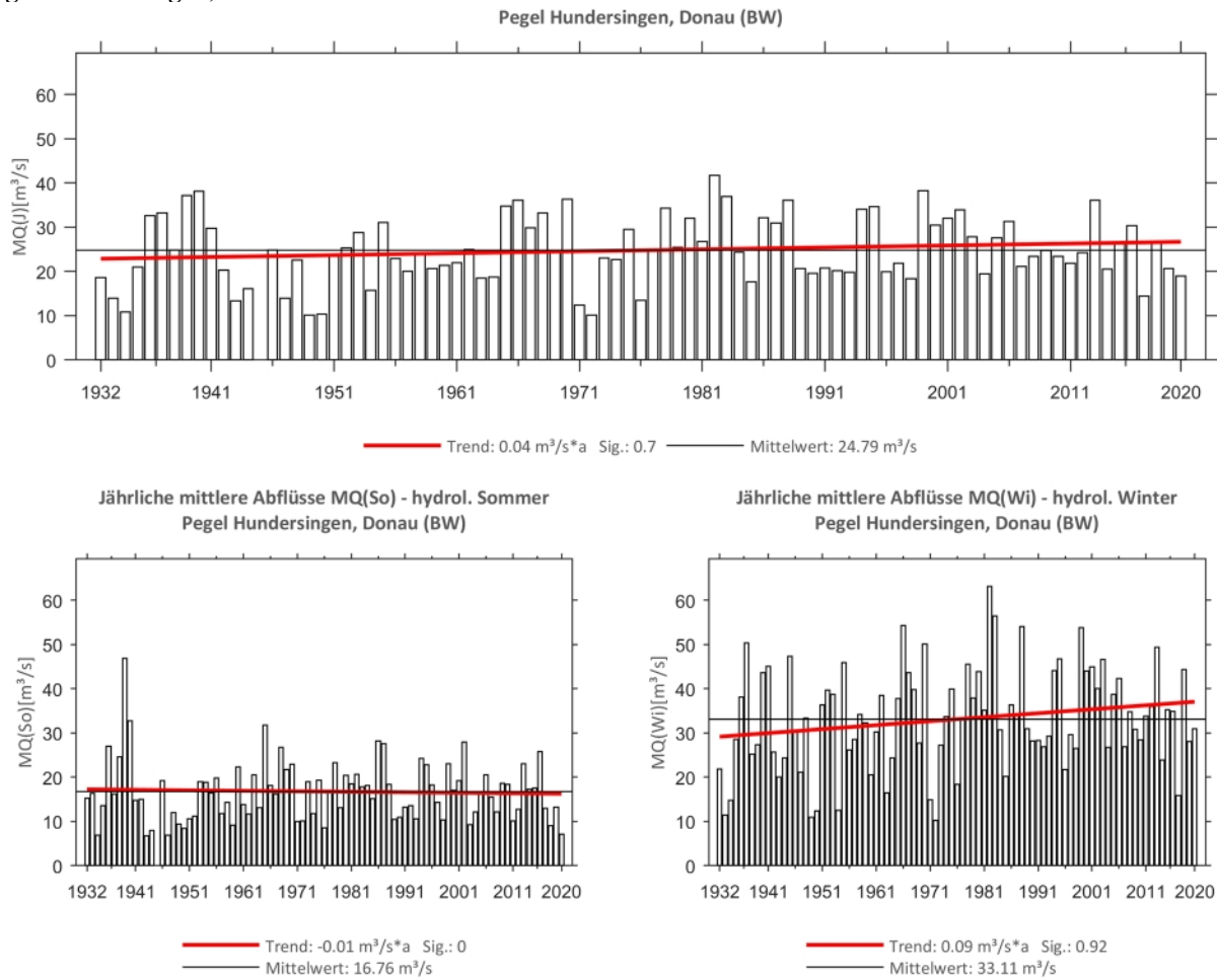
Abb. 54: Trenduntersuchungen von jährlichen mittleren Abflüssen für den Zeitraum 1932 bis 2020.
