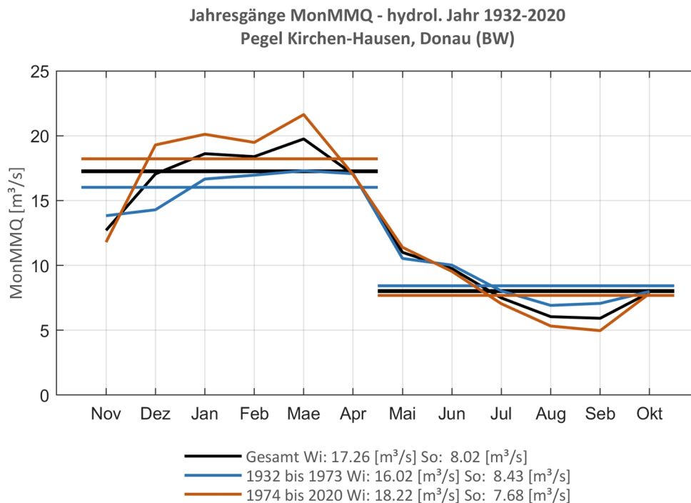
Abb. 57: Jahresgang des MonMMQ und Halbjahresmittel für 1932-2020 sowie 1932-1973 und 1974-2020.
