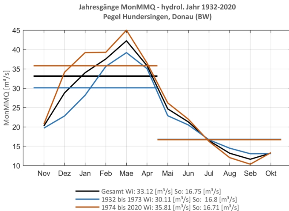
Abb. 55: Jahresgang des MonMMQ und Halbjahresmittel für 1932-2020 sowie 1932-1973 und 1974-2020.
