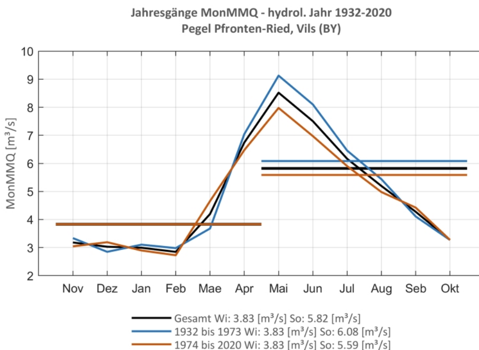
Abb. 91: Jahresgang des MonMMQ und Halbjahresmittel für 1932-2020 sowie 1932-1973 und 1974-2020
