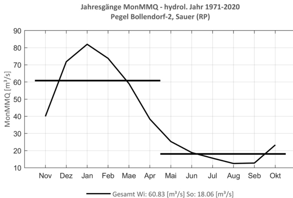
Abb. 202: Jahresgang des MonMMQ und Halbjahresmittel für 1971-2020.
