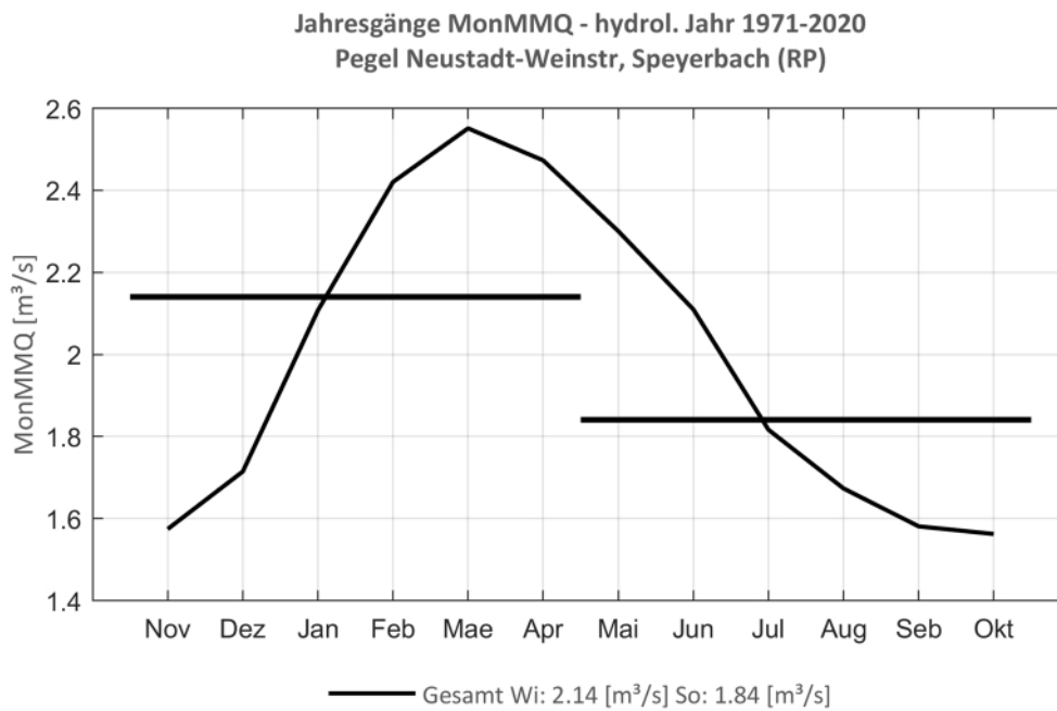
Abb. 260: Jahresgang des MonMMQ und Halbjahresmittel für 1971-2020.
