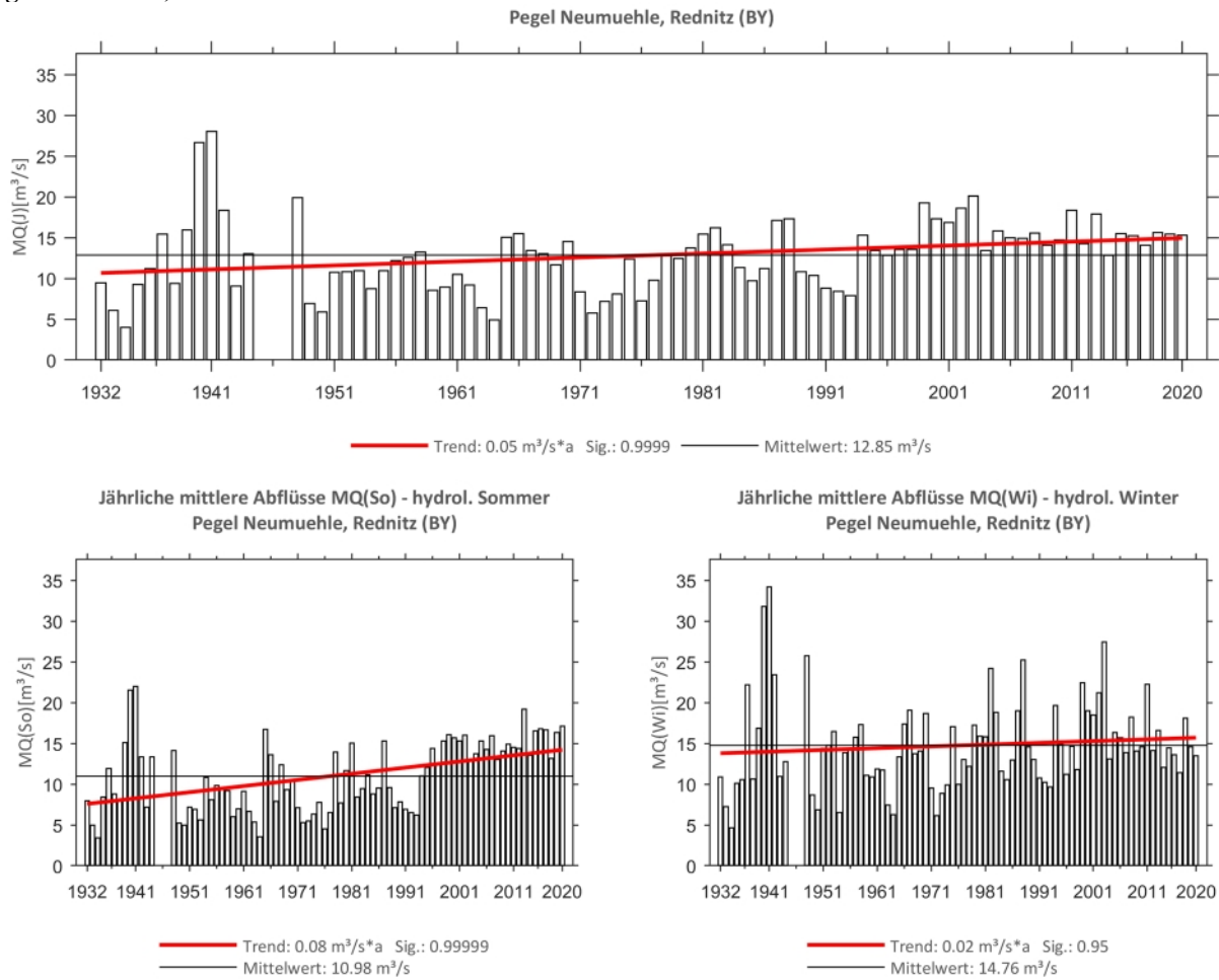
Abb. 166: Trenduntersuchungen von jährlichen mittleren Abflüssen für den Zeitraum 1932 bis 2020.
