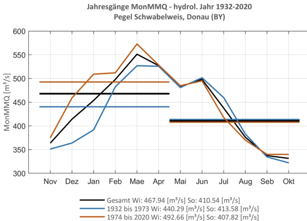
Abb. 153: Jahresgang des MonMMQ und Halbjahresmittel für 1932-2020 sowie 1932-1973 und 1974-2020
