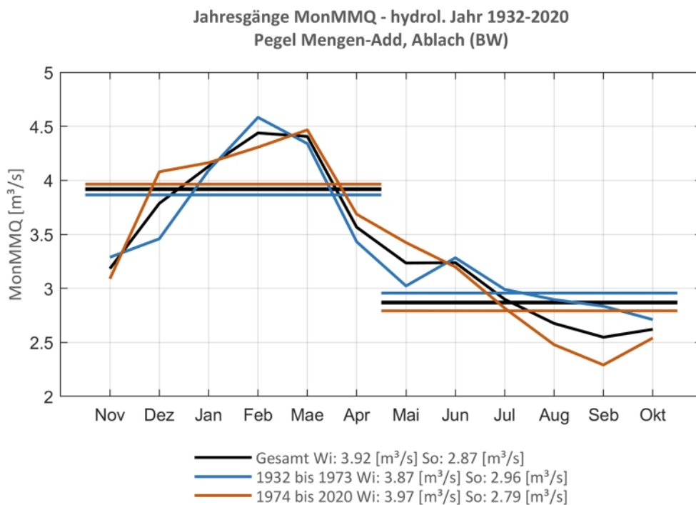
Abb. 59: Jahresgang des MonMMQ und Halbjahresmittel für 1932-2020 sowie 1932-1973 und 1974-2020.
