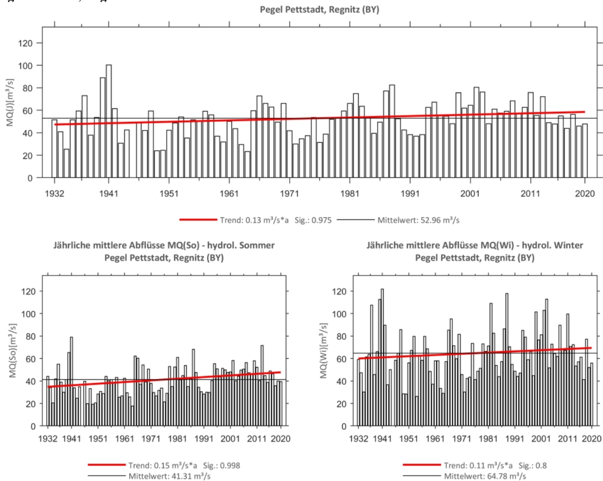
Abb. 170: Trenduntersuchungen von jährlichen mittleren Abflüssen für den Zeitraum 1932 bis 2020.
