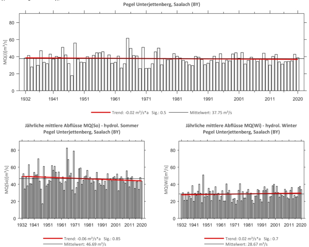
Abb. 136: Trenduntersuchungen von jährlichen mittleren Abflüssen für den Zeitraum 1932 bis 2020.
