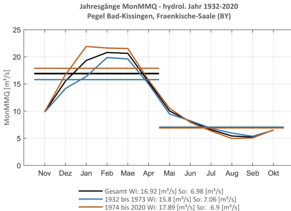
Abb. 177: Jahresgang des MonMMQ und Halbjahresmittel für 1932-2020 sowie 1932-1973 und 1974-2020
