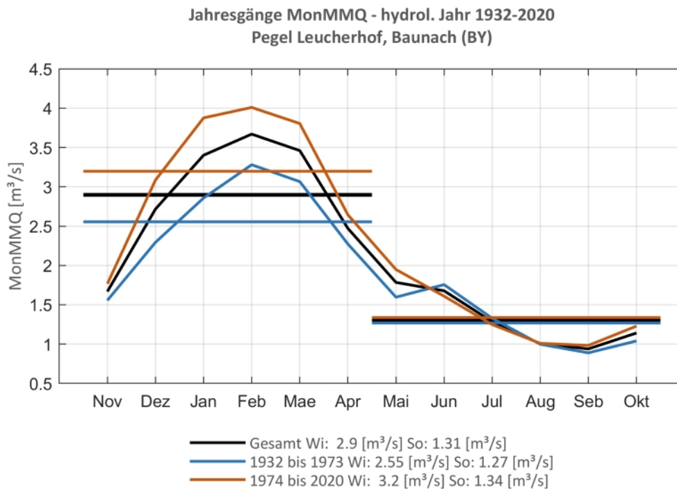
Abb. 165: Jahresgang des MonMMQ und Halbjahresmittel für 1932-2020 sowie 1932-1973 und 1974-2020
