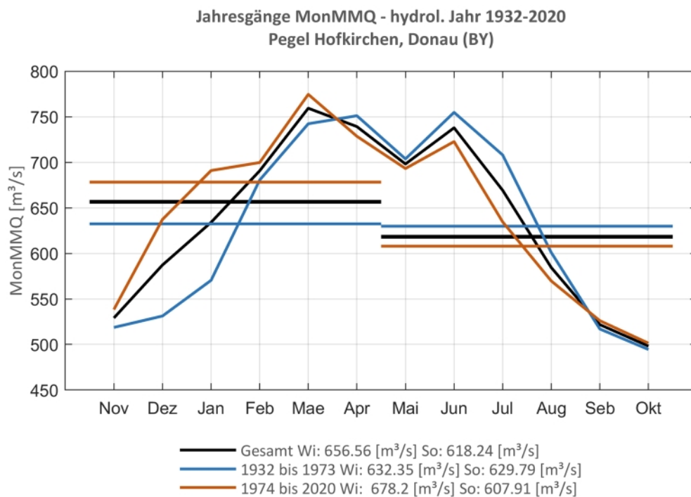
Abb. 71: Jahresgang des MonMMQ und Halbjahresmittel für 1932-2020 sowie 1932-1973 und 1974-2020
