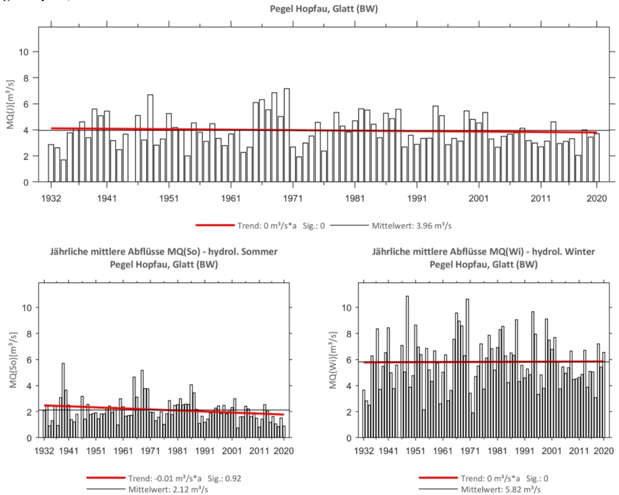
Abb. 24: Trenduntersuchungen von jährlichen mittleren Abflüssen für den Zeitraum 1932 bis 2020.
