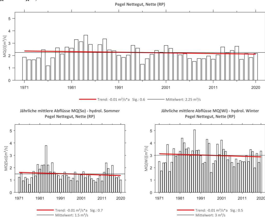
Abb. 214: Trenduntersuchungen von jährlichen mittleren Abflüssen für den Zeitraum 1971 bis 2020.
