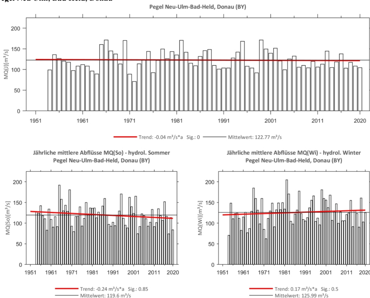
Abb. 86: Trenduntersuchungen von jährlichen mittleren Abflüssen für den Zeitraum 1954 bis 2020.
