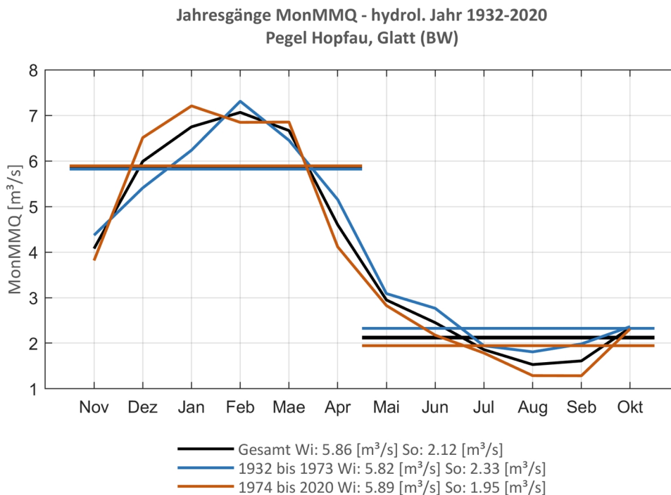
Abb. 25: Jahresgang des MonMMQ und Halbjahresmittel für 1932-2020 sowie 1932-1973 und 1974-2020.
