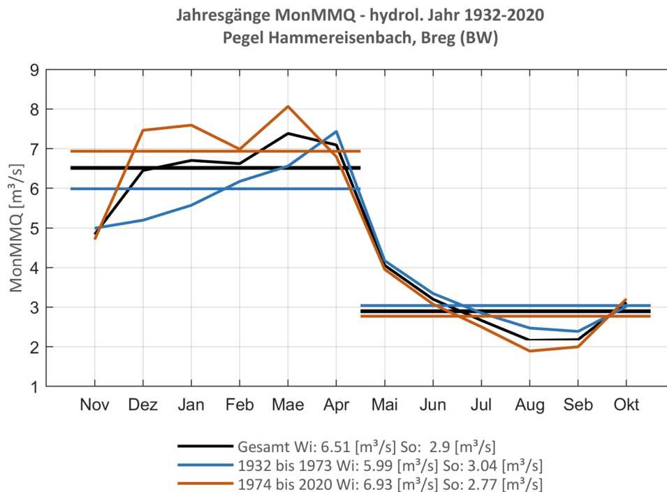
Abb. 53: Jahresgang des MonMMQ und Halbjahresmittel für 1932-2020 sowie 1932-1973 und 1974-2020.
