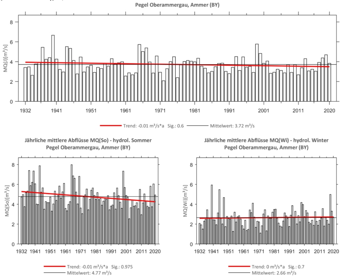
Abb. 120: Trenduntersuchungen von jährlichen mittleren Abflüssen für den Zeitraum 1932 bis 2020.
