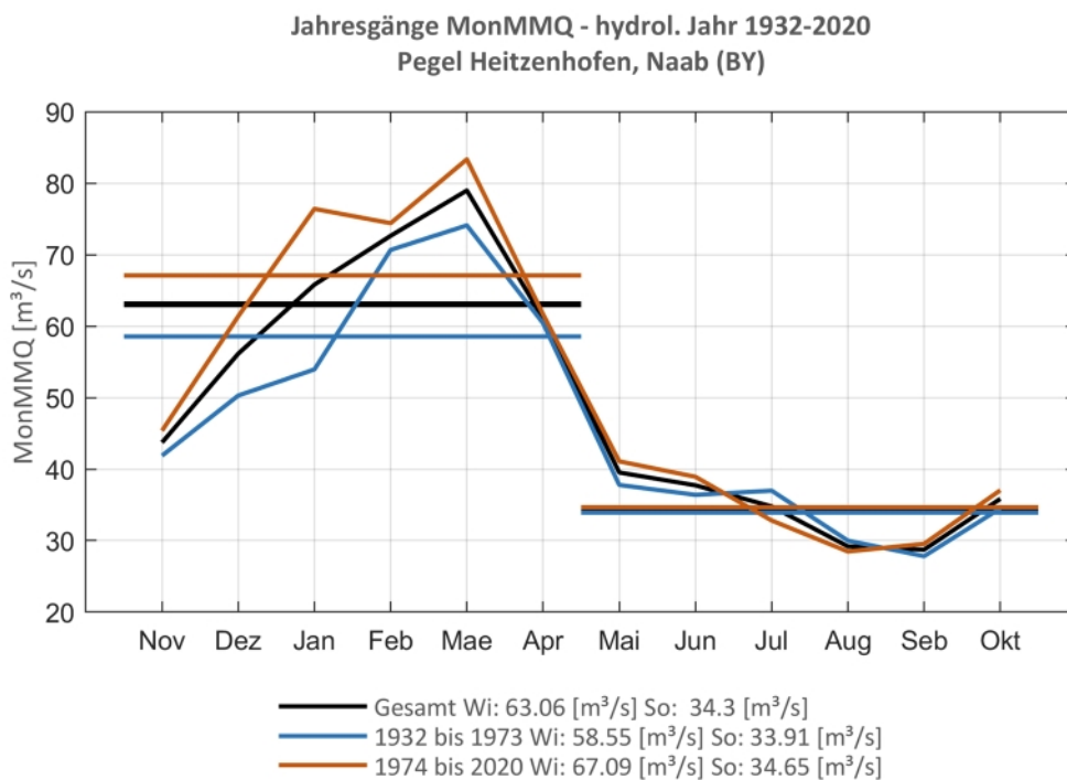
Abb. 67: Jahresgang des MonMMQ und Halbjahresmittel für 1932-2020 sowie 1932-1973 und 1974-2020
