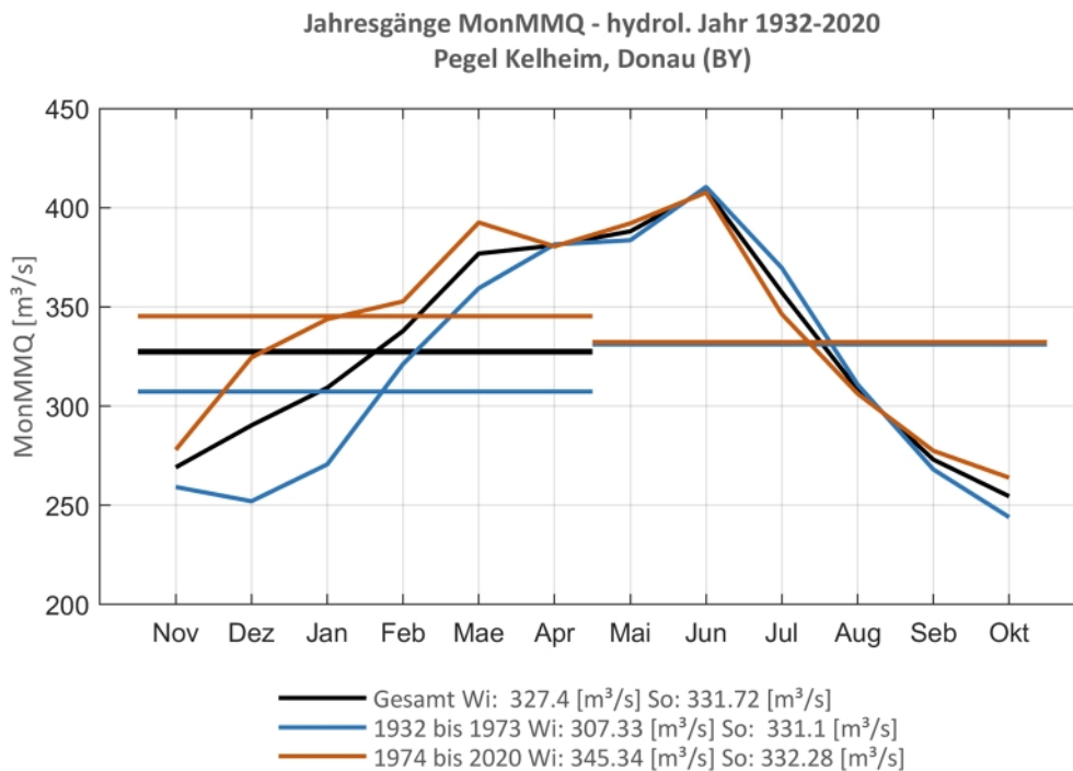
Abb. 145: Jahresgang des MonMMQ und Halbjahresmittel für 1932-2020 sowie 1932-1973 und 1974-2020
