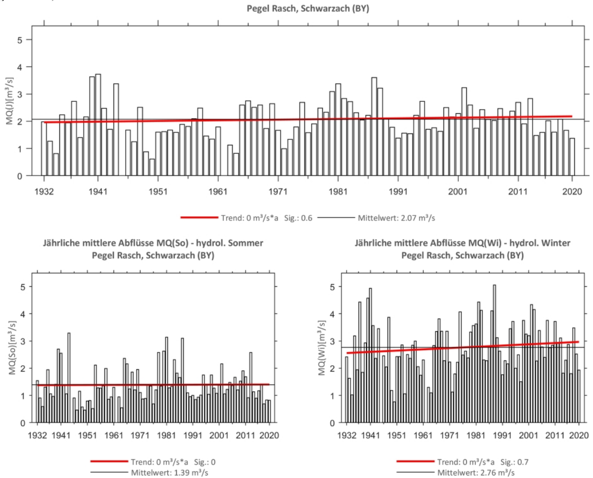
Abb. 172: Trenduntersuchungen von jährlichen mittleren Abflüssen für den Zeitraum 1932 bis 2020.
