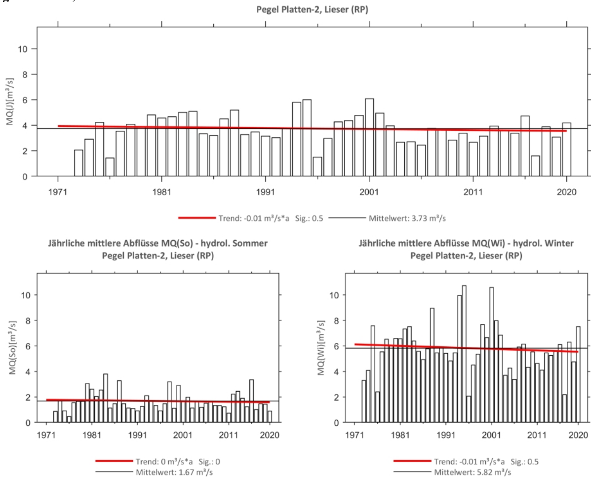
Abb. 222: Trenduntersuchungen von jährlichen mittleren Abflüssen für den Zeitraum 1973 bis 2020.
