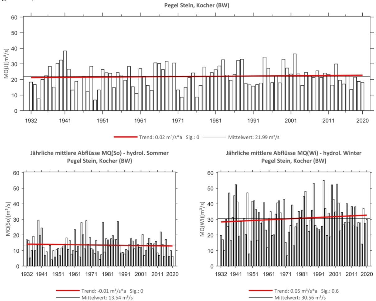
Abb. 44: Trenduntersuchungen von jährlichen mittleren Abflüssen für den Zeitraum 1932 bis 2020.
