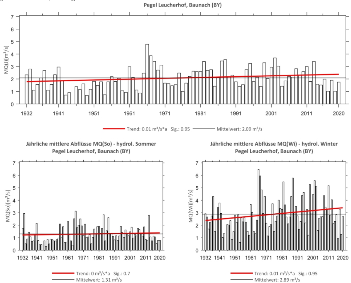
Abb. 164: Trenduntersuchungen von jährlichen mittleren Abflüssen für den Zeitraum 1932 bis 2020.
