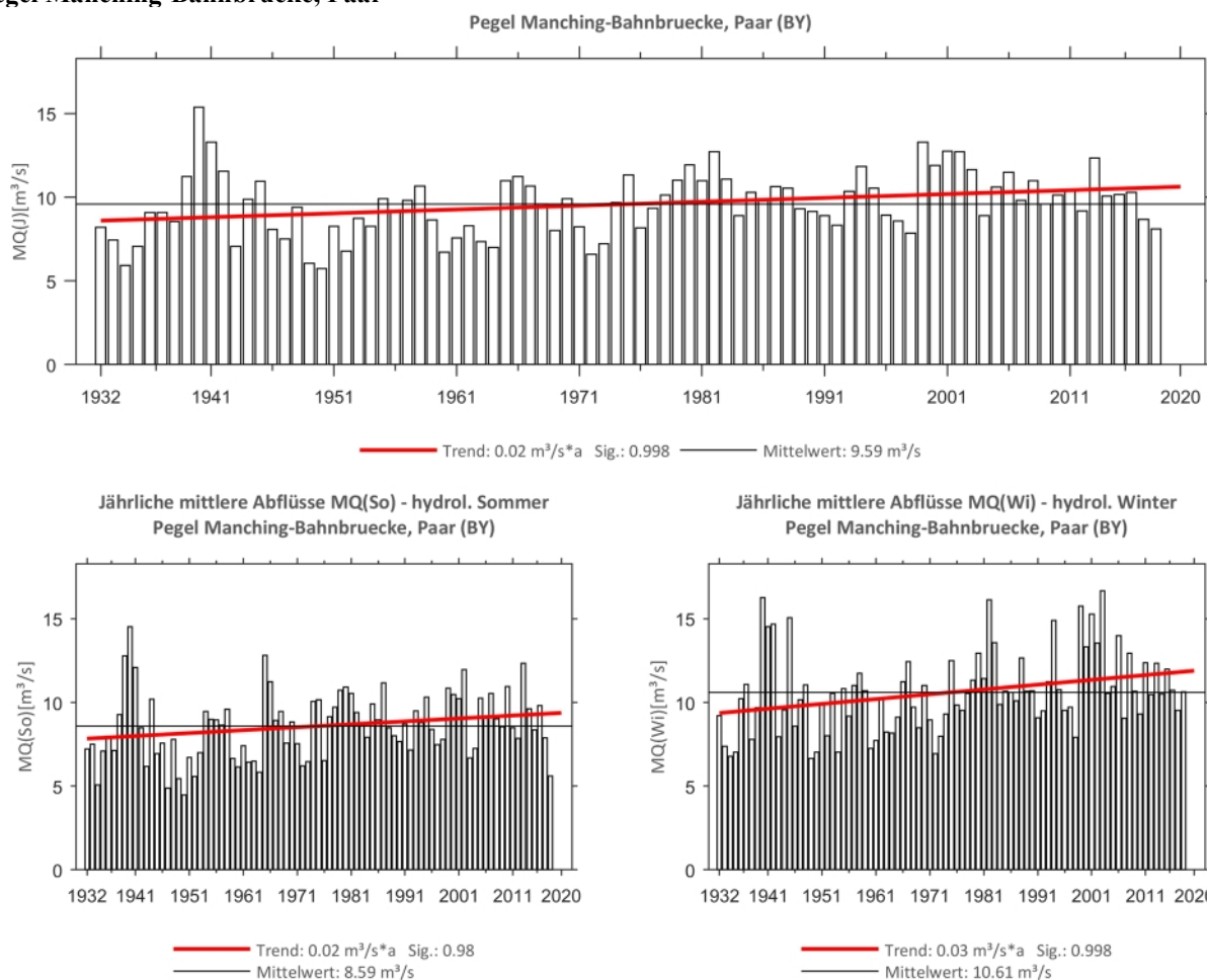
Abb. 146: Trenduntersuchungen von jährlichen mittleren Abflüssen für den Zeitraum 1932 bis 2020.
