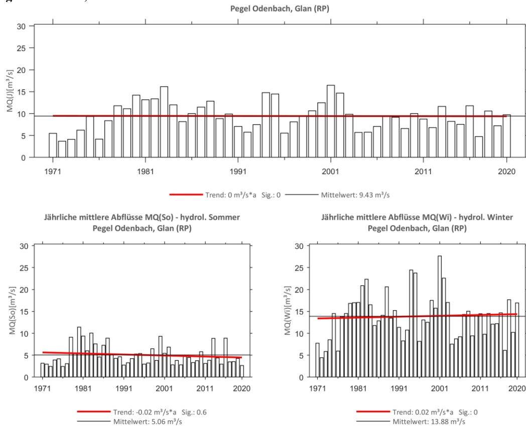
Abb. 264: Trenduntersuchungen von jährlichen mittleren Abflüssen für den Zeitraum 1971 bis 2020. Pegel Odenbach, Glan (RP)
