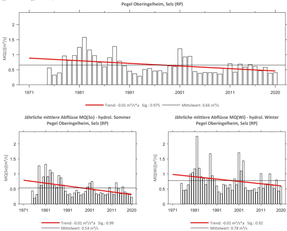
Abb. 262: Trenduntersuchungen von jährlichen mittleren Abflüssen für den Zeitraum 1975 bis 2020.
