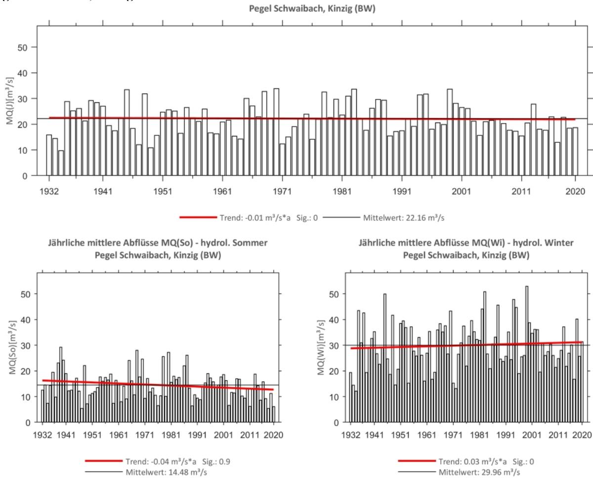
Abb. 18: Trenduntersuchungen von jährlichen mittleren Abflüssen für den Zeitraum 1932 bis 2020.
