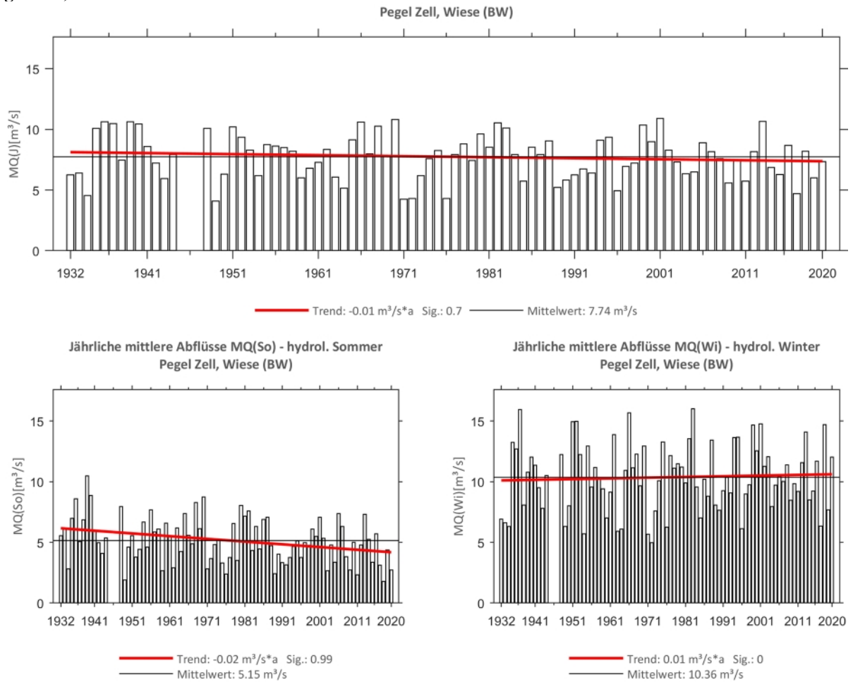
Abb. 20: Trenduntersuchungen von jährlichen mittleren Abflüssen für den Zeitraum 1932 bis 2020.
