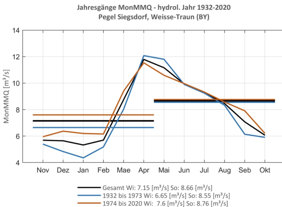
Abb. 131: Jahresgang des MonMMQ und Halbjahresmittel für 1932-2020 sowie 1932-1973 und 1974-2020
