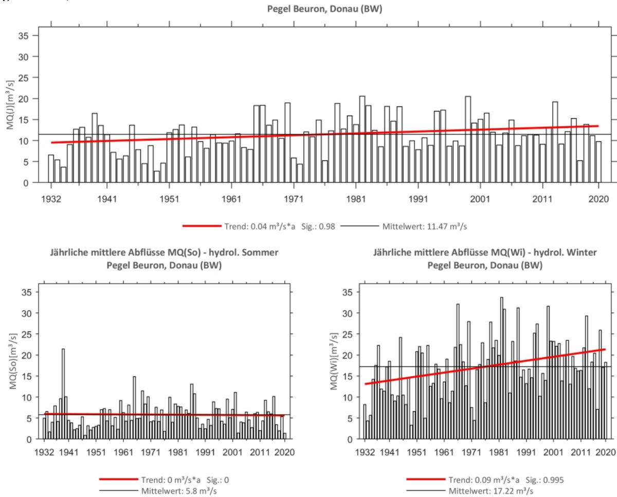
Abb. 50: Trenduntersuchungen von jährlichen mittleren Abflüssen für den Zeitraum 1932 bis 2020.
