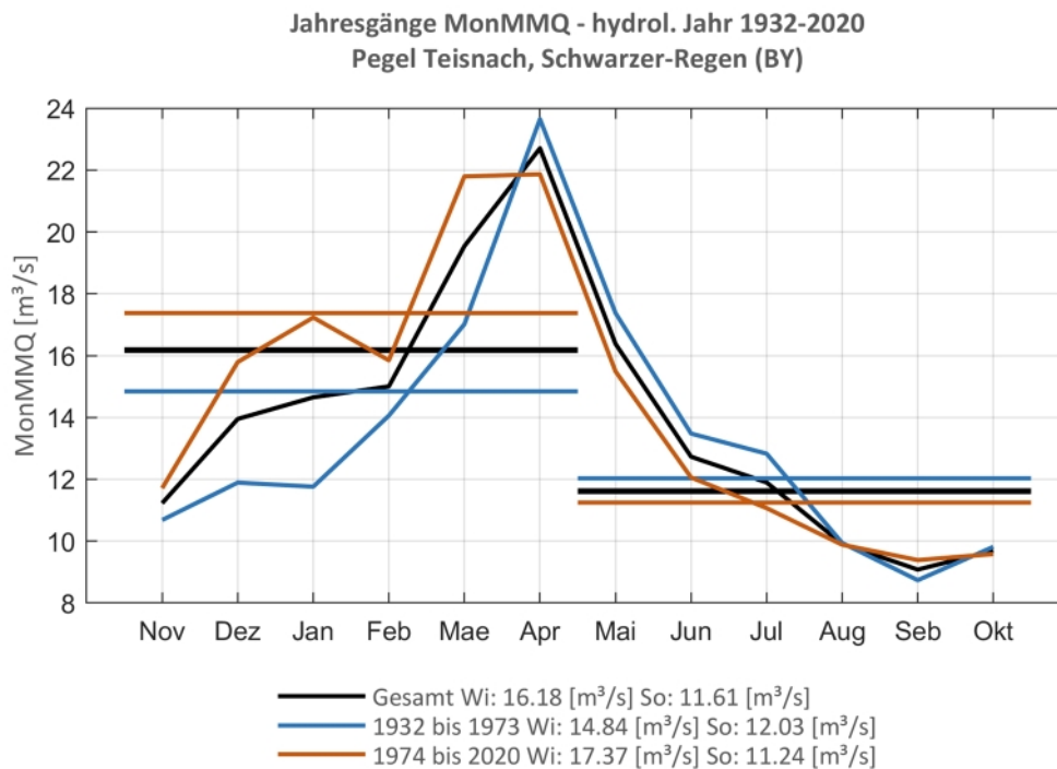
Abb. 77: Jahresgang des MonMMQ und Halbjahresmittel für 1932-2020 sowie 1932-1973 und 1974-2020
