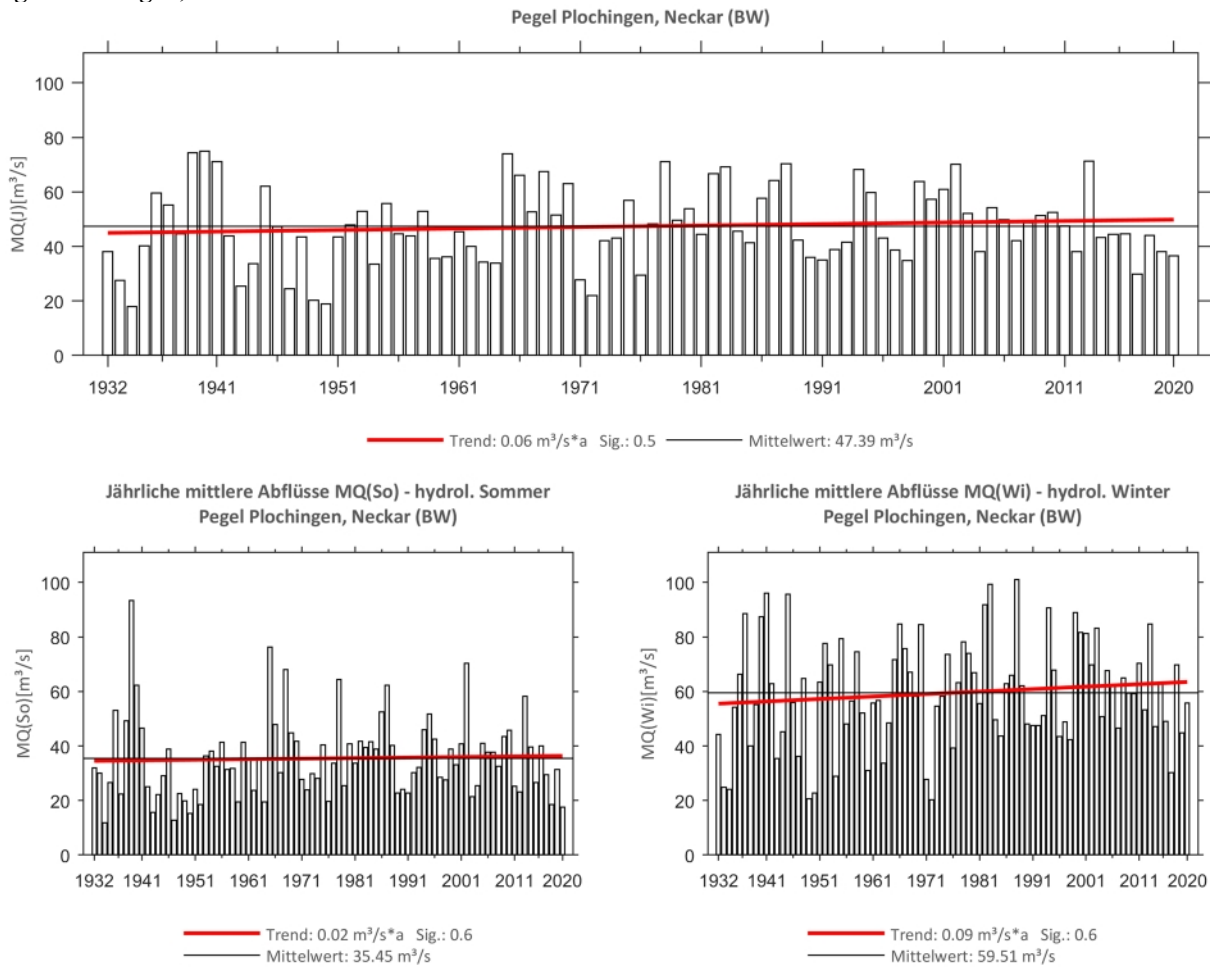
Abb. 40: Trenduntersuchungen von jährlichen mittleren Abflüssen für den Zeitraum 1932 bis 2020.
