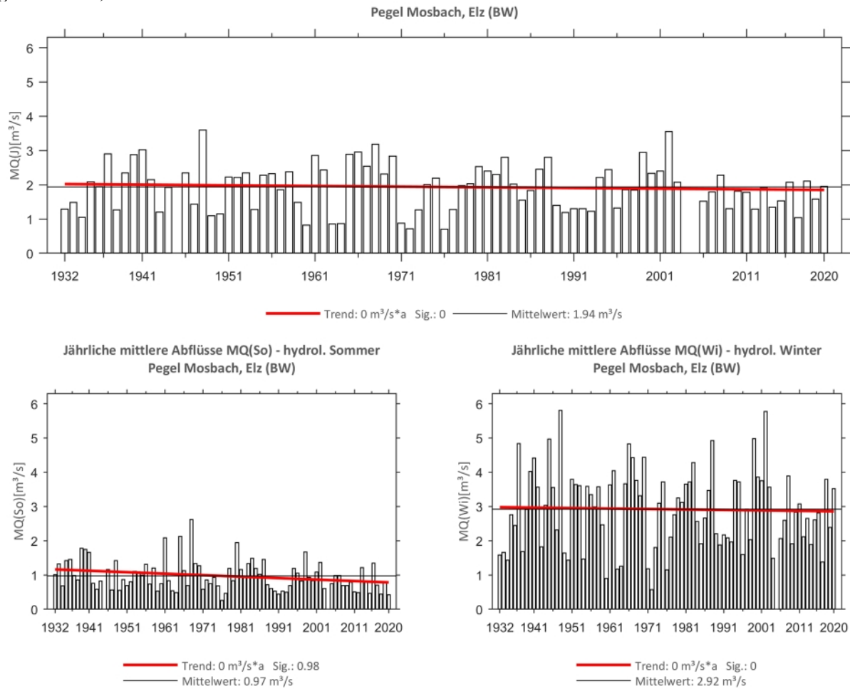
Abb. 32: Trenduntersuchungen von jährlichen mittleren Abflüssen für den Zeitraum 1932 bis 2020.
