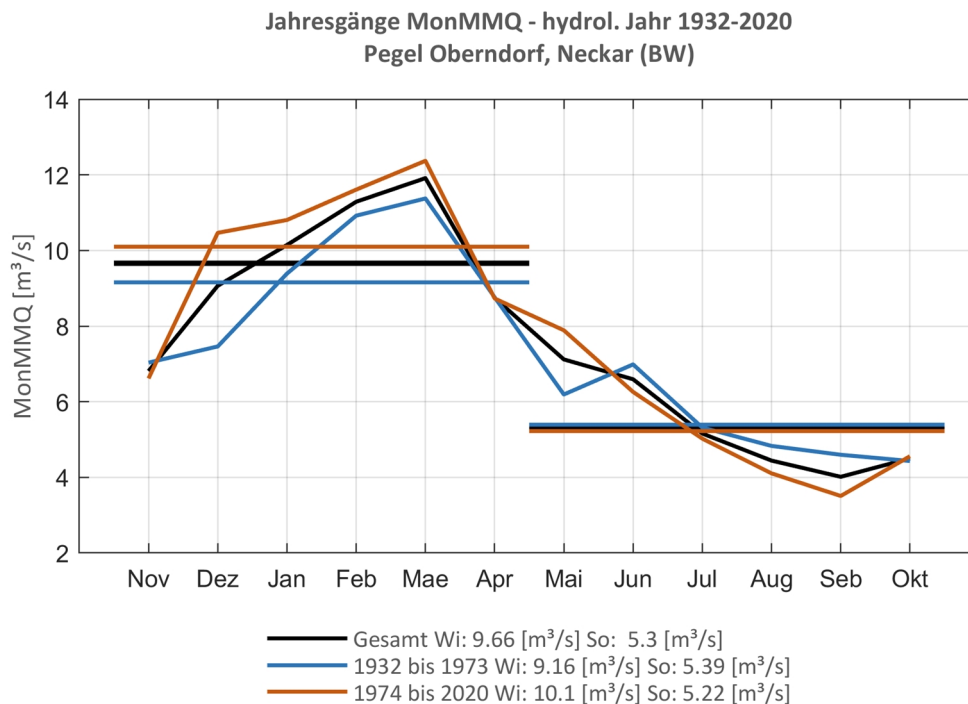
Abb. 37: Jahresgang des MonMMQ und Halbjahresmittel für 1932-2020 sowie 1932-1973 und 1974-2020.
