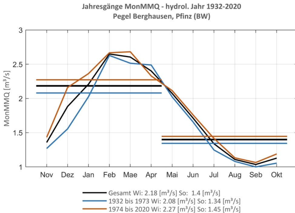
Abb. 5: Jahresgang des MonMMQ und Halbjahresmittel für 1932-2020 sowie 1932-1973 und 1974-2020.
