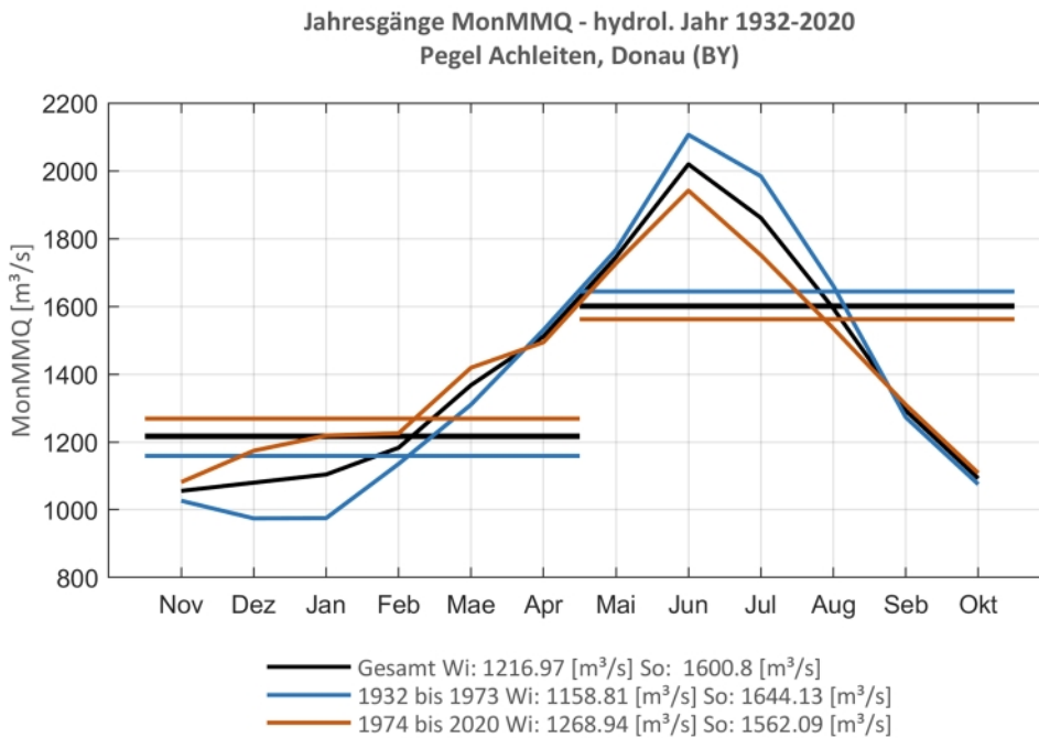
Abb. 63: Jahresgang des MonMMQ und Halbjahresmittel für 1932-2020 sowie 1932-1973 und 1974-2020
