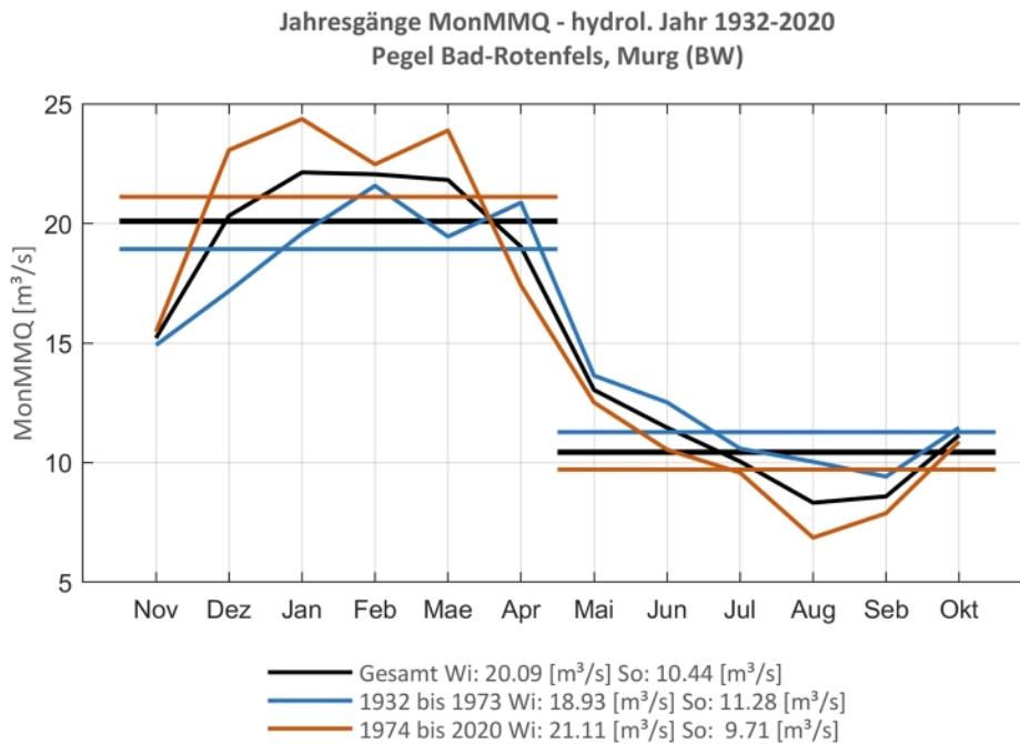
Abb. 3: Jahresgang des MonMMQ und Halbjahresmittel für 1932-2020 sowie 1932-1973 und 1974-2020.
