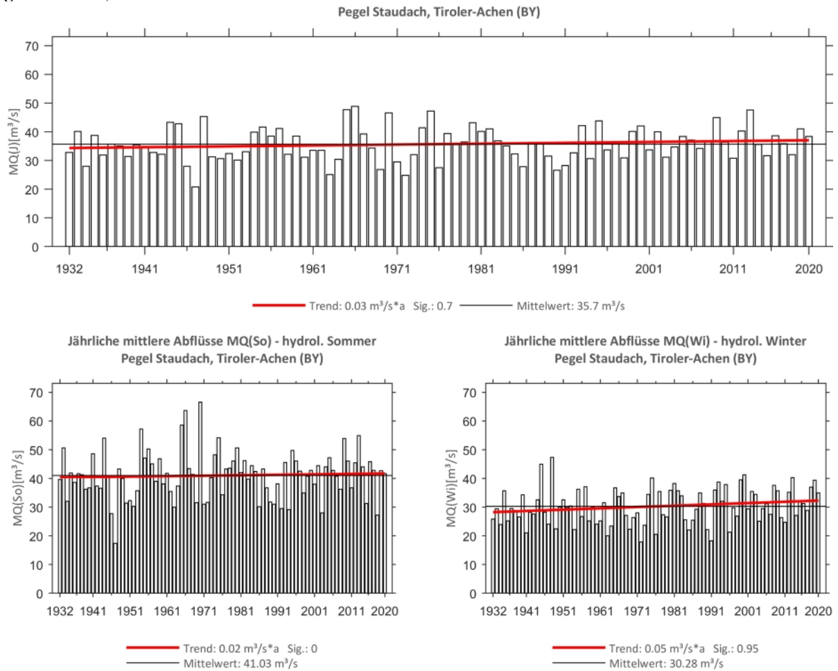
Abb. 132: Trenduntersuchungen von jährlichen mittleren Abflüssen für den Zeitraum 1932 bis 2020.
