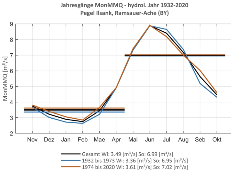
Abb. 113: Jahresgang des MonMMQ und Halbjahresmittel für 1932-2020 sowie 1932-1973 und 1974-2020
