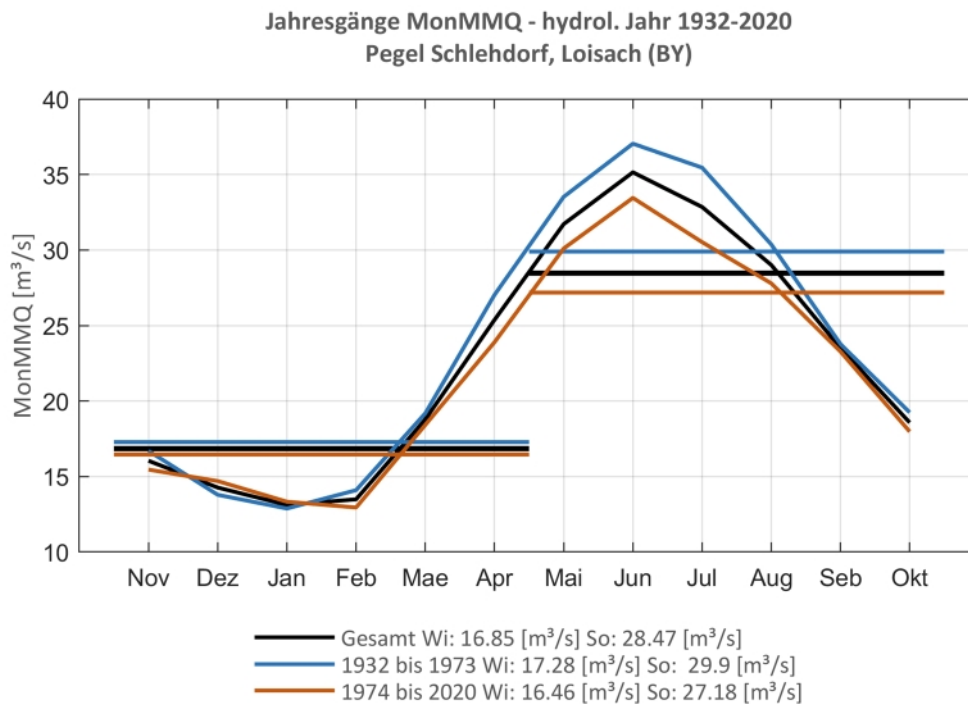
Abb. 129: Jahresgang des MonMMQ und Halbjahresmittel für 1932-2020 sowie 1932-1973 und 1974-2020
