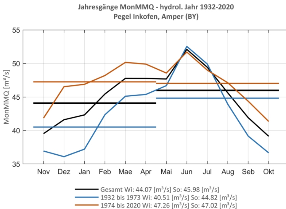
Abb. 115: Jahresgang des MonMMQ und Halbjahresmittel für 1932-2020 sowie 1932-1973 und 1974-2020
