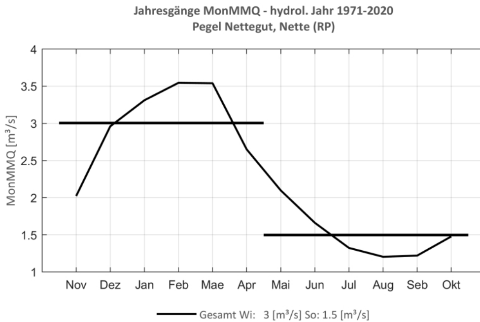
Abb. 216: Jahresgang des MonMMQ und Halbjahresmittel für 1971-2020.
