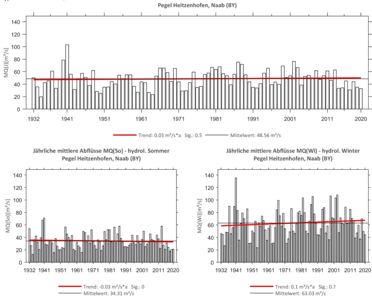
Abb. 66: Trenduntersuchungen von jährlichen mittleren Abflüssen für den Zeitraum 1932 bis 2020.
