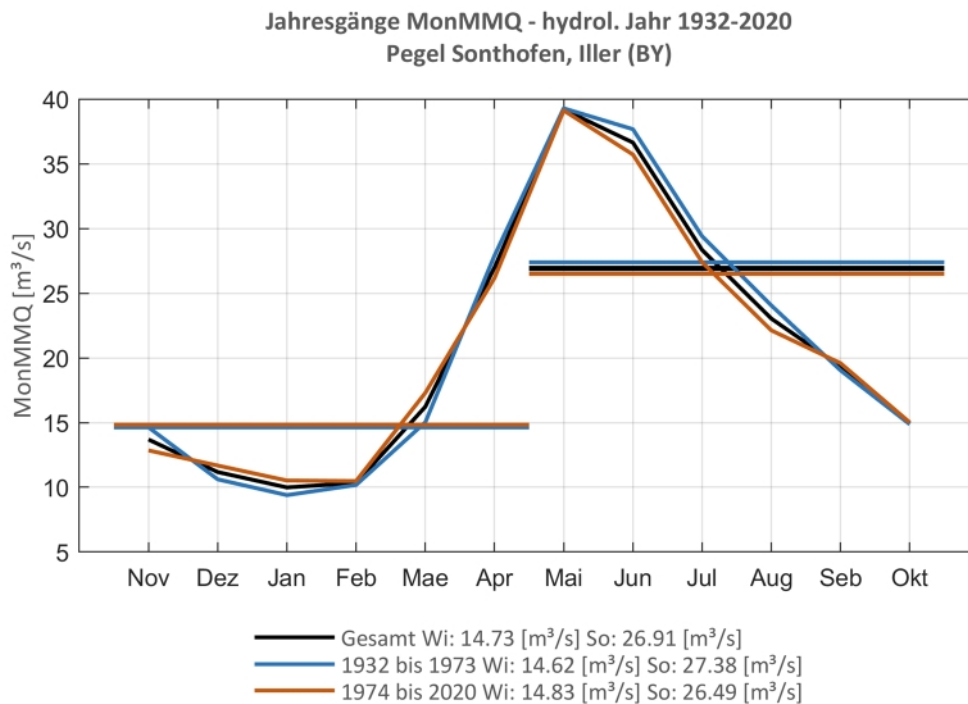
Abb. 93: Jahresgang des MonMMQ und Halbjahresmittel für 1932-2020 sowie 1932-1973 und 1974-2020
