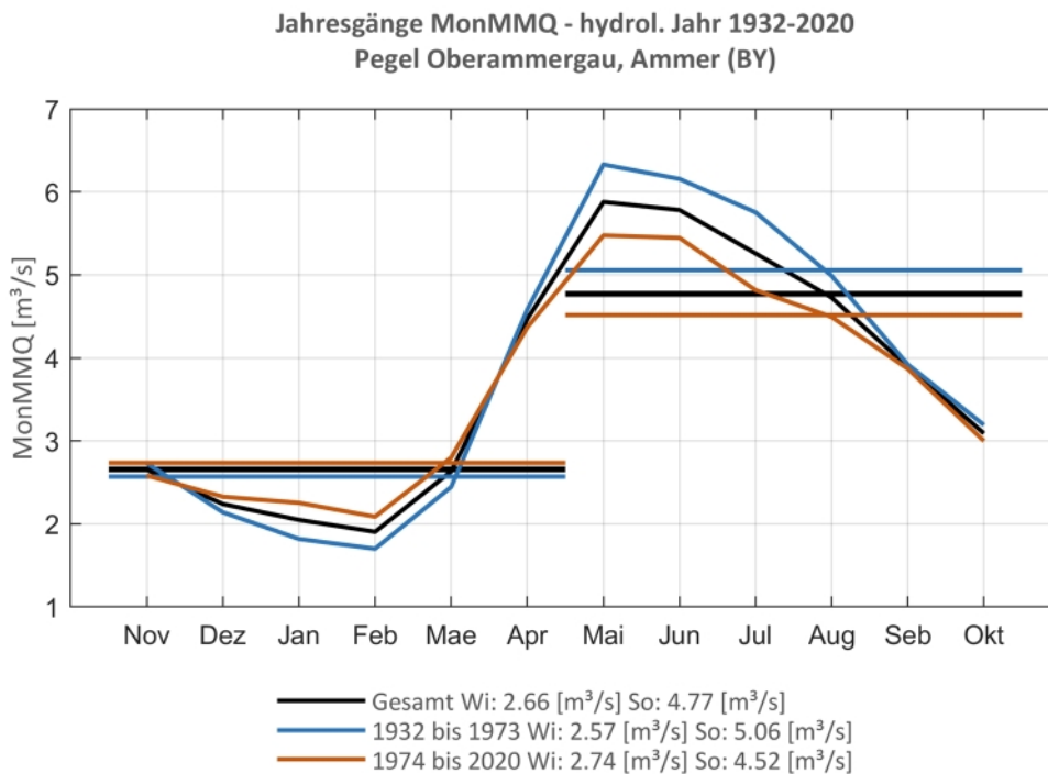
Abb. 121: Jahresgang des MonMMQ und Halbjahresmittel für 1932-2020 sowie 1932-1973 und 1974-2020
