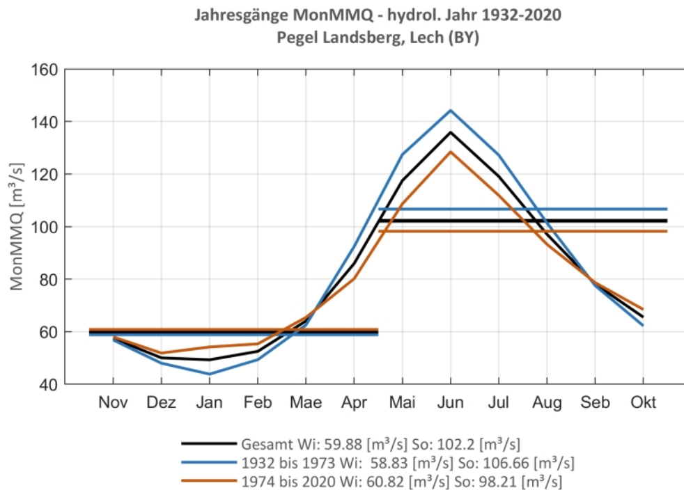
Abb. 85: Jahresgang des MonMMQ und Halbjahresmittel für 1932-2020 sowie 1932-1973 und 1974-2020
