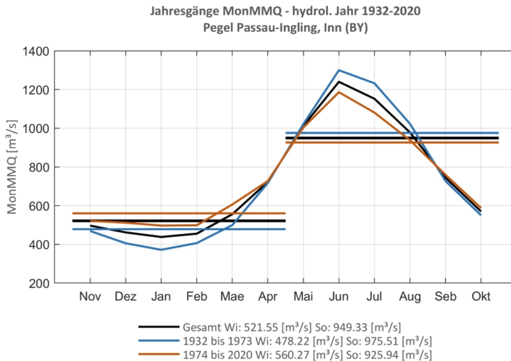
Abb. 125: Jahresgang des MonMMQ und Halbjahresmittel für 1932-2020 sowie 1932-1973 und 1974-2020
