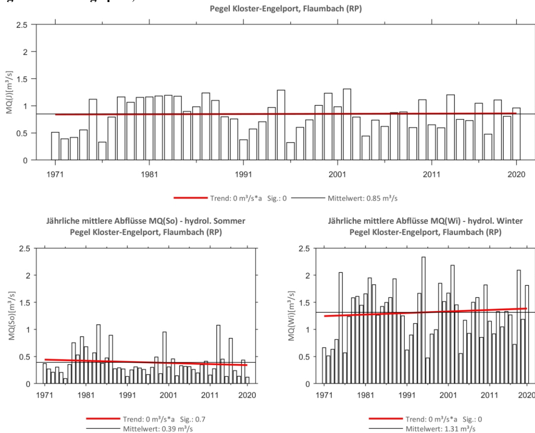
Abb. 210: Trenduntersuchungen von jährlichen mittleren Abflüssen für den Zeitraum 1971 bis 2020.
