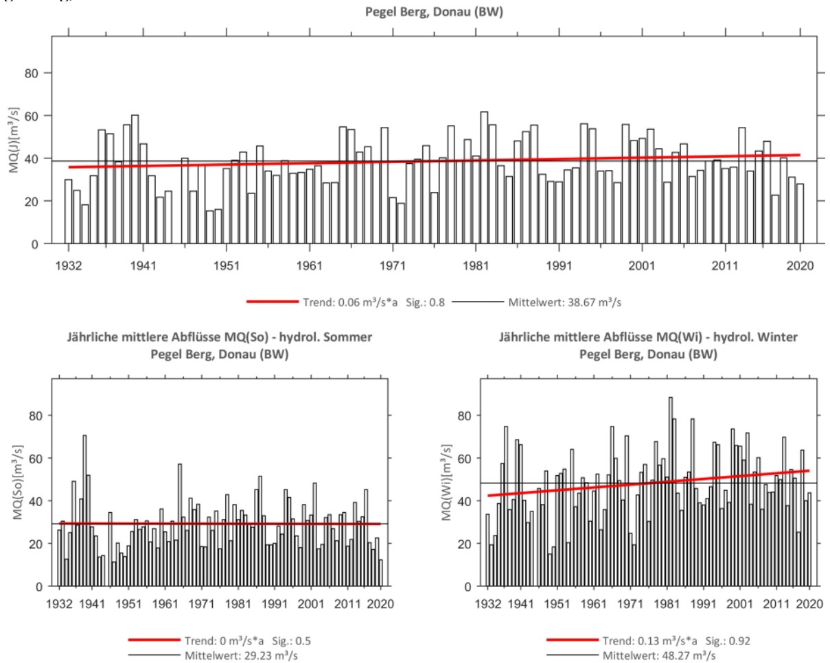
Abb. 48: Trenduntersuchungen von jährlichen mittleren Abflüssen für den Zeitraum 1932 bis 2020.
