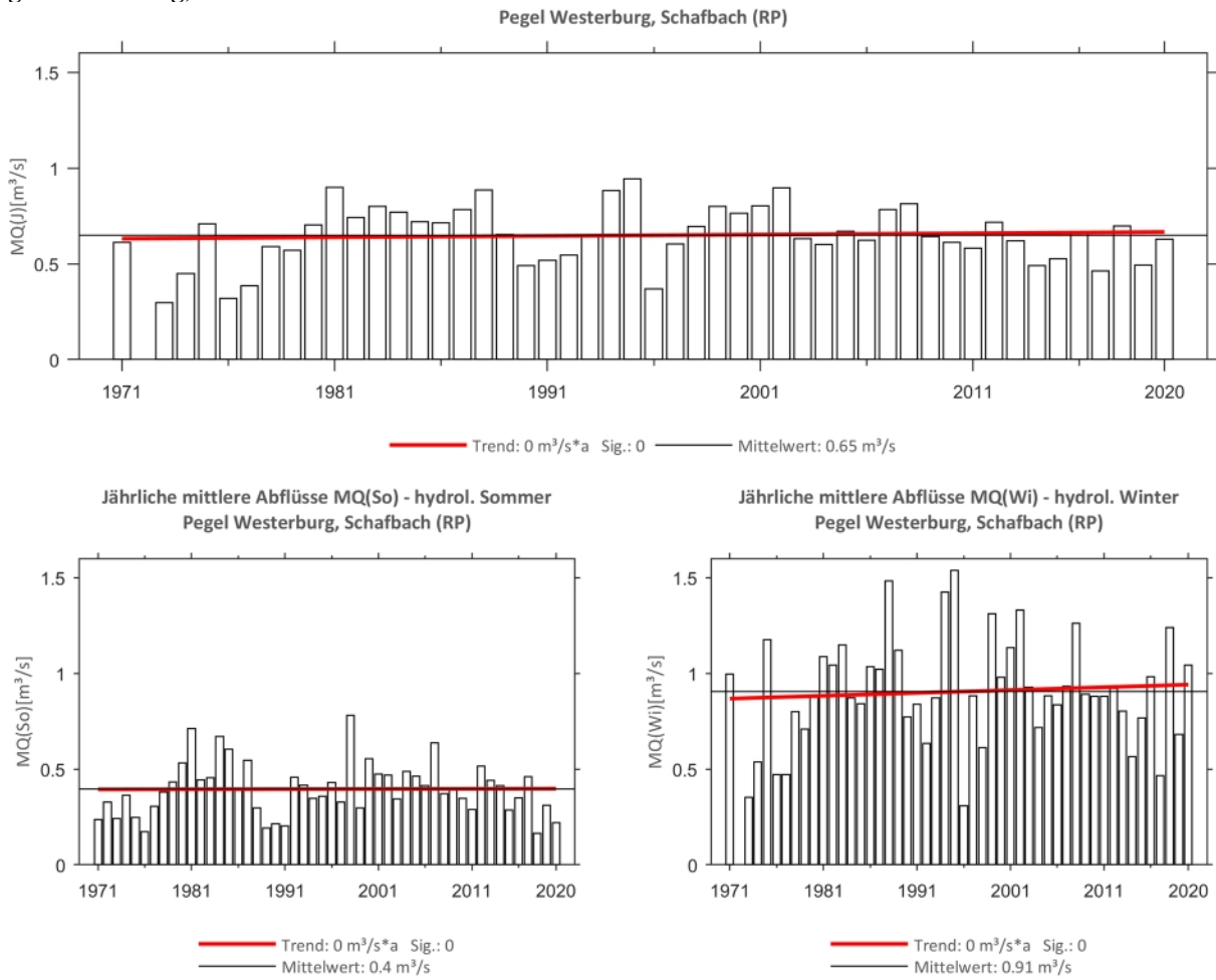
Abb. 186: Trenduntersuchungen von jährlichen mittleren Abflüssen für den Zeitraum 1971 bis 2020.
