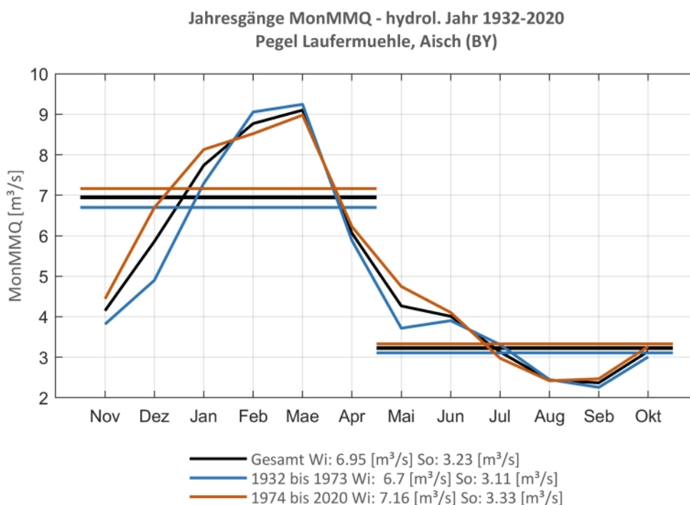
Abb. 163: Jahresgang des MonMMQ und Halbjahresmittel für 1932-2020 sowie 1932-1973 und 1974-2020
