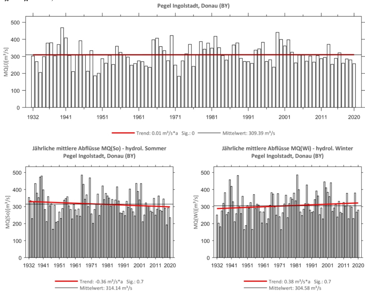
Abb. 142: Trenduntersuchungen von jährlichen mittleren Abflüssen für den Zeitraum 1932 bis 2020.
