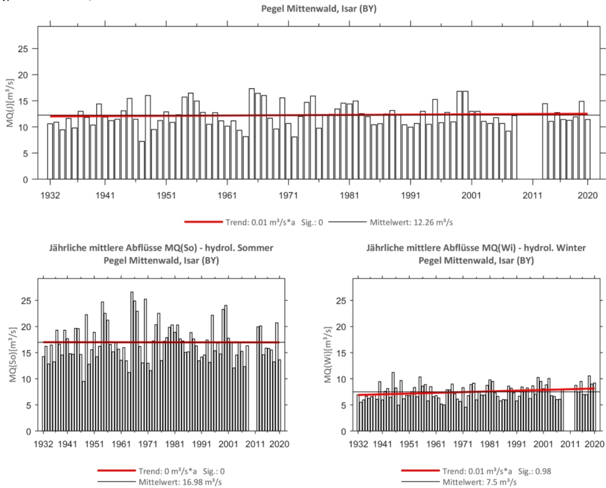
Abb. 118: Trenduntersuchungen von jährlichen mittleren Abflüssen für den Zeitraum 1932 bis 2020.
