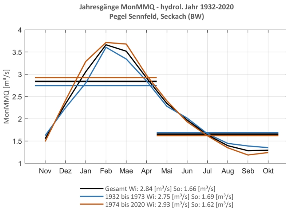
Abb. 43: Jahresgang des MonMMQ und Halbjahresmittel für 1932-2020 sowie 1932-1973 und 1974-2020.
