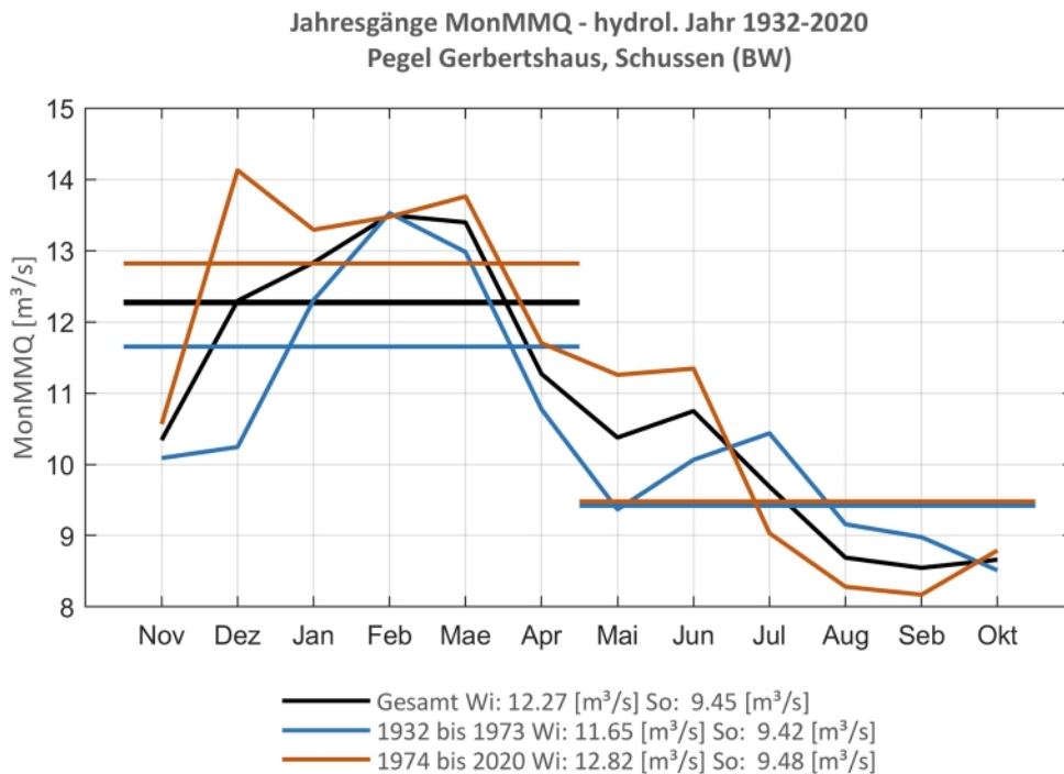
Abb. 7: Jahresgang des MonMMQ und Halbjahresmittel für 1932-2020 sowie 1932-1973 und 1974-2020.
