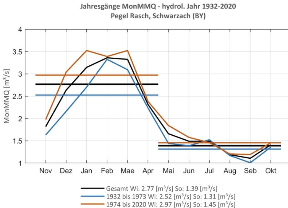
Abb. 173: Jahresgang des MonMMQ und Halbjahresmittel für 1932-2020 sowie 1932-1973 und 1974-2020
