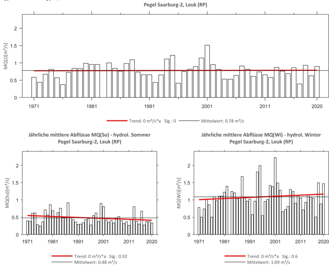
Abb. 224: Trenduntersuchungen von jährlichen mittleren Abflüssen für den Zeitraum 1971 bis 2020. Pegel Saarburtg-2, Leuk (RP)
