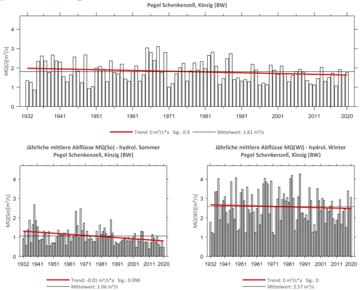
Abb. 16: Trenduntersuchungen von jährlichen mittleren Abflüssen für den Zeitraum 1932 bis 2020.
