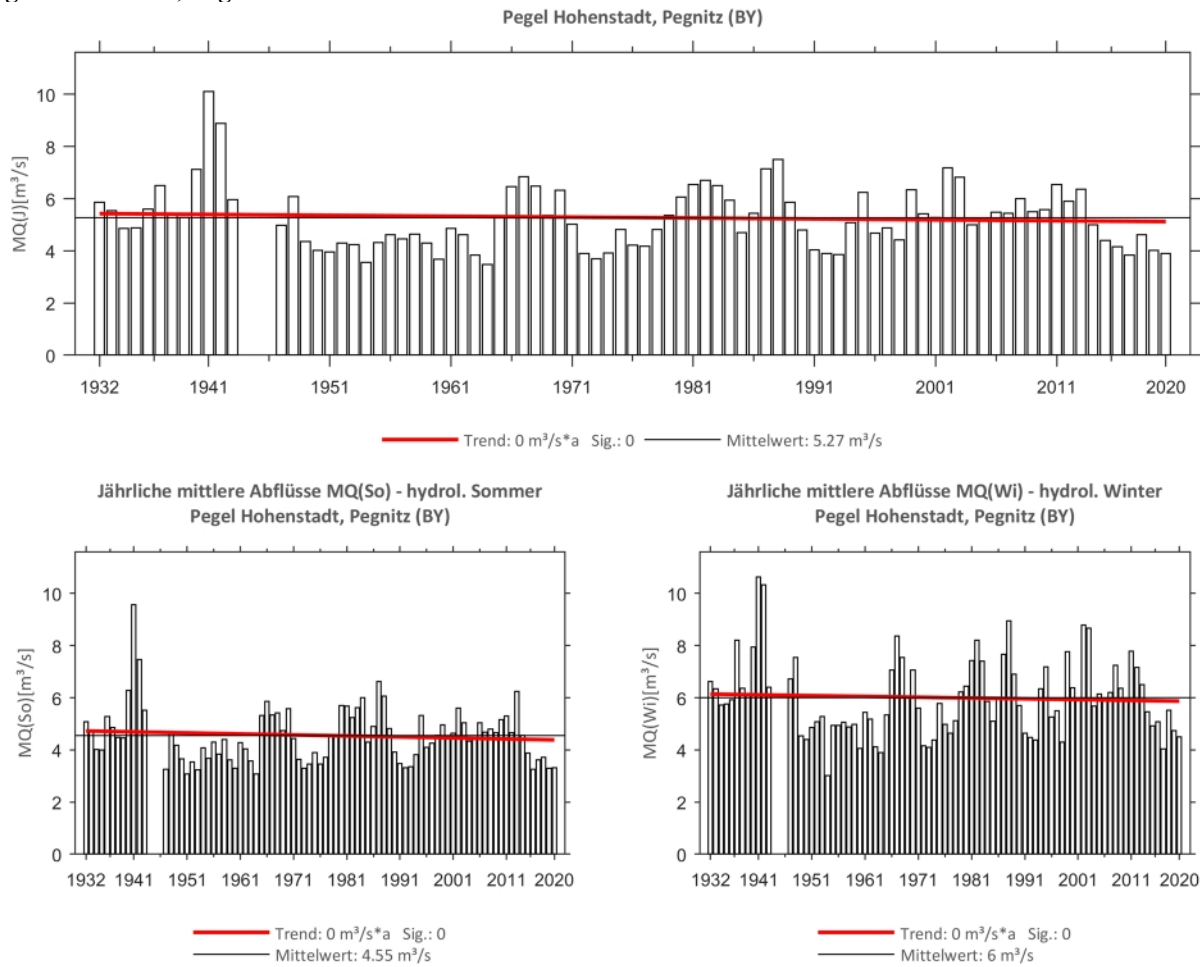
Abb. 158: Trenduntersuchungen von jährlichen mittleren Abflüssen für den Zeitraum 1932 bis 2020.
