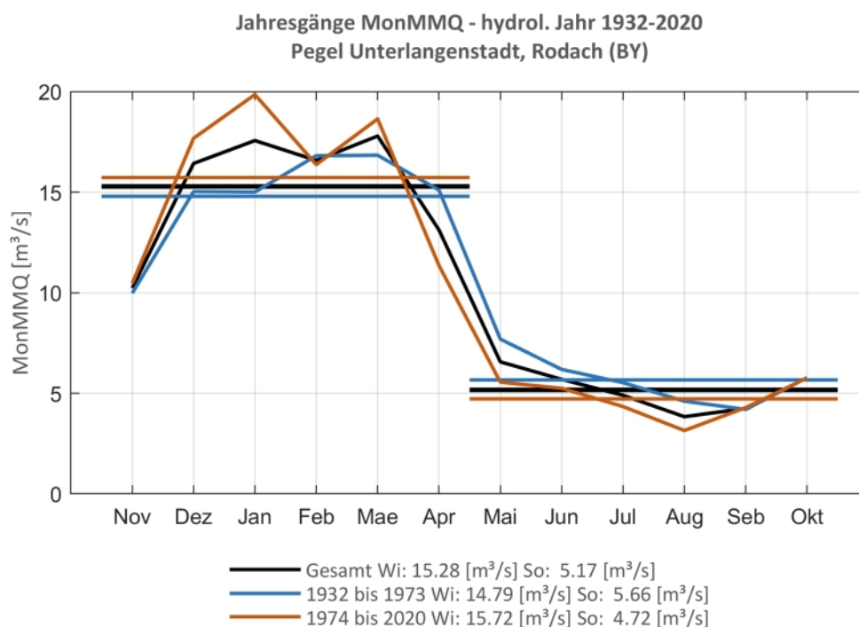
Abb. 175: Jahresgang des MonMMQ und Halbjahresmittel für 1932-2020 sowie 1932-1973 und 1974-2020
