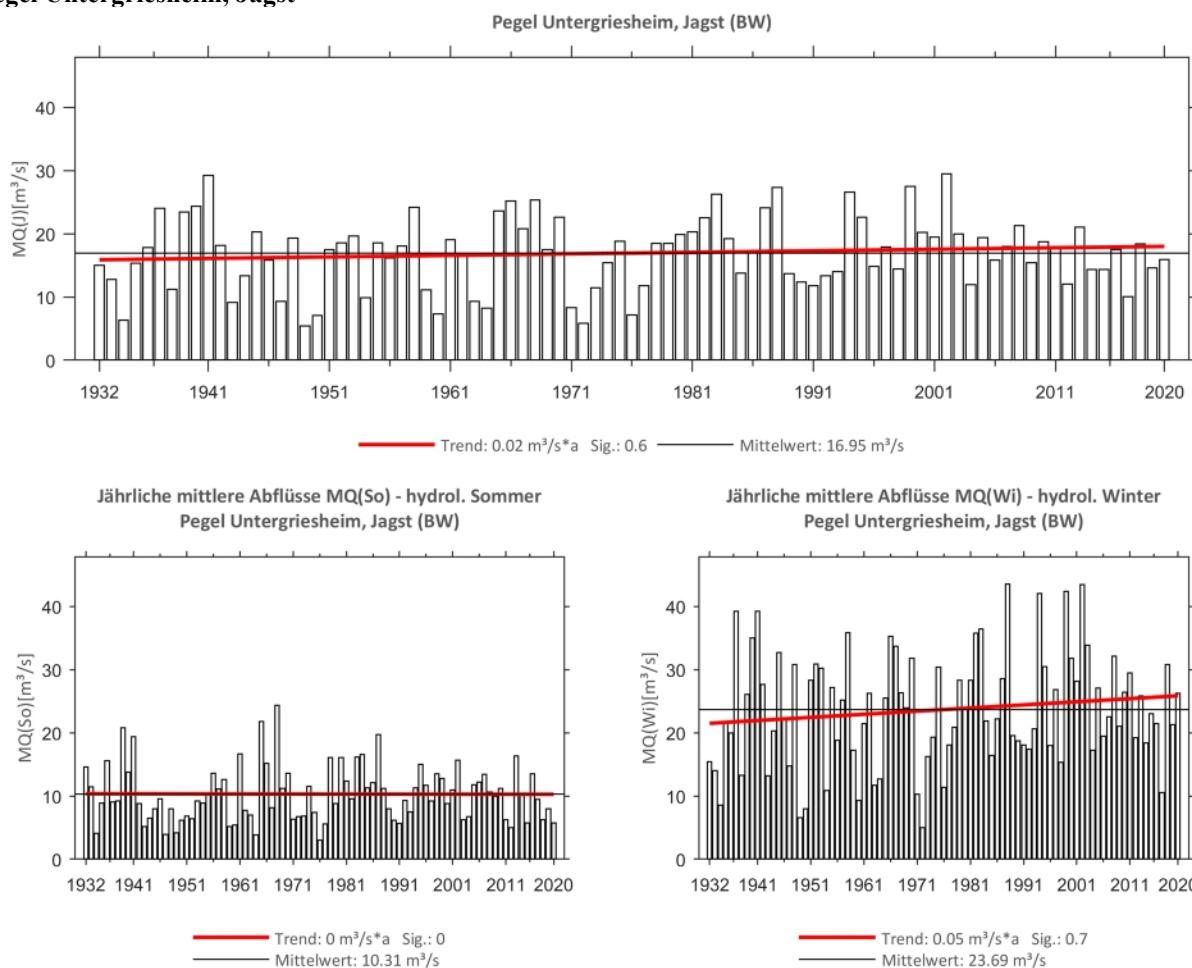
Abb. 46: Trenduntersuchungen von jährlichen mittleren Abflüssen für den Zeitraum 1932 bis 2020.
