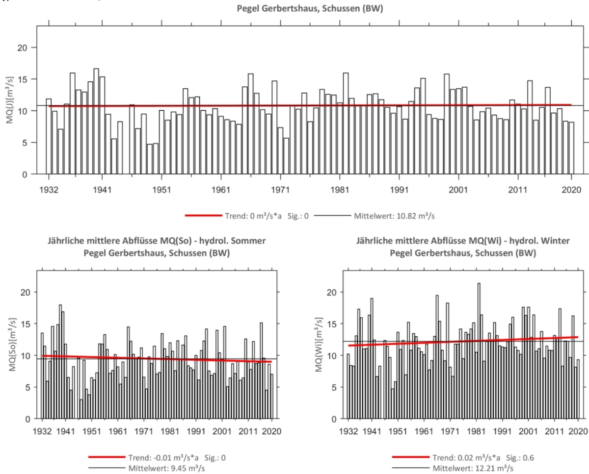
Abb. 6: Trenduntersuchungen von jährlichen mittleren Abflüssen für den Zeitraum 1932 bis 2020.
