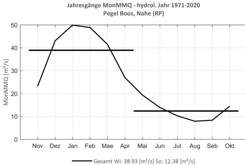
Abb. 238: Jahresgang des MonMMQ und Halbjahresmittel für 1971-2020.
