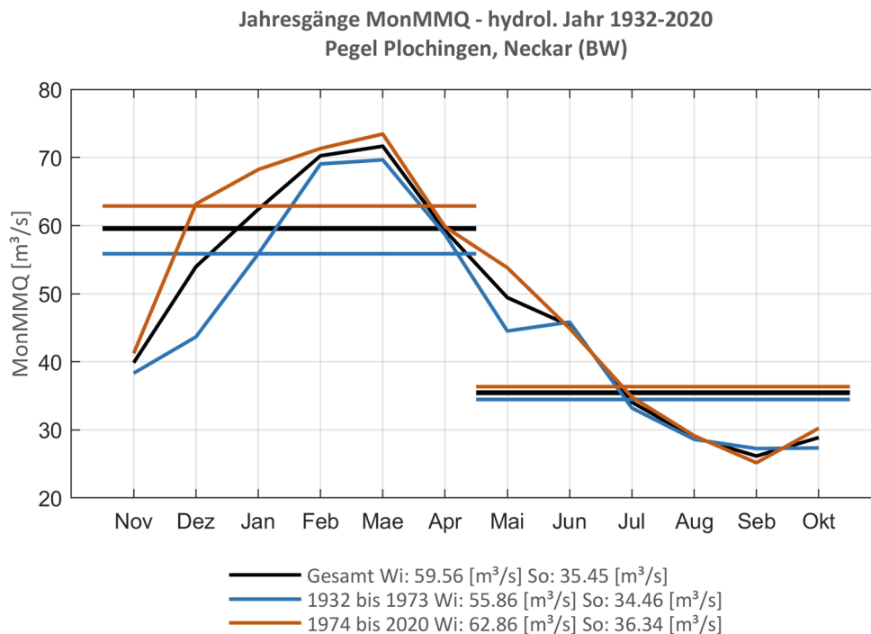
Abb. 41: Jahresgang des MonMMQ und Halbjahresmittel für 1932-2020 sowie 1932-1973 und 1974-2020.
