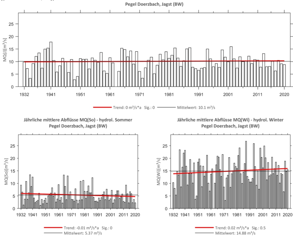
Abb. 22: Trenduntersuchungen von jährlichen mittleren Abflüssen für den Zeitraum 1932 bis 2020.
