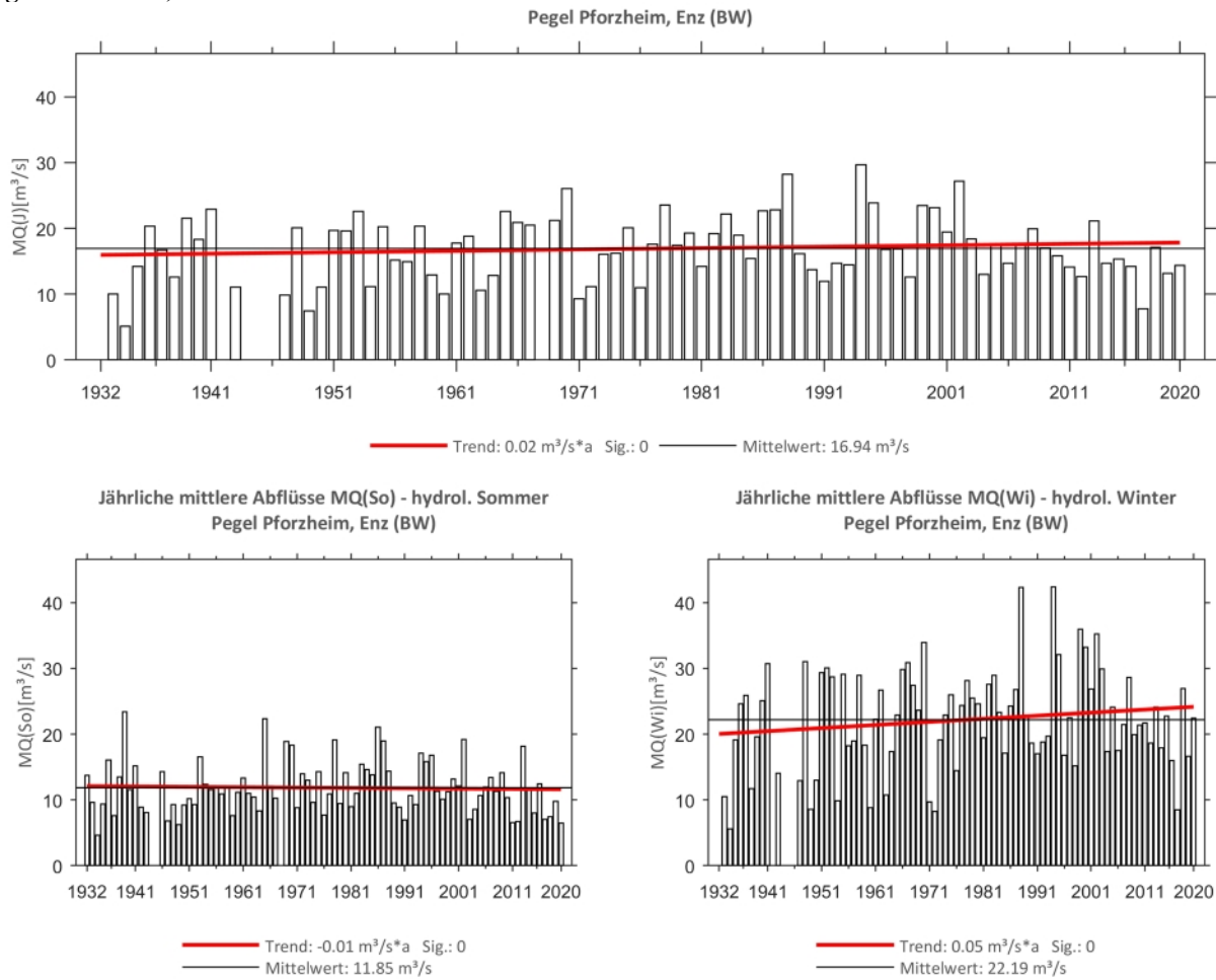
Abb. 38: Trenduntersuchungen von jährlichen mittleren Abflüssen für den Zeitraum 1933 bis 2020.
