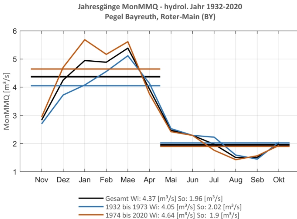
Abb. 157: Jahresgang des MonMMQ und Halbjahresmittel für 1932-2020 sowie 1932-1973 und 1974-2020
