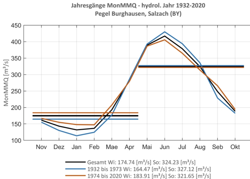
Abb. 105: Jahresgang des MonMMQ und Halbjahresmittel für 1932-2020 sowie 1932-1973 und 1974-2020
