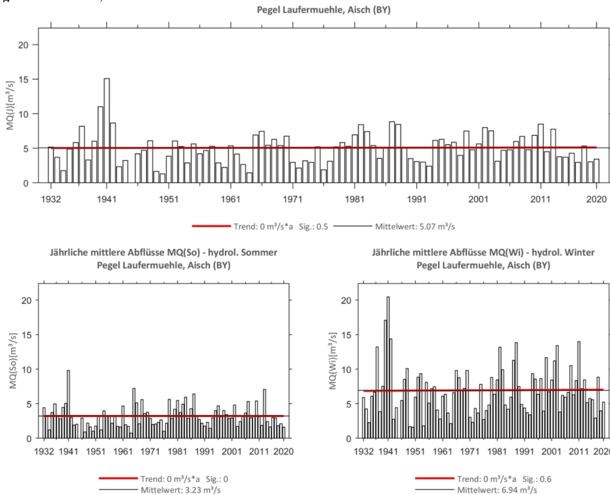
Abb. 162: Trenduntersuchungen von jährlichen mittleren Abflüssen für den Zeitraum 1932 bis 2020.
