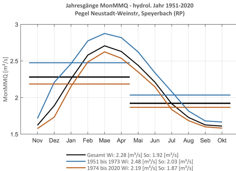
Abb. 261: Jahresgang des MonMMQ und Halbjahresmittel für 1951-2020 sowie 1974-2020.
