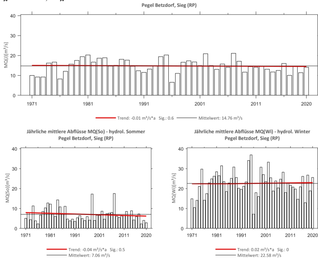
Abb. 196: Trenduntersuchungen von jährlichen mittleren Abflüssen für den Zeitraum 1971 bis 2020.
