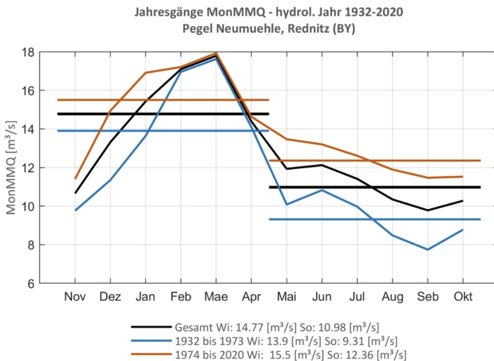
Abb. 167: Jahresgang des MonMMQ und Halbjahresmittel für 1932-2020 sowie 1932-1973 und 1974-2020
