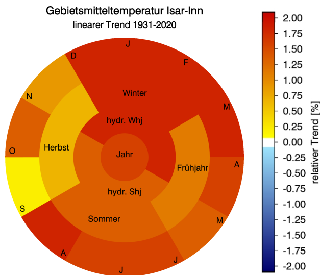
Abb. 18: Zeitreihen und Trends für die Jahresmitteltemperaturen in der KLIWA-Region Isar-Inn, mittlere Temperaturen der Halbjahre sowie Ringdiagramm mit Trendangaben (Zeitreihenlänge 1931 bis 2020)
