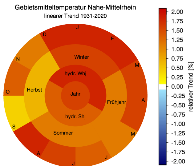
Abb. 7: Zeitreihen und Trends für die Jahresmitteltemperaturen in der KLIWA-Region Nahe-Mittelrhein, mittlere Temperaturen der Halbjahre sowie Ringdiagramm mit Trendangaben (Zeitreihenlänge 1931 bis 2020)
