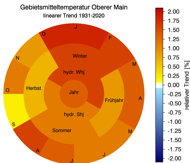
Abb. 13: Zeitreihen und Trends für die Jahresmitteltemperaturen in der KLIWA-Region Oberer Main, mittlere Temperaturen der Halbjahre sowie Ringdiagramm mit Trendangaben (Zeitreihenlänge 1931 bis 2020)
