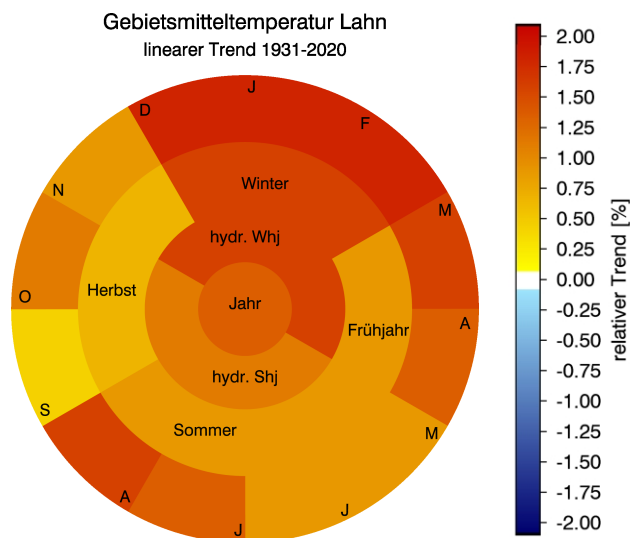
Abb. 9: Zeitreihen und Trends für die Jahresmitteltemperaturen in der KLIWA-Region Lahn, mittlere Temperaturen der Halbjahre sowie Ringdiagramm mit Trendangaben (Zeitreihenlänge 1931 bis 2020)
