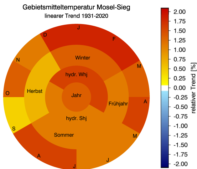
Abb. 10: Zeitreihen und Trends für die Jahresmitteltemperaturen in der KLIWA-Region : Mosel-Sieg, mittlere Temperaturen der Halbjahre sowie Ringdiagramm mit Trendangaben (Zeitreihenlänge 1931 bis 2020)
