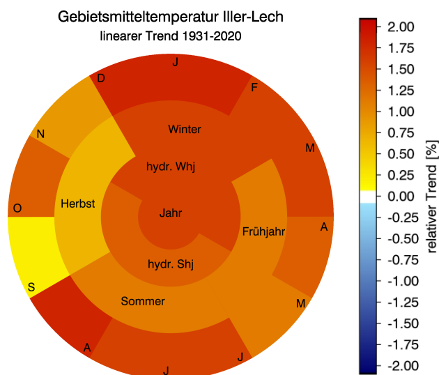
Abb. 19: Zeitreihen und Trends für die Jahresmitteltemperaturen in der KLIWA-Region Iller-Lech, mittlere Temperaturen der Halbjahre sowie Ringdiagramm mit Trendangaben (Zeitreihenlänge 1931 bis 2020)
