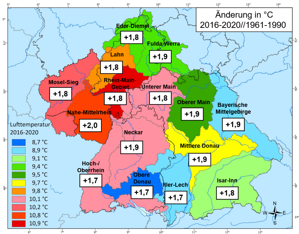
Abb. 5: Mittlere Lufttemperatur in °C im Zeitraum 2016-2020 (farbig) und die Abweichung vom Mittelwert 1961-1990 (Zahlen) für die KLIWA-Regionen.
