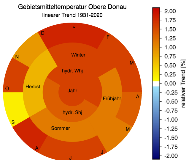
Abb. 20: Zeitreihen und Trends für die Jahresmitteltemperaturen in der KLIWA-Region Obere Donau, mittlere Temperaturen der Halbjahre sowie Ringdiagramm mit Trendangaben (Zeitreihenlänge 1931 bis 2020)
