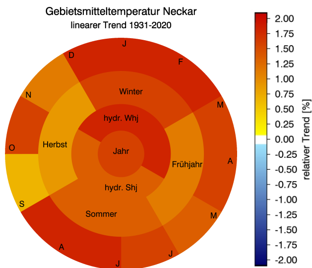
Abb. 14: Zeitreihen und Trends für die Jahresmitteltemperaturen in der KLIWA-Region Neckar, mittlere Temperaturen der Halbjahre sowie Ringdiagramm mit Trendangaben (Zeitreihenlänge 1931 bis 2020)
