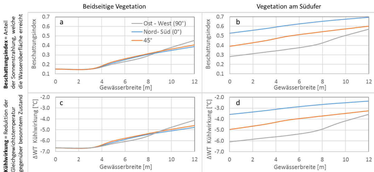
Abbildung 4: Tagesmittel des minimal erzielbaren Beschattungsindex (BI) und der maximal erzielbaren Kühlwirkung ( \Delta W T ) für unterschiedliche Fließrichtungen in Abhängigkeit von der Gewässerbreite. Bei beidseitiger Ufervegetation (a) und (c) sowie bei Vegetation nur am südlichen Ufer (b) und (d). Berechnungsgrundlagen: 15 m hohe Bäume mit 1,5 m Kronenüberhang, meteorologische Bedingungen eines charakteristischen 1. Augusts (Zeile 1 in Tabelle 1).
