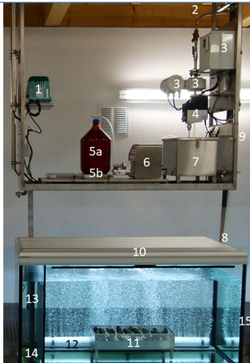
Abb. 14: Aquarium mit technischem Aufbau und Edelstahleinsatz mit Großen Flussmuscheln ( Unio tumidus ) zur Exposition mit PVC-Mikropartikeln
