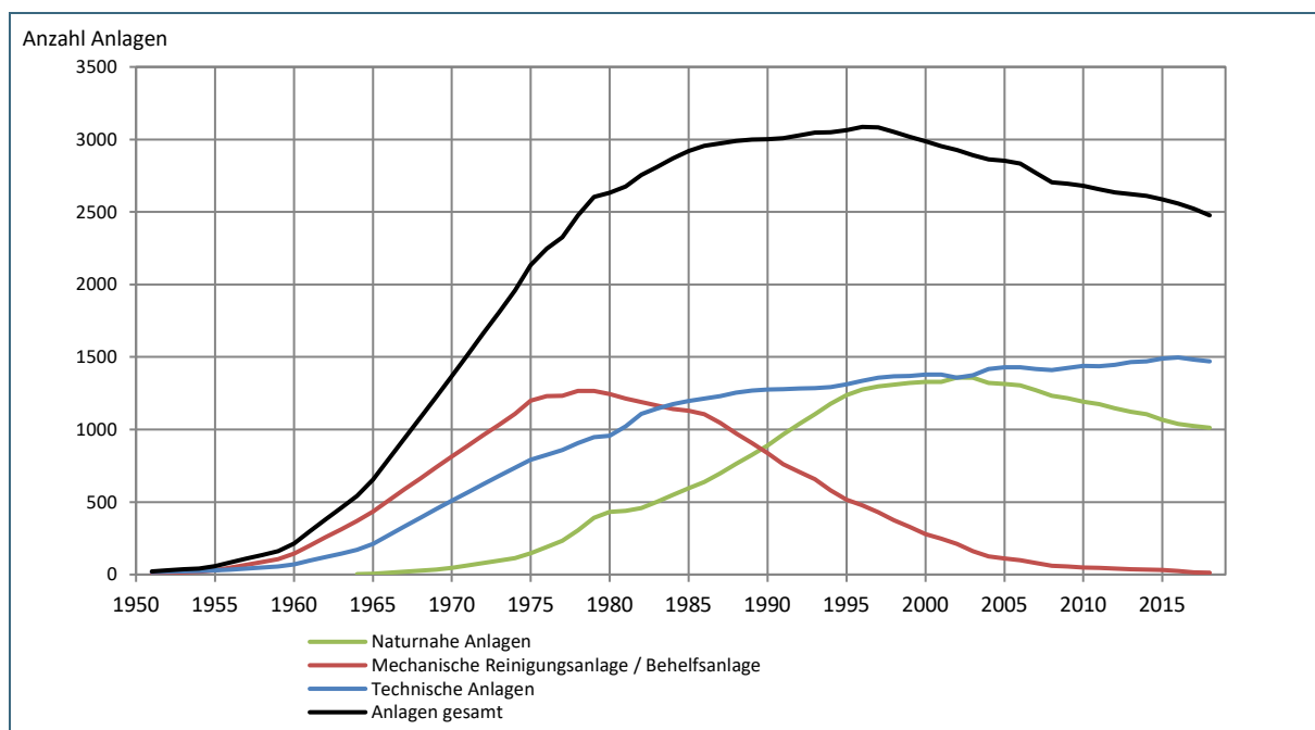
Abb. 6: Entwicklung der Anzahl der kommunalen Kläranlagen in Bayern von 1950 bis 2018
