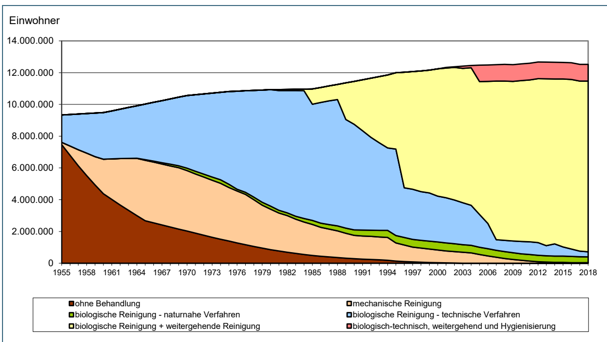
Abb. 11: Reinigungsniveau des kommunalen Abwassers in Bayern von 1955 bis 2018
