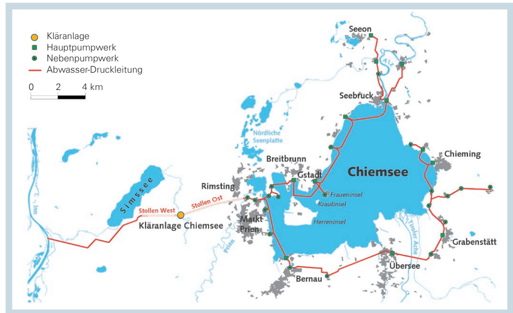
Ringkanalisation Chiemsee
