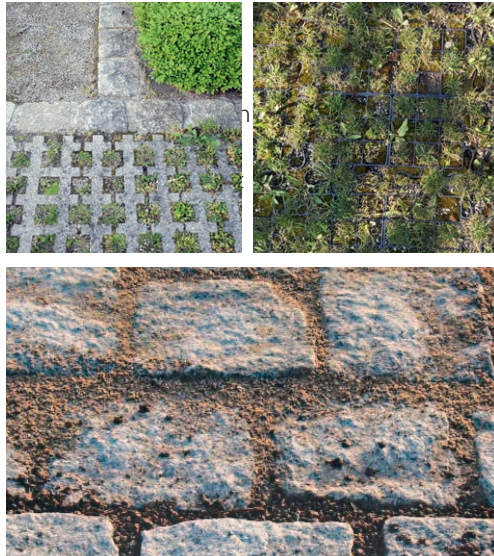
Wasserdurchlässige Bodenbefestigung
