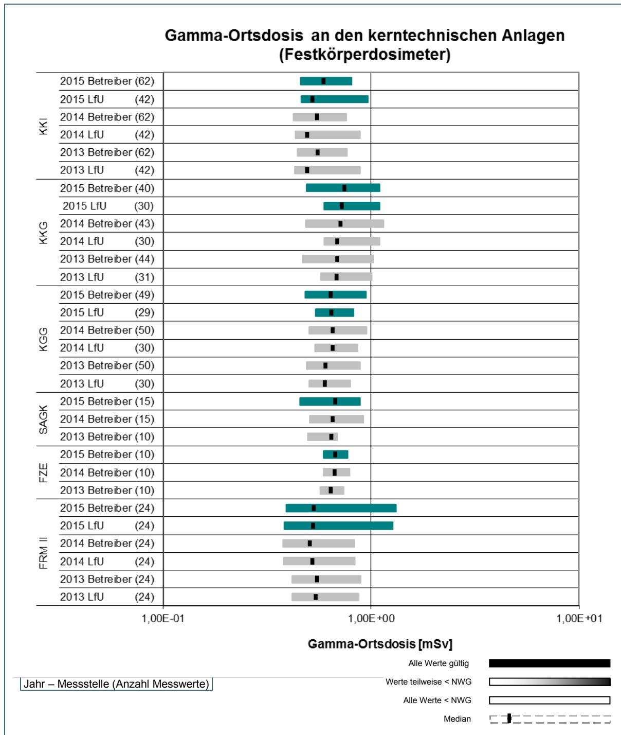
Abb. 11: Übersicht über die Wertebereiche der Gamma-Ortsdosis (Jahresdosis von Festkörperdosimetern) gem. REI, Tabelle A1, Punkt 1.1b und Tabelle A2, Punkt 1.1 im Jahr 2015 im Vergleich zu den Vorjahren 2014 und 2013.
