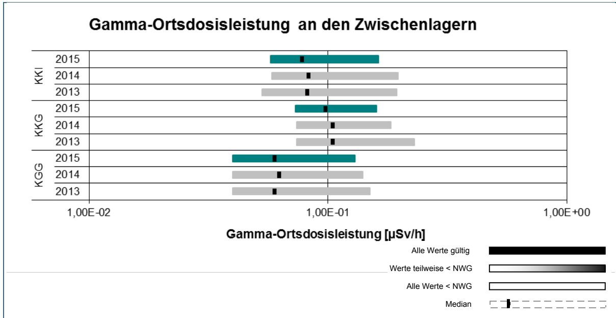
Abb. 13: Übersicht über die Wertebereiche der Gamma-Ortsdosisleistung (G-ODL) an den Brennelementzwischenlagern gem. REI, Tabelle C1.1, Punkt 1.1 im Jahr 2015 im Vergleich zu den Vorjahren 2014 und 2013
