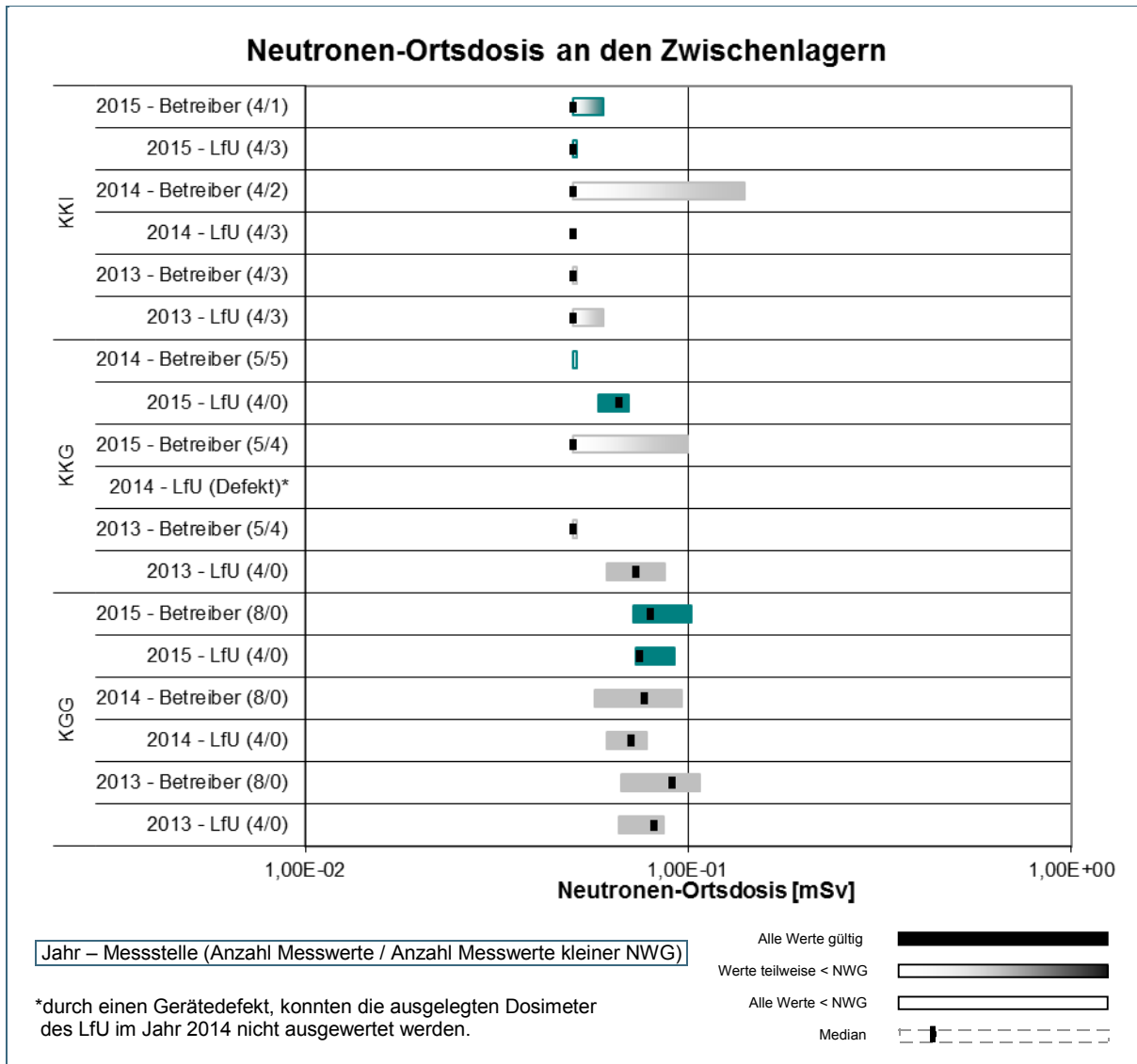
Abb. 16: Übersicht über die Wertebereiche der Neutronen-Ortsdosis (N-OD) an den Brennelementzwischenlagern gem. REI, Tabelle C.1.1, Punkt 1.4 und Tabelle C.1.2, Punkt 1.2 im Jahr 2015 im Vergleich zu den Vorjahren 2014 und 2013
