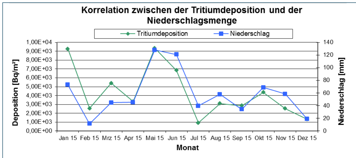
Abb. 12: Vergleich der Messwerte von Tritium und der Niederschlagsmenge am Messpunkt „FRM-Dachablauf“ der Forschungsneutronenquelle Heinz Maier-Leibnitz im Jahr 2015
