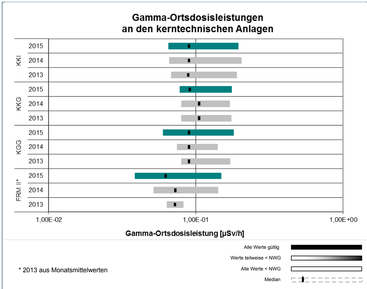
Abb. 10: Übersicht über die Wertebereiche der Gamma-Ortsdosisleistung an den kerntechnischen Anlagen (aus 10-Minuten-Messwerten) gem. REI, Tabelle A1, Punkt 1.1a im Jahr 2015 im Vergleich zu den Vorjahren 2014 und 2013.
