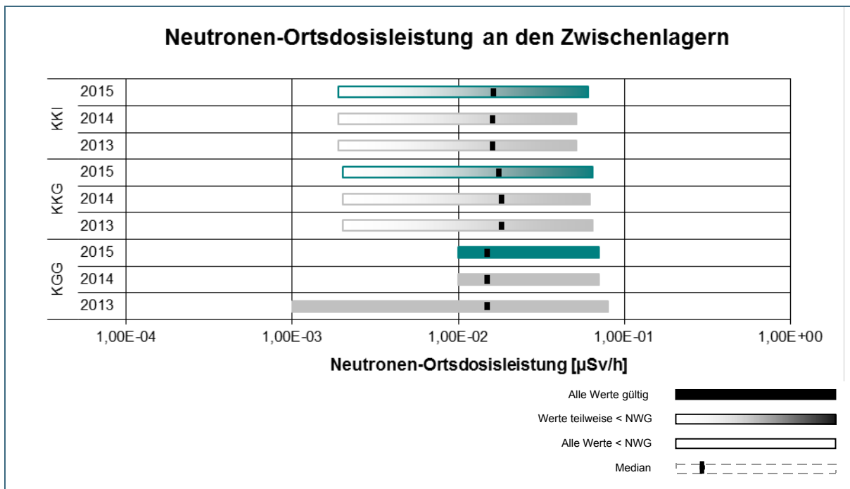
Abb. 14: Übersicht über die Wertebereiche der Neutronen-Ortsdosisleistung (N-ODL) an den Brennelementzwischenlagern gem. REI, Tabelle C1.1, Punkt 1.3 im Jahr 2015 im Vergleich zu den Vorjahren 2014 und 2013
