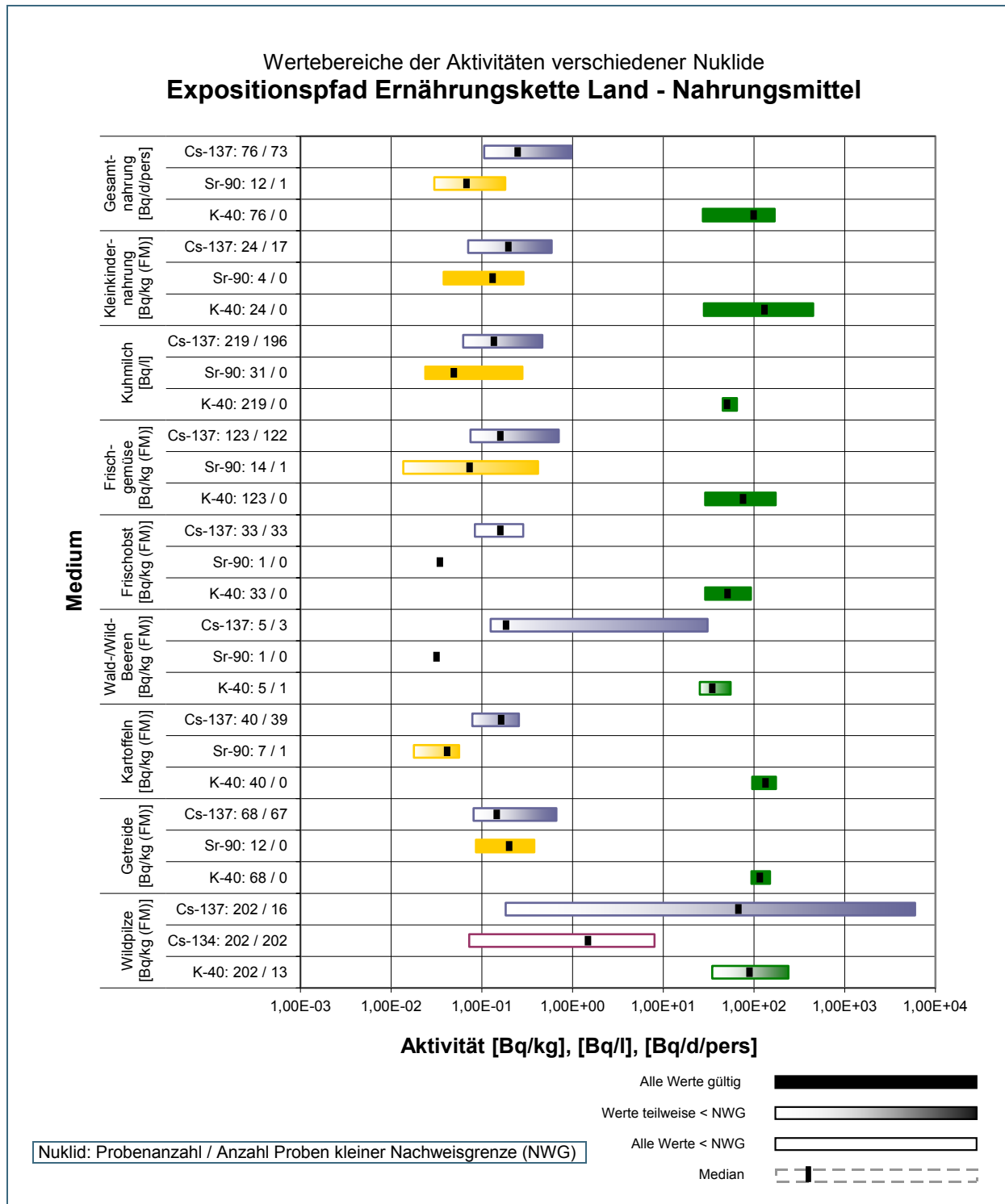
Abb. 4: Wertebereiche der in Bayern gemessenen Aktivitäten des Expositionspfad Ernährungskette Land – Nahrungsmittel (ohne tierische Lebensmittel) im Jahr 2014
