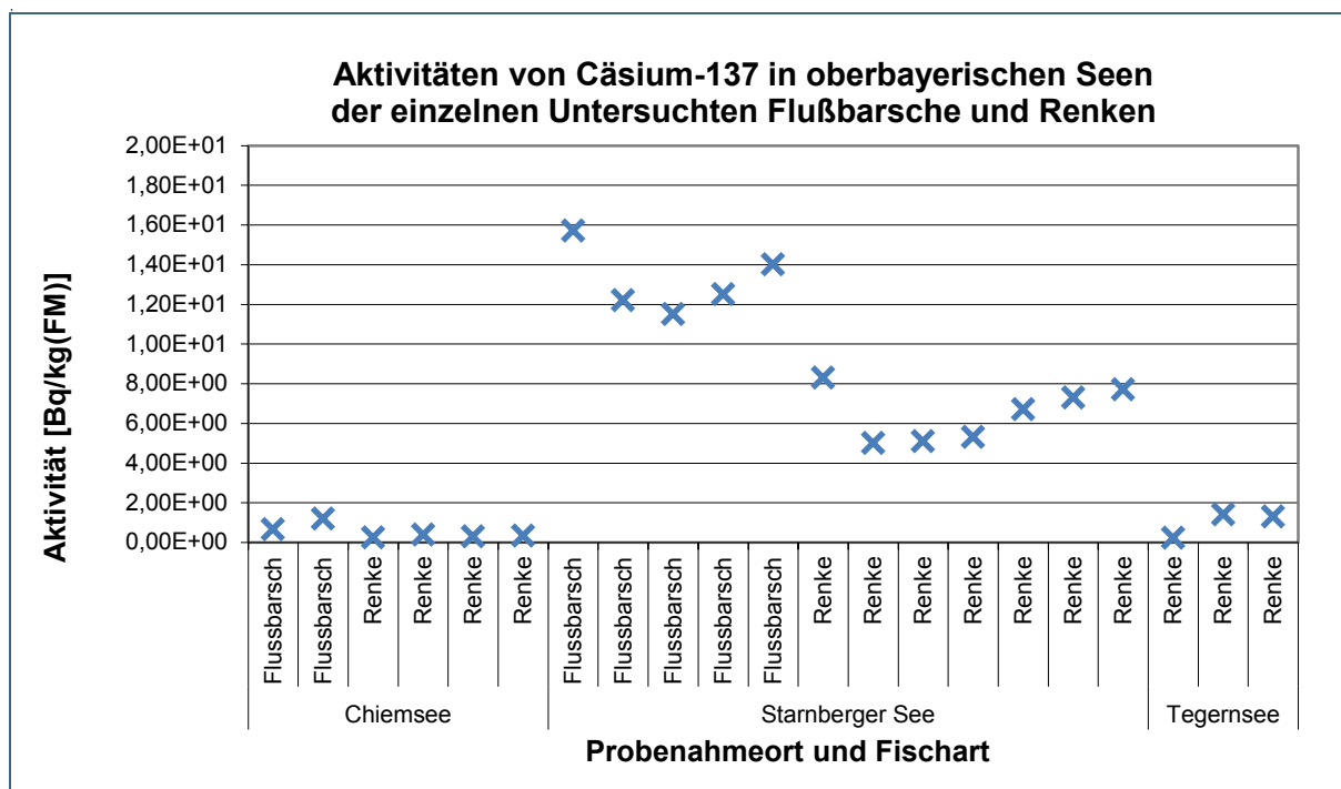
Abb. 8: Aktivitätsmesswerte (Cäsium-137) von 7 Flußbarschen und 14 Renken, die in den Jahren 2012 bis 2014 aus oberbayerischen Seen entnommen wurden
