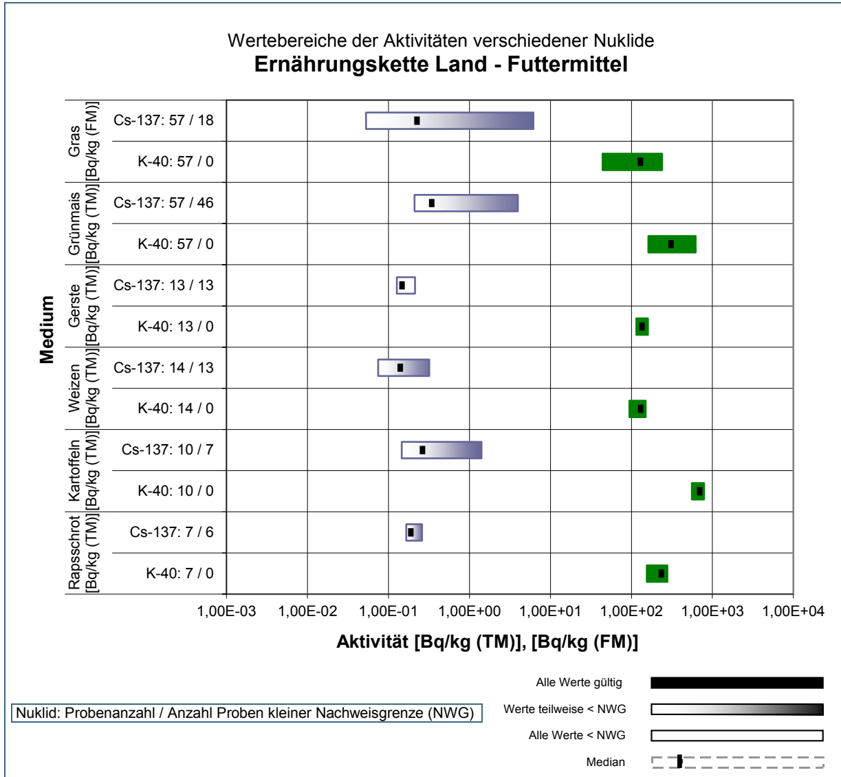
Abb. 6: Wertebereiche der in Bayern gemessenen Aktivitäten des Expositionspfads Ernährungskette Land – Futtermittel im Jahr 2014
