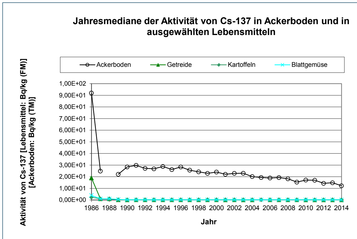
Abb. 3: Zeitlicher Verlauf der Aktivität von Cäsium-137 in Ackerboden und ausgewählten landwirtschaftlichen Produkten (für das Jahr 1988 liegen keine Messwerte für Ackerboden vor)
