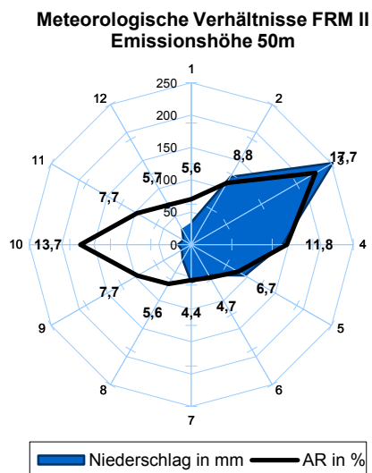
Abb. 18: Häufigkeitsverteilung der Ausbreitungsrichtung (AR) in % sowie die Niederschlagsmenge in mm pro Sektor der überwachten kerntechnischen Anlagen im Jahr 2013
