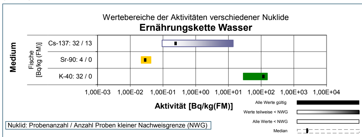
Abb. 7: Wertebereiche der in Bayern gemessenen Aktivitäten des Expositionspfades Ernährungskette Wasser im Jahr 2014
