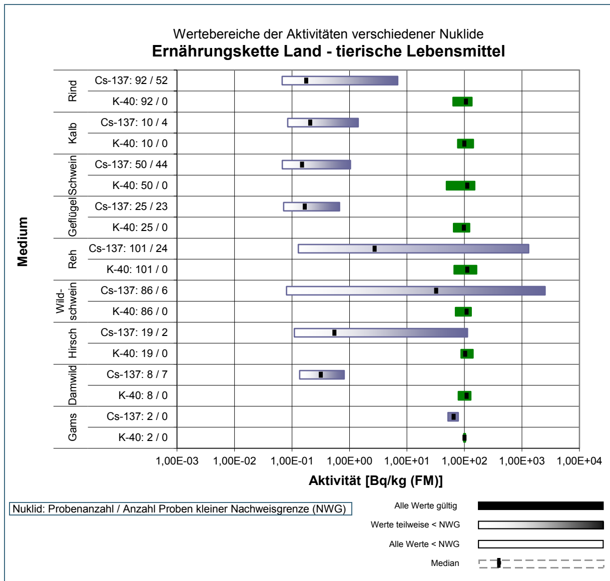
Abb. 5: Wertebereiche der in Bayern gemessenen Aktivitäten des Expositionspfads Ernährungskette Land – tierische Lebensmittel im Jahr 2014
