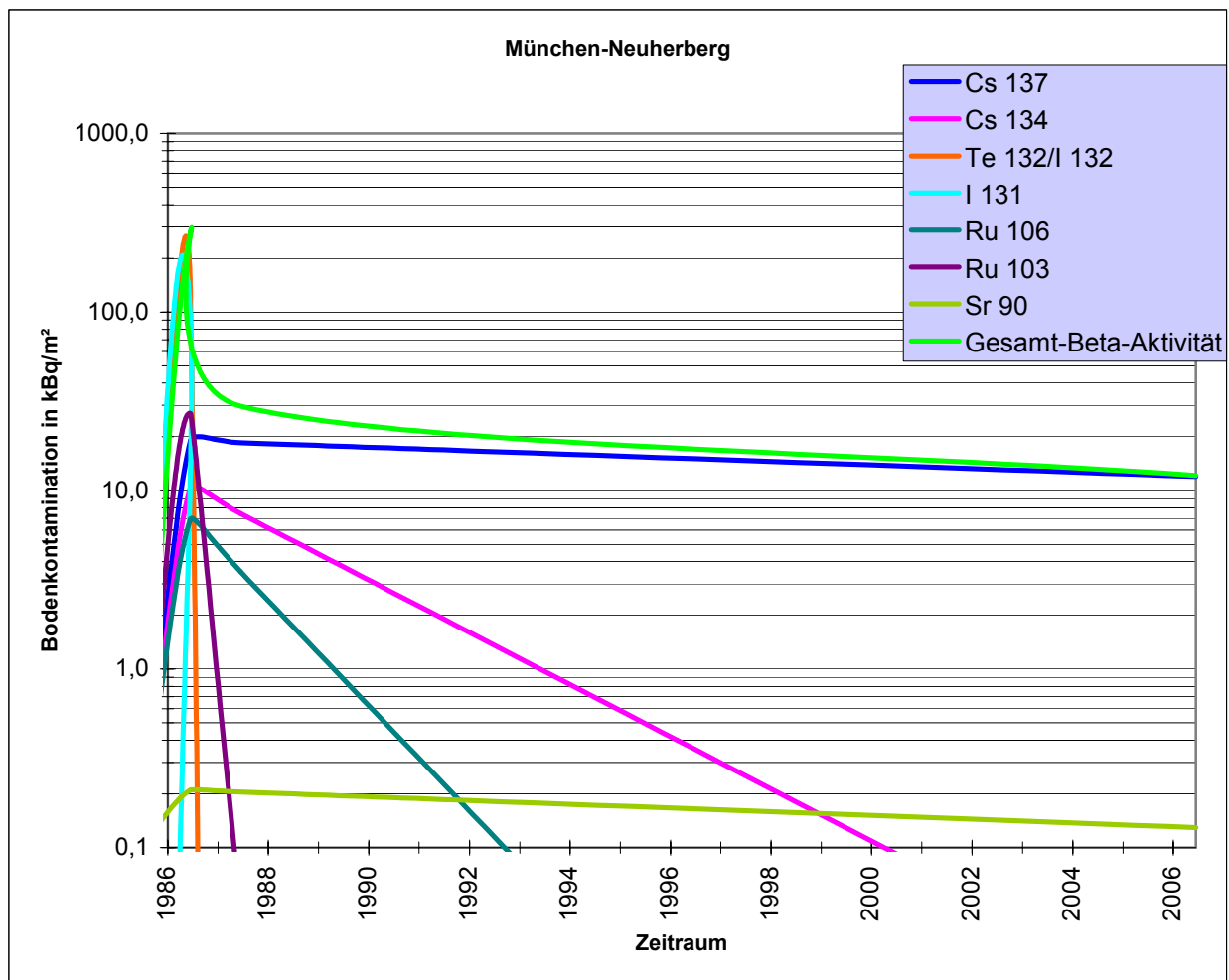
Abb. 10: Abklingkurven der aus dem natürlichen radioaktiven Zerfall zu erwartenden zeitlichen Veränderungen der seinerzeit in München-Neuherberg festgestellten Bodenkontamination.
