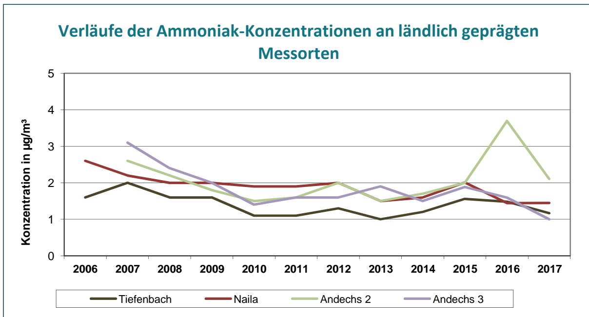
Abb. 6: Verläufe der Ammoniak-Konzentrationen an den ländlich geprägten Messorten über den gesamten Messzeitraum
