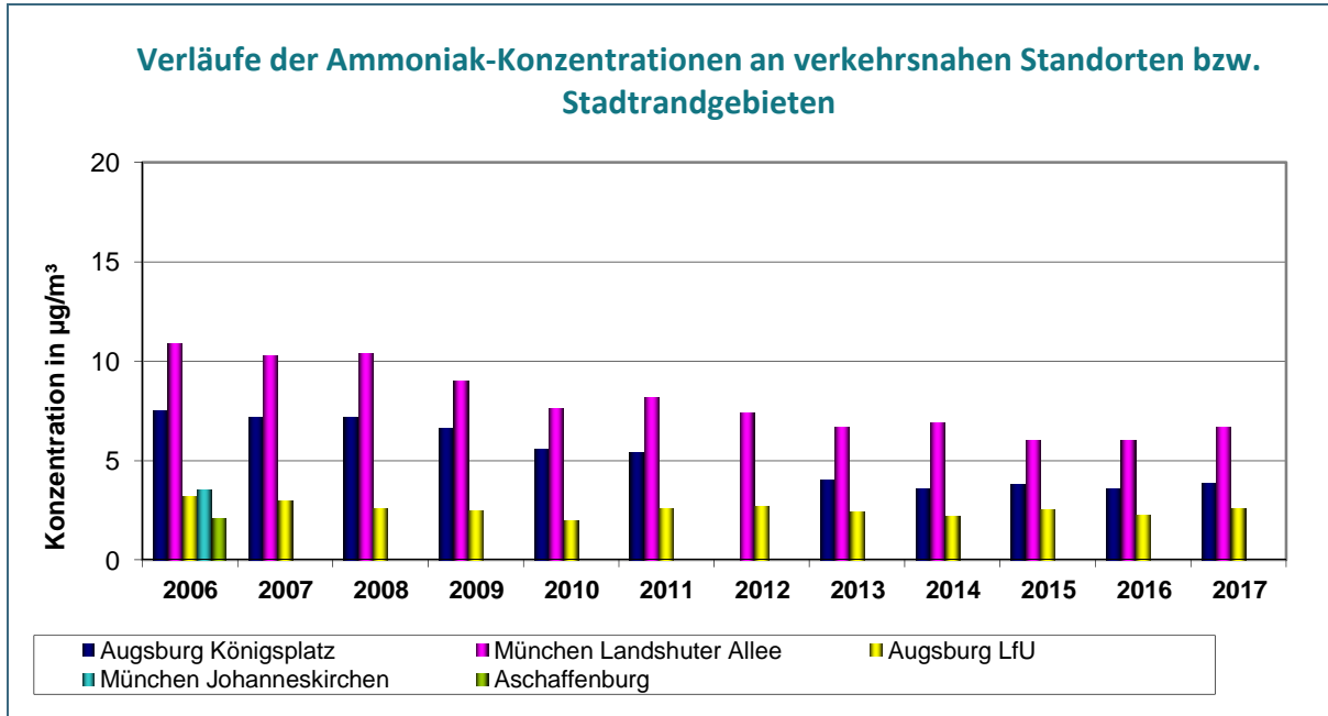
Abb. 9: Auswertung bis 2017 – verkehrsnaher Messort im Vergleich zu stadtrandnahen Messorten
