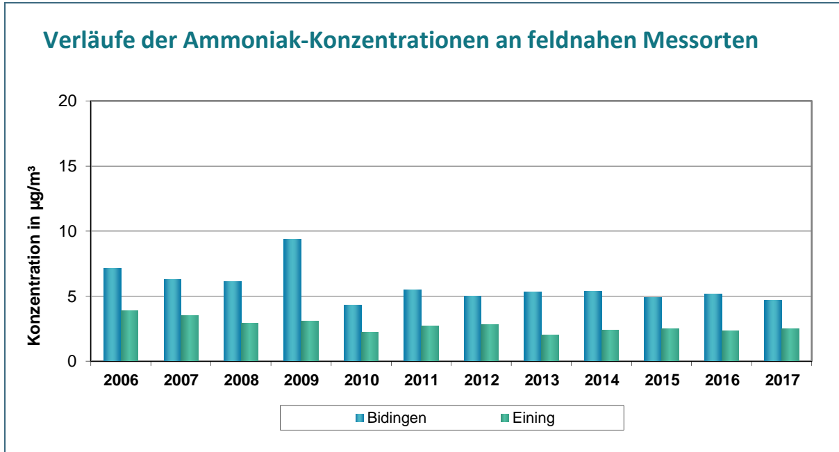
Abb. 3: Auswertung bis 2017 – feldnahe Messorte
