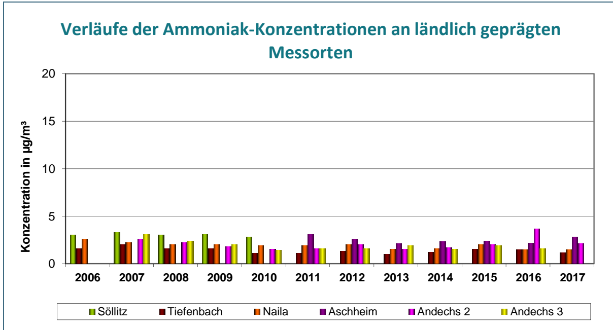
Abb. 5: Auswertung bis 2017 – ländlich geprägte Messorte
