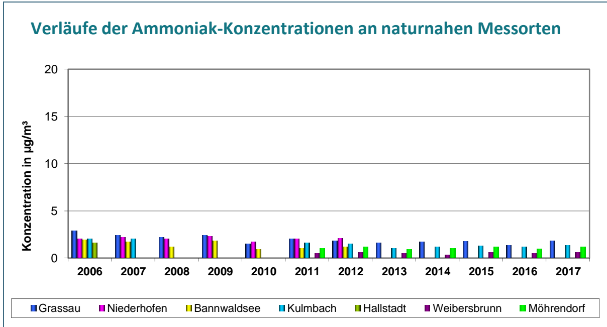
Abb. 7: Auswertung bis 2017 – naturnahe Messorte
