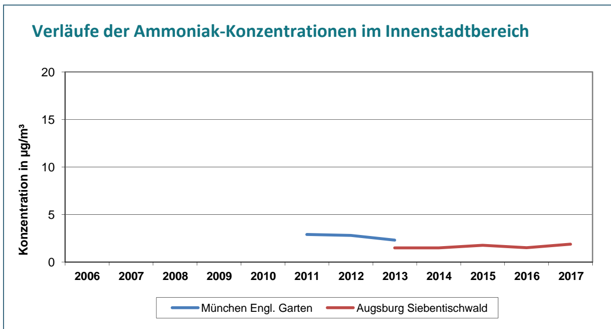
Abb. 12: Verläufe der Ammoniak-Konzentrationen im Innenstadtbereich von München und Augsburg von 2011 bis 2017
