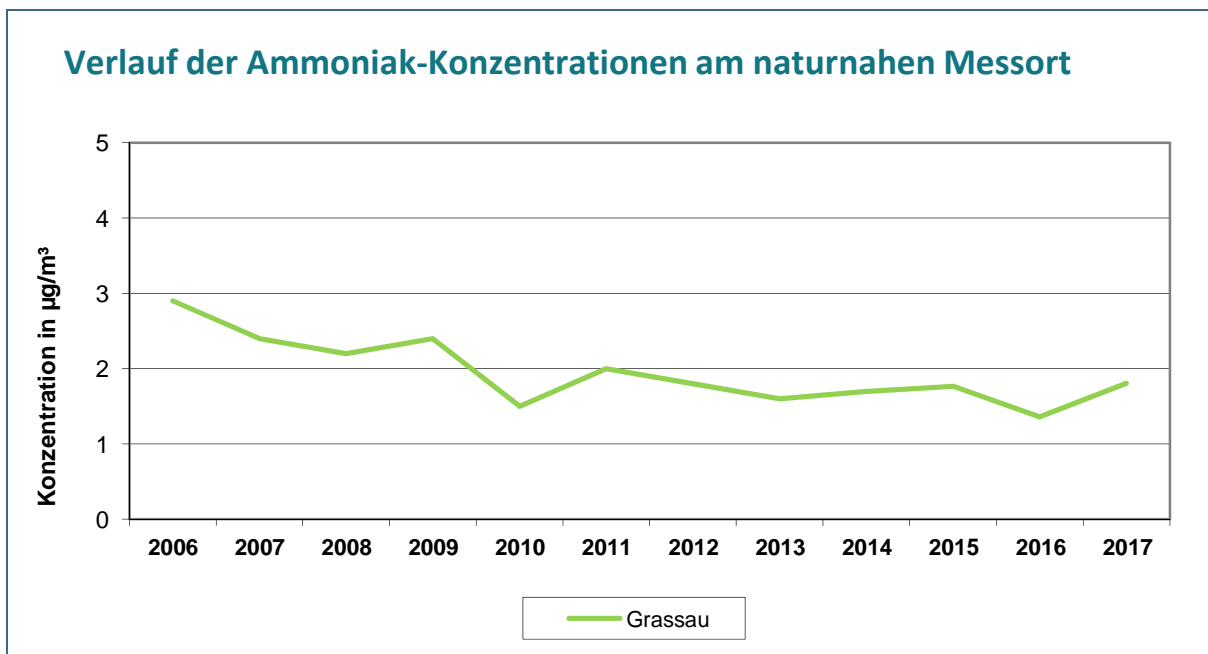
Abb. 8: Verlauf der Ammoniak-Konzentrationen am naturnahen Messort Grassau über den gesamten Messzeitraum
