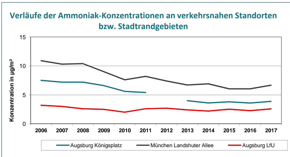
Abb. 10: Verläufe der Ammoniak-Konzentrationen an den verkehrsnahen Messorten in München und Augsburg im Vergleich zu dem Stadtrandgebiet Augsburg über den gesamten Messzeitraum
