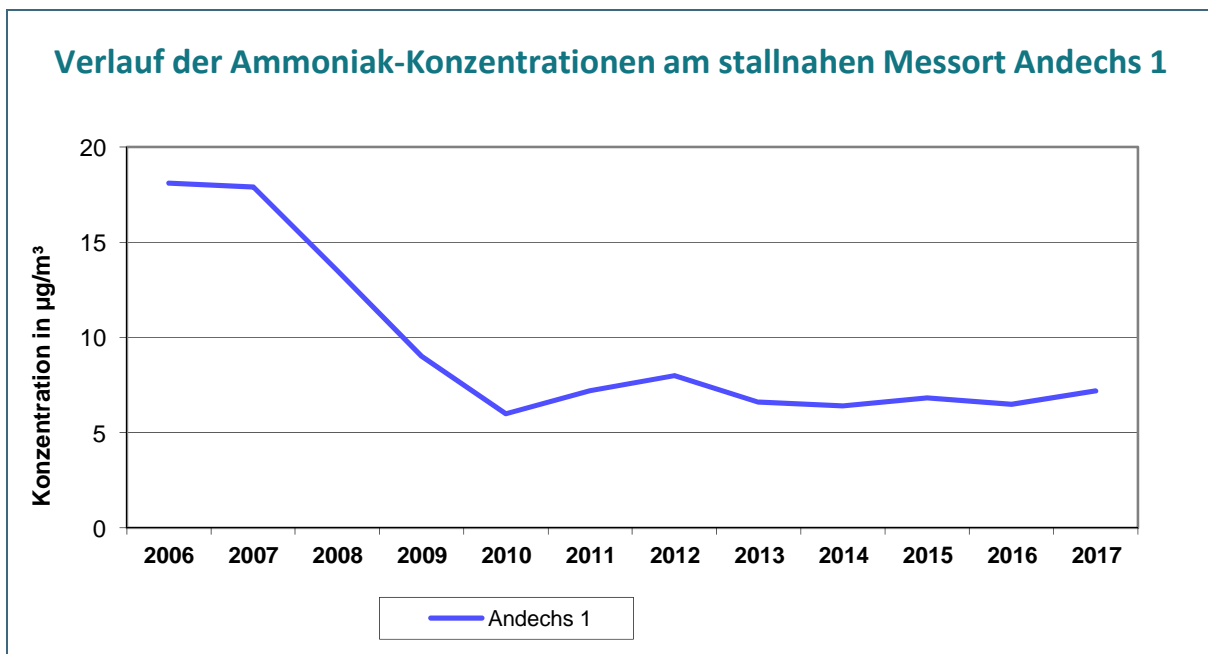
Abb. 2: Verlauf der Ammoniak-Konzentrationen am stallnahen Messort Andechs 1 über den gesamten Messzeitraum
