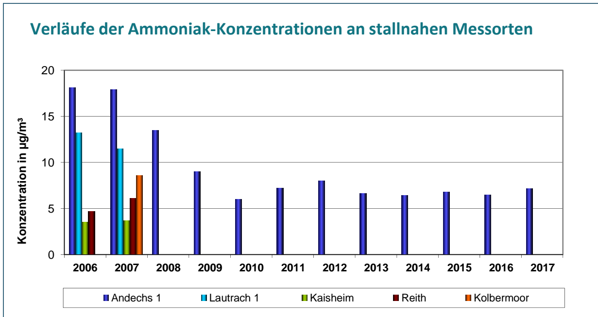
Abb. 1: Auswertung bis 2017 – stallnahe Messorte
