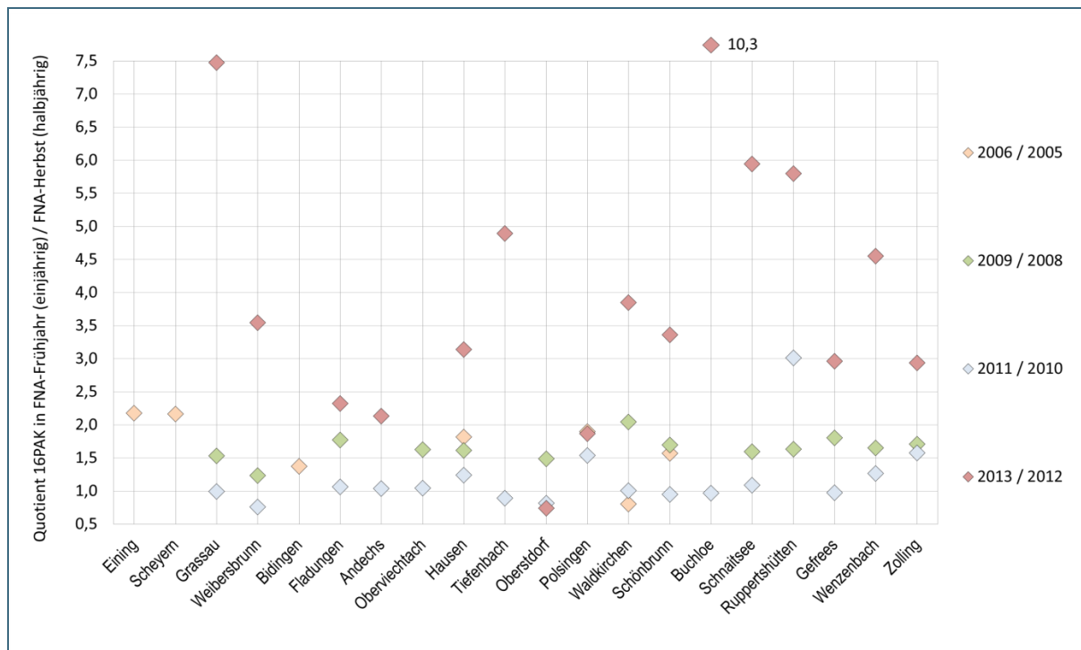
Abb. 18: Quotienten der 16PAK in Fichtennadeln im Frühjahr und Vorjahres-Herbst – Messpunktvergleich
