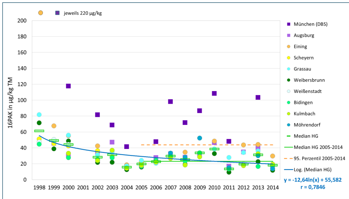
Abb. 9: 16PAK in Graskulturen im Mai bis Juli 1998 bis 2014 (TM = Trockenmasse)
