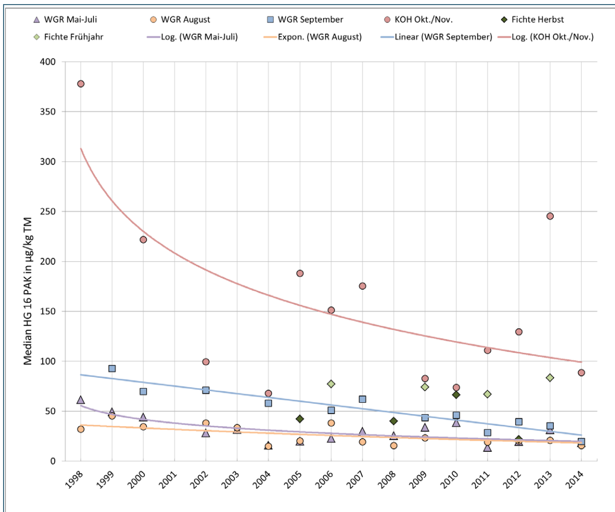
Abb. 19: Jährliche Mediane HG der 16PAK der verschiedenen Bioindikatoren (WGR – Standardisierte Graskultur, KOH – Grünkohl, Fichtennadeln) und Untersuchungsintervalle mit signifikanten Trendfunktionen
