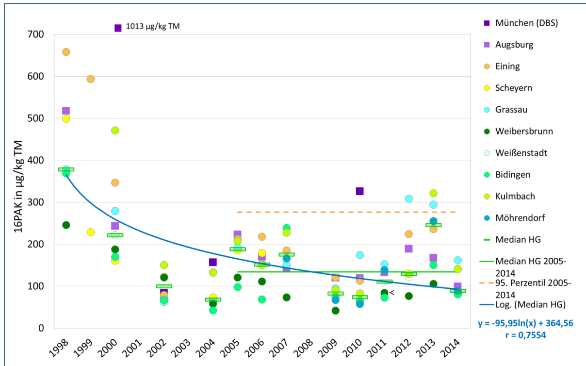
Abb. 15: 16PAK in Grünkohl im Oktober bis November 1998 bis 2014
