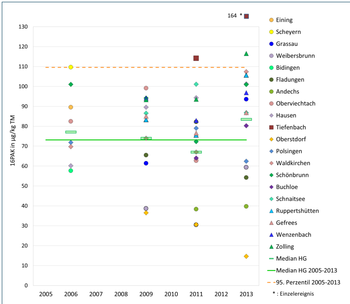
Abb. 17: 16PAK in Fichtennadeln von einjährigen Trieben vom Frühjahr 2006 bis 2013 (Dreiecke: siedlungsnah Lage)
