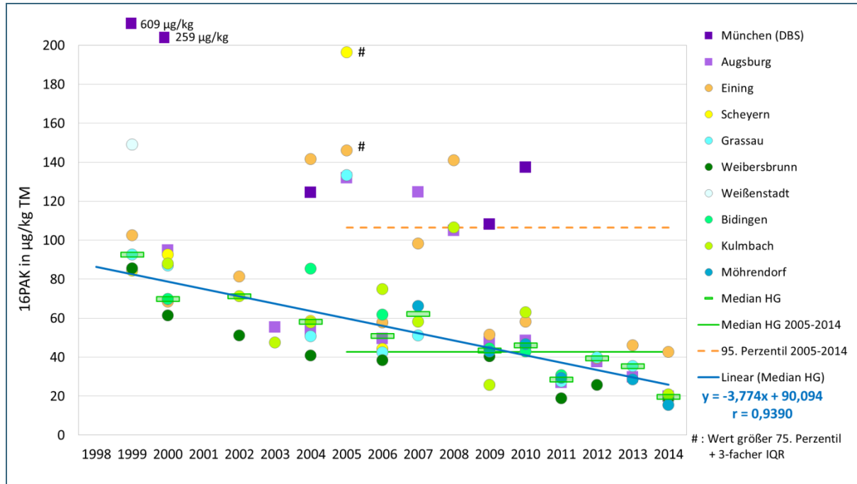
Abb. 11: 16PAK in Graskulturen im September 1998 bis 2014 (TM = Trockenmasse)
