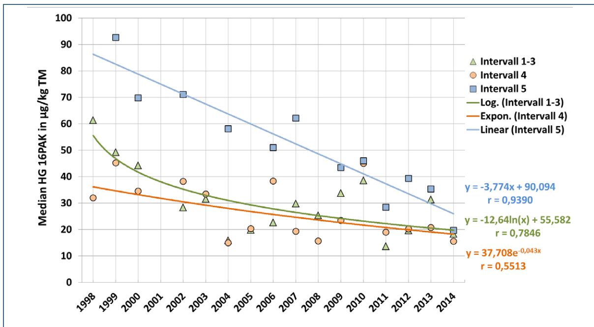
Abb. 14: Vergleich der 16PAK Graskultur-Intervalle anhand der Mediane HG und Trendfunktionen
