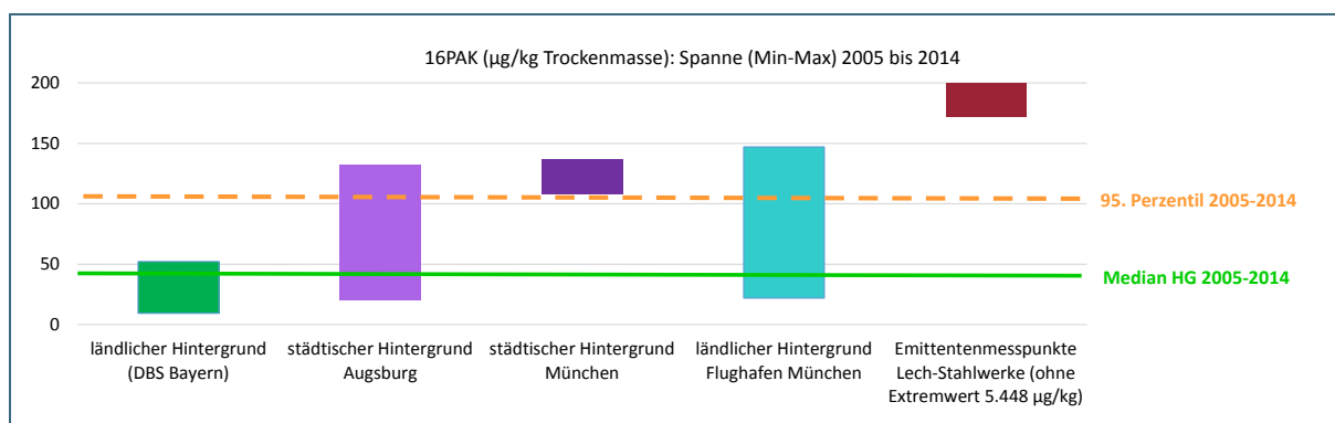
Abb. 21: Spanne (Minimum–Maximum) der 16PAK in Graskulturen vom September 2005 bis 2014 (in µg/kg Trockenmasse) (Quellen: TÜV 2014 UND 2015 für Flughafen München, LFU 2009 für Lech-Stahlwerke)
