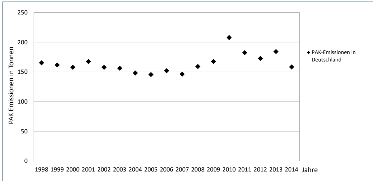
Abb. 20: PAK-Emissionsdaten für Deutschland 1998 bis 2014 (Quelle UBA 2016a)
