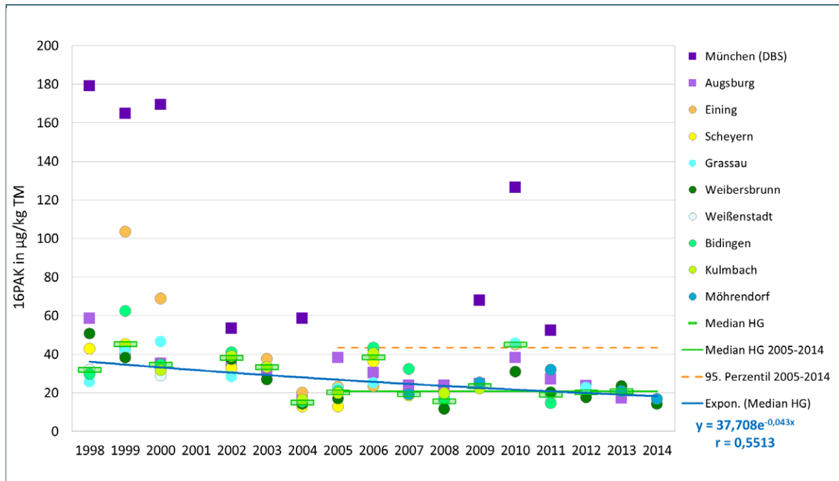
Abb. 10: 16PAK in Graskulturen im August 1998 bis 2014 (TM = Trockenmasse)
