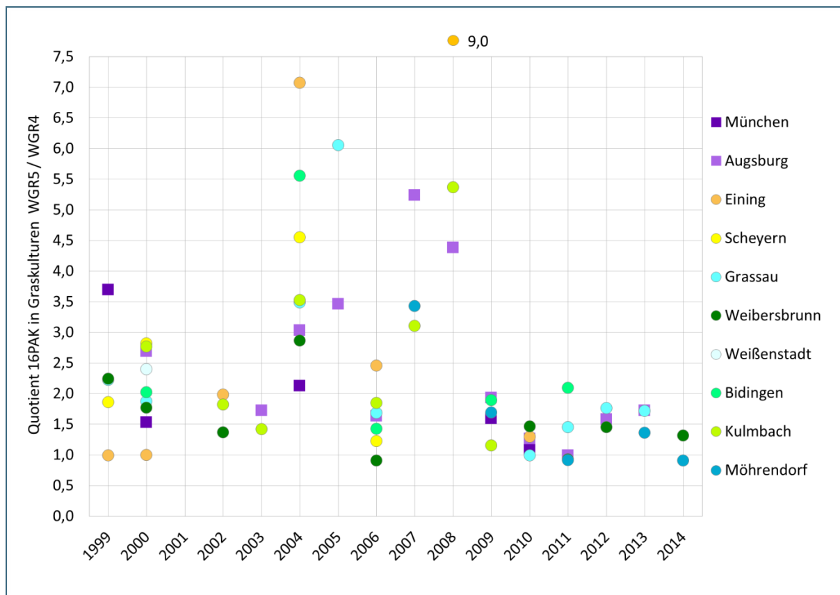
Abb. 12: Quotienten der 16PAK in Graskulturen vom September und August 1999 bis 2014 (WGR5/WGR4)
