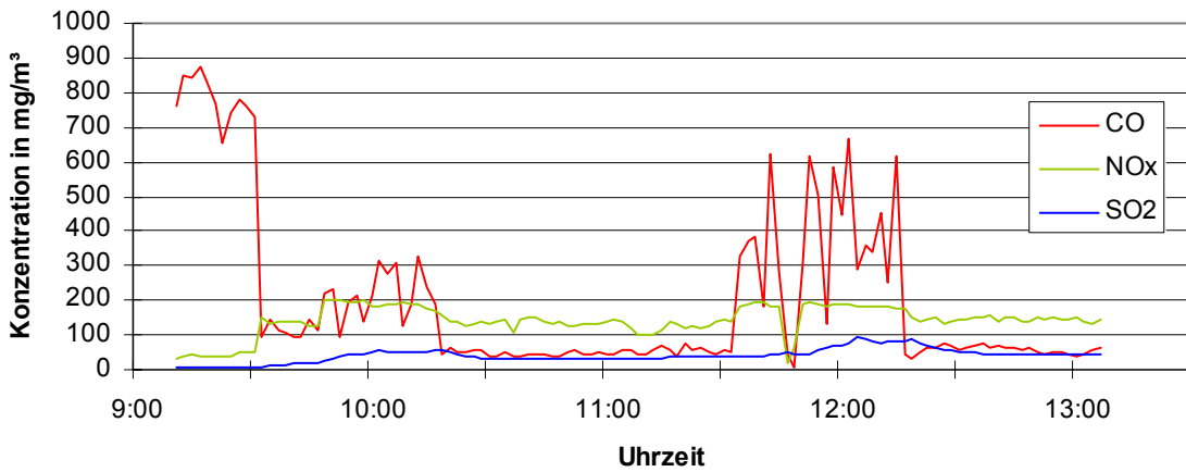
Emissionmessungen bei Einsatz von Getreide (Heizomat-Anlage) Messreihe 2 am 08.04.2003 - Brennstoff: 100 % Holzpellets
