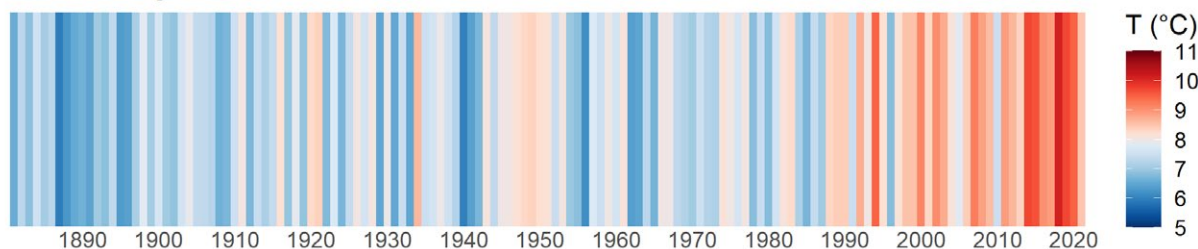
Abb. 1: Warming Stripes 1881–2021 für Niederbayern (Ein Jahr ist je nach mittlerer Temperatur mit einem farbigen Strich – von dunkelblau (kalt) über hellblau und hellrot bis dunkelrot (warm) – abgebildet.)
