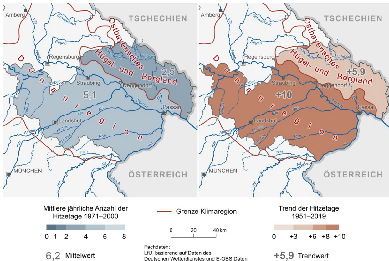
Abb. 4: Jährliche Anzahl der Hitzetage 1971–2000 (links) und Änderung der Hitzetage 1951–2019 (rechts) in Niederbayern
