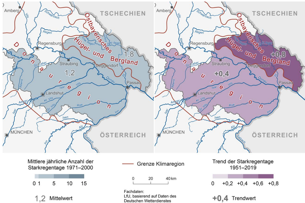
Abb. 3: Jährliche Anzahl der Starkregentage 1971–2000 (links) und Änderung der Starkregentage 1951–2019 (rechts) in Niederbayern
