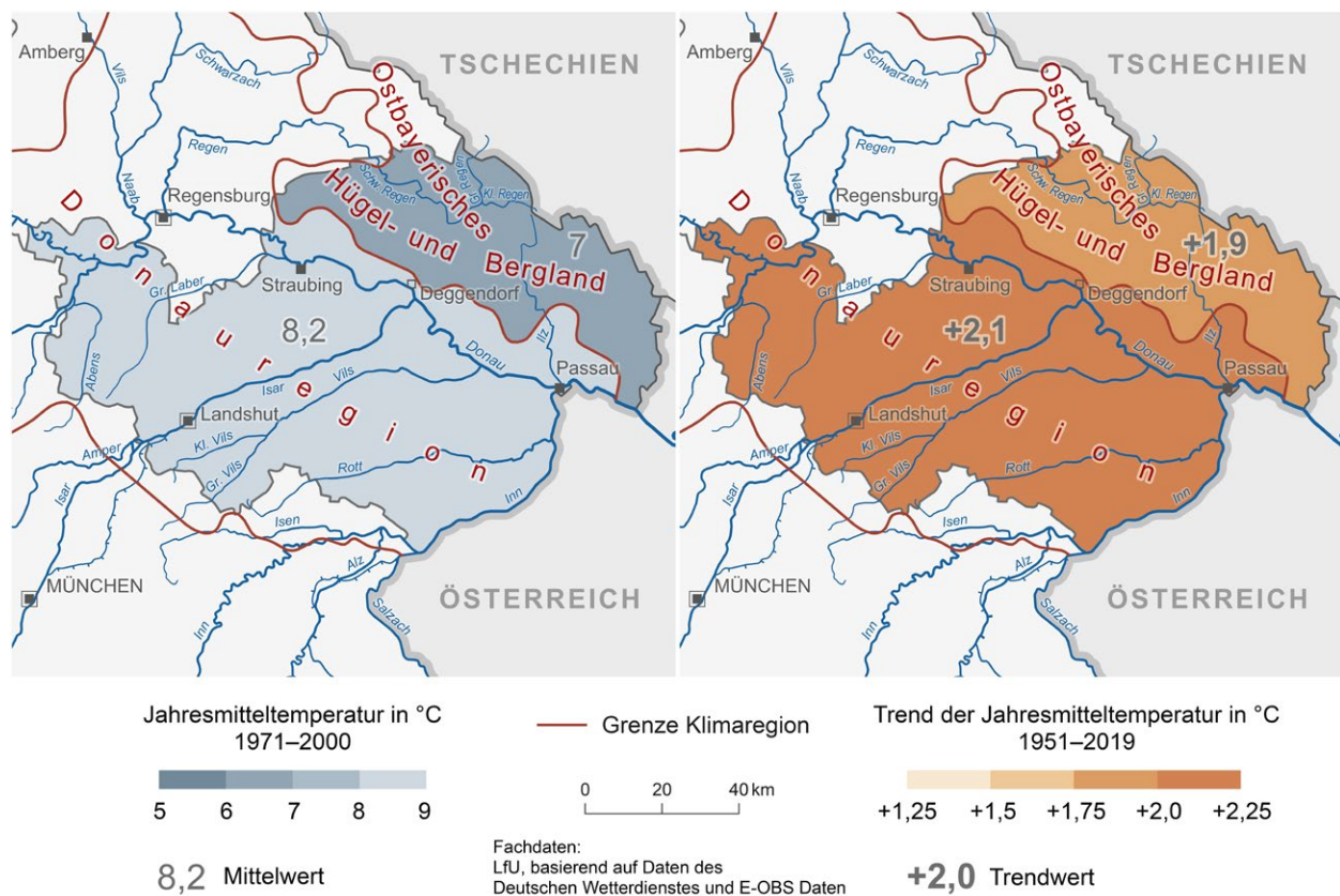
Abb. 2: Mittlere Lufttemperatur 1971–2000 (links) und Änderung der Temperatur 1951–2019 (rechts) in Niederbayern
