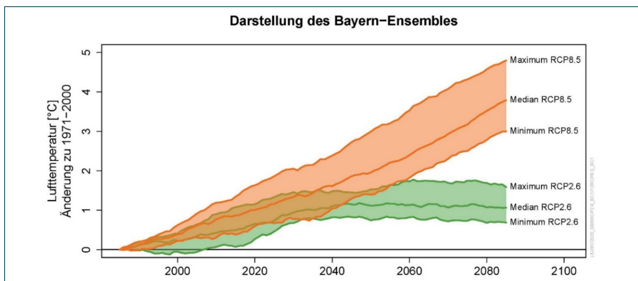
Abb. 12: Ergebnisse des Bayern-Ensembles am Beispiel der Lufttemperatur in Bayern.
