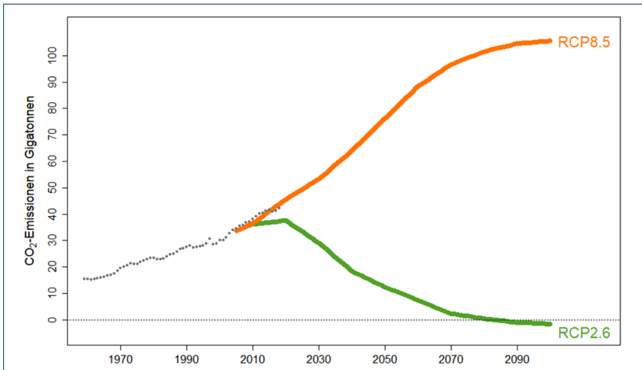
Abb. 10: Die Entwicklung der CO 2 -Emissionen (Kohlenstoffdioxid) in der Vergangenheit und unter den beiden Emissionsszenarien RCP2.6 (mit Klimaschutz) und RCP8.5 (ohne Klimaschutz). Die Abbildung basiert auf Daten des Global Carbon Budget 2019 [5] und des Weltklimarates IPCC [3].
