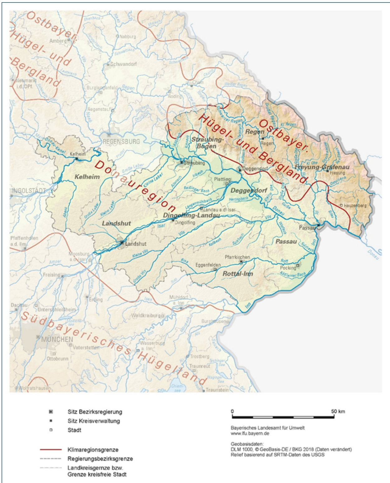
Abb. 5: Der Regierungsbezirk Niederbayern erstreckt sich über zwei unterschiedliche Klimaregionen: Donauregion und Ostbayerisches Hügelland- und Bergland.
