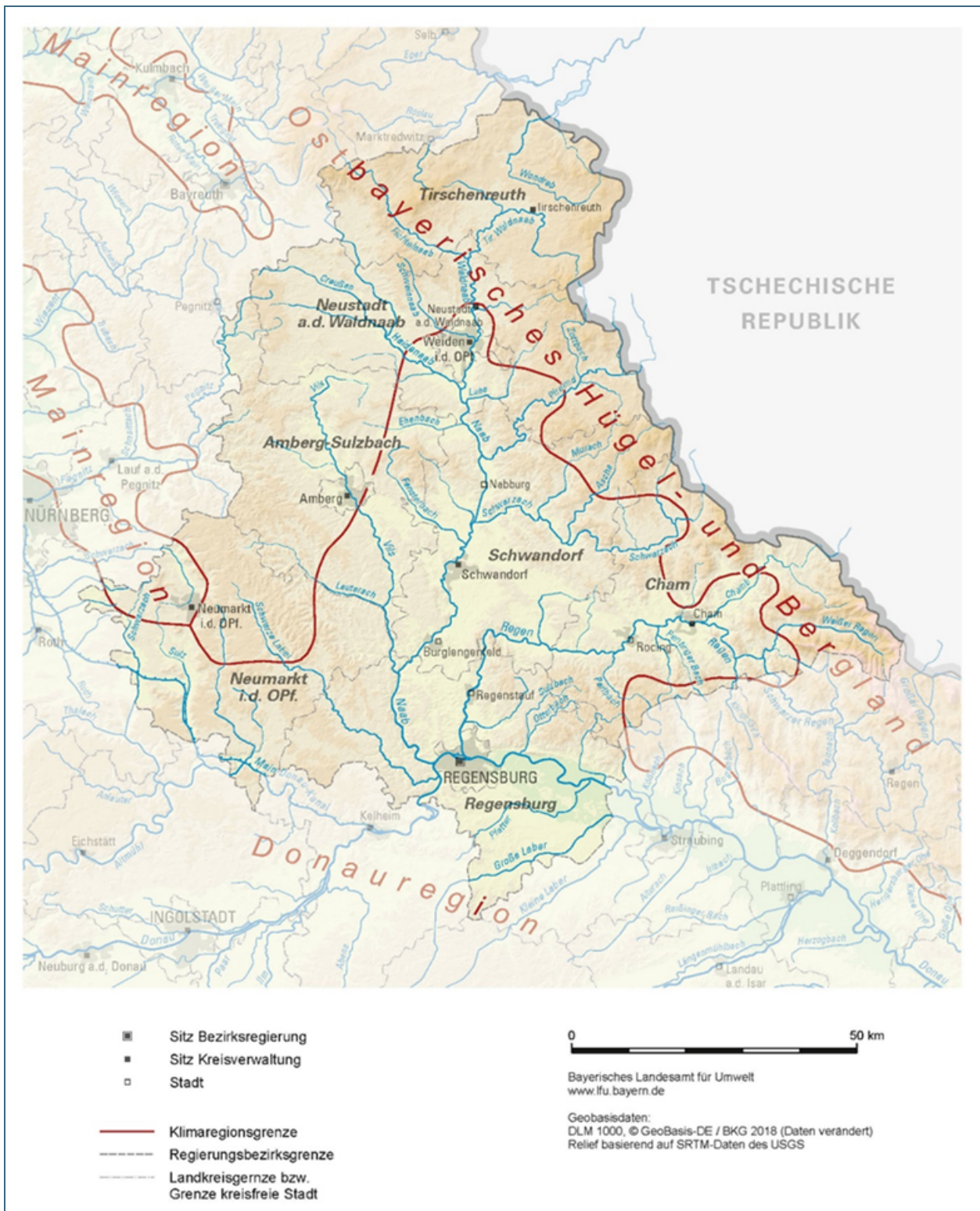
Abb. 6: Der Regierungsbezirk Oberpfalz erstreckt sich über drei unterschiedliche Klimaregionen: Donauregion, Mainregion und Ostbayerisches Hügelland und Bergland.
