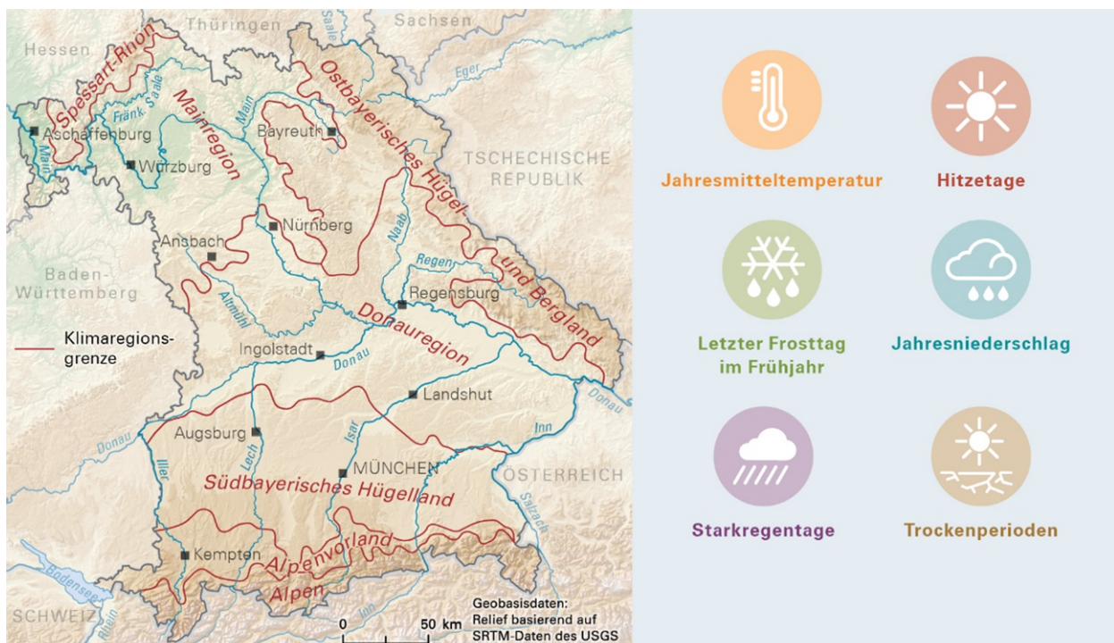
Abb. 9: Icons: Beispiele für klimatische Kennwerte, die in den Klima-Faktenblättern ausgewertet sind. Bayernkarte: Aufteilung in die Klimaregionen.
