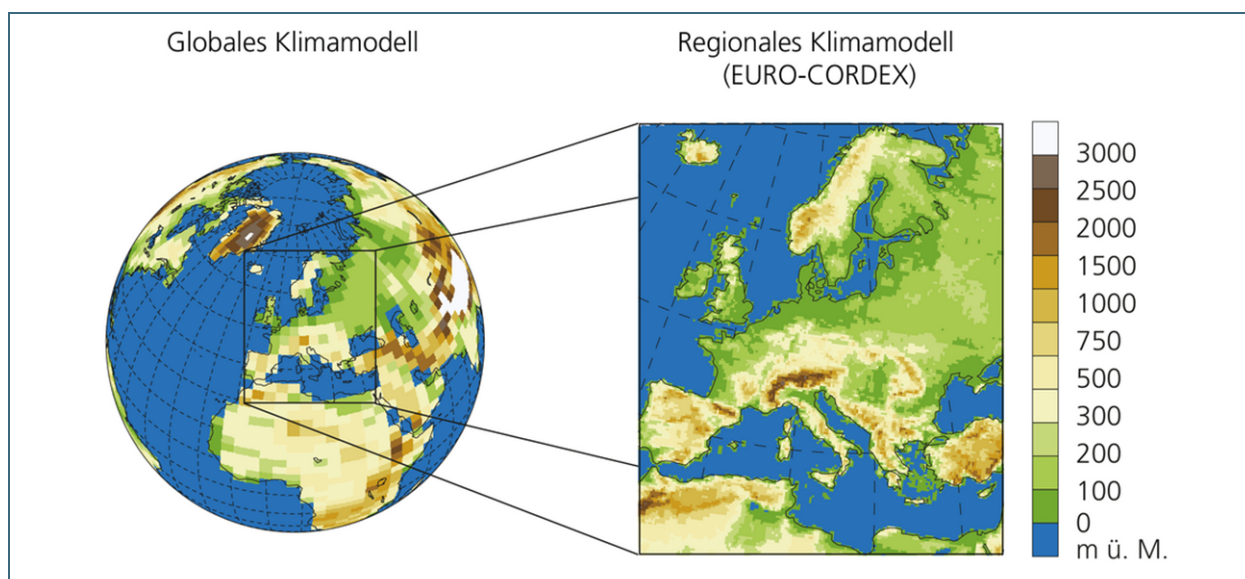
Abb. 11: Abbildung der Topographie bei verschiedenen räumlichen Auflösungen. Globale Klimamodelle haben meist eine Auflösung von mehr als 100 km x 100 km. Die regionalen Klimamodelle, welche für die Klima-Faktenblätter verwendet werden, haben eine Auflösung von 12,5 km x 12,5 km [8].
