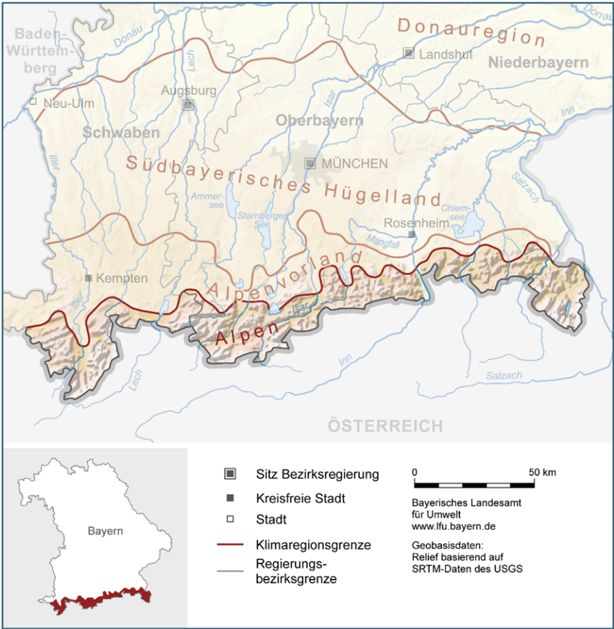
Abb. 5: Klimaregion Alpen
