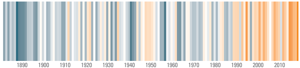
Das Farbband zeigt, wie sich die Durchschnittstemperatur in der Klimaregion Südbayerisches Hügelland von 1881 bis 2019 entwickelt hat. Jeder Streifen im Band steht für ein Jahr. Die Spanne reicht von 6,1 °C (dunkelblau) bis 10,1 °C (orange).
