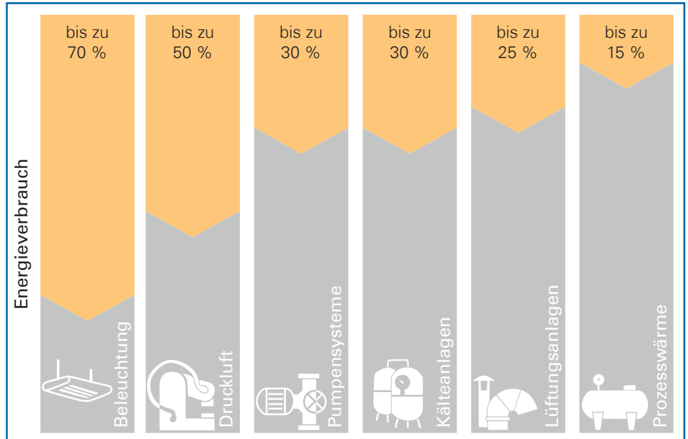
Typische Einsparpotenziale für branchenübergreifende Querschnittstechniken
