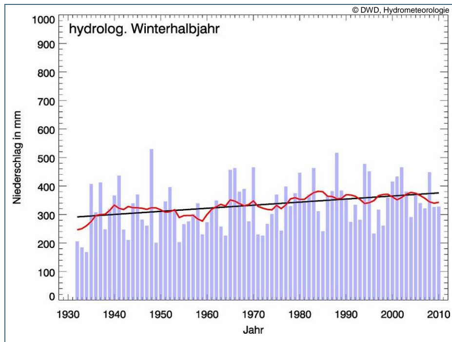
Abb. 3: Verlauf des mittleren Gebietsniederschlags im Flussgebiet Regnitz (blau), gleitender zehnjähriger Mittelwert (rot) und linearer Trend (schwarz) für das hydrologische Winter- halbjahr, Zeitreihe 1931–2010
