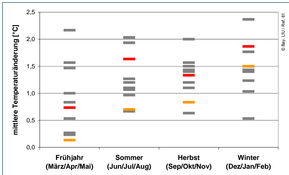
Abb. 6: Jahreszeitliche Spannweite der Änderung der durch- schnittlichen Tempera- tur von zehn regionalen Klimaprojektionen in [°C] für die Region Regnitz, Vergleich der Zeiträume 2021–2050 und 1971–2000; WETTREG2006 (in orange) und WETTREG2010 (in rot) sind hervorgehoben.
