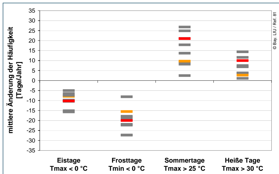
Abb. 8: Spannweite der mittleren Veränderung der Häufigkeit der Kenntage pro Jahr für die Region Regnitz; Vergleich der Zeiträume 2021–2050 und 1971–2000; Auswertung von zehn regionalen Klimaprojektionen (in grau); WETTREG2006 (in orange) und WETTREG2010 (in rot) sind hervorgehoben.
