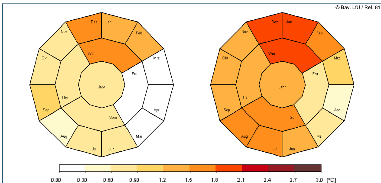
Abb. 7: Veränderung der Mitteltemperaturen 2021–2050 gegenüber 1971–2000 in [°C] bei WETTREG2006 (links) und WETTREG2010 (rechts) für die Region Regnitz. Darstellung der jährlichen (innerer Ring), der jahreszeitlichen (mittlerer Ring) und der monatlichen Änderungen (äußerer Ring).
