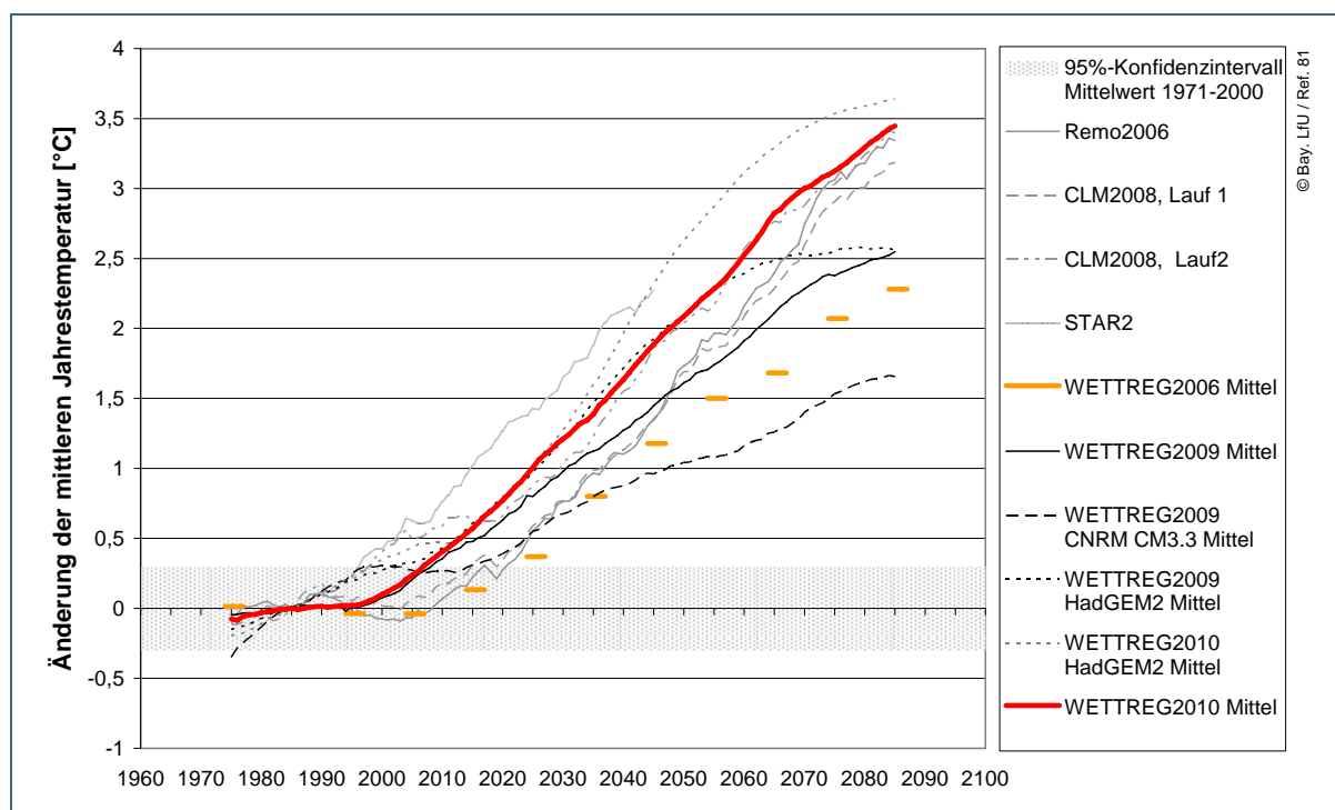
Abb. 5: Änderung des 30-jährigen, gleitenden Mittelwerts der Jahrestemperatur gegenüber dem Kontrollzeitraum 1971–2000 in [°C] für die Region Regnitz. Der Vertrauensbereich des Mittelwerts 1971–2000 ( \pm 0,3 °C, graues Band) berücksichtigt die natürliche Variabilität der Jahreswerte dieses Zeitraums und dient als Hinweis auf die Signifikanz des Änderungssignals. WETTREG2010 (rot, durchgezogene Linie) liegt im oberen, WETTREG2006 (orange, gestrichelt) im unteren Bereich der Bandbreite; für die WETTREG-Projektionen ist der Mittelwert aus zehn Realisationen dargestellt. Wenn nicht anders angegeben, ist ECHAM5 als antreibendes Globalmodell genutzt.
