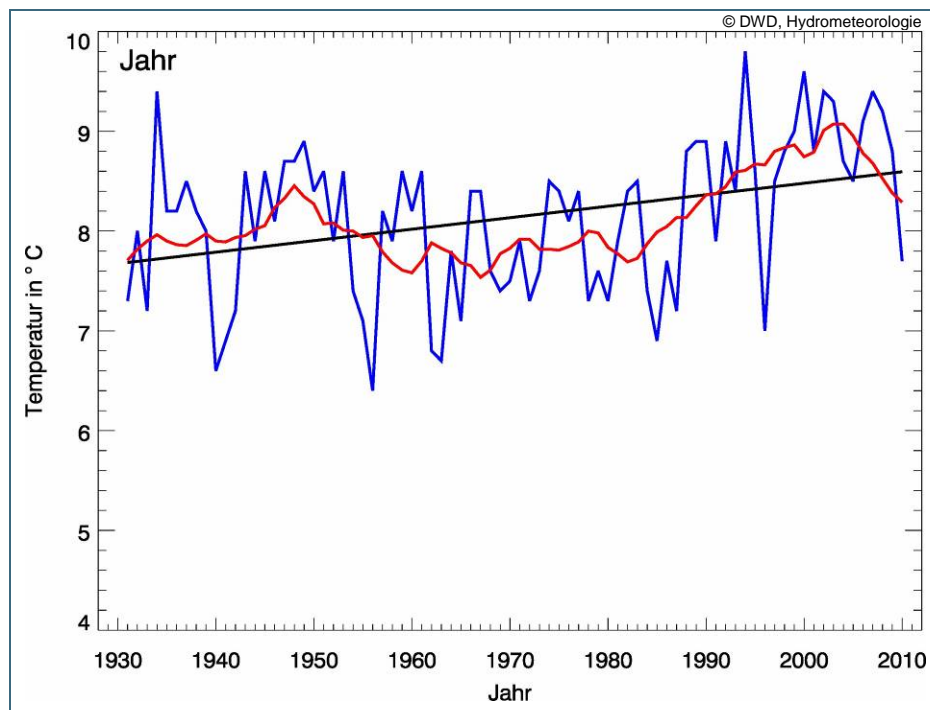
Abb. 2: Verlauf der Jahresmitteltemperatur im Flussgebiet Regnitz (blau); gleitender zehnjähriger Mittelwert (rot) und linearer Trend (schwarz) 1931–2010
