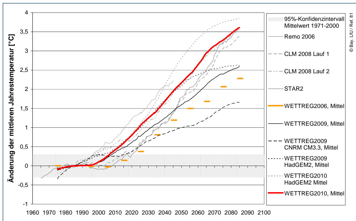
Abb. 5: Änderung des 30-jährigen, gleitenden Mittelwerts der Jahrestemperatur gegenüber dem Kontrollzeitraum 1971–2000 in [°C] für die Region Isar. Der Vertrauensbereich des Mittelwerts 1971–2000 ( \pm 0,3 °C, graues Band) berücksichtigt die natürliche Variabilität der Jahreswerte dieses Zeitraums und dient als Hinweis auf die Signifikanz des Änderungssignals. WETTREG2010 (rot, durchgezogene Linie) liegt im oberen, WETTREG2006 (orange, gestrichelt) im unteren Bereich der Bandbreite; für die WETTREG-Projektionen ist der Mittelwert aus zehn Realisationen dargestellt. Wenn nicht anders angegeben, ist ECHAM5 als antreibendes Globalmodell genutzt.
