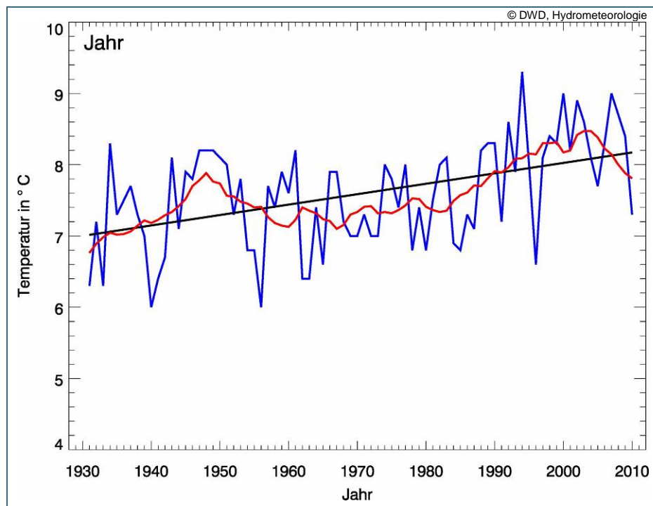
Abb. 2: Verlauf der Jahresmitteltemperatur im Flussgebiet Isar (blau); gleitender zehnjähriger Mittelwert (rot) und linearer Trend (schwarz) 1931–2010
