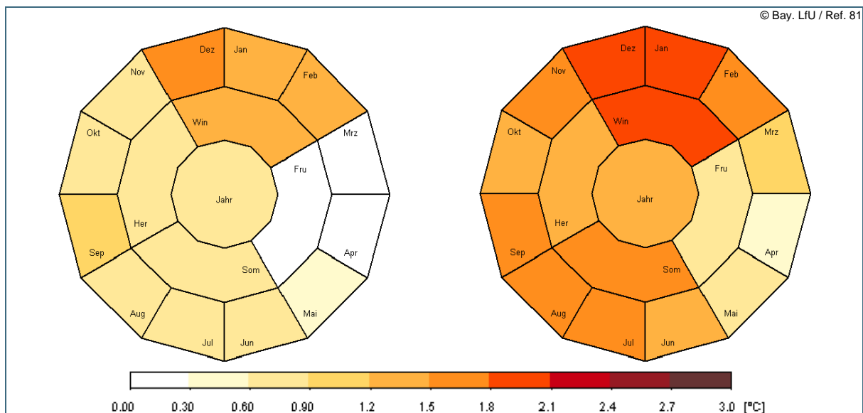
Abb. 7: Veränderung der Mitteltemperaturen 2021–2050 gegenüber 1971–2000 in [°C] bei WETTREG2006 (links) und WETTREG2010 (rechts) für die Region Isar. Darstellung der jährlichen (innerer Ring), der jahreszeitlichen (mittlerer Ring) und der monatlichen Änderungen (äußerer Ring).
