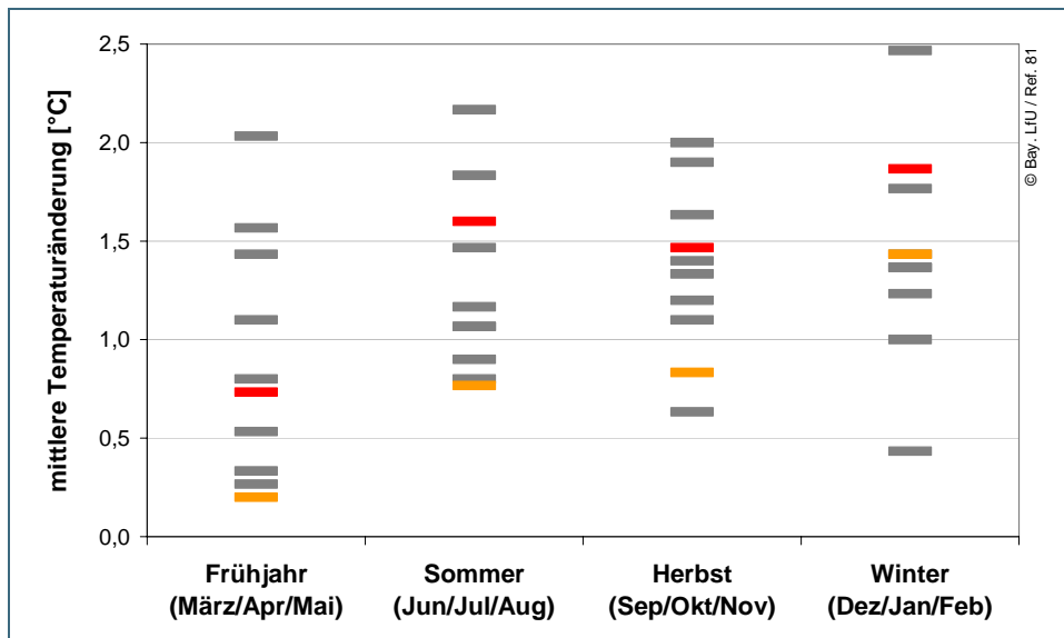
Abb. 6: Jahreszeitliche Spannweite der Änderung der durchschnittlichen Temperatur von zehn regionalen Klimaprojektionen in [°C] für die Region Isar, Vergleich der Zeiträume 2021–2050 und 1971–2000; WETTREG2006 (in orange) und WETTREG2010 (in rot) sind hervorgehoben.
