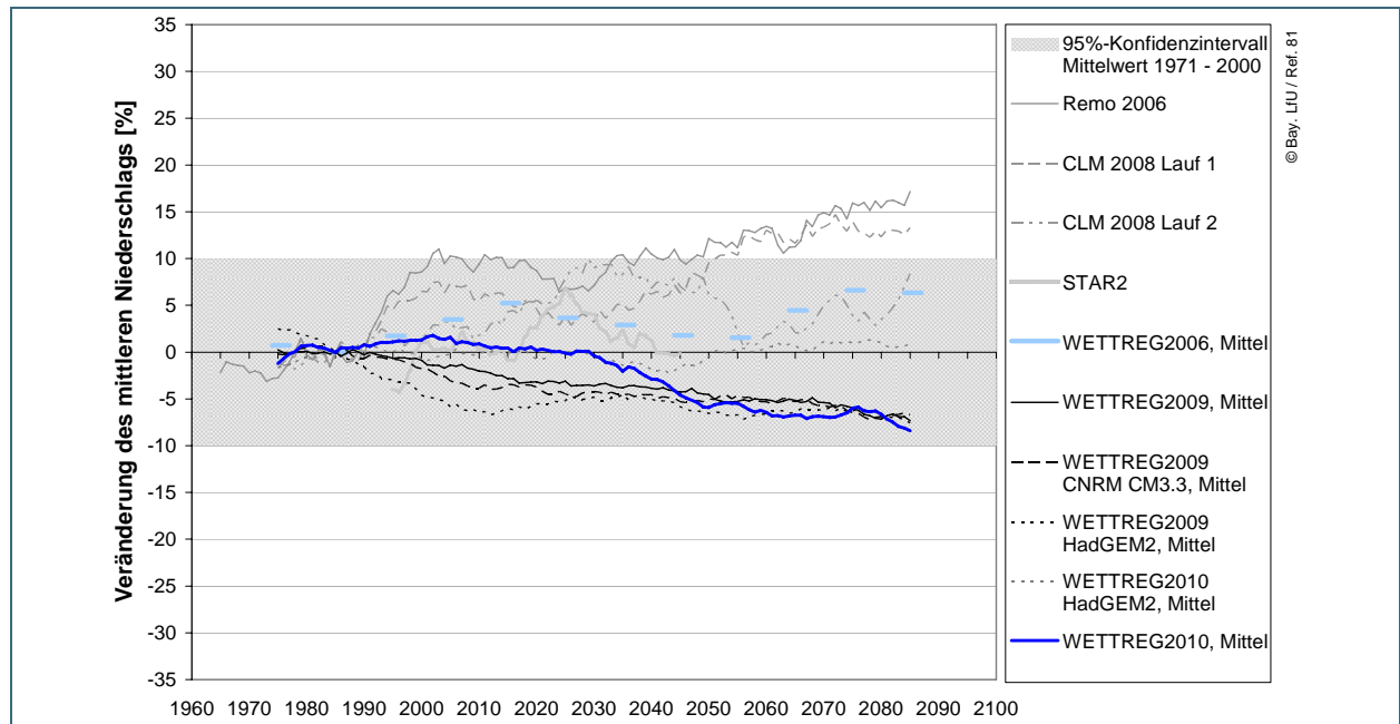
Abb. 9: Relative Änderung des 30-jährigen gleitenden Mittelwerts des Gebietsniederschlags im hydrologischen Winterhalbjahr gegenüber 1971–2000 in [%] für die Region Isar. Der Vertrauensbereich des Mittelwerts 1971–2000 ( \pm 10\% , graues Band) berücksichtigt die natürliche Variabilität der Halbjahreswerte dieses Zeitraums und dient als Hinweis auf die Signifikanz des Änderungssignals. WETTREG2010 (blau) und WETTREG2006 (hellblau) sind hervorgehoben; für die WETTREG-Projektionen ist der Mittelwert aus zehn Realisationen dargestellt. Wenn nicht anders angegeben, ist ECHAM5 als antreibendes GCM genutzt.
