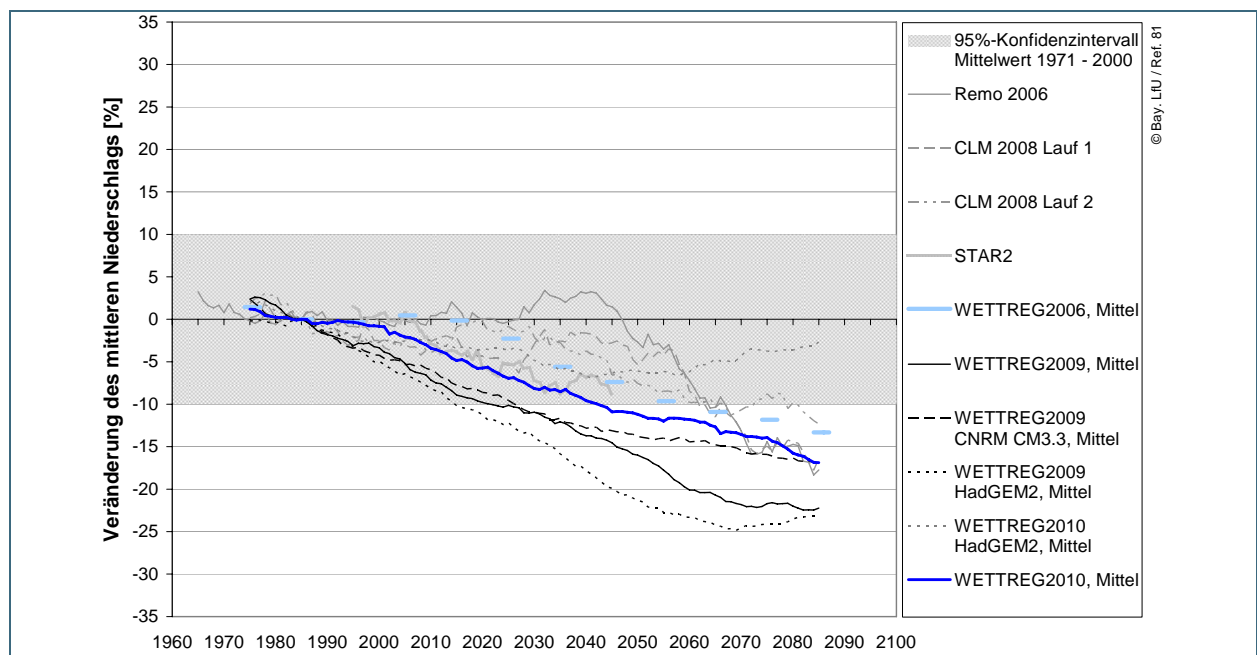
Abb. 10: Wie Abb. 9, für das hydrologische Sommerhalbjahr
