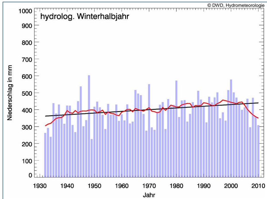
Abb. 3: Verlauf des mittleren Gebietsniederschlags im Flussgebiet Isar (blau), gleitender zehnjähriger Mittelwert (rot) und linearer Trend (schwarz) für das hydrologische Winter- halbjahr, Zeitreihe 1931–2010
