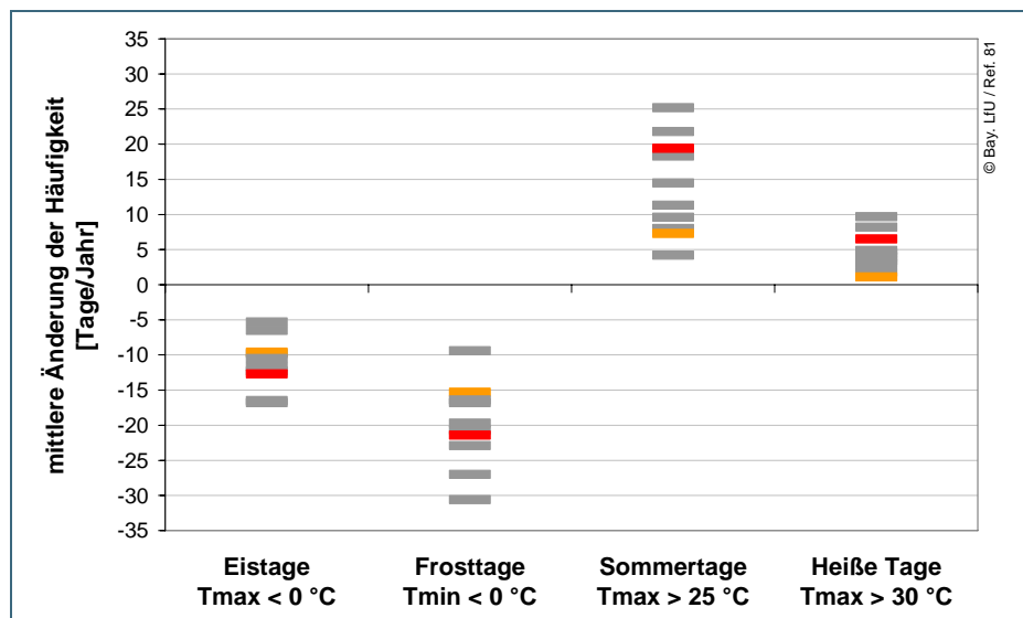
Abb. 8: Spannweite der mittleren Veränderung der Häufigkeit der Kenntage pro Jahr für die Region Isar; Vergleich der Zeiträume 2021–2050 und 1971–2000; Auswertung von zehn regionalen Klimaprojektionen (in grau); WETTREG2006 (in orange) und WETTREG2010 (in rot) sind hervorgehoben.
