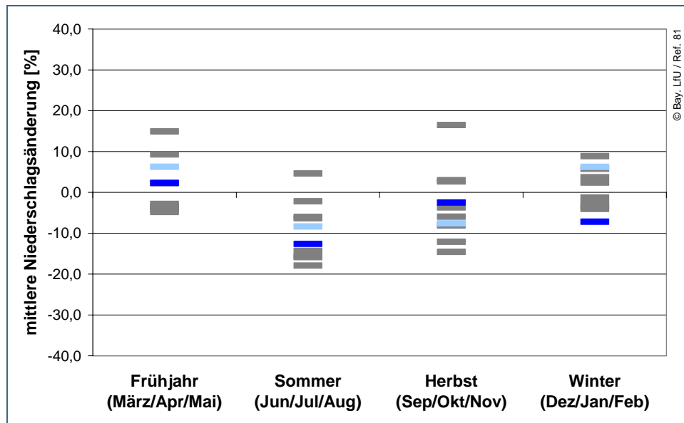
Abb. 11: Jahreszeitliche Spannweite der relativen Änderung des Gebietsniederschlags für die Region Isar in [%]; Vergleich der Zeiträume 2021–2050 und 1971–2000; Auswertung von zehn regionalen Klimaprojektionen (in grau), WETTREG2006 (in hellblau) und WETTREG2010 (in dunkelblau) sind hervorgehoben.
