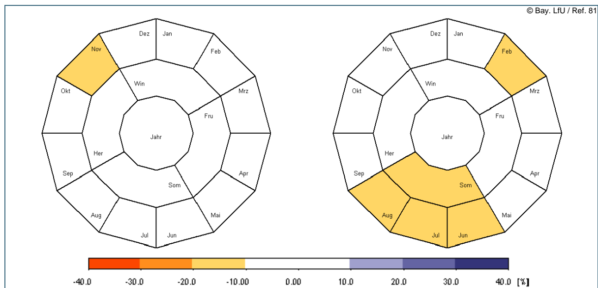
Abb. 12: Relative Veränderung der Gebietsniederschlagssumme für die Region Isar von 2021–2050 gegenüber 1971–2000 in [%] bei WETTREG2006 (links) und WETTREG2010 (rechts). Darstellung der mittleren jährlichen Änderung (innerer Ring), der mittleren jahreszeitlichen Änderung (mittlerer Ring) und der mittleren monatlichen Änderung (äußerer Ring).
