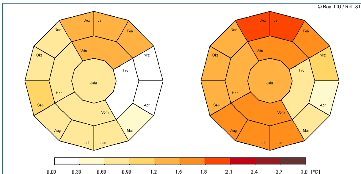
Abb. 7: Veränderung der Mitteltemperaturen 2021–2050 gegenüber 1971–2000 in [°C] bei WETTREG2006 (links) und WETTREG2010 (rechts) für die Region Inn. Darstellung der jährlichen (innerer Ring), der jahreszeitlichen (mittlerer Ring) und der monatlichen Änderungen (äußerer Ring).
