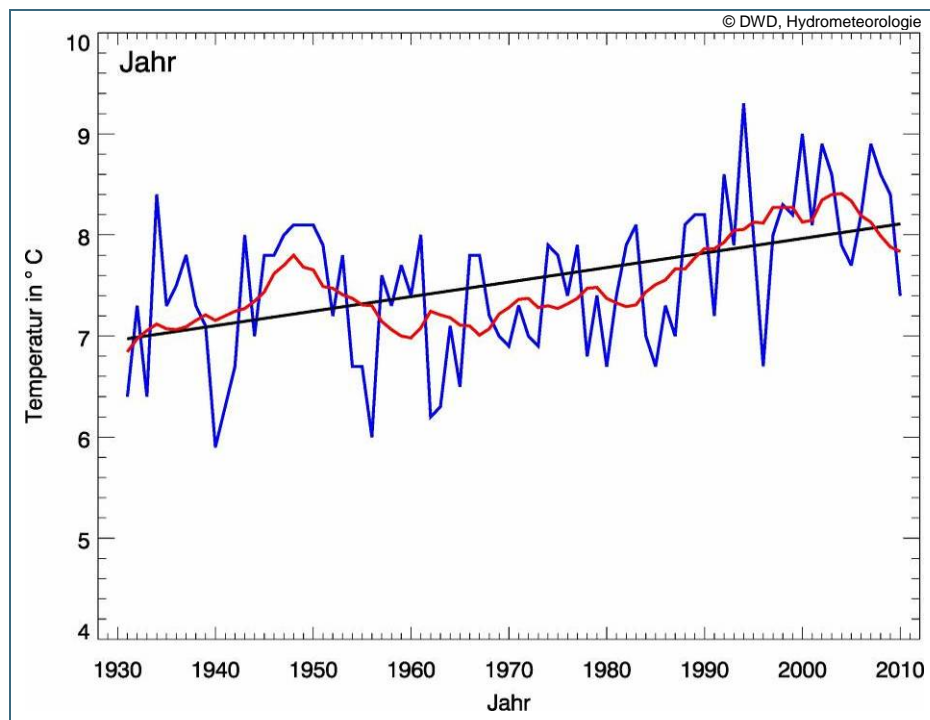
Abb. 2: Verlauf der Jahresmitteltemperatur im Flussgebiet Inn (blau); gleitender zehnjähriger Mittelwert (rot) und linearer Trend (schwarz) 1931–2010
