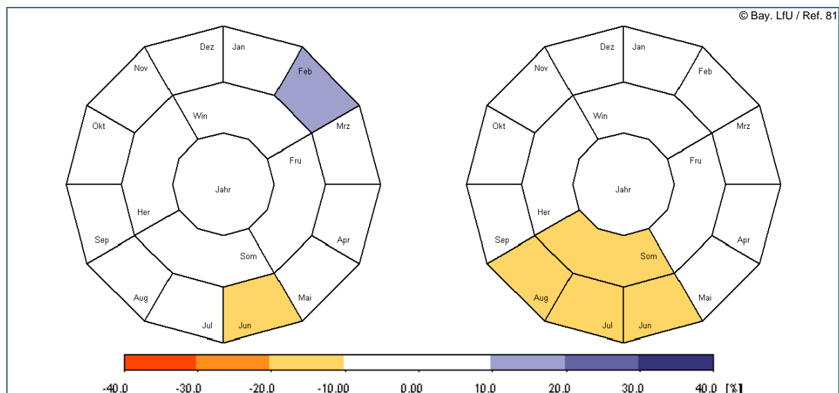
Abb. 12: Relative Veränderung der Gebietsniederschlagssumme für die Region Inn von 2021–2050 gegenüber 1971–2000 in [%] bei WETTREG2006 (links) und WETTREG2010 (rechts). Darstellung der mittleren jährlichen Änderung (innerer Ring), der mittleren jahreszeitlichen Änderung (mittlerer Ring) und der mittleren monatlichen Änderung (äußerer Ring).
