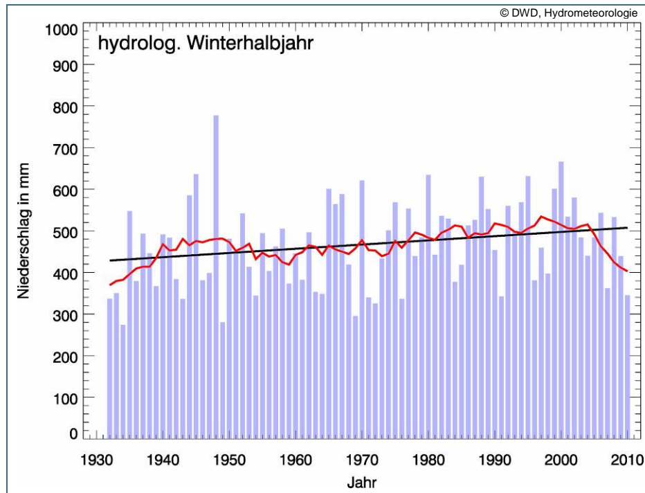
Abb. 3: Verlauf des mittleren Gebietsniederschlags im Flussgebiet Inn (blau), gleitender zehnjähriger Mittelwert (rot) und linearer Trend (schwarz) für das hydrologische Winter- halbjahr, Zeitreihe 1931–2010
