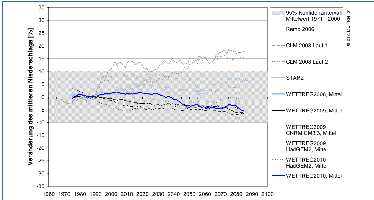
Abb. 9: Relative Änderung des 30-jährigen gleitenden Mittelwerts des Gebietsniederschlags im hydrologischen Winterhalbjahr gegenüber 1971–2000 in [%] für die Region Inn. Der Vertrauensbereich des Mittelwerts 1971–2000 ( \pm 10\% , graues Band) berücksichtigt die natürliche Variabilität der Halbjahreswerte dieses Zeitraums und dient als Hinweis auf die Signifikanz des Änderungssignals. WETTREG2010 (blau) und WETTREG2006 (hellblau) sind hervorgehoben; für die WETTREG-Projektionen ist der Mittelwert aus zehn Realisationen dargestellt. Wenn nicht anders angegeben, ist ECHAM5 als antreibendes GCM genutzt.
