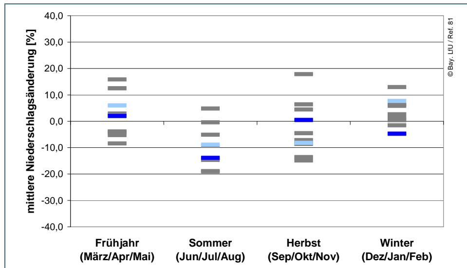
Abb. 11: Jahreszeitliche Spannweite der relativen Änderung des Gebietsniederschlags für die Region Inn in [%]; Vergleich der Zeiträume: 2021–2050 und 1971–2000; Auswertung von zehn regionalen Klimaprojektionen (in grau), WETTREG2006 (in hellblau) und WETTREG2010 (in dunkelblau) sind hervorgehoben.
