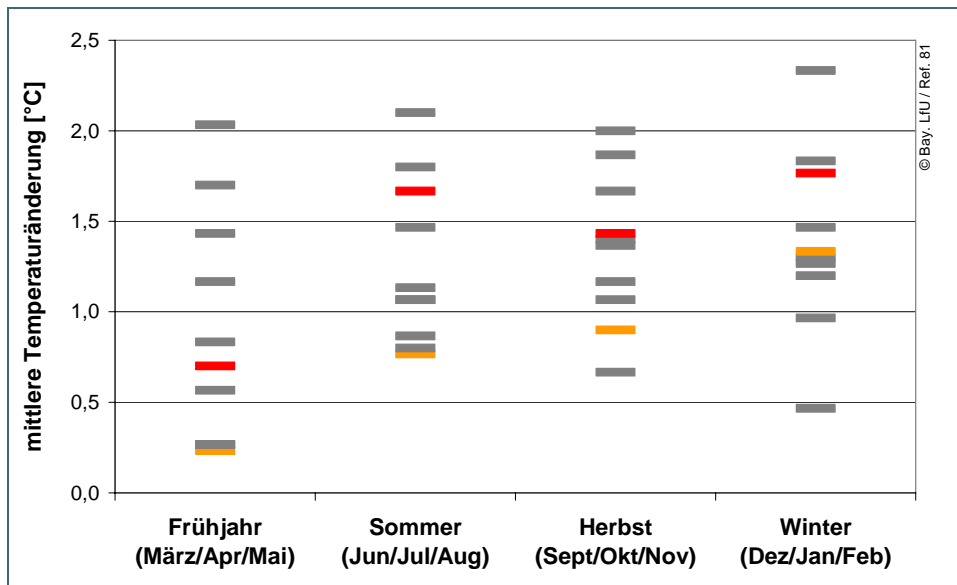
Abb. 6: Jahreszeitliche Spannweite der Änderung der durchschnittlichen Temperatur von zehn regionalen Klimaprojektionen in [°C] für die Region Inn, Vergleich der Zeiträume 2021–2050 und 1971–2000; WETTREG2006 (in orange) und WETTREG2010 (in rot) sind hervorgehoben.
