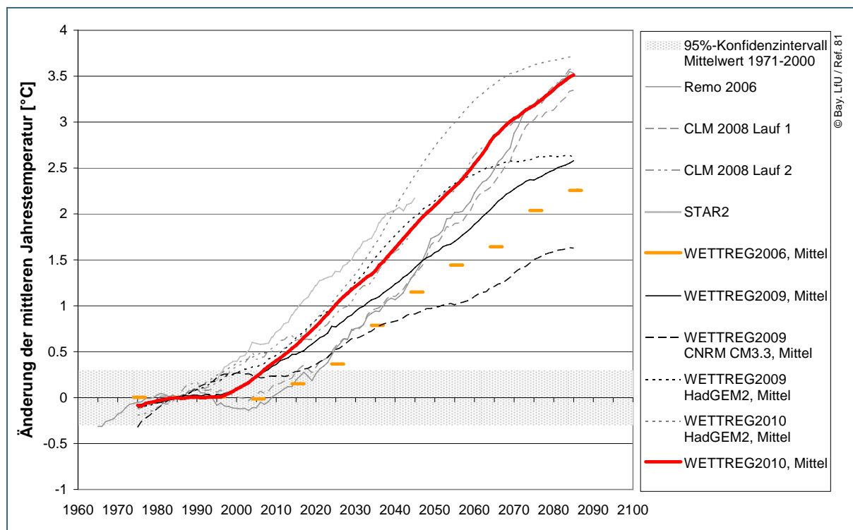
Abb. 5: Änderung des 30-jährigen, gleitenden Mittelwerts der Jahrestemperatur gegenüber dem Kontrollzeitraum 1971–2000 in [°C] für die Region Inn. Der Vertrauensbereich des Mittelwerts 1971–2000 ( \pm 0,3 °C, graues Band) berücksichtigt die natürliche Variabilität der Jahreswerte dieses Zeitraums und dient als Hinweis auf die Signifikanz des Änderungssignals. WETTREG2010 (rot, durchgezogene Linie) liegt im oberen, WETTREG2006 (orange, gestrichelt) im unteren Bereich der Bandbreite; für die WETTREG-Projektionen ist der Mittelwert aus zehn Realisationen dargestellt. Wenn nicht anders angegeben, ist ECHAM5 als antreibendes Globalmodell genutzt.
