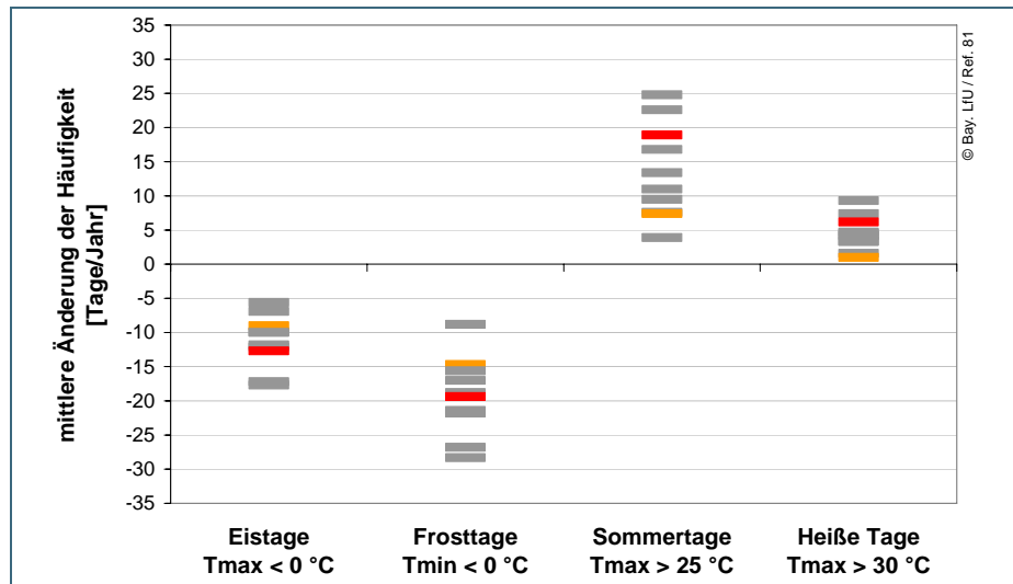
Abb. 8: Spannweite der mittleren Veränderung der Häufigkeit der Kenntage pro Jahr für die Region Inn; Vergleich der Zeiträume 2021–2050 und 1971–2000; Auswertung von zehn regionalen Klimaprojektionen (in grau); WETTREG2006 (in orange) und WETTREG2010 (in rot) sind hervorgehoben.
