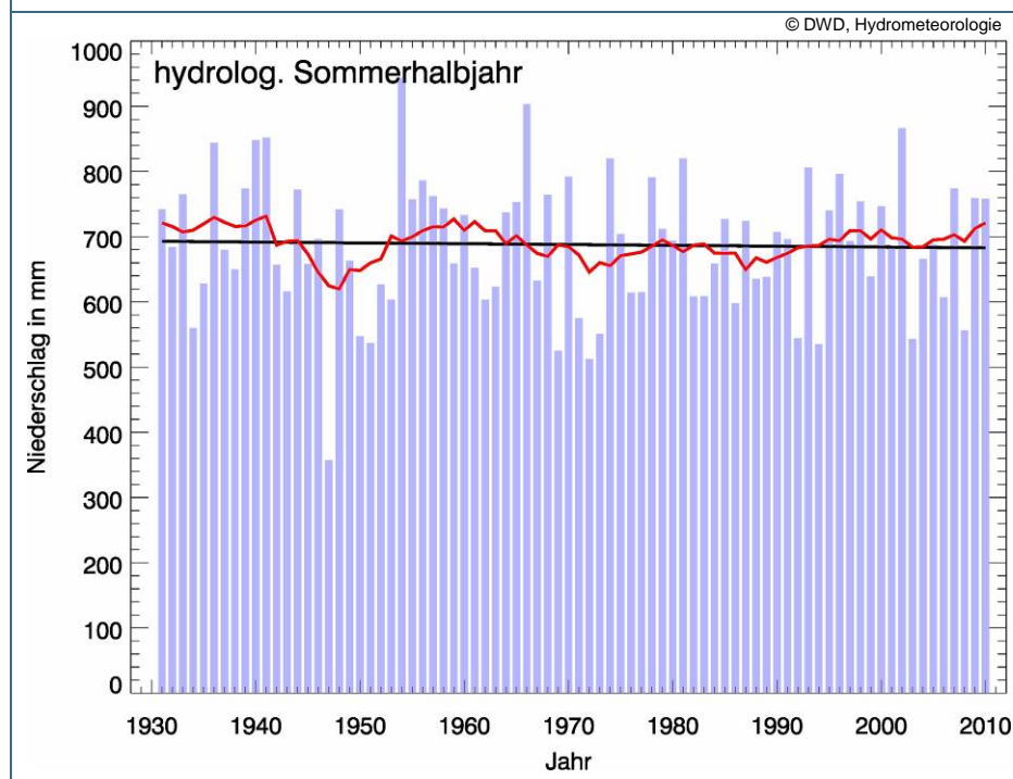
Abb. 4: analog Abb. 3 für das hydrologische Som- merhalbjahr 1931–2010
