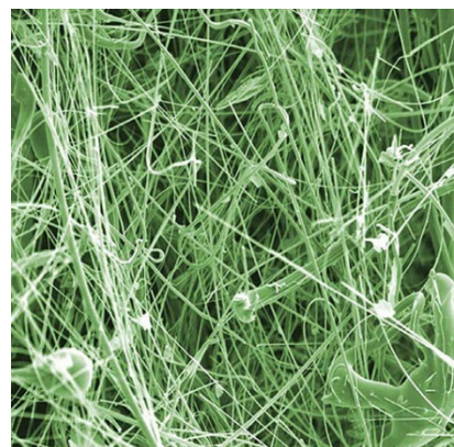
Abb. 4: Keramikfasern, Bildbreite 10 µm
