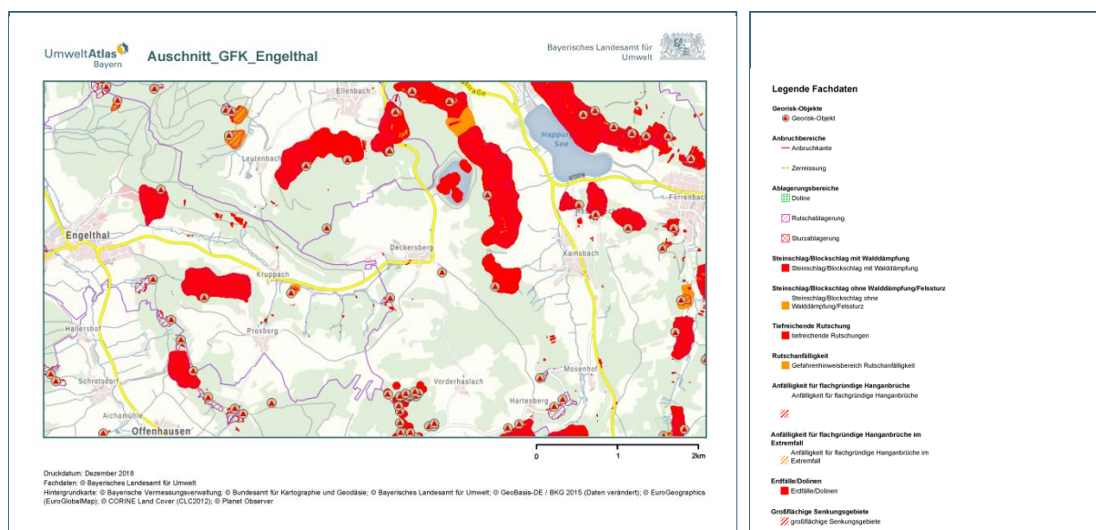
Abb. 1: Beispiel der Darstellung verschiedener geogener Naturgefahren im UmweltAtlas Bayern
