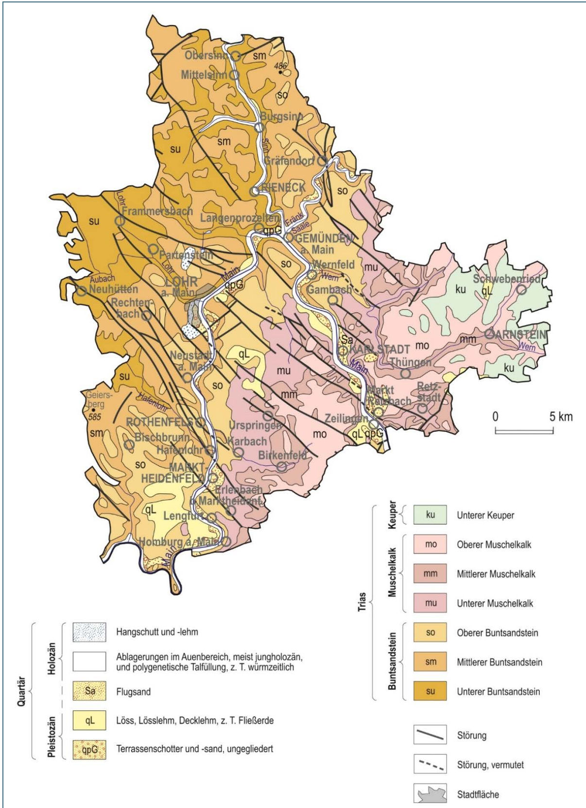
Abb. 8: Geologische Karte Landkreis Main-Spessart (Datengrundlage: Geologische Karte von Bayern 1 : 500 000)
