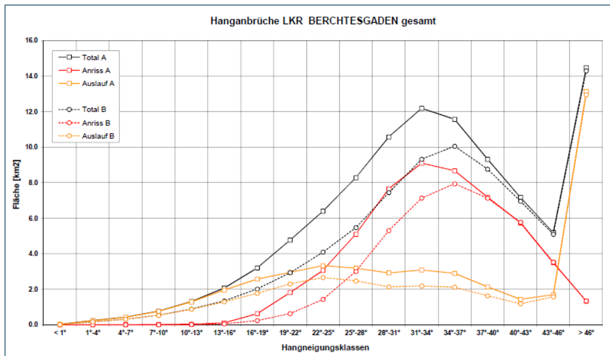
Abb. 4: Statistik der Prozessflächen für Szenarien A und B nach Hangneigungsklassen
