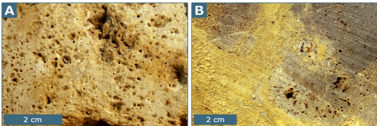
Abb. 44: Detailaufnahme von Gestein der Bohrung AL-9.
