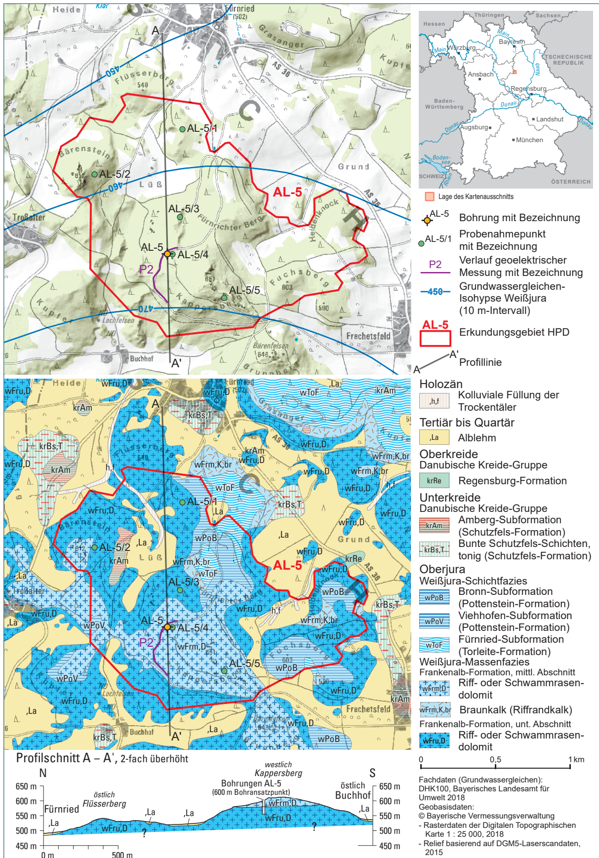
Abb. 69: Lage des Potenzialgebiets AL-5 mit Profilschnitt und Probenlokationen.
