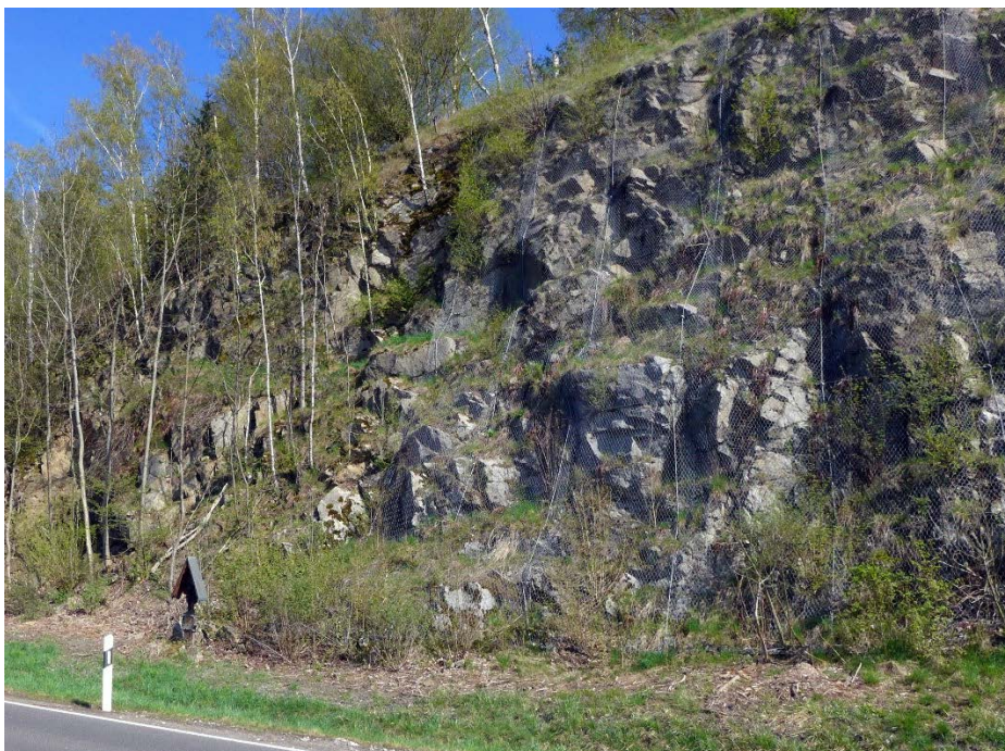
Abb. 11: Straßenböschung mit erfolgter Sicherung
