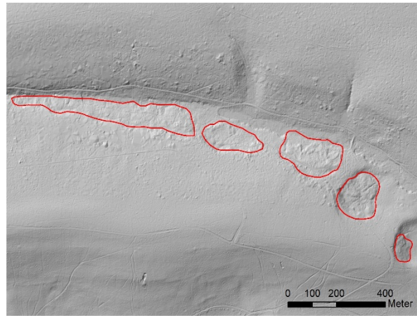
Abb. 5: Mehrere Rutschungsbereiche entlang des Dürrnbachtales im Schattenbild
