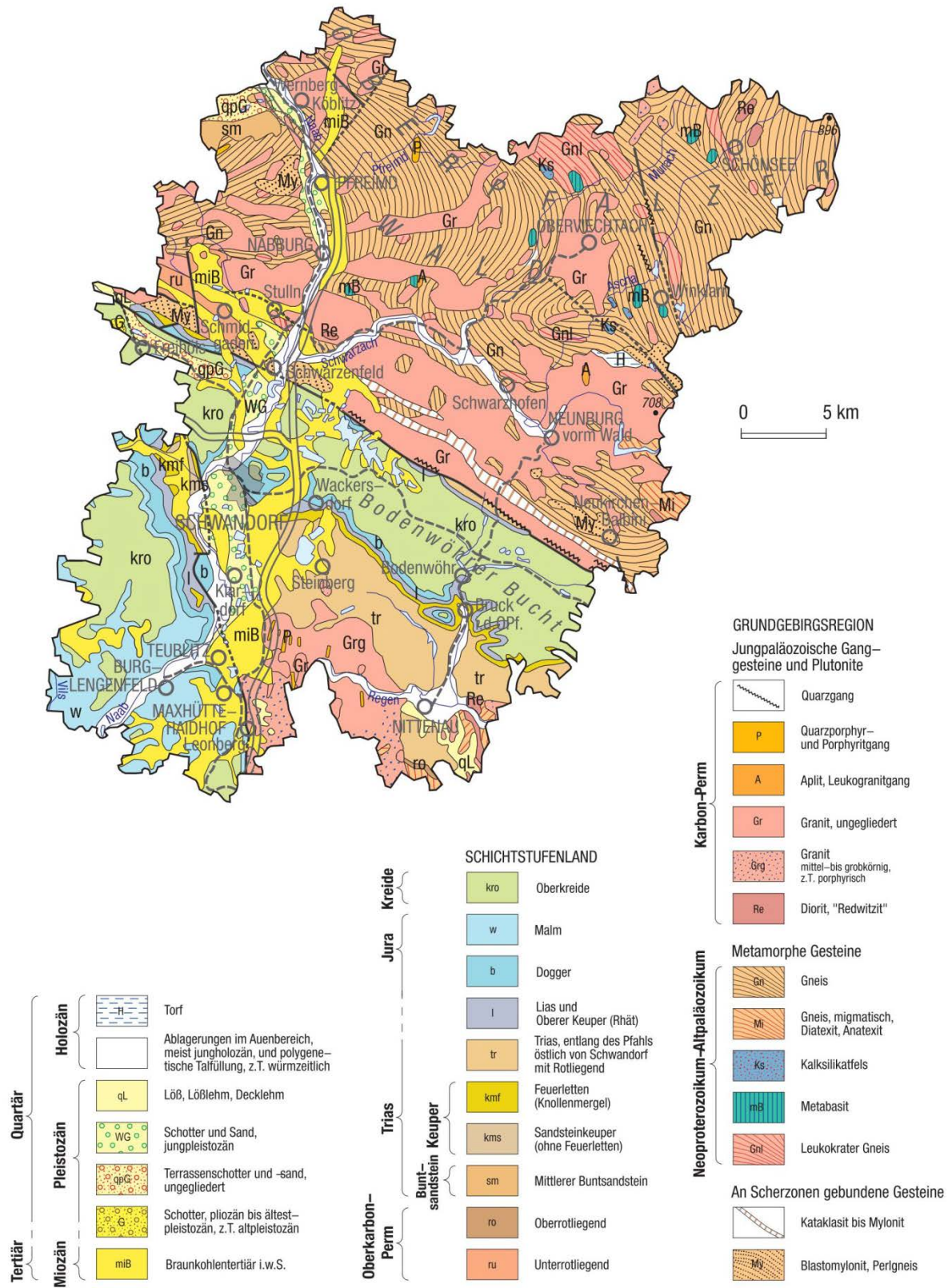
Abb. 8: Geologische Karte Landkreis Schwandorf (Datengrundlage: Geologische Karte von Bayern 1 : 500.000)
