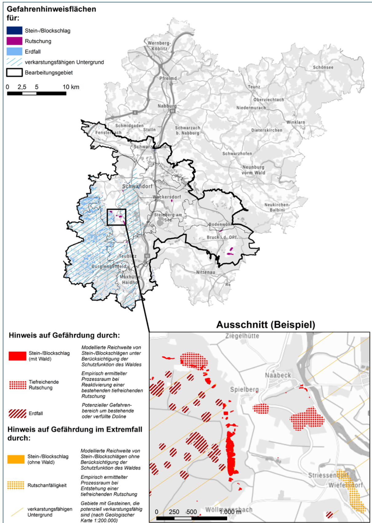
Abb. 9: Verschiedene Kartendarstellungen unterschiedlicher geogener Naturgefahren im Bearbeitungsgebiet des Landkreises Schwandorf
