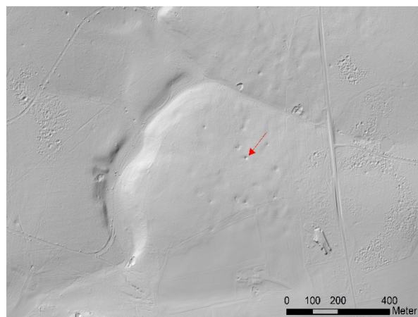
Abb. 7: Schattenbild einer Doline nördlich von Rödlhof. Im Bild sind noch weitere Dolinen erkennbar.
