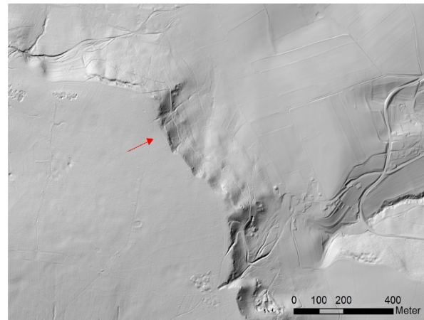
Abb. 3: Steilhänge am Schlottberg bei Spielberg im Schattenbild
