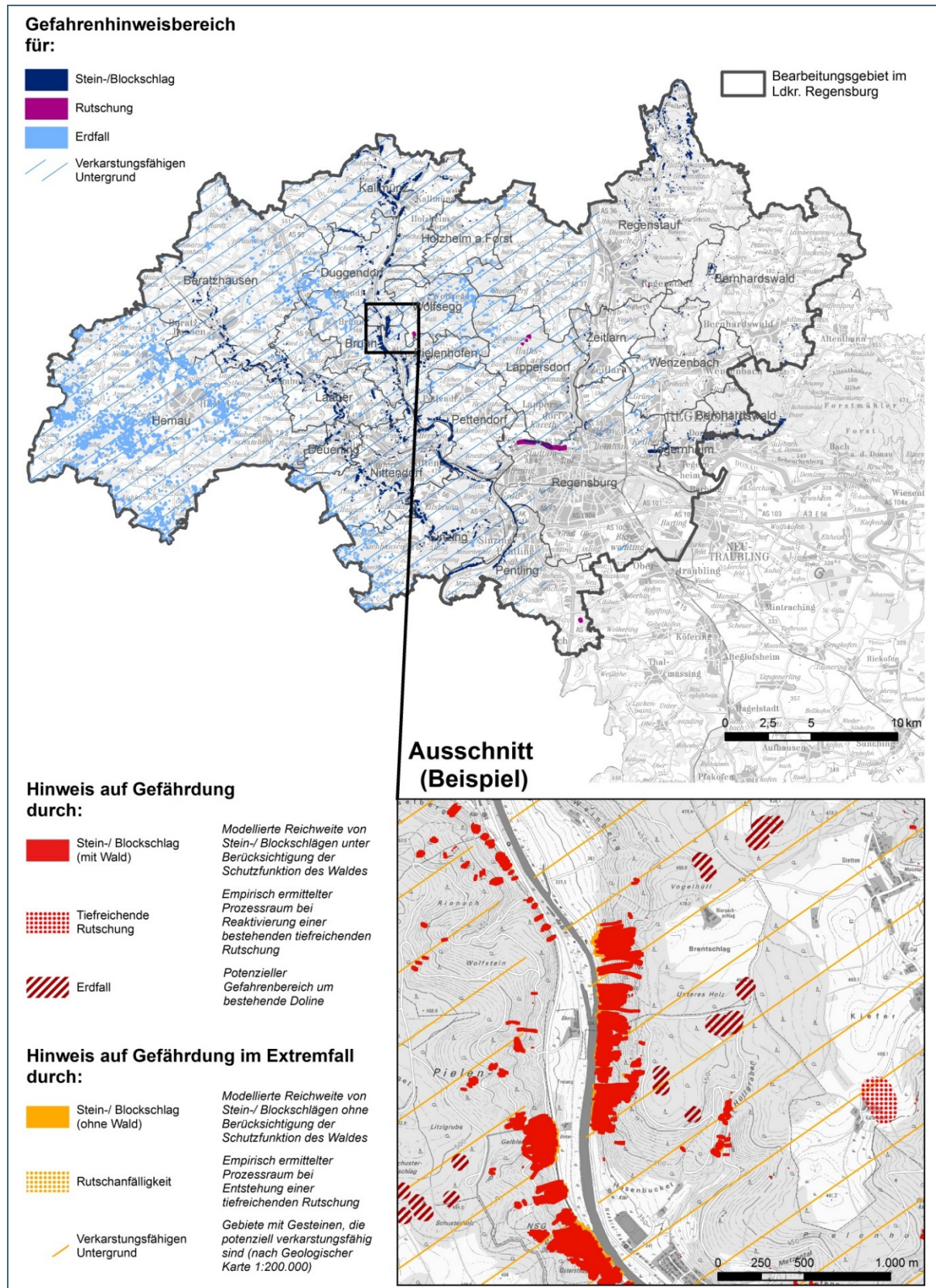
Abb. 9: Gefahrenhinweiskarte Stadt und Landkreis Regensburg
