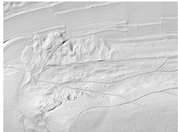
Abb. 4: Rutschung im Landkreis Eichstätt: im Schattenbild sind die Formen oft gut zu erkennen.
