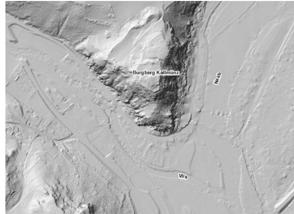
Abb. 2: Schattenbild des Burgbergs in Kallmünz oberhalb der Auen von Vils und Naab.
