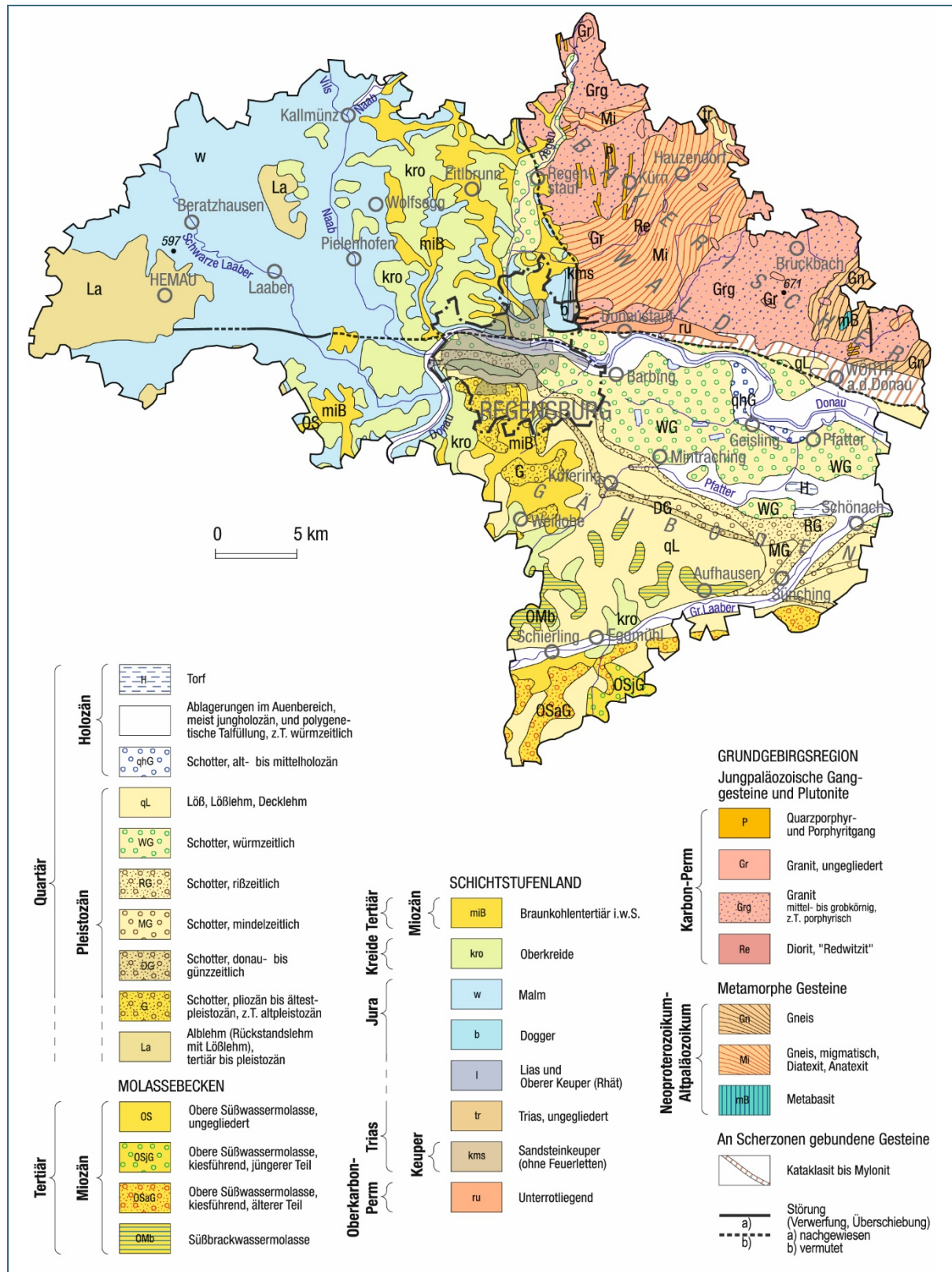
Abb. 7: Geologische Karte Stadt und Landkreis Regensburg (Datengrundlage: GK 1 : 500.000)
