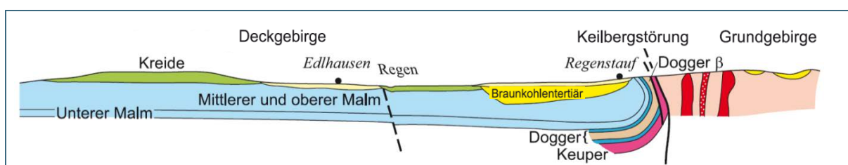
Abb. 8: West-Ost-Profilschnitt durch die Fränkische Alb im nördlichen Landkreis Regensburg (verändert nach BAUBERGER, W. & CRAMER, P. (1961): Erläuterungen zur Geologischen Karte von Bayern 1:25.000, Blatt Nr. 6838 Regenstauf.-220 S.; München)
