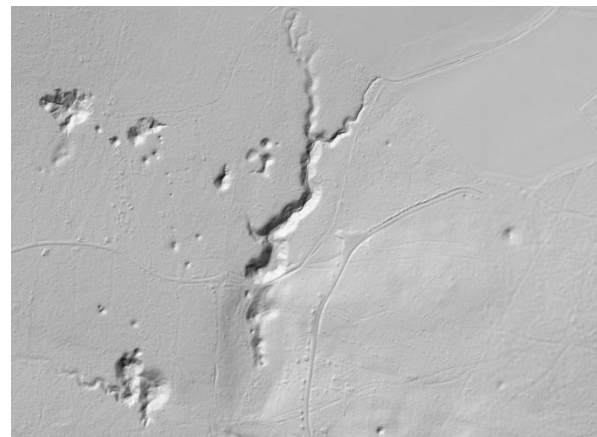
Abb. 6: Dolinenfeld südöstlich Wischenhofen im Schattenbild.
