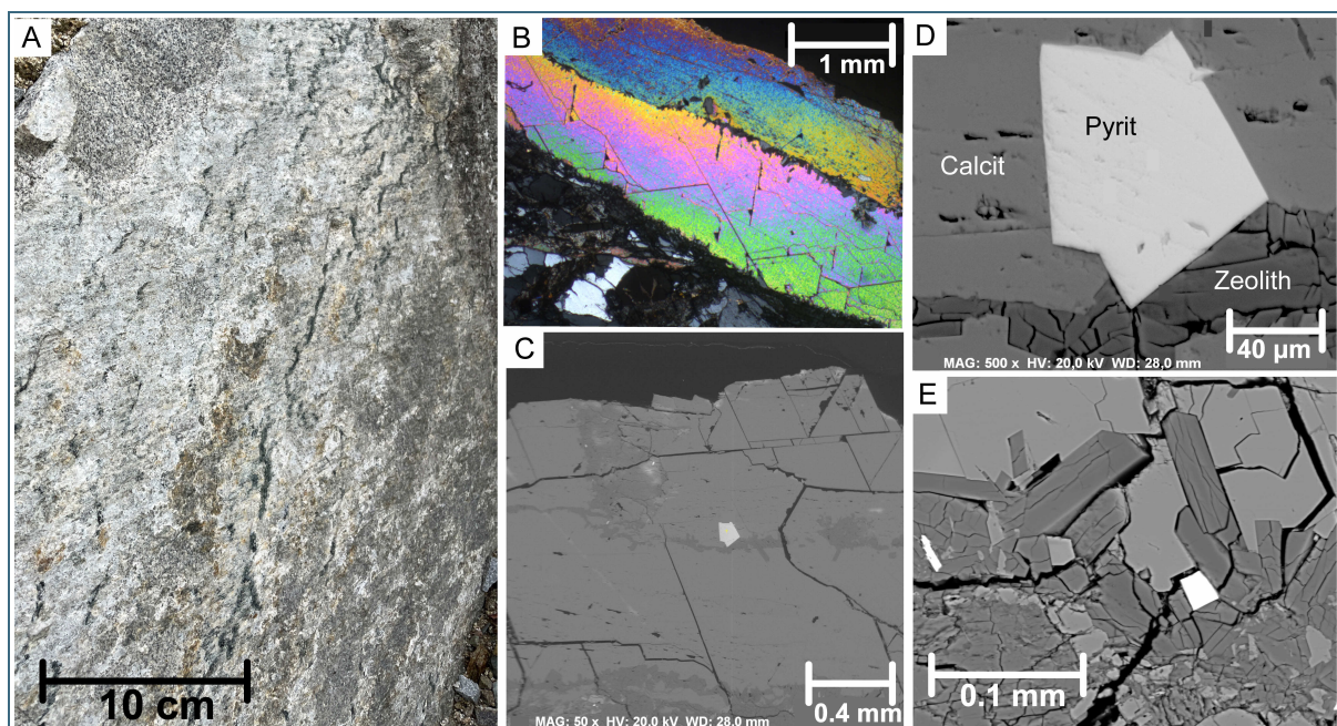
Abb. 7: Calcit im Steinbruch Hötzelsberg: A) Feldfoto von Calcit auf Störungsfläche im Steinbruch Hötzelsberg; B) Calcit-Belag auf der Störungsfläche im Dünnschliff unter gekreuzten Polarisatoren; C) BSE Bild von Calcit-Belag auf der Störungsfläche; D) Pyrit am Kontakt zwischen Zeolith und Calcit-Belag; E) BSE-Bild von Zeolith-Rasen bedeckt von Calcit.
