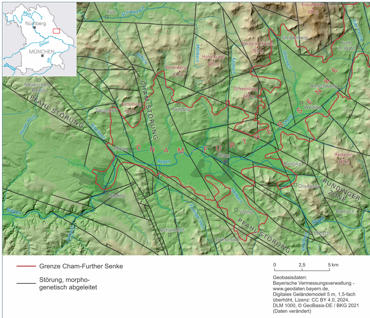
Abb. 1: Morphologisch-topographische Karte der Cham-Further Senke und ihres Umfeldes mit morphogenetisch abgeleiteten Störungen
