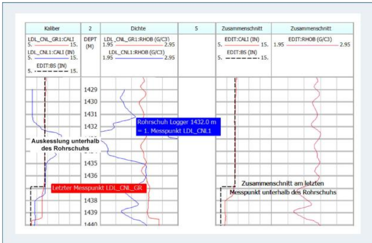
Abb. 13: Beispiel eines Zusammchnitts am Rohrschuh.
